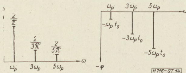
14. ábra. Szimmetrikus váltójel amplitúdó- és fázisspektruma
