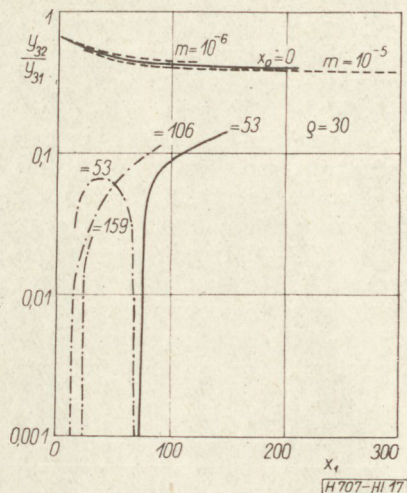
17. ábra. Az alapha vonatkoztatott második harmonikus \rho_2 = 30 esetében
