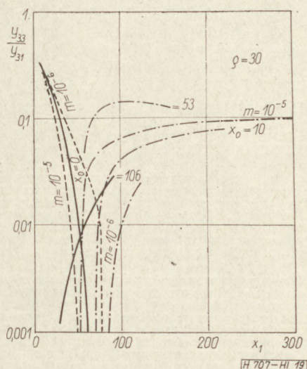
19. ábra. Az alapha vonatkoztatott harmadik harmonikus \rho_2 = 30 esetében
