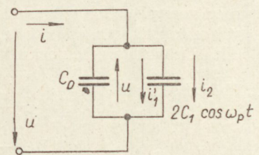
2. ábra. A kapacitáson fellépő feszültség és átfolyó áram
