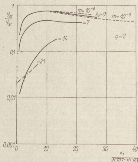
16. ábra. Az alapha vonatkoztatott második harmonikus \rho_2 = 2 esetében
