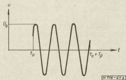
3. ábra. Elemi jel A1 üzemmódban
