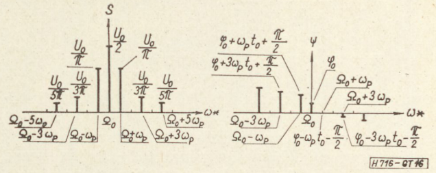
16. ábra. A1 adás amplitúdó- és fázis-spektruma szimmetrikus négysszögjellel történő moduláció esetén
