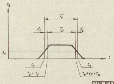
2. ábra. Elemi jel torzítás meghatározása
