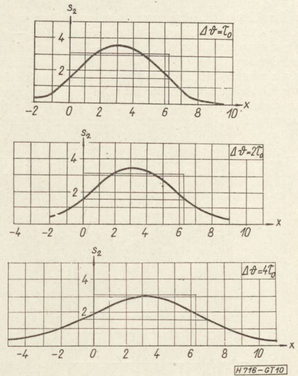
10. ábra. Vételfüggvény \frac{\Delta\omega}{2} = 2\omega_p és aszimmetrikus fázistorzítású négyszög alakú átviteli karakterisztika esetén
