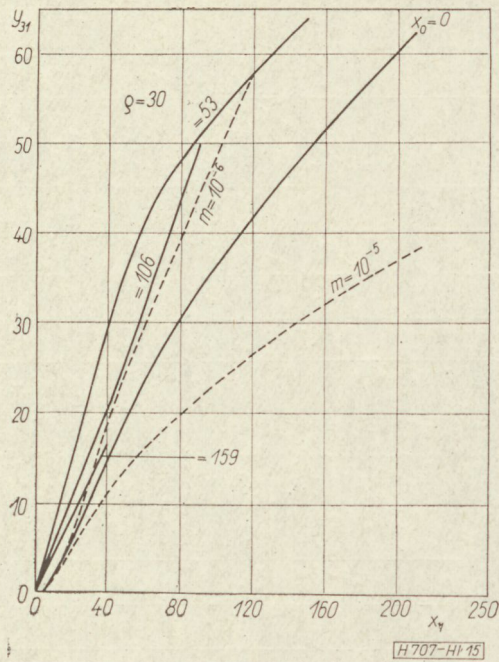
15. ábra. Az alapharmonikus normalizált értéke \varphi_2 = 30 esetében
