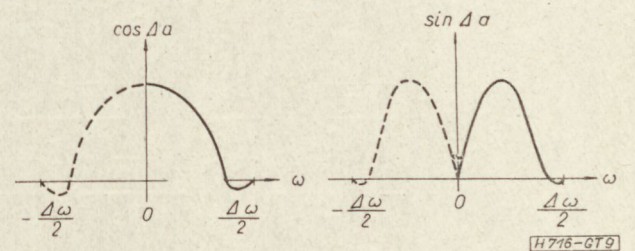
9. ábra. A vivőfrekvenciához képest szimmetrikus négyyszög alakú átviteli tényezőjű, aszimmetrikus szögtényezőjű átvitel Fourier-sorba fejtése
