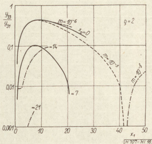
18. ábra. Az alapha vonatkoztatott harmadik harmonikus \rho_2 = 2 esetében
