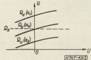
2. ábra. A feszültséggel hangolható oszcillátorok kimenő körfrekvenciájának változása a hangoló feszültség függvényében
