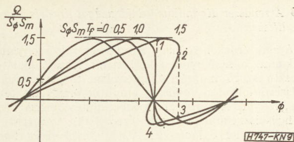
9. ábra. A szűrőnélküli APC rendszer fázisrajektóriája, ha a nagyfrekvenciás futási idő nem hanyagolható el
