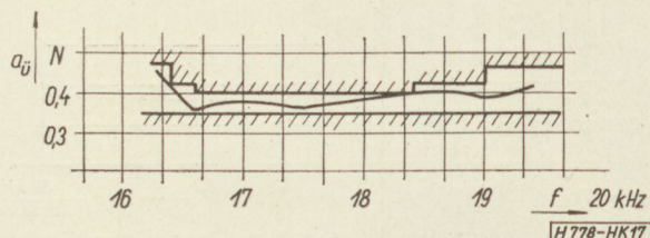
17. ábra. A megvalósított sávszűrő csillapításkarakterisztikája és toleranciái
