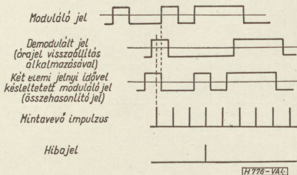
4. ábra. Hibajel előállítása távirótorzítás mentes demodulált jel esetén
