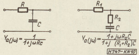
10. ábra. Az APC rendszerekben használatos aluláteresztő szűrők felépítése
