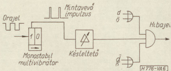
6. ábra. Hibajel előállítása ( d a demodulált jel, \bar{o} az összehasonlító jel)
