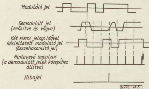
5. ábra. Hibajel előállítása távirótorzításos demodulált jel esetén
