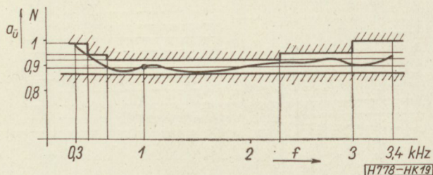
19. ábra. A megvalósított csatornamodulátor csillapításkarakterisztikája
