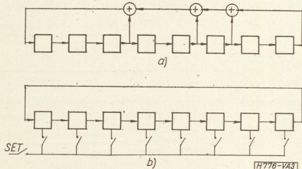
3. ábra. Jelsorozat generátor tömbvázlata (egy-egy négyzet egy-egy dinamikus vezérlésű flip-flopot jelképez; a léptető impulzus nincs ábrázolva)
