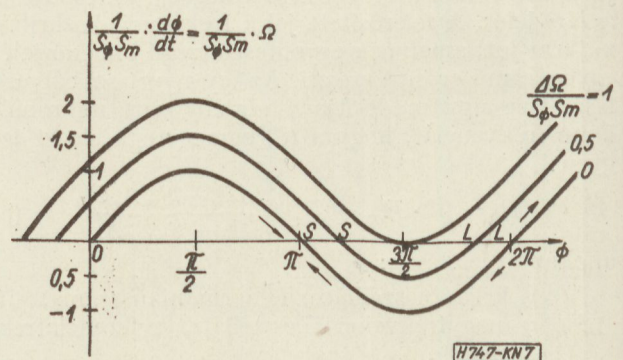
7. ábra. APC rendszer fázisrajtóriái szűrőmentes esetben
