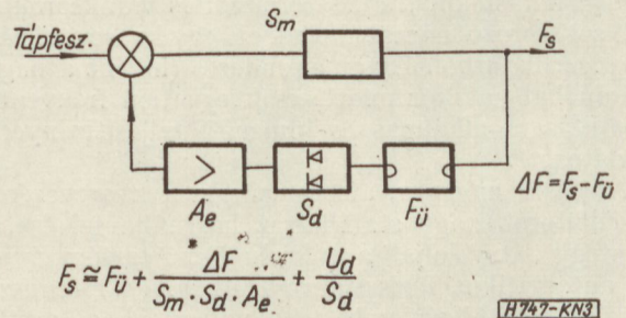
3. ábra. Kétmódusú üregrezonátort tartalmazó egyszerű frekvenciastabilizáló rendszer
