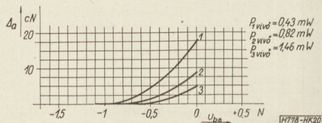
20. ábra. A csatornamodulátor csillapításának \Delta a változása a 800 Hz-es bemenő jel U_{be} feszültségének függvényében, különböző N_v vivőteljesítmény mellett
