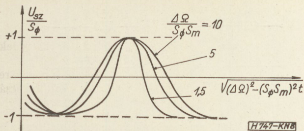
8. ábra. A szűrő nélküli APC rendszer fázisdiszkriminátorának kimenő feszültségalakja, különböző relatív elhangolódások mellett
