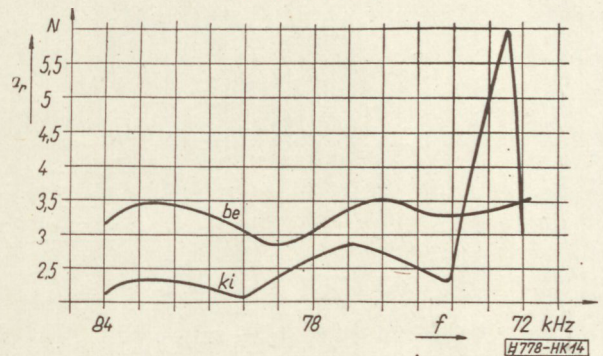
14. ábra. A megvalósított modulátor áramkör bemenő és kimenőoldali reflexiós csillapítás karakterisztikája
