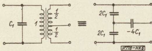
5. ábra. A 4. ábrán szereplő helyettesítő kép kiegészítése
