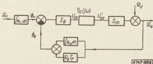
6. ábra. Fázisszabályozáson alapuló frekvenciaszabályozó körök hatásvázlata
