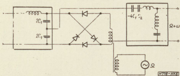
6. ábra. A szekunder oldali negatív kapacitás összevonása a sávszűrő soros kapacitásával
