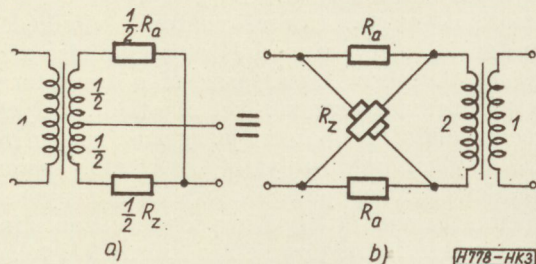
3. ábra. A levezetésnél használt áramköri equivalencia
