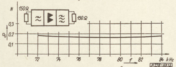
13. ábra. A megvalósított modulátor áramkör csillapításkarakterisztikája
