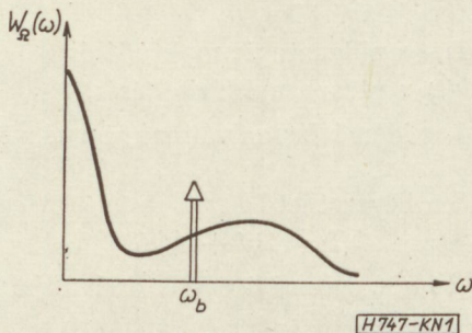
1. ábra. A mikrohullámú oszcillátorok pillanatnyi frekvenciaeltéréseinek teljesítmény spektruma
