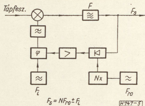
5. ábra. Fázisszabályozáson alapuló AFC rendszer felépítése
