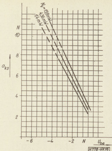
16. ábra. Az előcsoport modulátor a_{k3} harmadrendű torzítási csillapítása a 18 kHz-es bemenő jel U_{be} feszültségének függvényében, különböző N_v vivőteljesítmény mellett
