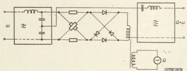
8. ábra. A modulátor alapszűrésének megnövelése beiktatott X csillapító taggal
