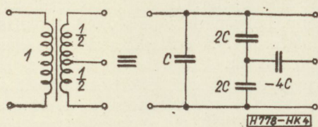
4. ábra. Középleágazású ideális transzformátor kapacitív helyettesítő képe (Hibaigazítás: a C kondenzátor negatív)
