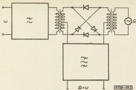
2. ábra. Gyűrűs modulátor soros vivőtáplálása
