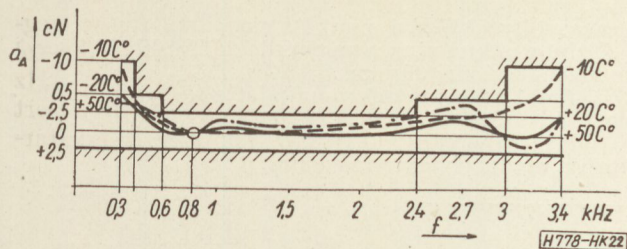
22. ábra. A modulátor csillapításkarakterisztikája különböző hőmérsékleteken
