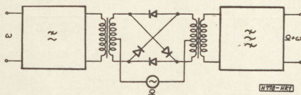
1. ábra. Gyűrűs modulátor párhuzamos vivőtáplálása
