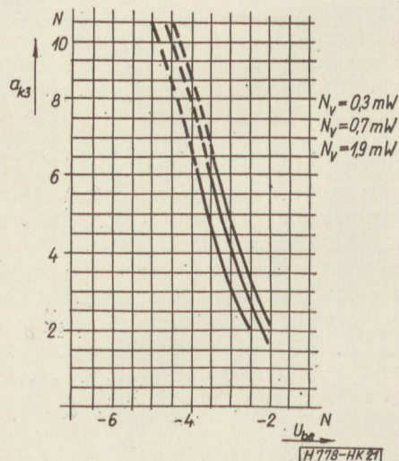
21. ábra. A csatornamodulátor a_{k3} harmadrendű torzítási csillapítása a 800 Hz-es bemenő jel U_{be} feszültségének függvényében, különböző N_v vivőteljesítmény mellett
