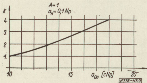
9. ábra. Az ütközési csillapítás a K függvényében
