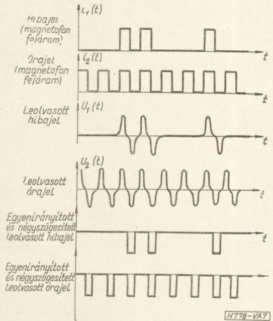
7. ábra. Hibajel rögzítése magnetofon szalagra
