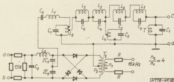
18. ábra. Szűrőkkel egybeépített csatornamodulátor elvi kapcsolása
