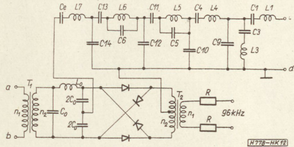
12. ábra. Szűrőkkel egybeépített előcsoport modulátor elvi kapcsolása
