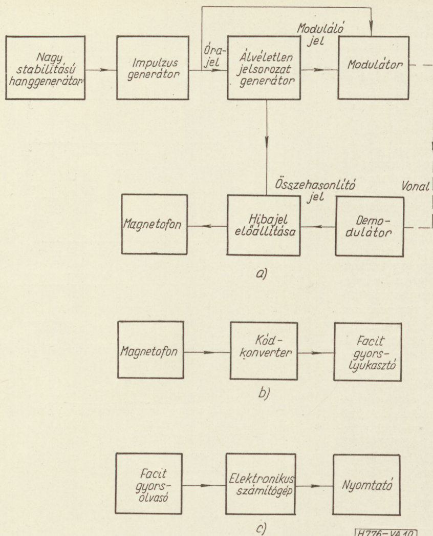
10. ábra. Statisztikus hibavizsgálat elvégzésének lépései: a) mérés; b) lyukasztás; c) kiértékelés
