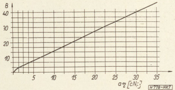
7. ábra. Az a_\eta többletszűrés csillapítás a B sávzélességi tényező függvényében
