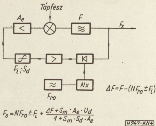
4. ábra. Szuperheterodin elven működő AFC rendszer felépítése
