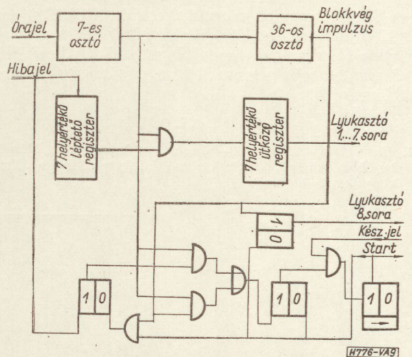
9. ábra. Kódkonverter magnetofonszalagról lyukszalagra
