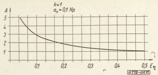
11. ábra. Az \eta -érkenységi tényező változása az A illetlenség függvényében, rögzített K és a_n mellett
