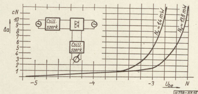
15. ábra. Az előcsoport modulátor csillapításának \Delta a változása a 18 kHz-es bemenő jel U_{be} feszültségének függvényében, különböző N_v vivőteljesítmény mellett
