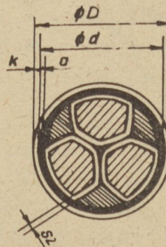
2. ábra. Ívelt ötszögszelvényű vezetőjű ALPLAST 0,6/1 kV kábelek szerkezeti felépítése
