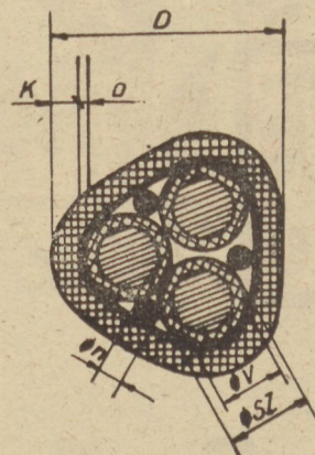
1. ábra. Tömör körszelvényű vezetőjű ALPLAST 0,6/1 kV kábelek szerkezeti felépítése
