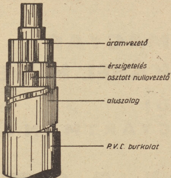
1. ábra. Tömör körszelvényű vezetőjű ALPLAST 0,6/1 kV kábelek szerkezeti felépítése
