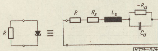
4. ábra. Ellenállással lezárt tunneldiódás áramkör és helyettesítő kapcsolása
