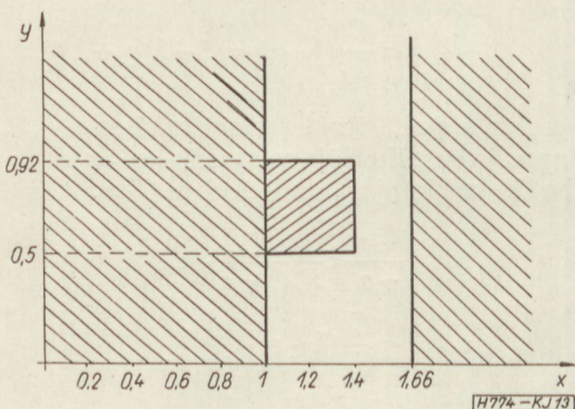
13. ábra. A három üzemmód közelítő határai az xy síkon
