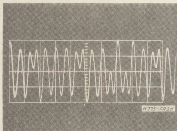
3d. ábra. A sávhatárolt modulált vivő
