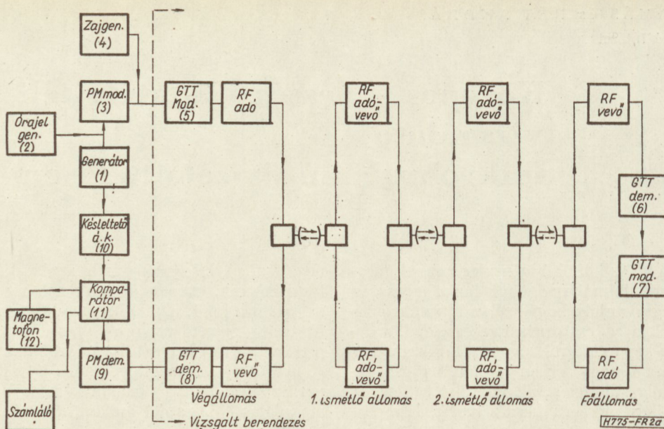
2a. ábra. Mérési elrendezés
