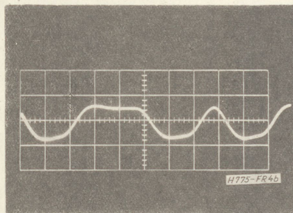
4b. ábra. A demodulált adatjel szűrés után
