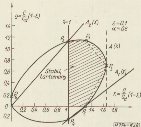
8. ábra. Normalizált Routh-stabilitás-diagram: \varepsilon = 0,1 ; \alpha = 0,8
