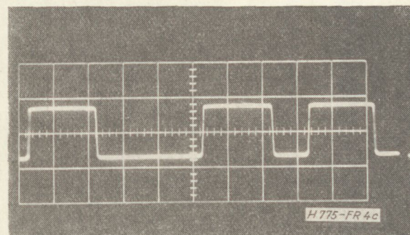
4c. ábra. A demodulált adatjel négyzetösítés után
