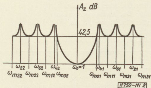
2. ábra. Sávszűrő csillapításkarakterisztikája
