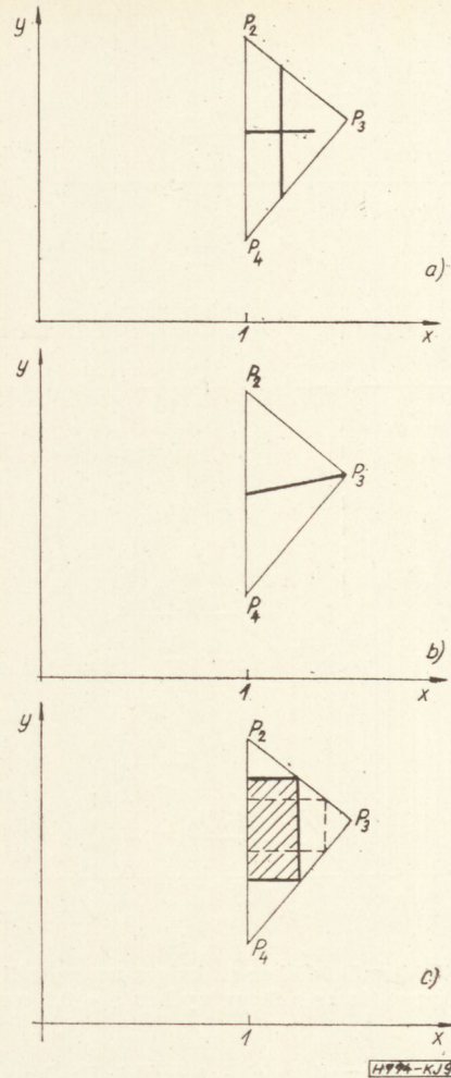
9. ábra. Stabil tartomány közelítése a súlyponton átmenő egyenesekkel és maximális területű téglalappal \alpha > 1 esetén
