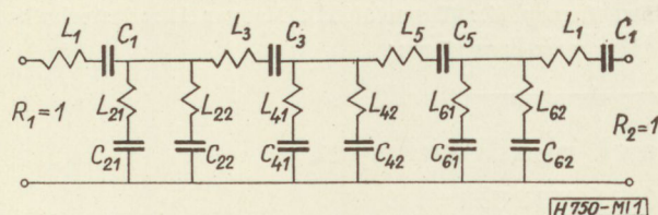
1. ábra. Inverz Csebishev sávszűrő
