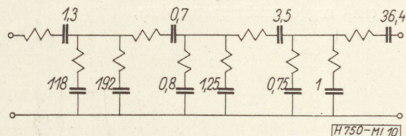
10. ábra. A sávszűrő elemeinek %-os tűréshatárai
