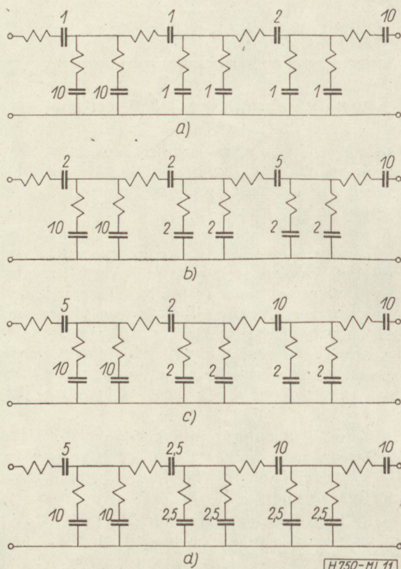
11. ábra. A sávszűrő kondenzátorainak %-os tűrőhatárai. Az elemek mellé írt számok a névleges értéktől való eltérést %-ban jelentik ( f_1 ).
