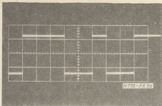
3a. ábra. Az adatjel szűrés előtt
