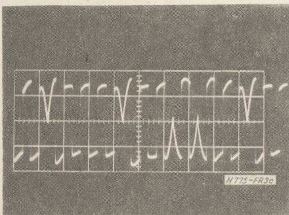
3c. ábra. Az adatjellel modulált vivő
