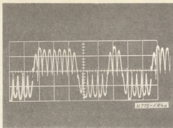
4a. ábra. A demodulált adatjel szűrés előtt
