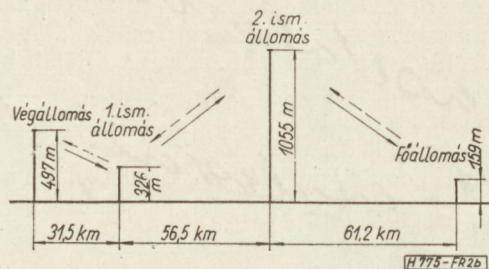
2b. ábra. Állomás távolságok és magasságok
