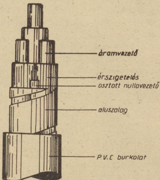
2. ábra. Ívelt ötszögszelvényű vezetőjű ALPLAST 0,6/1 kV kábelek szerkezeti felépítése
