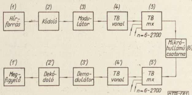
1. ábra. Az adat útja előfizetőtől előfizetőig
