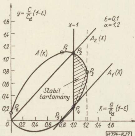
7. ábra. Normalizált Routh-stabilitás-diagram: \varepsilon = 0,1 ; \alpha = 1,2
