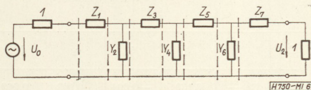
6. ábra. Az aluláteresztő, mint négypólusok láncbakapcsolása
