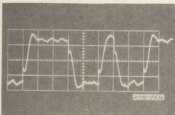
3b. ábra. Az adatjel szűrés után
