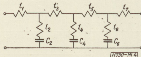
4. ábra. Sávszűrő aluláteresztő ekvivalense
