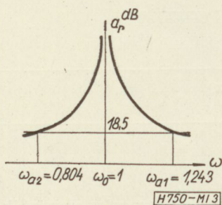
3. ábra. Sávszűrő reflexiós csillapításkarakterisztikája
