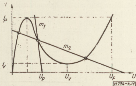
1. ábra. Tunneldióda statikus karakterisztikája. U_p a max I_p -hez tartozó feszültség
