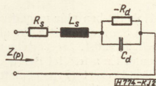
2. ábra. Tunneldióda helyettesítő kapcsolása
