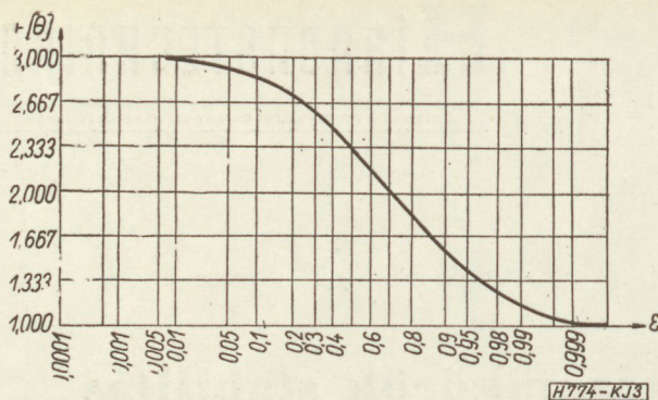
3. ábra. Diagram a feltételes stabilitás megállapításához
