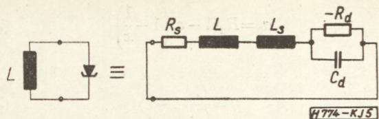
5. ábra. Induktivitással lezárt tunneldiódás áramkör és helyettesítő kapcsolása
