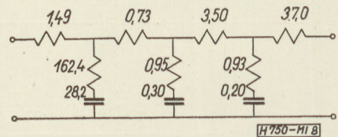
8. ábra. Az aluláteresztő elemeinek %-os tűréshatárai
