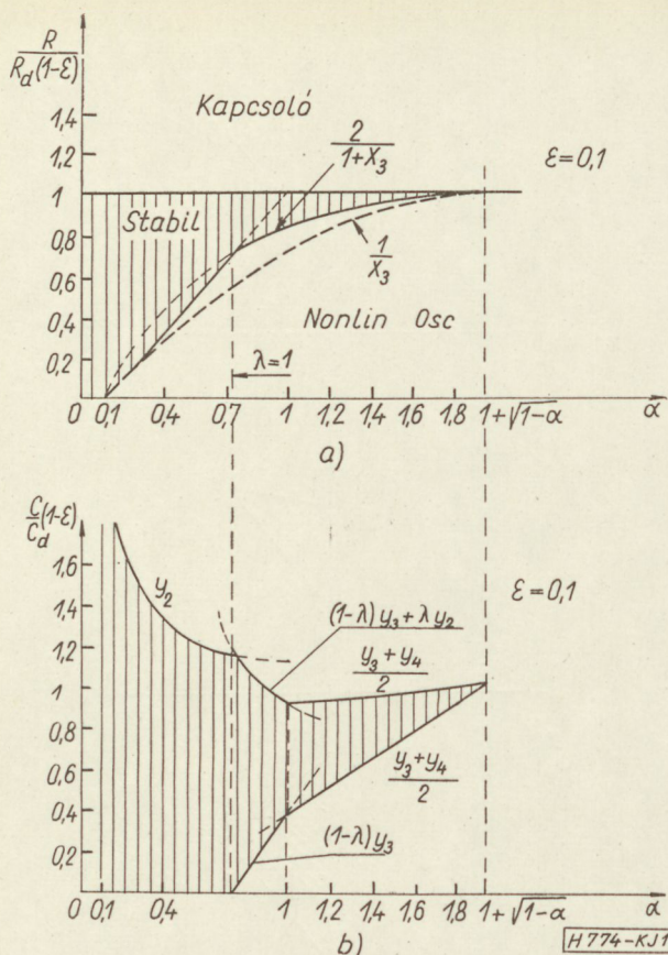
11. ábra. Stabil működéshez szükséges normalizált ellenállás és kapacitás az \alpha függvényében \varepsilon = 0,1 esetén
