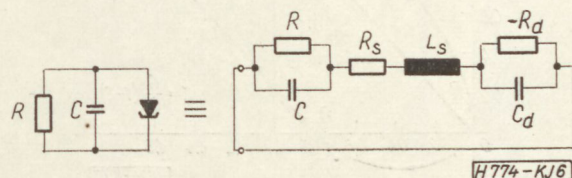
6. ábra. Ellenállással és kapacitással lezárt tunneldiódás áramkör és helyettesítő kapcsolása
