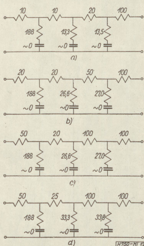
12. ábra. Az aluláteresztő kondenzátorainak %-os tűrőhatárai. Az elemek mellé írt számok a névleges értéktől való eltérést %-ban jelentik ( f_1 ).
