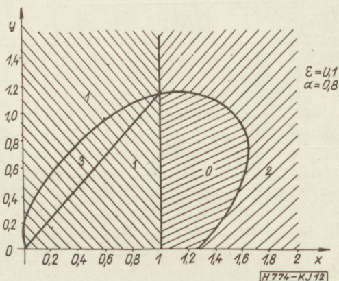
12. ábra. A három üzemmód határai az xy síkon
