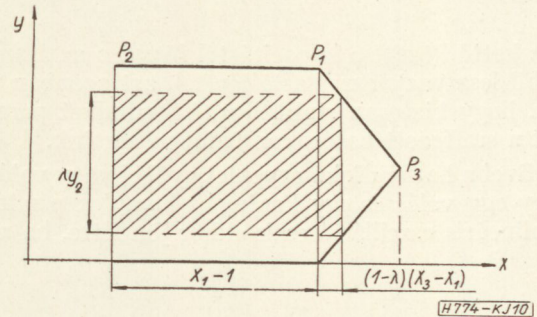
10. ábra. Stabil tartomány közelítése maximális területű téglalappal \alpha < 1 esetén
