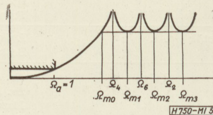
5. ábra. Aluláteresztő csillapításkarakterisztikája
