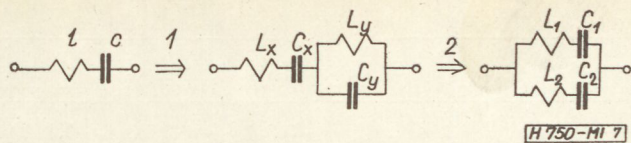
7. ábra. Aluláteresztő sávszűrő transzformáció és ekvivalens átalakítás
