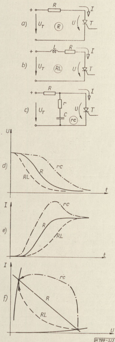
3. ábra. A tirisztor terhelési viszonyai
