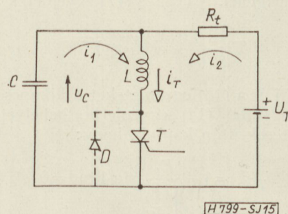
15. ábra. Rezgőkörös kikapcsolóáramkör
