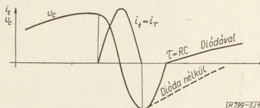
19. ábra. Az i_t , u_c időfüggvénye
