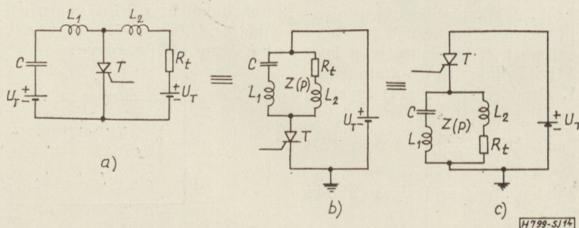
14. ábra. A 10. ábra kapcsolásának ekvivalensei
