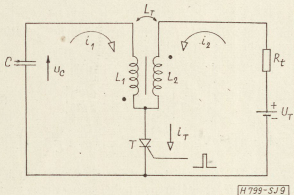
9. ábra. Csatoltkörös kikapcsolóáramkör
