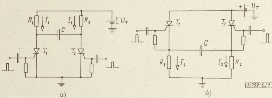
7. ábra. Tirisztoros flip-flop áramkör
