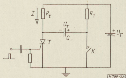
6. ábra. A tirisztor kikapcsolása a K kapcsoló zárásával
