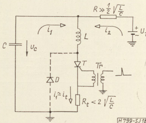
18. ábra. A terhelésre félszínusz áramot adó generátor
