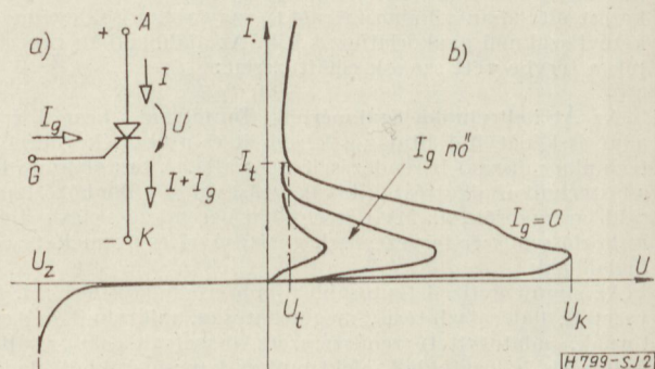
2. ábra. A tirisztor jelölése és karakterisztikája
