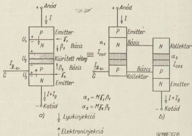
1. ábra. A tirisztor felépítése és helyettesítése
