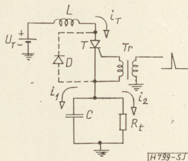
17. ábra. A 15. ábra ekvivalens áramköre
