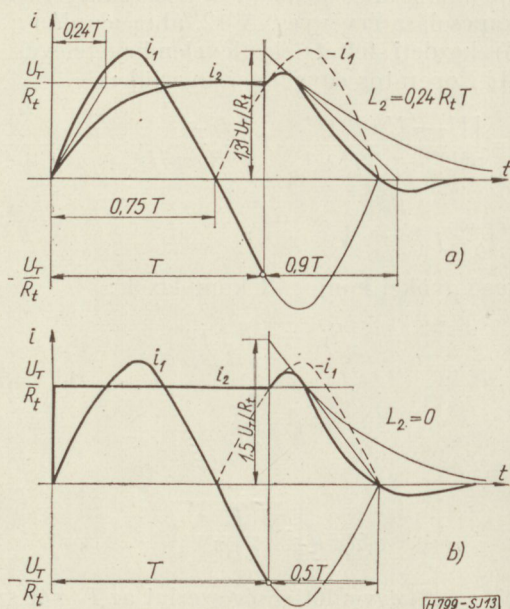
13. ábra. Az i_2 áram időfüggvénye
