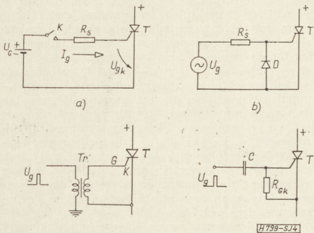
4. ábra. Tirisztorok bekapszolása
