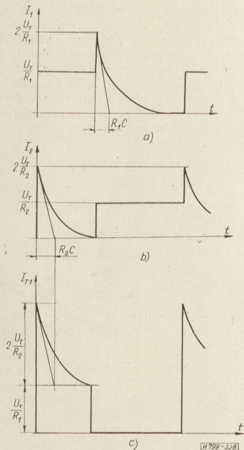
8. ábra. Az R_1 , R_2 terhelésen és a T_1 tirisztoron átfolyó áram
