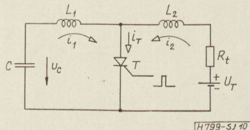
10. ábra. Rezgőkörös kikapcsolóáramkör
