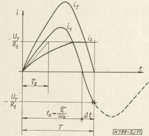
11. ábra. A rezgőkörön és a terhelésen folyó áram a tirisztor vezetési állapotában
