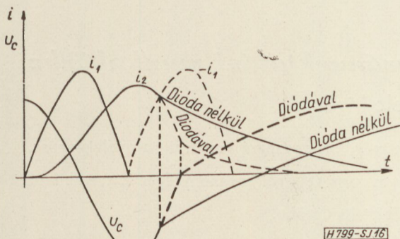
16. ábra. Az i_1 , i_2 , u_c időfüggvények
