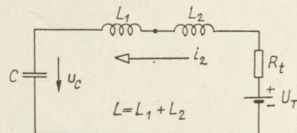
12. ábra. Működés a tirisztor kikapcsolása után
