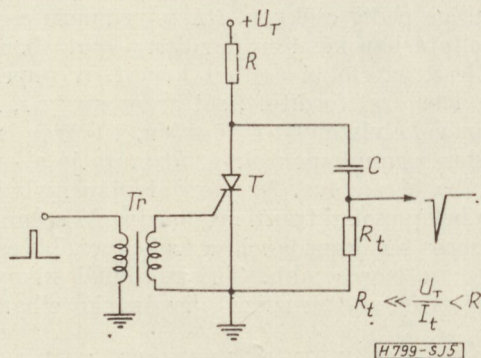
5. ábra. Impulzusgenerátor
