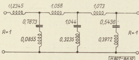
10. ábra. Hatodfokú, inverz-Csebisev karakterisztikájú aluláteresztő szűrő
