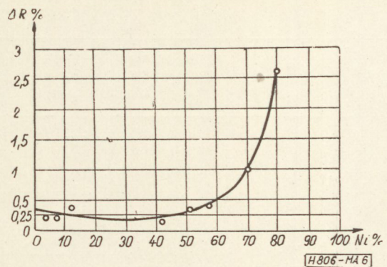
6. ábra. Lakkkal burkolt NiCr rétegek ellenállásváltozása 10 napos, 40 C°-os, 96% rel. nedvességtű térben való tárolás után, az összetétel függvényében
