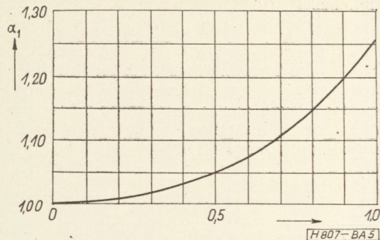
5. ábra. Az \alpha_1 paraméter b függvényében
