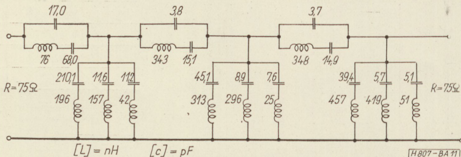
11. ábra. A számpélda előírásainak megfelelő szimmetrikus sávszűrő
