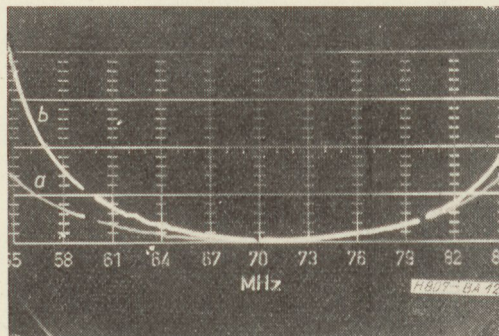
12. ábra. A sávszűrő mért futási idő karakterisztikája a) a példa szerinti szimmetrikus sávszűrő esetében, b) a 10. ábra aluláteresztő szűrőjéből szokásos transzformációval nyert sávszűrő esetében. A függőleges tengelyen egy kis osztás 2 ns-nak felel meg
