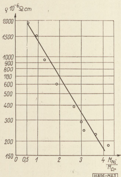
3. ábra. A fajlagos ellenállás a Ni/Cr mólarány függvényében, logaritmikusan lejtékben
