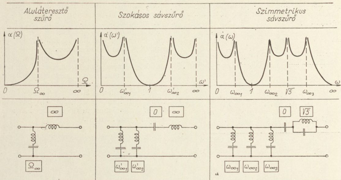
7. ábra. A szokásos és a szimmetrikus sávszűrő struktúrája
