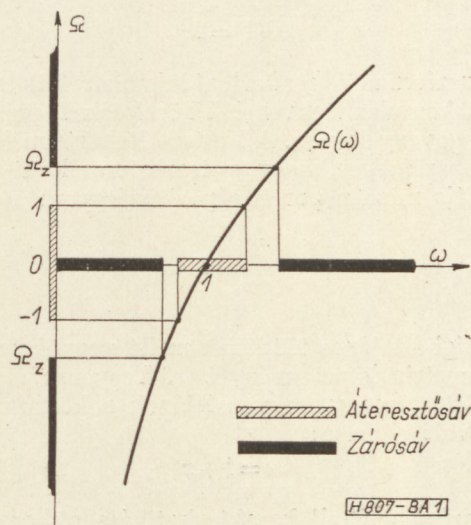
1. ábra. A szokásos aluláteresztő-sáváteresztő transzformáció
