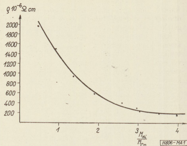
1. ábra. A réteg fajlagos ellenállása a Ni/Cr molarány függvényében
