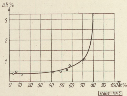
5. ábra. Lakkozatlan NiCr rétegek ellenállásváltozása 10 napos, 40 C°-os, 96% rel. nedvességtű térben való tárolás után, az összetétel függvényében
