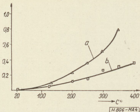
4. ábra. Ellenállásváltozás levegőn (a), ill. 5 \cdot 10^{-3} Hgmm vákuumban (b) a hőkezelés hőmérsékletének függvényében
