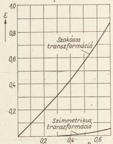
9. ábra. Az aszimmetriára jellemző \varepsilon paraméter b függvényében
