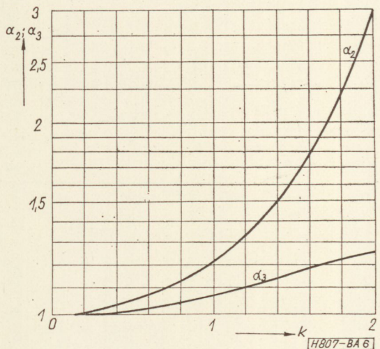
6. ábra. Az \alpha_2 és \alpha_3 paraméterek k függvényében
