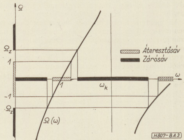
3. ábra. Harmadfokú aluláteresztő-sáváteresztő transzformáció
