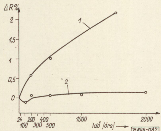
7. ábra. Az ellenállásérték változása raktározás során, az idő függvényében. 1 — lakkozatlan; 2 — lakkozott
