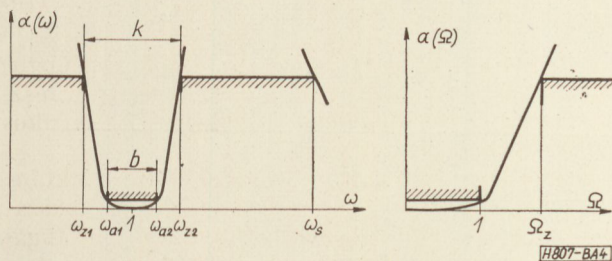
4. ábra. A csillapításkarakterisztika tolerancia-sémája, a) a szimmetrikus sávszűrőnél, b) az aluláteresztő szűrőnél
