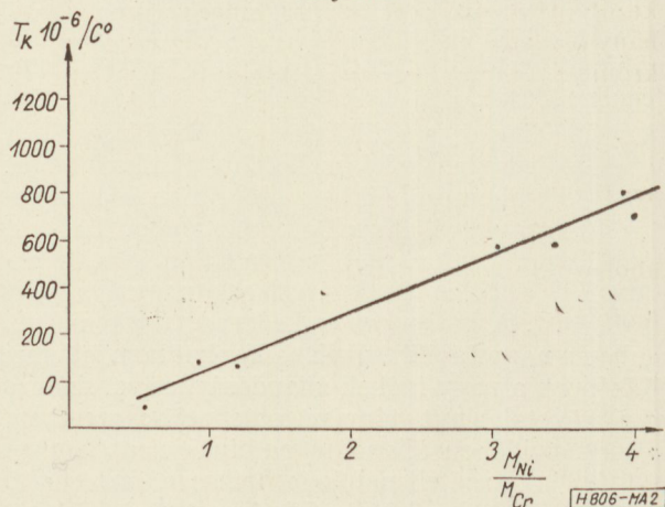
2. ábra. A réteg hőmérsékleti együtthatója a Ni/Cr molarány függvényében
