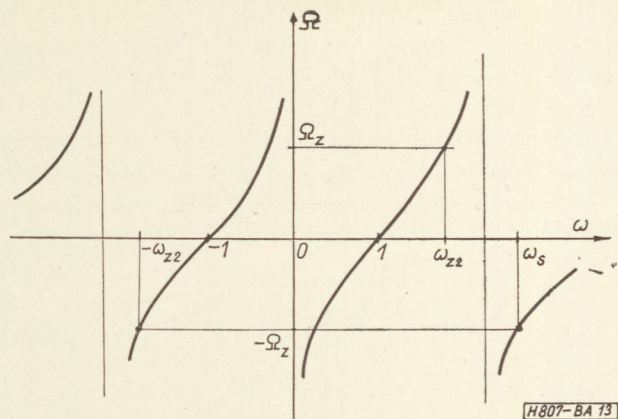
13. ábra. Ábra az \omega_s frekvencia számításához
