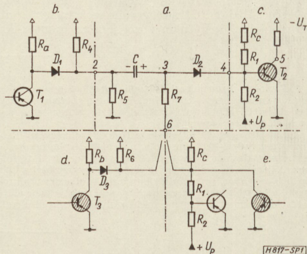
1. ábra. Az impulzuskapu és a hozzá kapcsolódó áramkörök. a) impulzuskapu; b) vezérlő áramkör; c) impulzust érzékelő áramkör; d), e), kapu nyitását, illetve lezárását végző áramkörök. Vagy d, vagy e csatlakozik a 6 ponthoz
