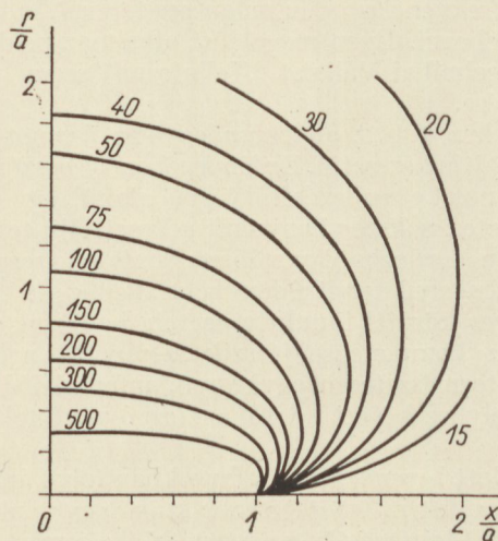
3. ábra. 10^3 \frac{H}{I/a} értéke a relatív távolságok függvényében
