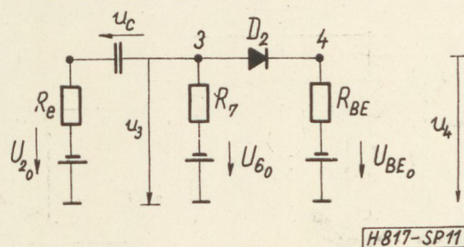
11. ábra. Az impulzuskapu helyettesítő képe impulzusadás végén
