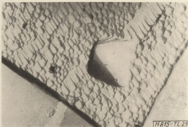
29. ábra. 0,1% Ca-iont tartalmazó Mn-Zn-ferrit törete
