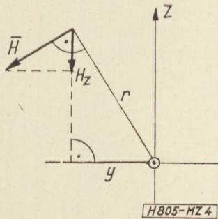
4. ábra. A térerősség vertikális komponensének számítása
