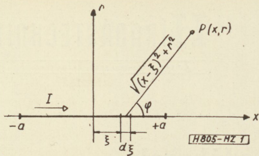
1. ábra. Koordináta-rendszer egyenes vezető terének számításához
