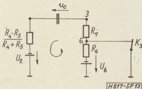
13. ábra. Az impulzuskapú helyettesítő képe a kapu vezérlése esetén
