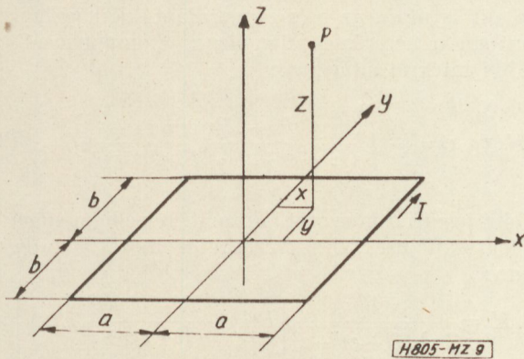
9. ábra. Téglalap alakú hurok
