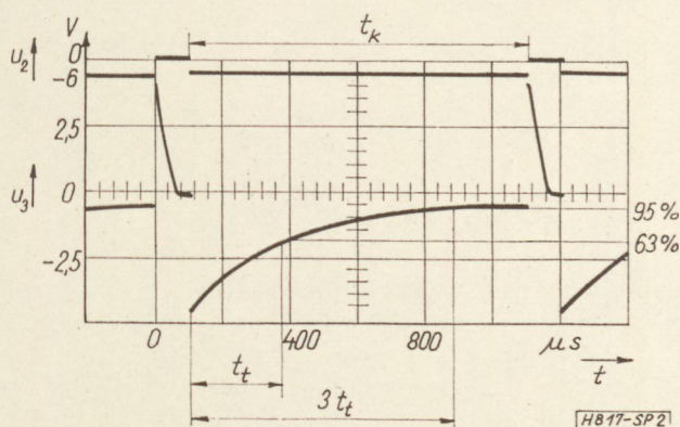
2. ábra. Az impulzuskapu feszültséggörbéi impulzusadás esetén. Az 1. ábra 2 pontjára adott impulzusok hatására a 3, 4 és 5 pontokon megjelenő feszültséggörbék. Kapcsolási idők definíciói
