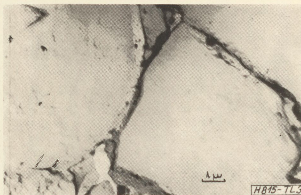
30. ábra. 0,25% Ca- és 0,25% Si-iont tartalmazó Mn-Zn-ferrit törete
