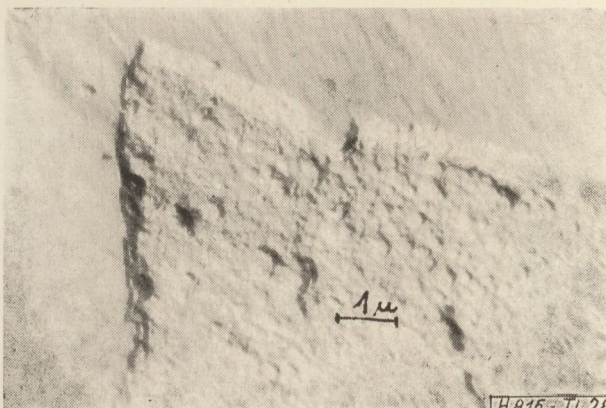
28. ábra. Szennyező anyag nélküli Mn-Zn-ferrit törete
