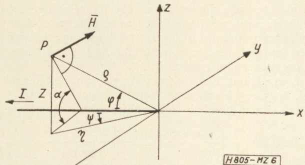
6. ábra. Koordináta-rendszer a vezető végpontjának közelében a vertikális térerősségkomponens számításához
