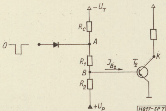
7. ábra. A logikai fordító vezérlése sztatikus bemenetről
