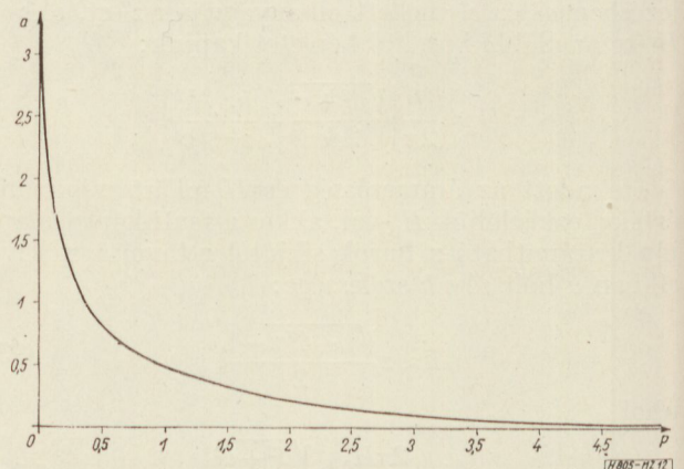
12. ábra. H_z minimális értéke kör alakú hurok esetén
