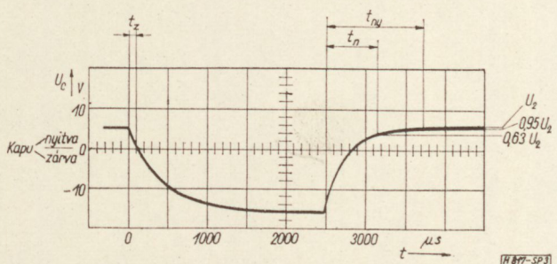
3. ábra. A C kondenzátor feszültséggörbéje a kapu vezérlése esetén. Kapcsolási idők definíciói
