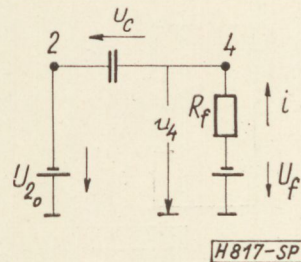
10. ábra. Az impulzuskapu helyettesítő képe impulzusadás alatt
