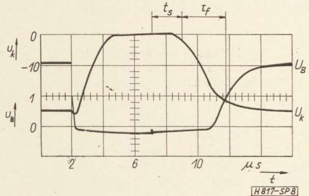
8. ábra. A logikai fordító feszültséggörbéi sztatikus vezérlés esetén
