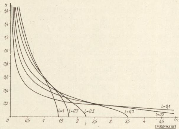
10. ábra. H_z minimális értéke téglalap alakú hurok esetén
