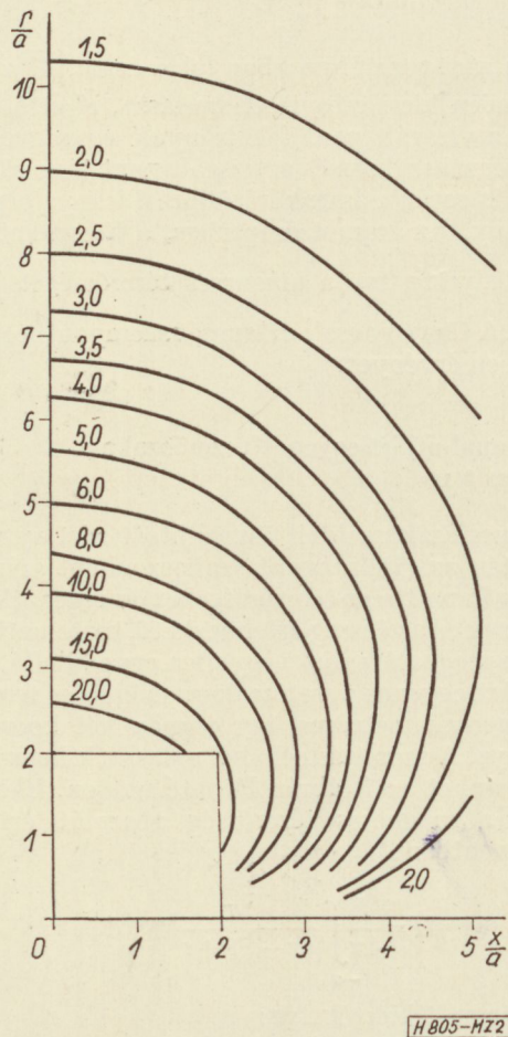
2. ábra. 10^3 \frac{H}{I/a} értéke a relatív távolságok függvényében
