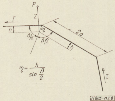
8. ábra. Holt sáv a töréspont környezetében
