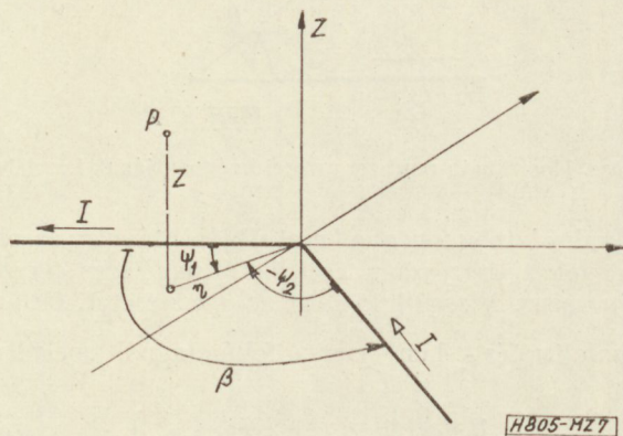
7. ábra. A töréspont környezete
