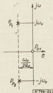
3. ábra. Párhuzamos veszteségű, párhuzamos rezgőkörös csatolófokozat pólus-zérus elrendezése
