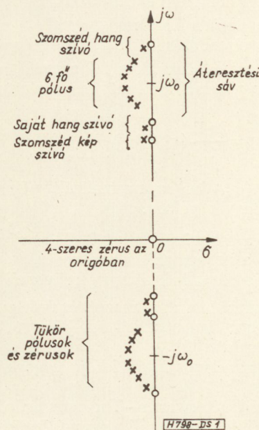
1. ábra. Televízió-vevőkészülék video KF erősítőjének pólus-zérus elrendezése
