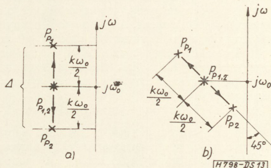
13. ábra. A pólusok helyének változása a visszacsatolás következtében
