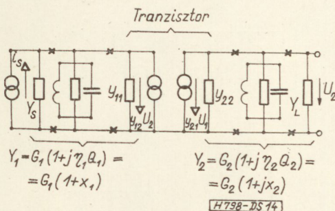
14. ábra. Erősítőfokozat helyettesítő képe
