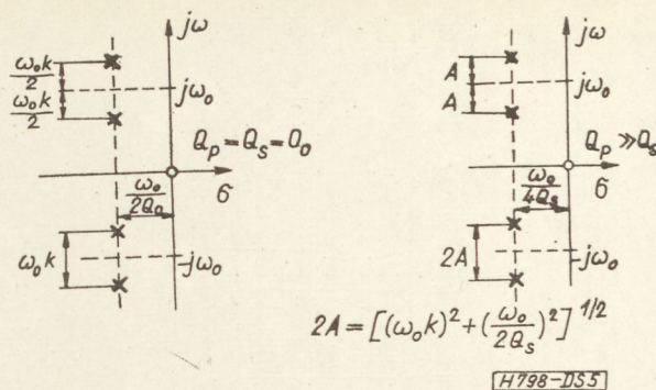
5. ábra. Két-hangoltkörös csatolóáramkörök pólus-zérus elrendezése azonos és erősen különböző jósági tényezők esetén
