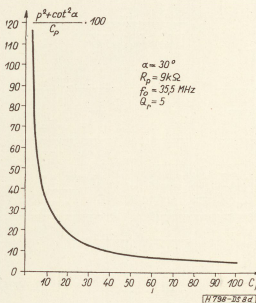
8. ábra. A \frac{p^2 + \cot^2 \alpha}{C_p} függvény menete a) \alpha = 80^\circ ; b) \alpha = 70^\circ ; c) \alpha = 60^\circ ; d) \alpha = 30^\circ
