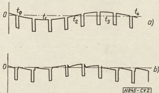
2. ábra. A clamper fokozat hatása a szuperponált zavarójelekre a) szinkronjelek szuperponált zavarójelekkel, b) az a) alatti jel clamping után. Láthatóan a hátsó kioltások azonos szintre kerültek, és a zavarójelek csökkent
