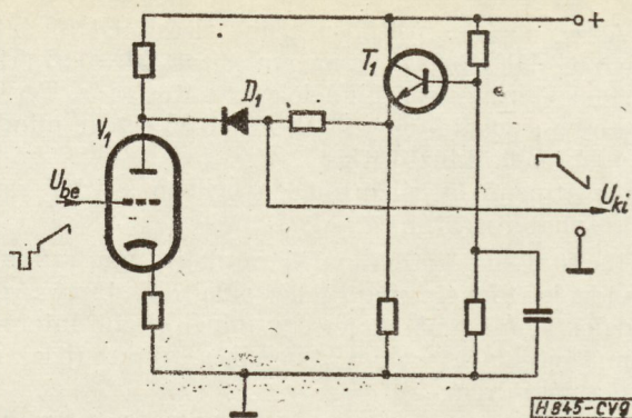
9. ábra. Ténylegesen megvalósított vágóáramkör
