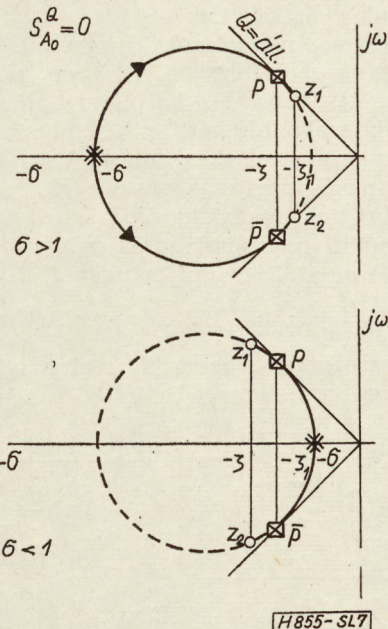
7. ábra. Gyökhelygörbe Q -ra vonatkozó zérus érzékenység esetén
