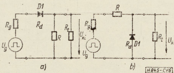
6. ábra. a) Soros vágó, b) párhuzamos vágó
