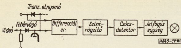
14. ábra. A fehérszint-túllépéssjelző áramkör tömbvázlata
