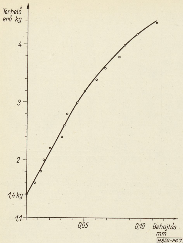
8. ábra. Terhelőerő-behajlás diagram 20 °C hőmérsékleten
