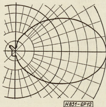
12. ábra. A 8. ábra paneljének horizontális sugárzási karakterisztikája, \varnothing 80 mm-es árbocon nézve
