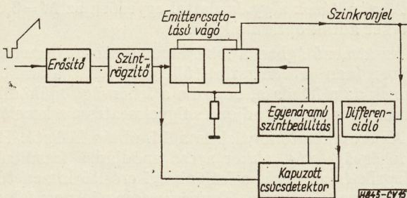
15. ábra. A szinkronjel közepét vágó áramkör tömbvázlata
