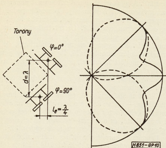
10. ábra. Fázistolt táplálású kórsugárzó antennarendszer és sugárzási karakterisztikája (egynegyed szektor)
