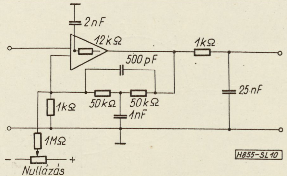
10. ábra. Erősítő, másodfokú, maximális laposságú frekvencia menettel. f_H=4,5 kHz. Erősítés: 100. A pólusérzékenység abszolút értéke minimalizálva
