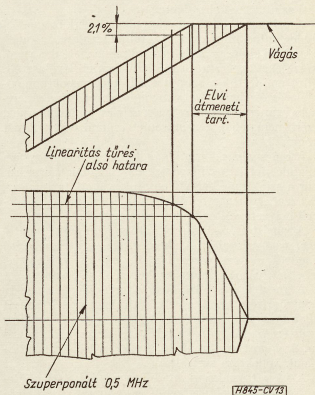
13. ábra. A fehérvágó linearitásának mérése
