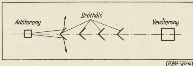
14. ábra. Földreflexió-csökkentő dróthálók elhelyezése
