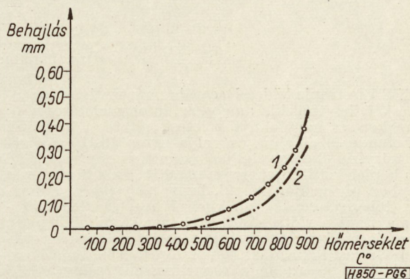
6. ábra. Összehasonlító hőmérsékletbehajlás diagram ugyanazon 1,3 mm átmérőjű molibdénhuzalból készült próbatesten 4 órás felfűtés esetén (1), 15 perces felfűtés esetén (2)
