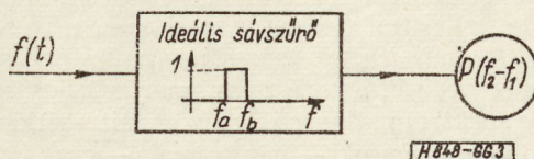
3. ábra. P(f_2 - f_1) \equiv P(f_b - f_a)
