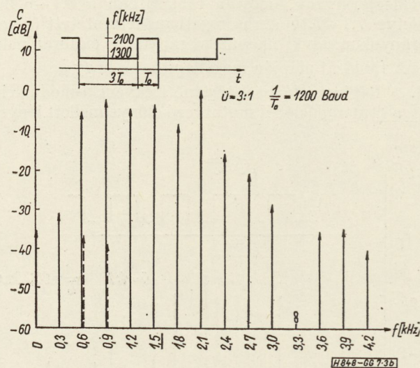
7.3a ábra. 1200 Baud-os periodikus adatjellel modulált folytonos fázisú FM-jel spektruma
