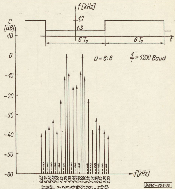
6.3e ábra. 600 Baud-os periodikus adatjellel modulált folytonos fázisú FM-jel spektruma
