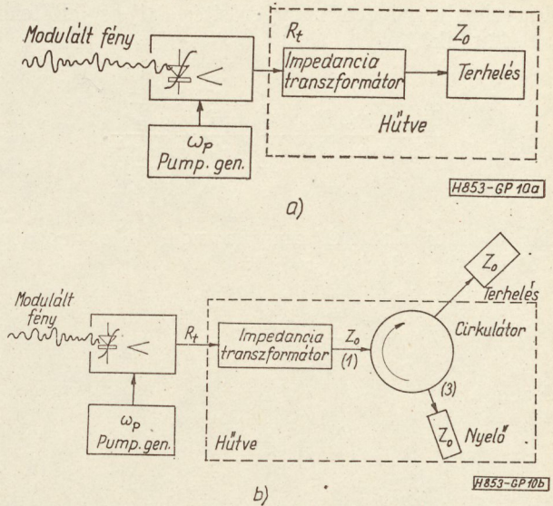
10. ábra. A fotoparametrikus erősítő és a terhelés összekapcsolása
