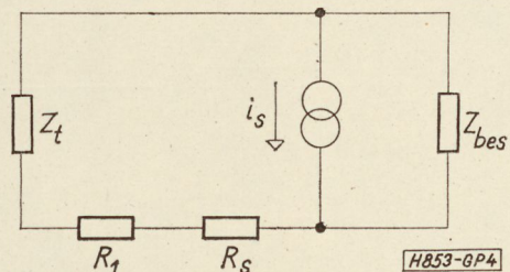
4. ábra. Helyettesítő kép P_s(\gamma) számításához
