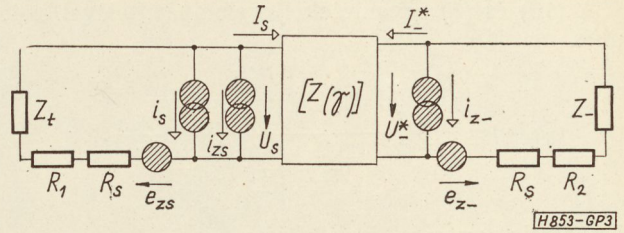
3. ábra. Fotoparametrikus erősítő helyettesítő képe
