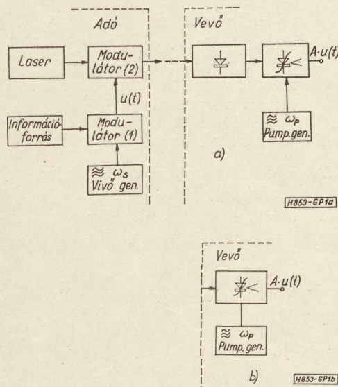
1. ábra. Információátvitel intenzitásmodulált laser-sugárral
