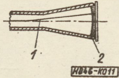
11. ábra. Szállemez alkalmazása katódsugárcsőben. 1 elektron-sugár, 2 fénypor, szállemez, fényképlemez
