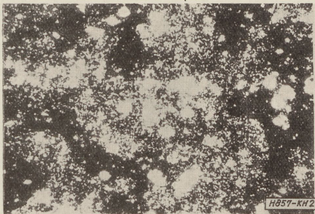
2. ábra. 2 jelzésű elektrolitkondenzátor-sorozat záróréteg-elektrolit határfelületéről készített fénymikroszkópos felvétel alapállapotban (90×)
