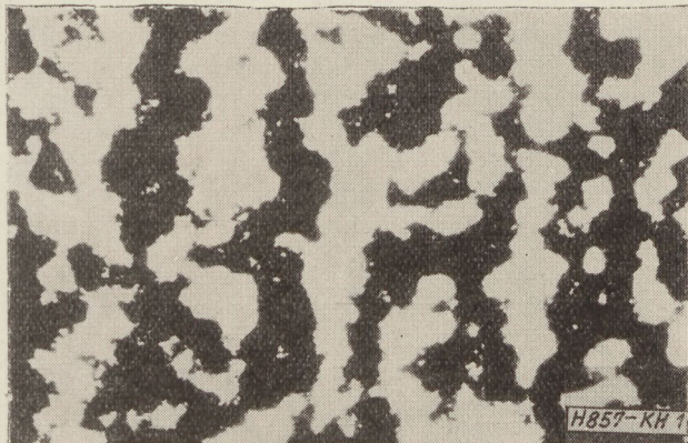
1. ábra. 1 jelzésű elektrolitkondenzátor-sorozat záróréteg-elektrolit határfelületéről készített fénymikroszkópos felvétel alapállapotban (90×)
