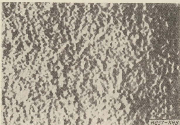
8. ábra. 10., 11., 12., 13. jelzésű kondenzátorsorozatok zárórétgére jellemző fénymikroszkópos felvétel 10 000 órás elektromos és hőigénybevétel után (90×)
