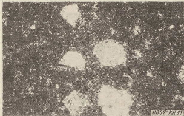
11. ábra. 99,99% tisztaságú alumínium fólián „Eloxál 1” előrétegzéssel készült nagyfeszültségű záróréteg fénymikroszkópos képe (90×)
