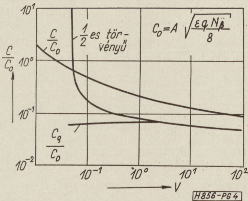
4. ábra. A különféle elméletekkel számított kapacitásfeszültség-függvények összehasonlítása
