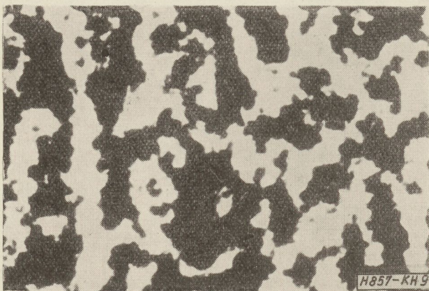
9. ábra. 99,99% tisztaságú alumíniumfólián „Böhmit A” elő-réteggel készült nagyfeszültségű zárórétg fénymikroszkópos képe (90×)
