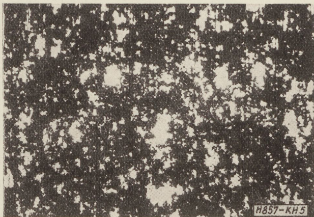
5. ábra. 2 jelzésű elektrolitkondenzátor-sorozat záróréteg-elektrolit határfelületéről készített fénymikroszkópos felvétel 10 000 órás elektromos és hőterhelés után (90×)
