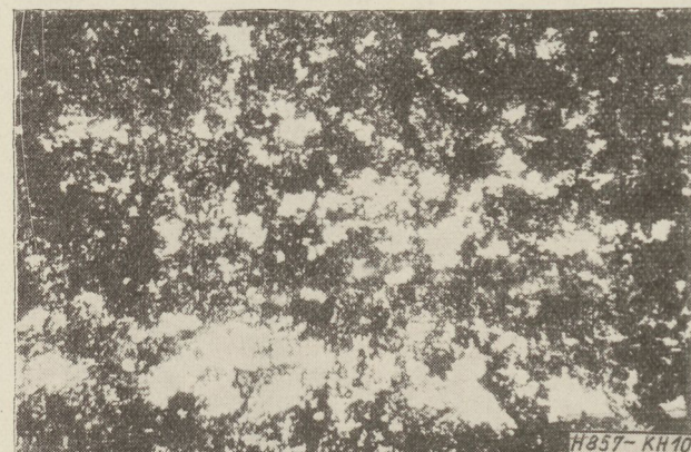
10. ábra. 99,99% tisztaságú alumínium fólián „Böhmit B” előréteggel készült nagyfeszültségű zárórétg fénymikroszkópos képe (90×)
