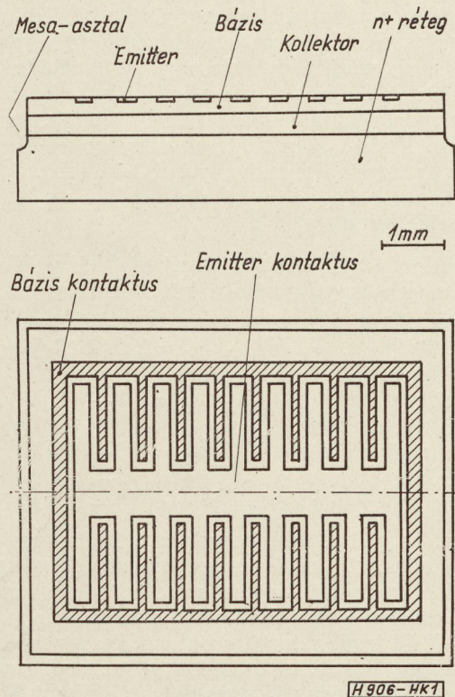
1. ábra. A hazai nagy teljesítményű szilícium kapcsolótranzisztor metszete és felülnézeti rajza
