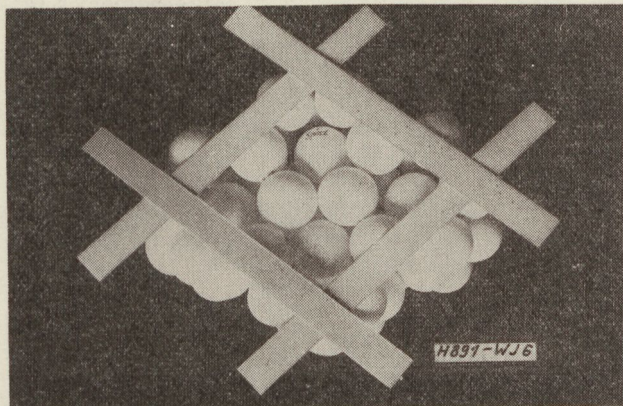
6. ábra. A \sigma -fázis elemi cellájának modellje, felülnézetben
