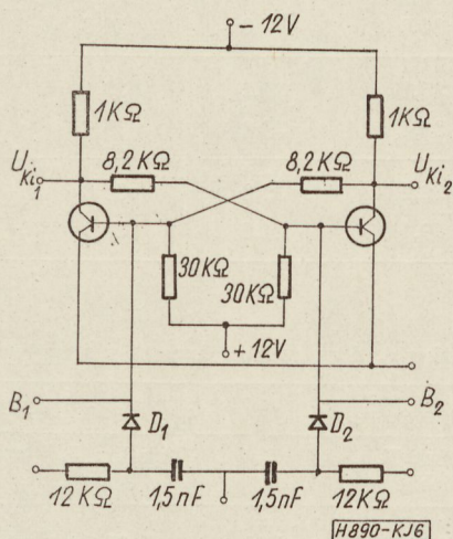
6. ábra. Egy multivibrátor kapcsolási rajza, ami hibrid kivitelben elkészült
