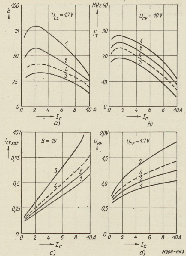
3. ábra. Nagy teljesítményű kapcsoló tranzisztorok karakterisztikái: a) az áramerősítési tényező, b) a határfrekvencia, c) a telítési feszültség, d) a nyitófeszültség a kollektoráram függvényében, hazai kis (1), közepes (2) és nagy (3) áramerősítési tényezővel rendelkező tranzisztorokra, valamint a céltípusként szereplő tranzisztorra (4) vonatkozóan
