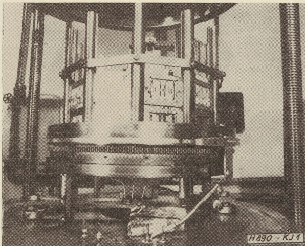
1. ábra. A vákuum párolgató berendezés recipiense a karusszel
