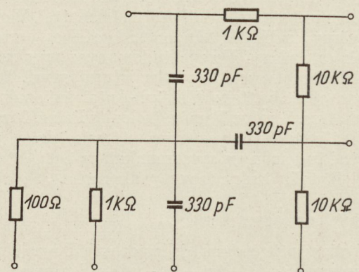
3. ábra. Egy fázis-diszkriminátor passzív elemeinek kapcsolási rajza
