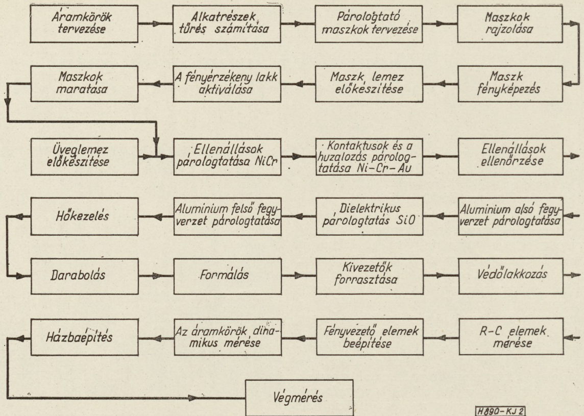
2. ábra. A szigetelő alapú integrált vékonyréteg áramkörök műveleteinek blokksémája
