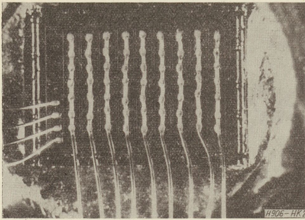
2. ábra. A nagy teljesítményű tranzisztor képe szerelés után
