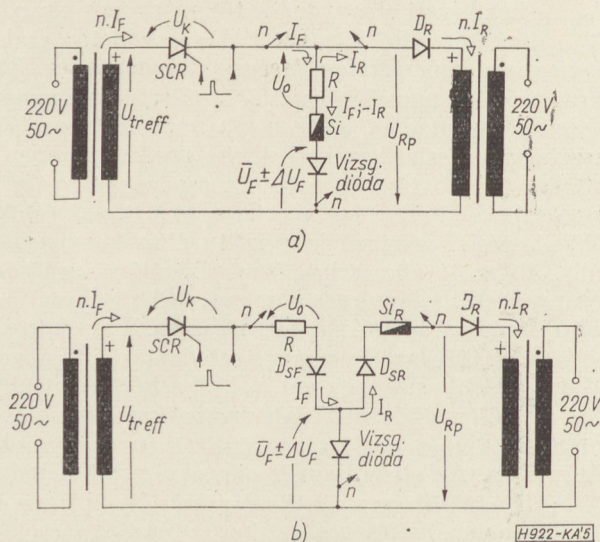
5. ábra. Szintetikus áramkörű kapcsolások a max. átlagáramú (ohmos terheléses) vizsgálatokhoz. A vizsgált diódák egyedi zárlatvédelme az azokkal soros és az effektív nyitóárammal „előfeszített” biztosítókkal történik (a), vagy mindegyik vizsgált dióda nyitó- és záróáram útjai a D_{SF} , ill. D_{SR} diódákkal vannak különválasztva, utóbbival sorban a zárlatvédő biztosítóval (b)
