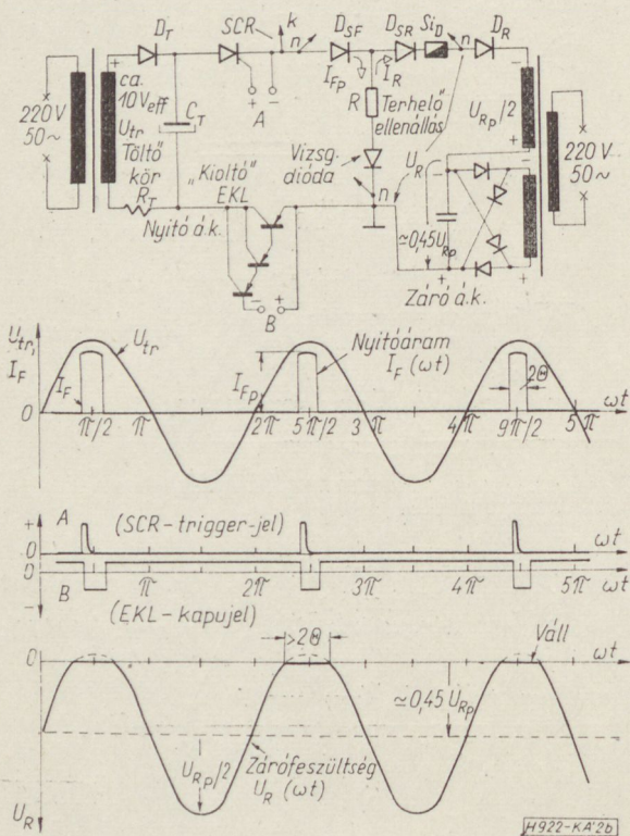
2b. ábra. Periodikus csúcsáramvizsgálatra szolgáló szintetikus áramkör egy formája emitterkövető láncot alkalmazó kioltó áramkörrel, és jellegzetes hullámformái
