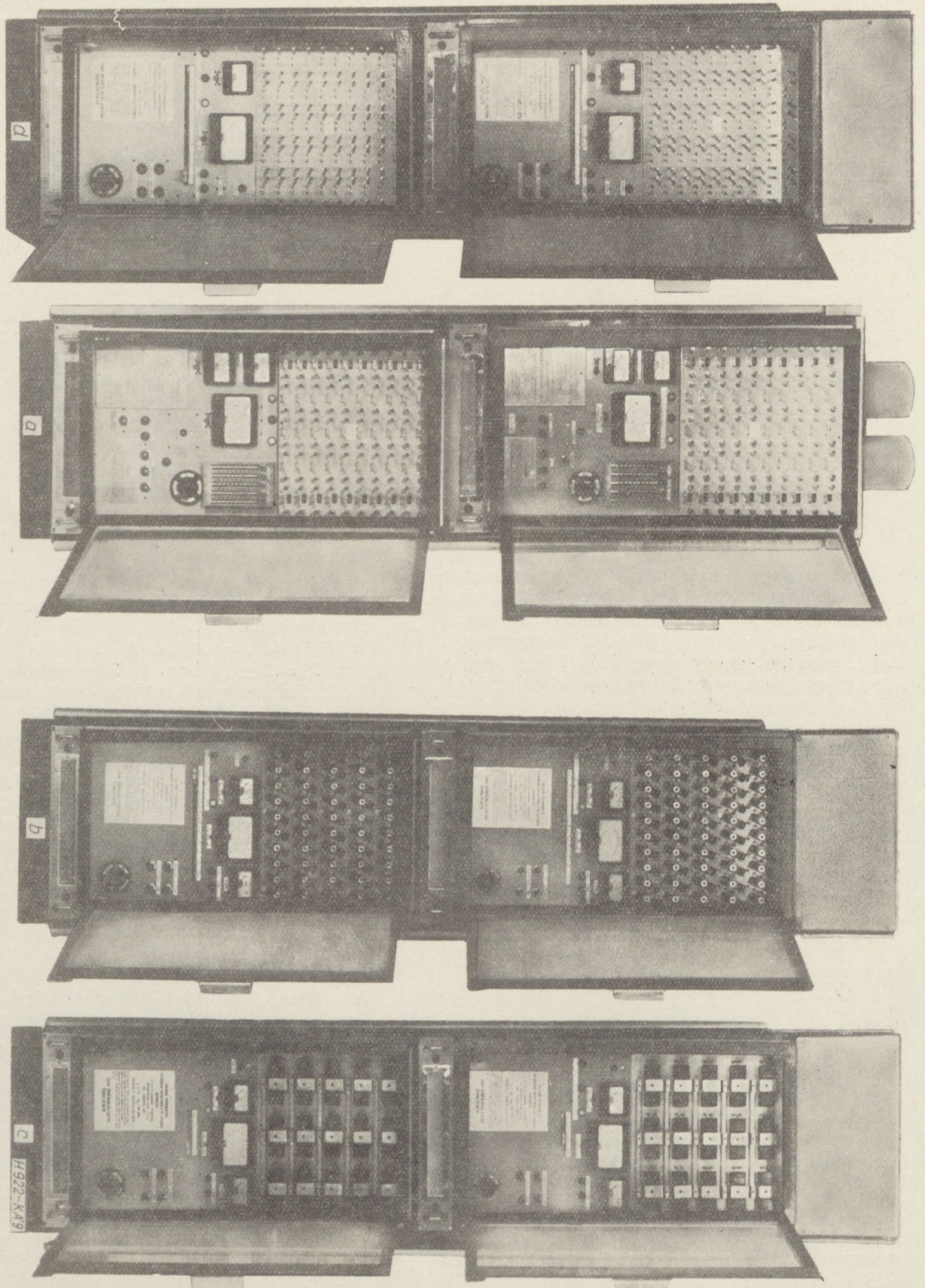
9. ábra. Kivitelezett dióda élettartamvizsgálók : a) 100 vizsgálóhelyes átlagáramterhelő berendezés 1 A-es egyenirányítókhoz, b) ugyanaz, de a 3 A-es diódákhoz, c) 30 vizsgálóhelyes átlagáramterhelő berendezés 12 A-es egyenirányítókhoz, d) periodikus csúcsáramvizsgáló 100 db 1 A-es tv-diódához, vizsgálóhelyenként 6 A max csúcsárammal. A zárfeszültség csúcsértéke az összes berendezésben 800 V-ig állítható
