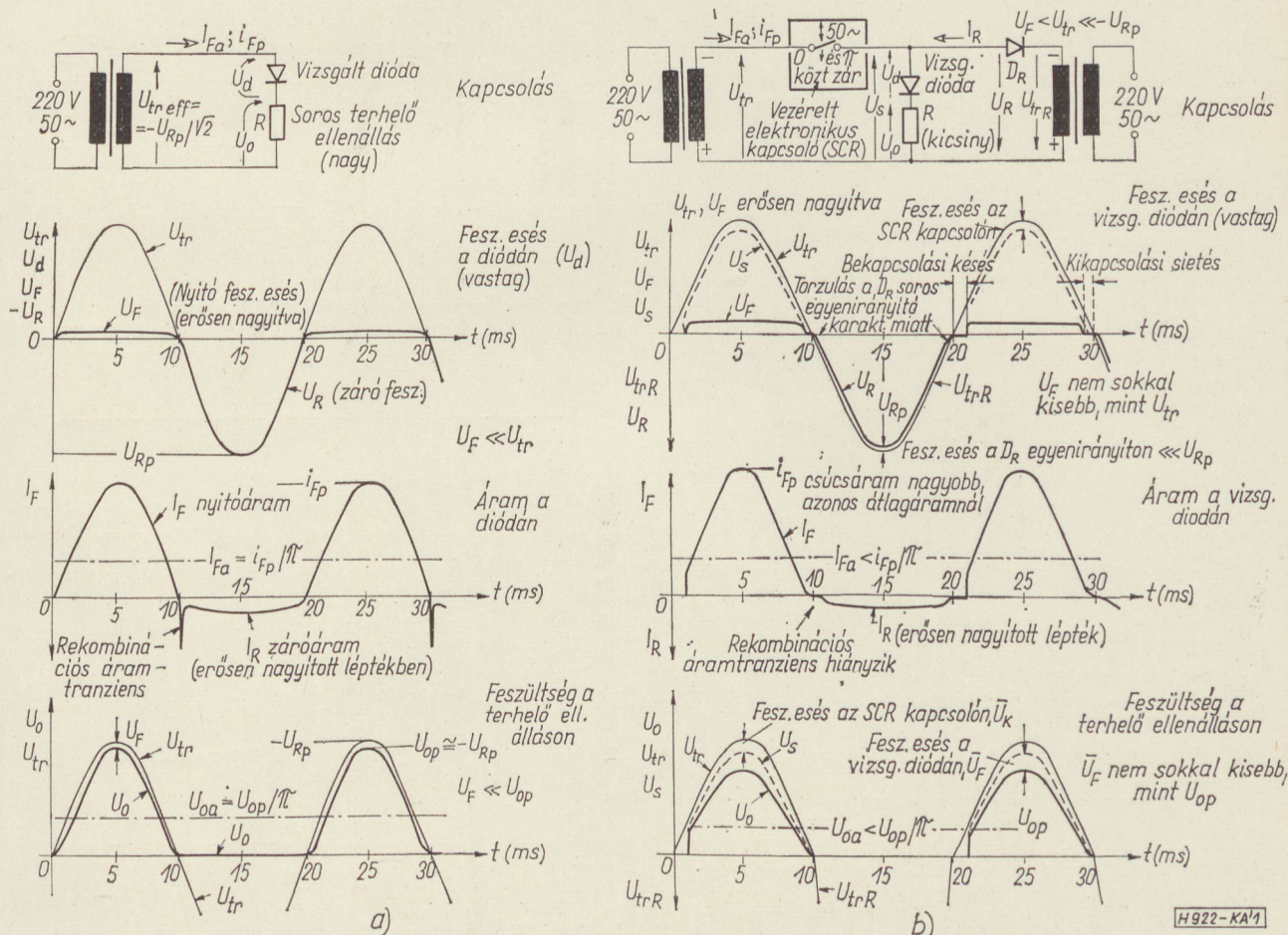
1. ábra. a) A szokásos egyutas ellenállásterhelésű egyenirányító kapcsolás és jellegzetes hullámformái; b) Szintetikus áramkör vázlatos kapcsolása egyenirányító diódák max átlagáram vizsgálatára és jellemző hullámformái.
