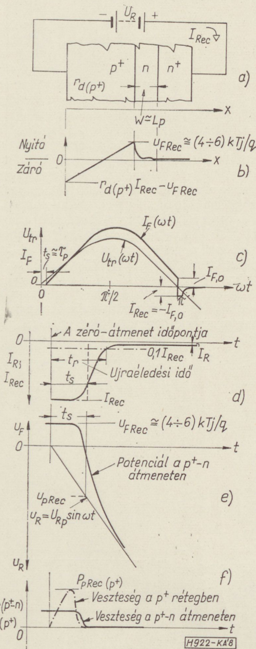
8. ábra. A rekombinációs tranziens feszültség- és áram-hullámformái: a) szilícium PIN egyenirányító struktúrája és b) tengelymenti potenciálosztás a tranziens alatt; a p^+-n átmeneten még nyitóirányú előfeszítés van, c) transzformátorfeszültség és a t_s idővel késő nyitóáram időfüggvényei, d) az áramtranziens időfüggvénye, e) U_R szinuszos zárófeszültség és az átmeneten eső feszültség a zárófélperiódus kezdetén, f) a tranziens aktív (folytonos vonal) és meddő teljesítménykomponenseinek (szaggatott vonal) időfüggvényei (utóbbi a függőleges irányban nem léptékhű)
