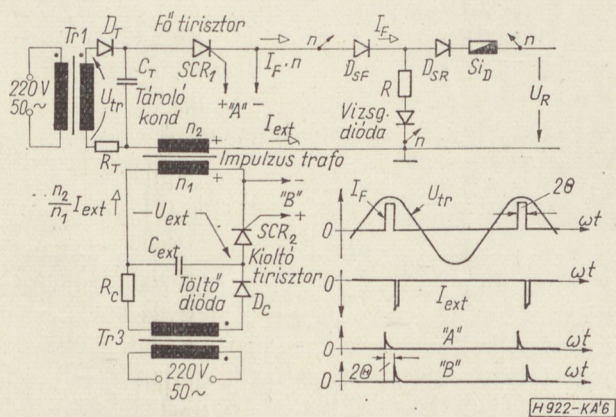
6. ábra. A max. periodikus csúcsáramvizsgálatra szolgáló szintetikus kapcsolás egy eltérő formája, ahol a kioltó áramkör egy másik SCR 2 tirisztort és impulzustranzisztort tartalmaz
