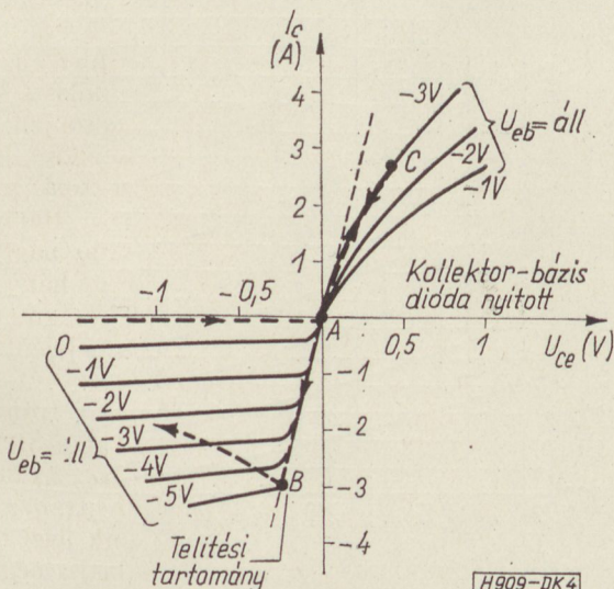
4. ábra. PNP teljesítménytranzisztor kollektor-jelleggörbéi
