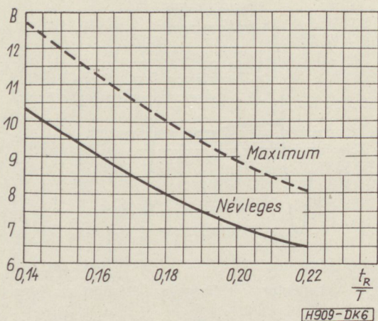
6. ábra. A tranzisztor kollektorán fellépő maximális feszültség és a tápfeszültség hányadosa a visszafutási idő függvényében
