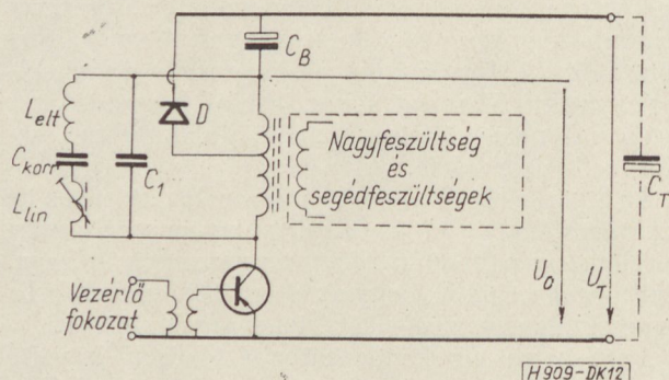
12. ábra. Feszültségvisszanyerő alapáramkör
