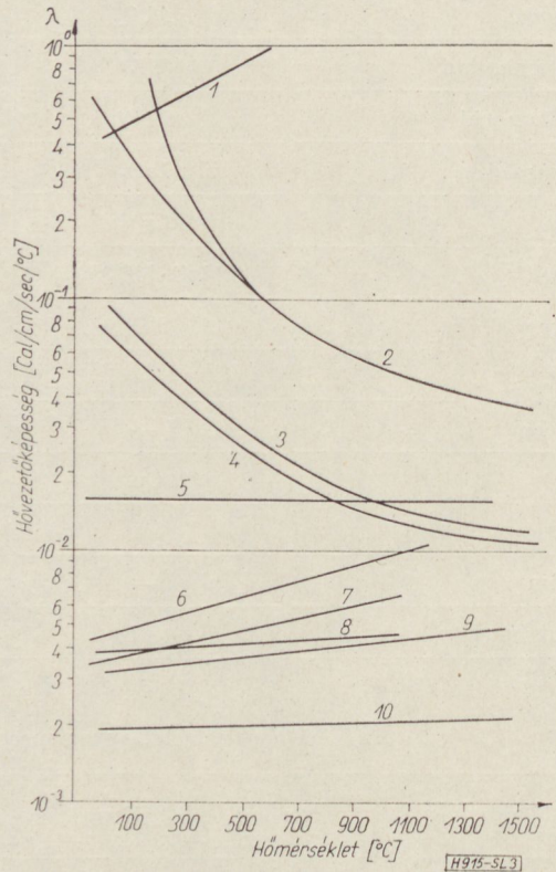
3. ábra. Néhány ismertebb anyag hővezetőképességének hőmérséklet-függése. (10, 11, 12) 1. Alumínium; 2. Berilliumoxid; 3. Magnéziumoxid; 4. Korund; 5. Szilíciumkarbid; 6. Szén; 7. Kvarc-üveg; 8. Zirkonszilikát; 9. Porcelán; 10. Stabilizált zirkonoxid
