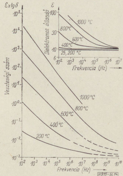
14. ábra. Dielektromos állandó és dielektromos veszteség (veszteségi szám) frekvencia-függése különböző hőmérséklet-nél; 99% \text{Al}_2\text{O}_3 tartalmú zsugorított korund (15)
