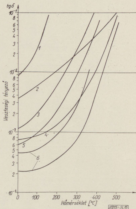
15. ábra. Üvegek veszteségi tényezőjének hőmérsékletfüggése. (6) Mérőfrekvencia: 1 MHz
