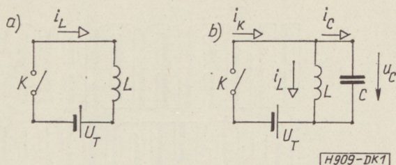
1. ábra. Az eltérítő áramkörök legegyszerűbb formái
