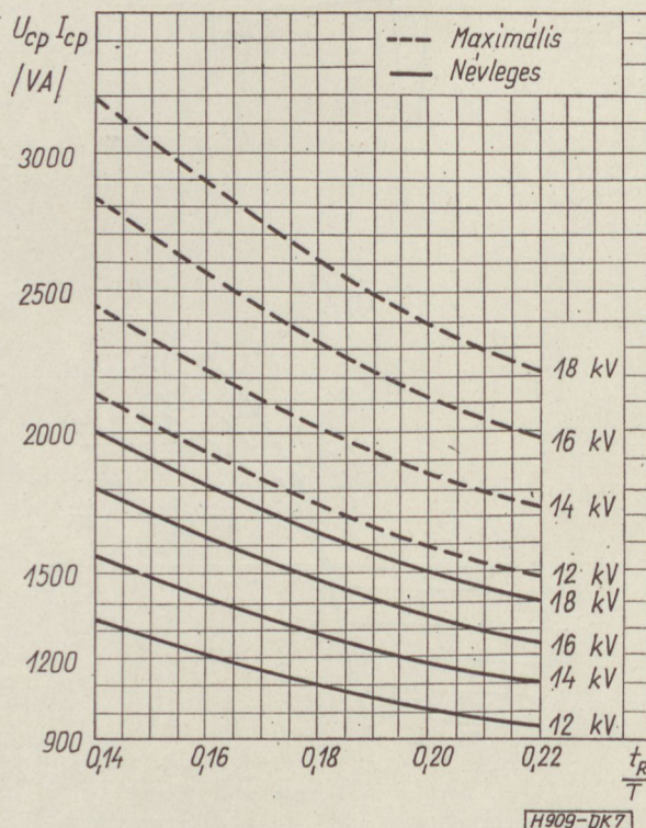
7. ábra. Kapcsolási teljesítmény a visszafutási idő függvényében, paraméter a képcső anódfeszültsége
