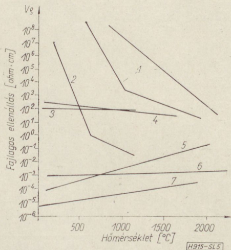
5. ábra. Ismertebb anyagok fajlagos (térfogati) ellenállásának hőmérsékletfüggése. (13) 1. Tűzálló oxidok (olvadáspont > 2000 °C); 2. Félvezetők; 3. Kanthal DS ötvözet; 4. Elektrolitok; 5. Karbidok; 6. Grafit; 7. Használatosabb fémek
