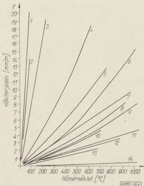
4. ábra. Lineáris hőterjedés — hőmérséklet összefüggés különböző anyagoknál. (10, 11, 12) 1. Szilikongumi; 2. Polietilén; 3. Teflon; 4. Alumínium; 5. Réz; 6. Kanthal DS ötvözet; 7. Zirkonoxid; 8. Szteatit; 9. Korund; 10. Berilliumoxid; 11. Wolfram; 12. Porcelán; 13. Pyrex-üveg; 14. Kvarcüveg
