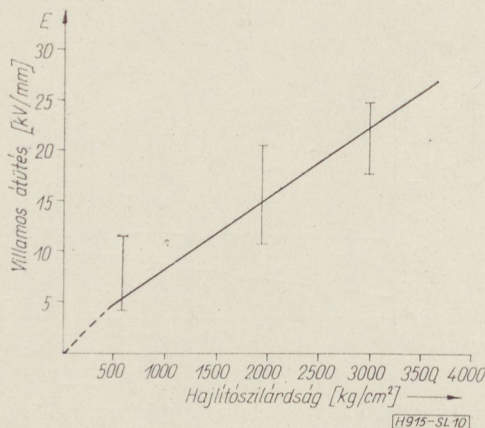
10. ábra. Villamos átütés — hajlítoszilárdság összefüggés zsugorított alumíniumoxid kerámiákon végzett vizsgálat alapján (17)
