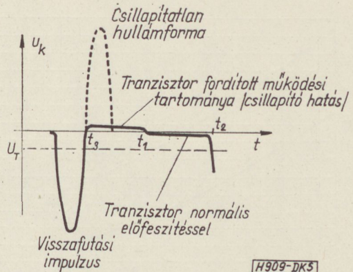
5. ábra. A kollektor feszültsége az eltérítési periódus alatt
