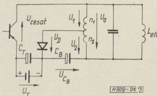
13. ábra. Feszültségvisszanyerő soreltérítő áramkör egyszerűsített kapcsolási rajza
