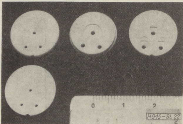
22. ábra. Fémréteghordozó potenciométerpályák titföld alapa nyagból
