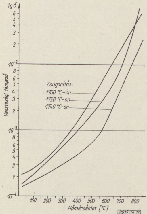
13. ábra. Különböző hőmérsékleten zsugorított korundok veszteségi tényezőjének hőmérsékletfüggése. HIKI korund, \text{Al}_2\text{O}_3 tartalom > 99,7\% ; Mérőfrekvencia 10 MHz. (Rhode Schwartz Leitwertmesser.)
