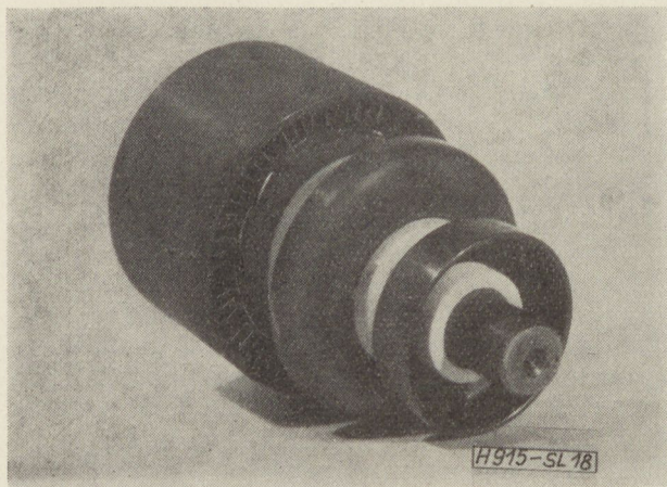
18. ábra. Adócső korund szigetelőkkel
