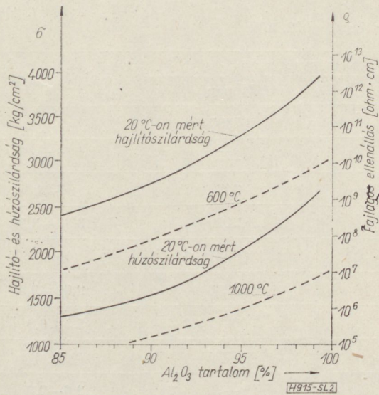
2. ábra. Hajlító- és húzószilárdság, továbbá fajlagos ellenállás (600, 1000 C°-on mért) értékének függése a kerámia alumíniumoxid-tartalmától (12)
