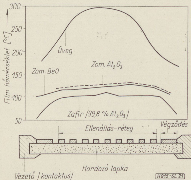
21. ábra. Különböző minőségű, integrált áramkörti hordozó lapkák hőprofiljai terhelés alatt. (23) Zománe vastagság kb. 0,07 mm
