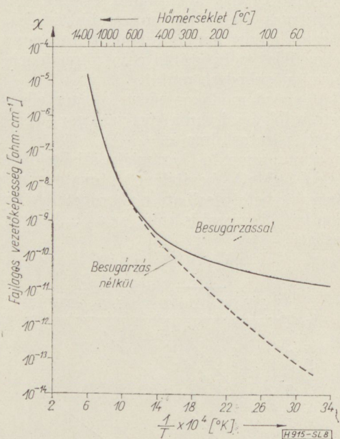
8. ábra. >99% \text{Al}_2\text{O}_3 tartalmú zsugorított korund fajlagos vezetőképességének hőmérsékletfüggése 6 kW/liter teljesítménysűrűségű, 5 percig tartó neutron-besugárzás esetén (16)
