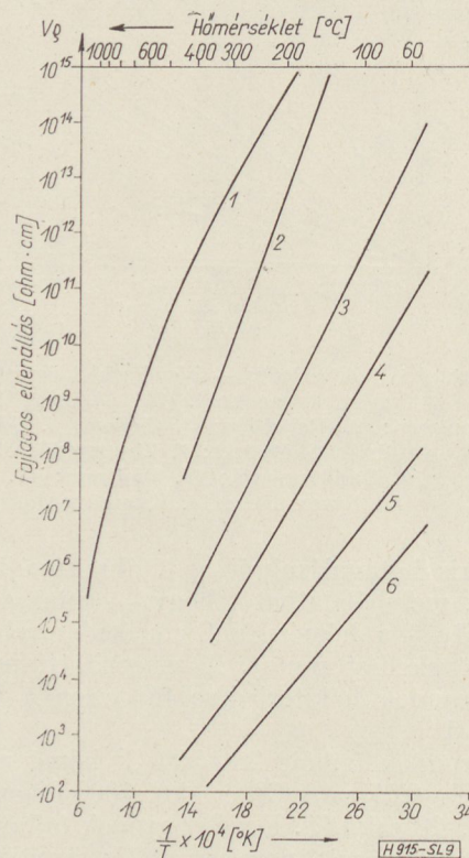
9. ábra. Különböző összetételű üvegek (6) és HIKI-ben készült alumíniumoxid kerámia fajlagos ellenállásának hőmérsékletfüggése.
