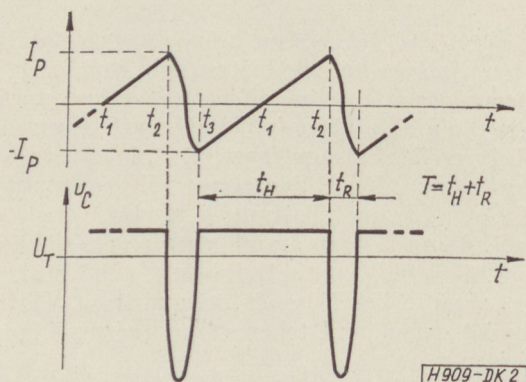
2. ábra. A soreltérítő áramkör áram- és feszültség-hullám-alakjai
