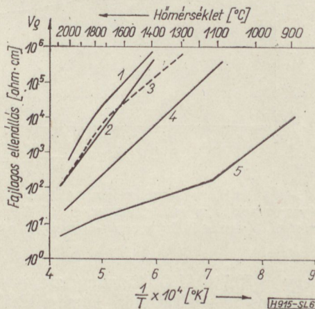
6. ábra. Különböző fémoxid-kerámiák fajlagos ellenállásának hőmérsékletfüggése. (14) Egyenfeszültséggel, nitrogén atmoszférában végzett vizsgálatok.
