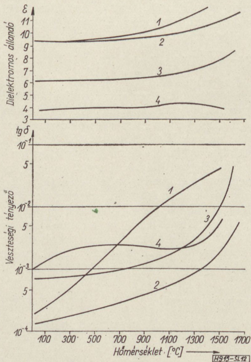
12. ábra. Tűzálló oxidkerámiák és \text{SiO}_2 -üveg dielektromos állandójának, továbbá veszteségi tényezőjének hőmérséklet-függése. (18) Mérőfrekvencia: 10^{10} Hz.
