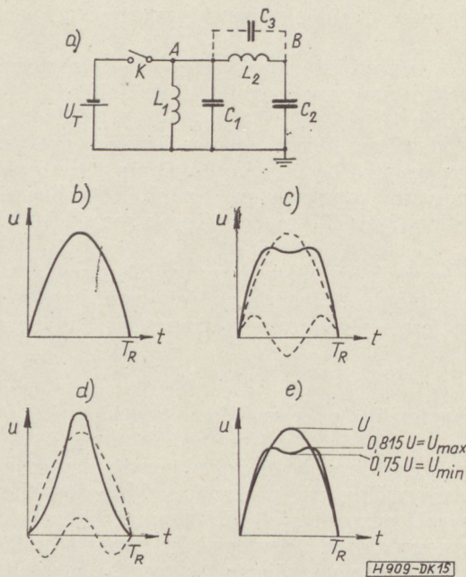
15. ábra. Soreltérítő áramkör nagyfeszültségű részének helyettesítő kapcsolása és hullámformái: a) helyettesítő kapcsolás, b) feszültség-hullámok L_2 és C_2 eltávolításával, c) feszültség-hullámok az A pontban, d) feszültség-hullámok a B pontban, e) az optimális hangoláshoz tartozó hullámok az A pontban
