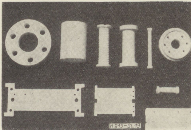
19. ábra. Csőfoglatok, tekercstestek >99,5\% \text{Al}_2\text{O}_3 tartalmú timföld alapanyagból
