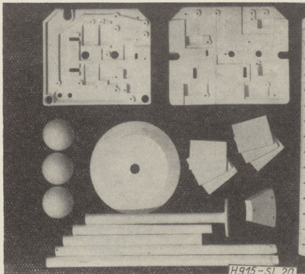
20. ábra. Nyomatott áramkörti panelek, örlőgolyók, ellenállás-értékköszörű kő, integrált áramkörti hordozó lapkák, tengelyek, továbbá nagyfeszültségű szigetelő szegmens timföld alapanyagú alfa-korundból
