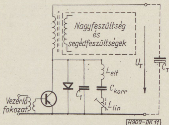
11. ábra. Az eltérítő tekercs bekötésének másik módja áramvisszanyerő végfokozatban
