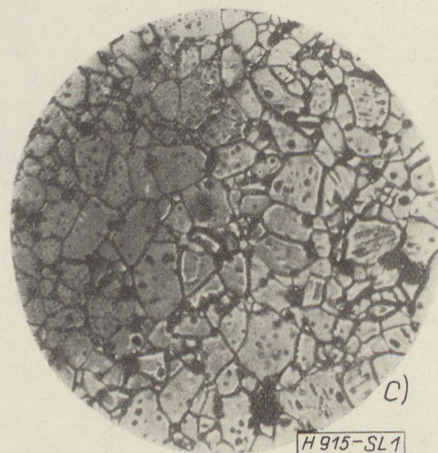
1. ábra. Mikroszkópos felvételek alumíniumoxid kerámia csiszolatokról. HIKI korund, \text{Al}_2\text{O}_3 tartalom > 99,7%. + 0,1% \text{MgO} . Nagyítás: 250 \times .
