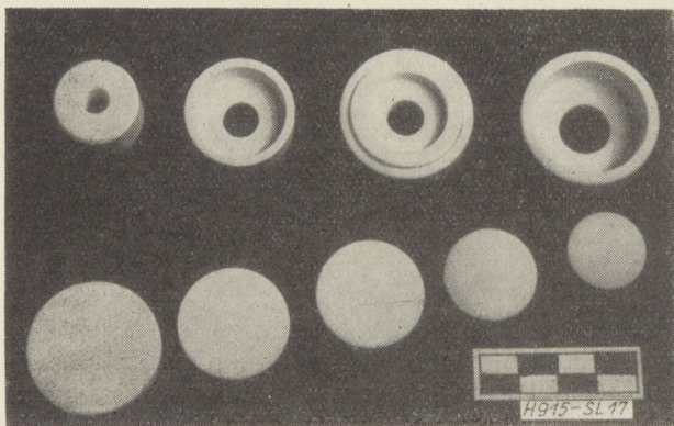
17. ábra. Különböző elektromos szigetelők és mérőtárcsák zsugorított alumíniumoxidból
