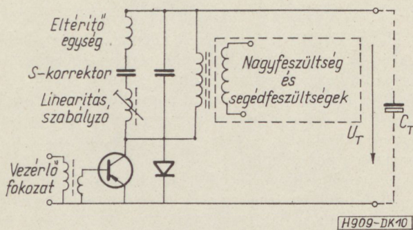
10. ábra. Áramvisszanyerő alapáramkör
