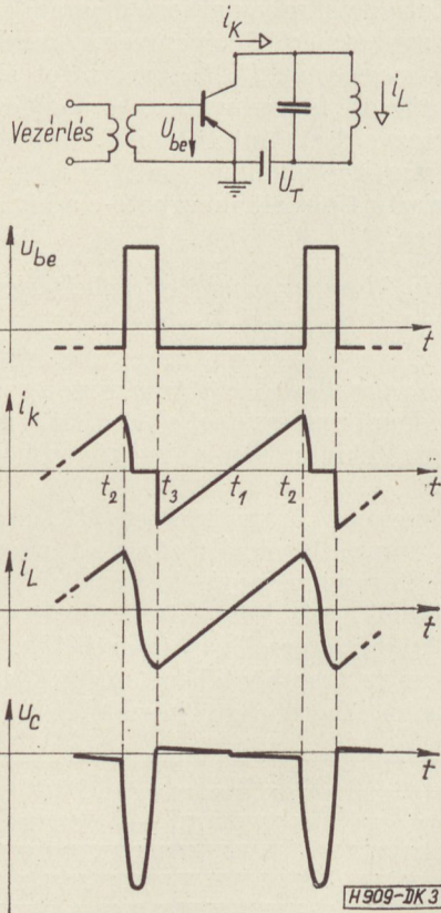
3. ábra. Tranzisztoros sorreltérítő alapáramkör a feszültségek és áramok hullámalakjaival
