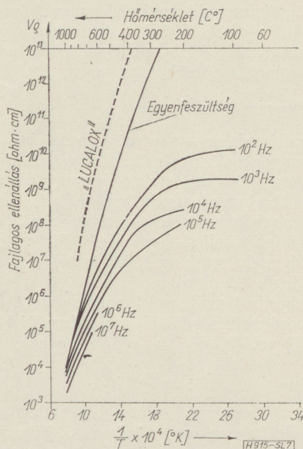
7. ábra. Fajlagos ellenállás és fajlagos veszteségi ellenállás hőmérsékletfüggése egyenfeszültséggel, ill. különböző frekvenciákkal történt meghatározás alapján. (15) 99% \text{Al}_2\text{O}_3 tartalmú zsugorított korund; 99,9% \text{Al}_2\text{O}_3 tartalmú, kb. 90% fényáteresztő-képességű „Lucalox” polikristályos korund
