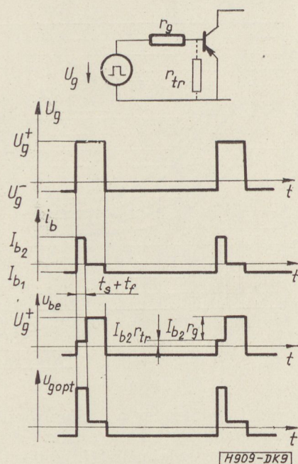
9. ábra. A vezérlőfokozat helyettesítő képe és elméleti hullámformái
