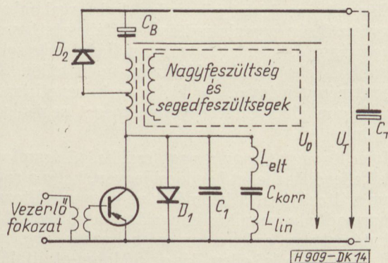
14. ábra. Feszültség- és áramviszanyerő alapáramkör
