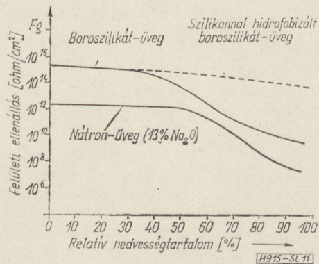
11. ábra. Üvegek fajlagos felületi ellenállásának változása a relatív nedvességtartalom függvényében (6)
