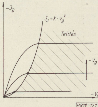
7. ábra. A MOS tranzisztor vázlatos áram-feszültség karakterisztikáserége
