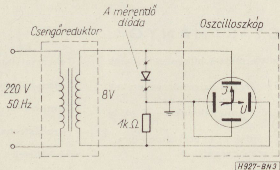
3. ábra. Karakterisztika rajzoló
