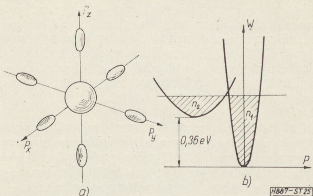
25. ábra. GaAs konstans energiafelületei az impulzustérben
