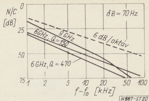
20. ábra. Gunn-diódás oszcillátor FM zaja
