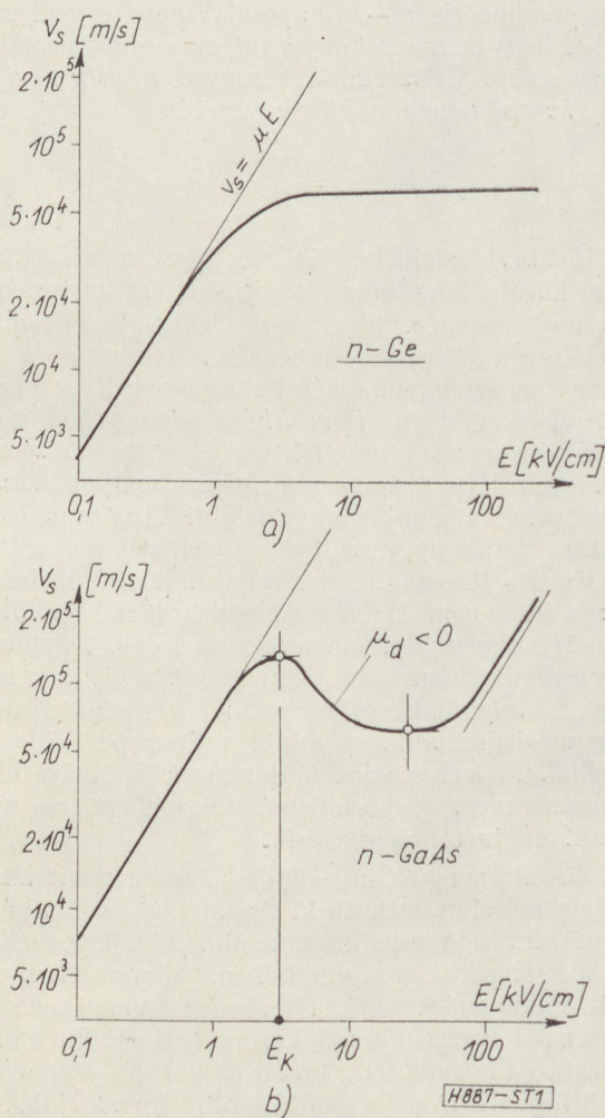
1. ábra. A sodródási sebesség és térerősség kapcsolata: a) n-germánium, b) n-GaAs
