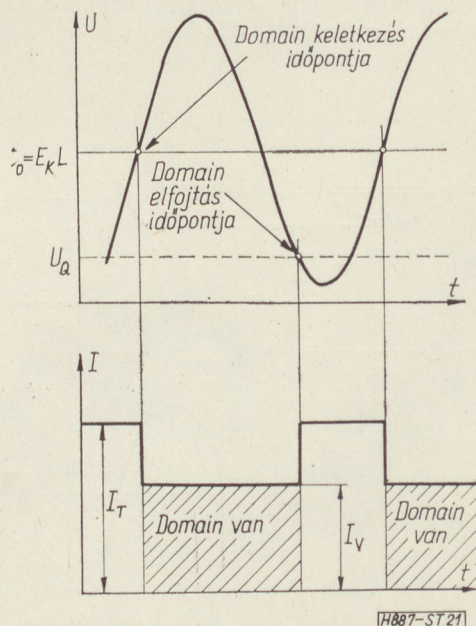
21. ábra. Az üregekben oszcilláló Gunn-dióda kapcsolási feszültsége és árama. A domaint az elektromos erőter elfojtja, ha a kapcsolási feszültség U_0 alá csökken
