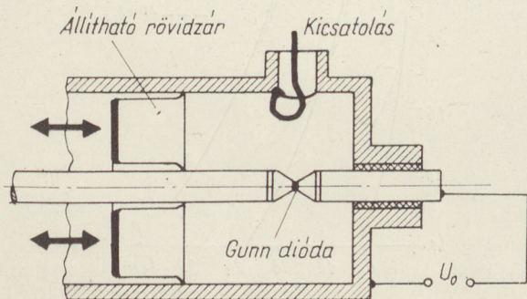
16. ábra. Gunn-diódás oszcillátor. A koaxiális üreg mechanikus hangolása az állítható rövidzárral végezhető
