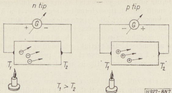
7. ábra. Termofeszültség keletkezésének elvi vázlata
