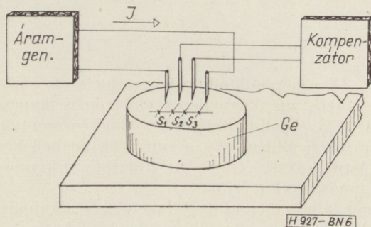
6. ábra. Négy tűs fajlagosellenállás-mérés elvi elrendezése
