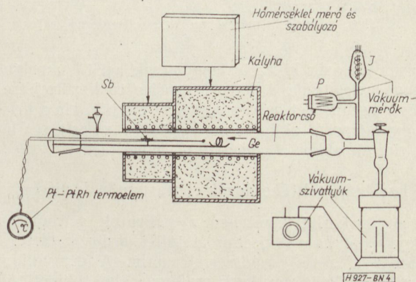
4. ábra. Vákuum diffúziós kályha
