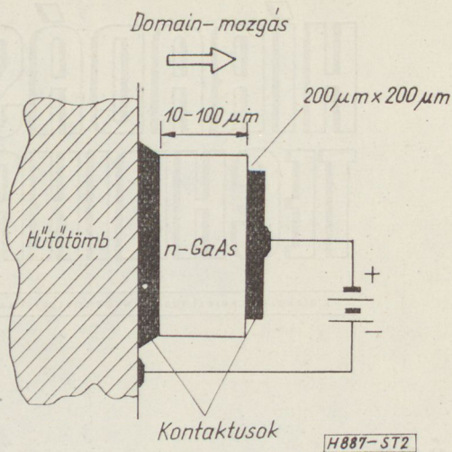
2. ábra. Gunn-dióda
