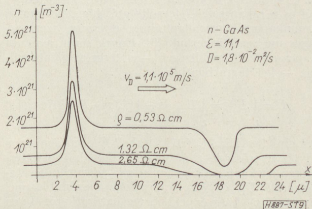
9. ábra. Elektronsűrűség-eloszlás különböző fajlagos ellenállású mintákban (számítógépi eredmény)
