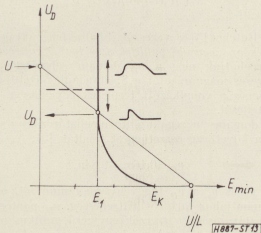
13. ábra. A domain-munkapont meghatározása grafikus módszerrel: a függőleges tengelyen a mintára kapcsolt U feszültségnek megfelelő pontot a vízszintes tengelyen az U/L átlagtérerősségnek megfelelő ponttal összekötve, a metsző egyenes és a görbe metszéspontja megadja a domain-többletpotenciált és a maximális térerősséget
