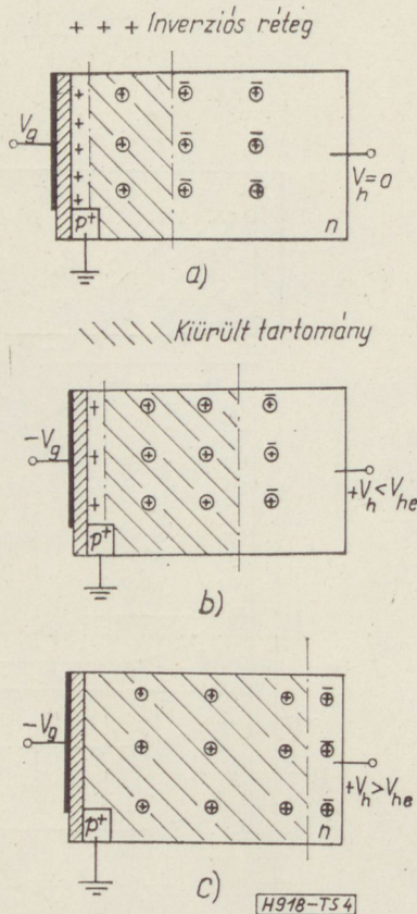
4. ábra. Az inverziós réteg megszüntetése a hordozóhoz viszonyított előfeszítéssel: a) az inverziós réteg előfeszítés nélkül, b) az elzáródási feszültség alatt, c) az elzáródás után
