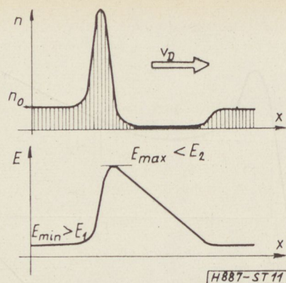
11. ábra. Elektronsűrűség és térerősség-eloszlás háromszög-domain esetén
