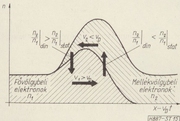
15. ábra. A domainnal egyensúlya magyarázható az elektronoknak a fővölgy és mellékvölgyek közötti szóródásával is
