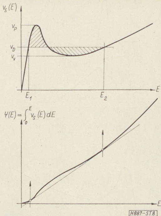
8. ábra. Lapos tetejű domain dinamikus egyensúlyának feltétele: a) az egyenlő területek szabálya, b) érintő egyenes módszer
