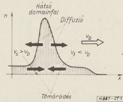
7. ábra. A sodródási áramlás domainfalat tömörítő hatásával a diffúziós áramlás tart egyensúlyt
