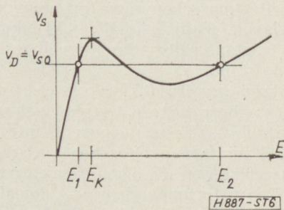
6. ábra. A domainegyensúly ábrázolása a v_s — E diagramban
