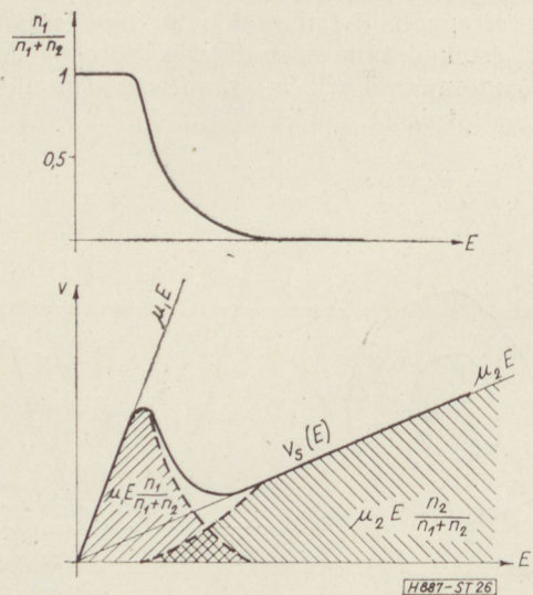
26. ábra. Az átlagos mozgékony-ság származtatása
