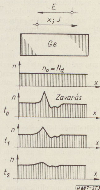
3. ábra. A homogén germániumtömbben a külső behatás megszűntével visszaáll az n=n_0 egyensűlyi állapot
