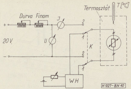
10. ábra. Mérőkapcsolás termisztor karakterisztikák felvételére
