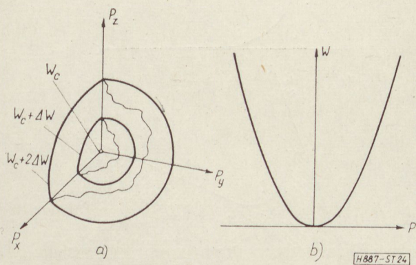
24. ábra. Konstans energiafelületek az impulzustérben
