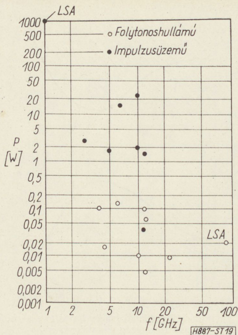
19. ábra. Gunn-diódás oszcillátorokkal elért teljesítményértékek
