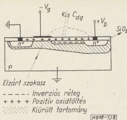
8. ábra. Nagyfrekvenciás, kiürített, n csatornás MOS tranzistor szerkezete
