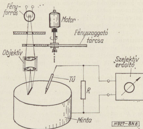
8. ábra. „Valdes” mérési módszer elrendezési rajza
