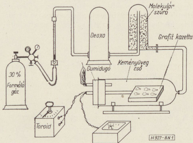
1. ábra. Ötvöző berendezés vázlata
