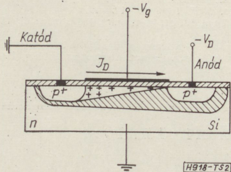
2. ábra. Az inverziós csatorna és a kiürült tartomány vázlata előfeszített, p csatornás MOS tranzisztorban
