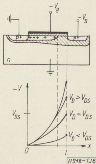
6. ábra. Potenciálviszonyok a telítési állapotban
