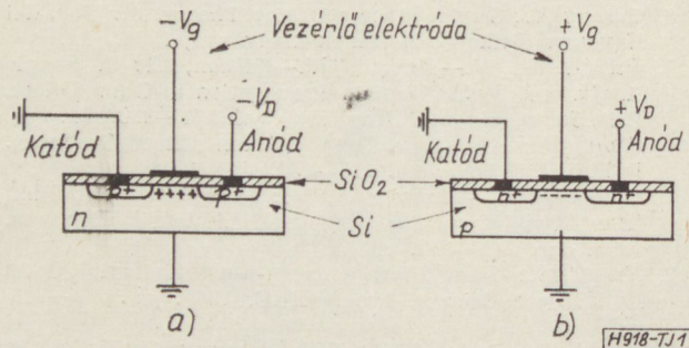
1. ábra. a) p csatornás, b) n csatornás MOS tranzisztorszerkezet vázlat
