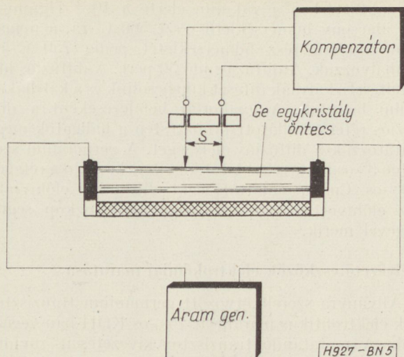
5. ábra. Fajlagosellenállás-mérő műszer vázlata
