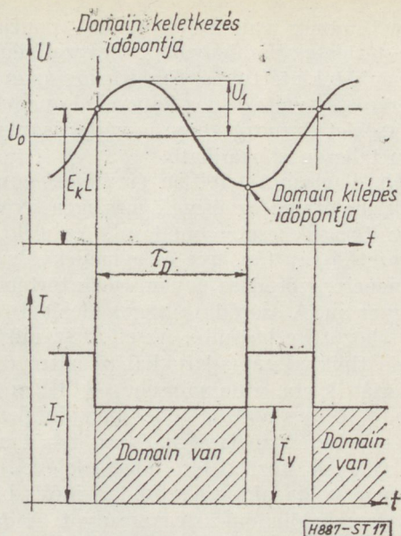
17. ábra. Az üregben oszcilláló Gunn-dióda kapcsolófeszültsége és árama. A domain minden periódusban akkor keletkezik, amikor a kapcsolófeszültség eléri a küszöbfeszültséget
