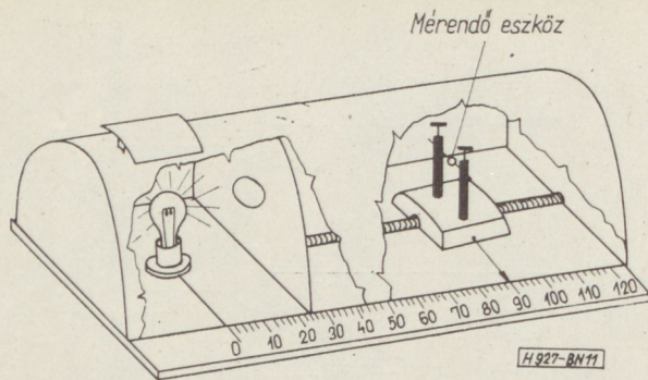
11. ábra. Fotodióda és fototranzisztor mérő berendezés
