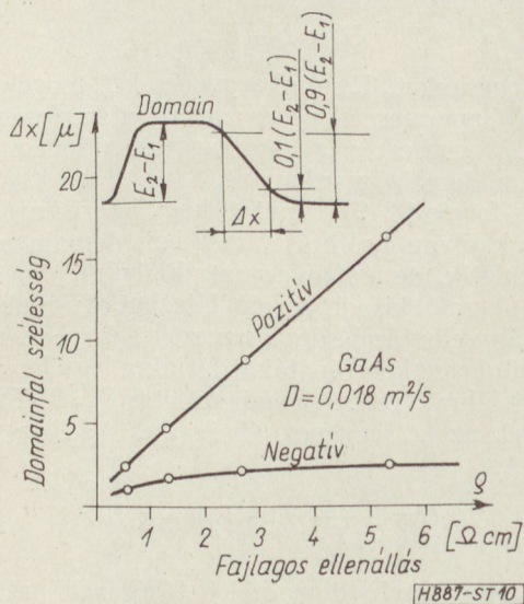
10. ábra. Az anódoldali (pozitív tértöltésű) és a katódoldali (negatív tértöltésű) domainfal szélessége a fajlagos ellenállás függvényében (számítógépi eredmény)
