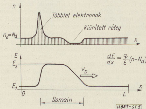
5. ábra. Az instabilitás által okozott elektronsűrűség és térerősség-hullám. v_D a nagy térerősségű domain sodródási sebessége
