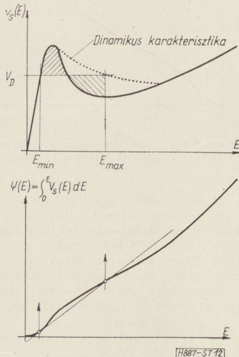
12. ábra. Háromszög-domain dinamikus egyensúlyának feltétele: a) az egyenlő területek szabálya, b) érintő-metsző egyenes módszer
