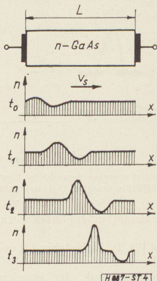
4. ábra. A küszöbtérerősség felett táplált n-GaAs tömbben instabilitás lép fel
