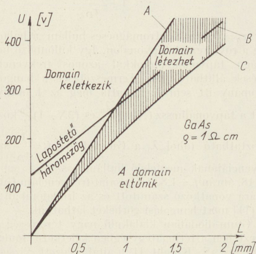
14. ábra. Lehetséges üzemmállapotok a kapcsolási feszültség — mintahossz koordinátákban
