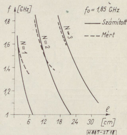
18. ábra. Gunn-diódás oszcillátor frekvenciája a rövidrezárt tápvonal hosszának függvényében. Több rezgési módus lehetséges
