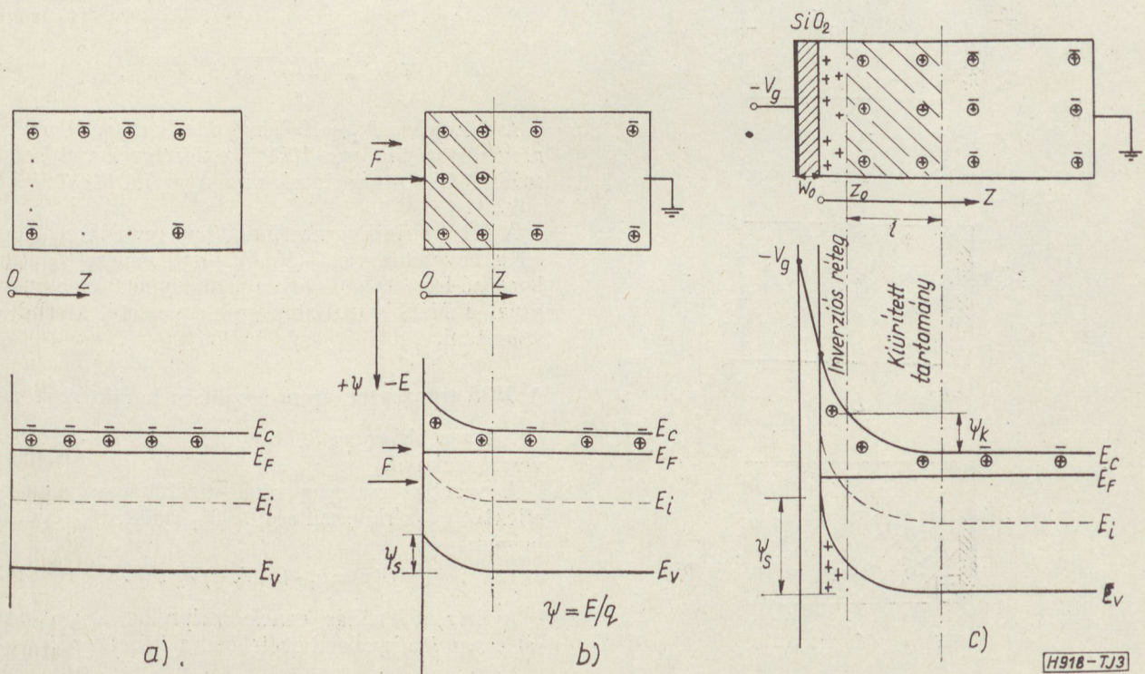
3. ábra. A felületi inverziós réteg kialakulása: a) külső erőter nélkül állapot, b) az inverzióhoz nem elegendő nagy erőterrel előállított helyzet, c) a sáv szerkezet és a töltéeloszlás inverziós réteg kialakulásakor
