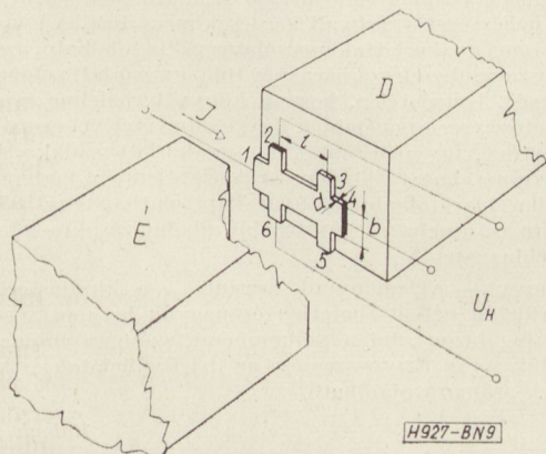
9. ábra. Hall-minta elhelyezése a mágnes légrésében
