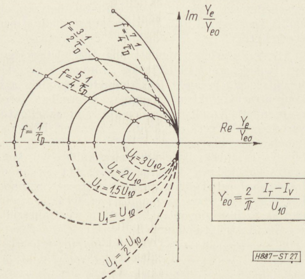
27. ábra. Gunn-dióda elektronikus admittanciája
