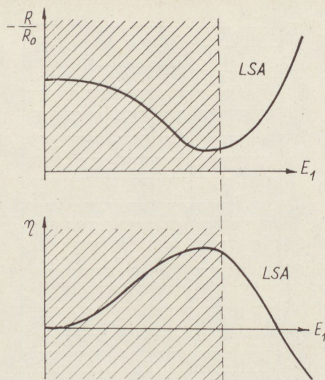
23. ábra. A Gunn-dióda ellenállása és hatásfoka a rádiófrekvenciás térerősség függvényében
