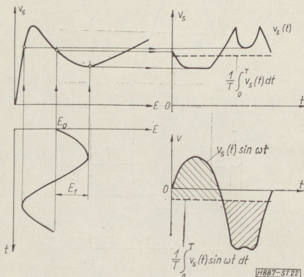
22. ábra. A Gunn-dióda aktív elemként viselkedik, ha az egy periódusra átlagolt differenciális mozgékonyaság negatív
