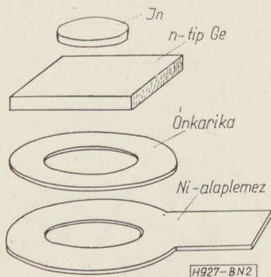
2. ábra. Ötvözött dióda elemei
