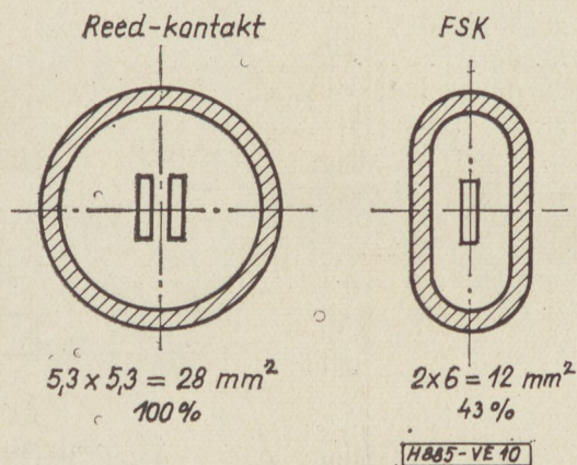
10. ábra. Normál méretű és az FSK kontaktus helyszükséglete
