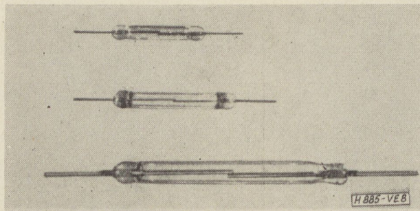
8. ábra. Miniatűr érintkező összehasonlítása normál méretű érintkezővel
