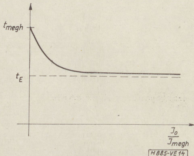
14. ábra. A meghúzási idő változása a túlgerjesztés függvényében
