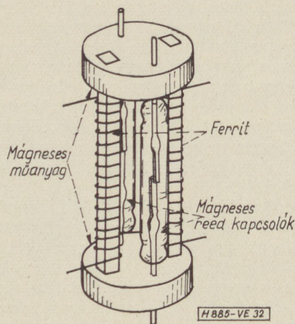
32. ábra. Paralel ferreed
