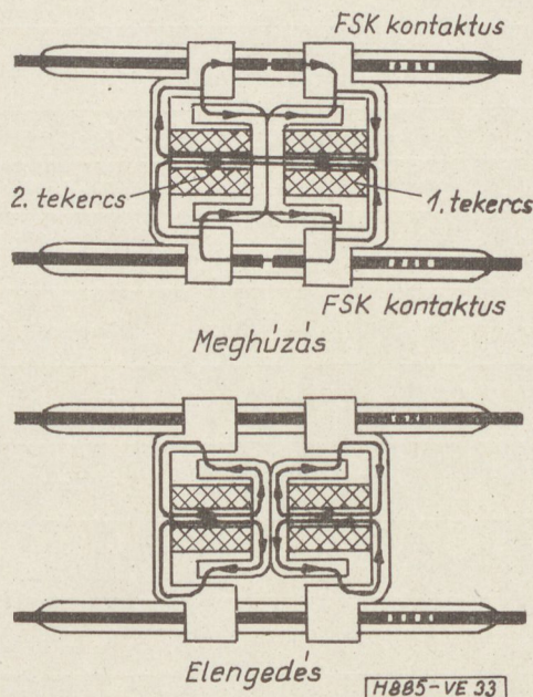
33. ábra. FSK kontaktussal készült soros ferreed elvi felépítése és mágneses fluxusok
