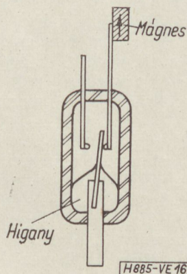
16. ábra. Előfeszített higanyérintkezős jelfogó
