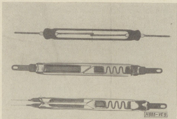
9. ábra. Egy záró és egy morse FSK érintkező összehasonlítva egy normál méretű záró érintkezővel
