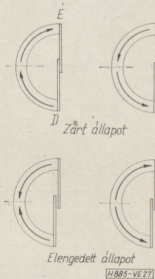
27. ábra. Soros ferreed működési elve
