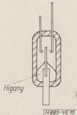
15. ábra. Semleges higanyérintkezős jelfogó
