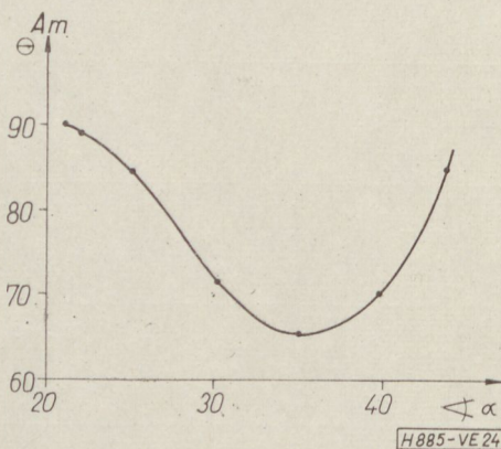
24. ábra. FSK relénél a gerjesztés változása a levágási szög mértéke szerint
