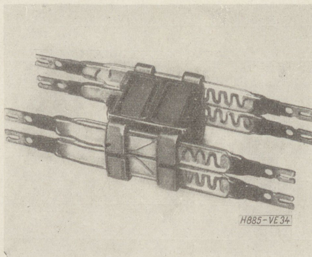
34. ábra. FSK kontaktussal készült soros ferreed gyakorlati megvalósítása
