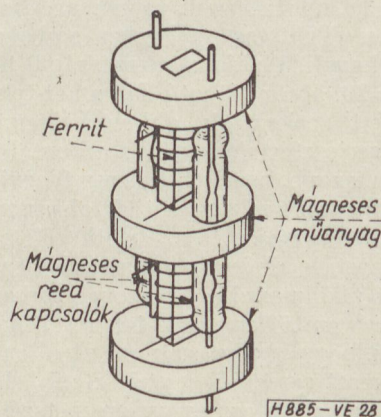
28. ábra. Additív gerjesztésű soros ferreed
