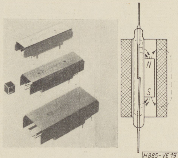
19. ábra. HRE 806 típusú herkon jelfogó
