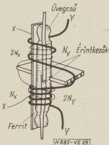
29. ábra. Differenciál gerjesztésű soros ferreed
