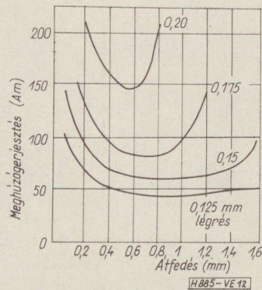
12. ábra. A gerjesztés változása az átfedés függvényében különböző légrések esetén
