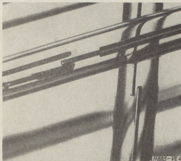
4. ábra. Előtérben a Siemens und Halske cég morse érintkezője, mögötte egy normál méretű záró érintkező
