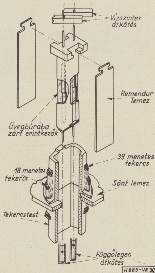
30. ábra. Kapcsolómező keresztpontjaként alkalmazott soros ferreed
