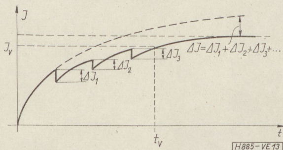
13. ábra. A gerjesztőáram változása többérintkezőjű jelfogó meghúzása esetén
