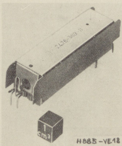
18. ábra. HRE 804/1 típusú herkon jelfogó
