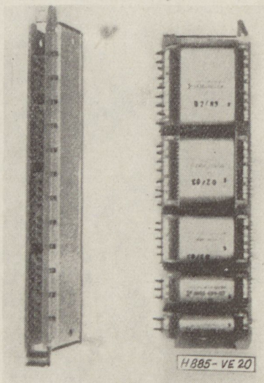
20. ábra. HRM 813 típusú herkon jelfogó
