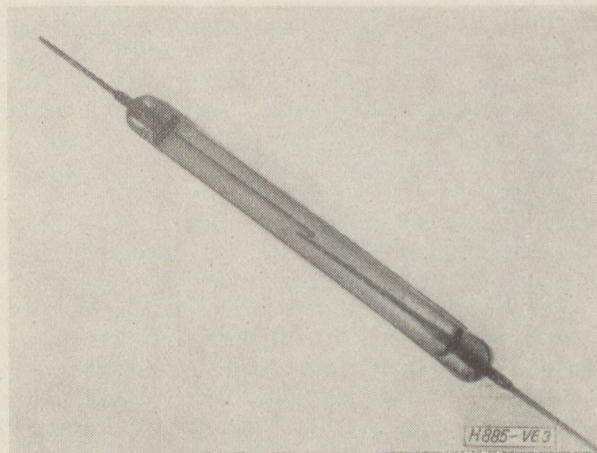
3. ábra. Normál méretű száraz érintkezős kapcsolóelem
