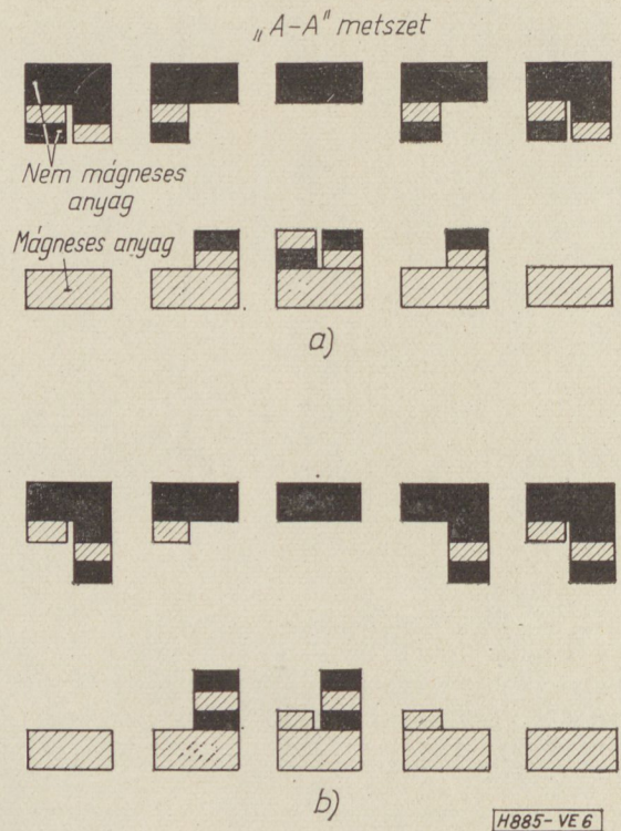
6. ábra. Előbb záró, aztán bontó érintkezők működése
