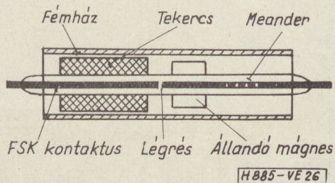
26. ábra. Tartó jelfogó FSK kontaktussal
