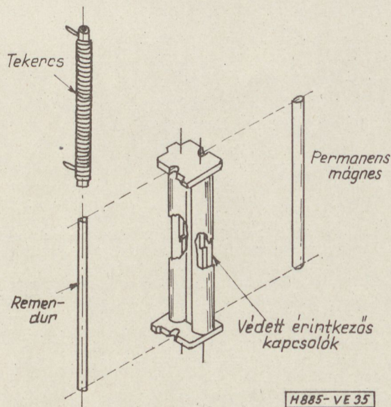
35. ábra. Bipoláris ferreed
