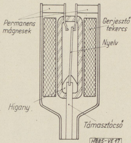
17. ábra. Polarizált higanyérintkezős jelfogó
