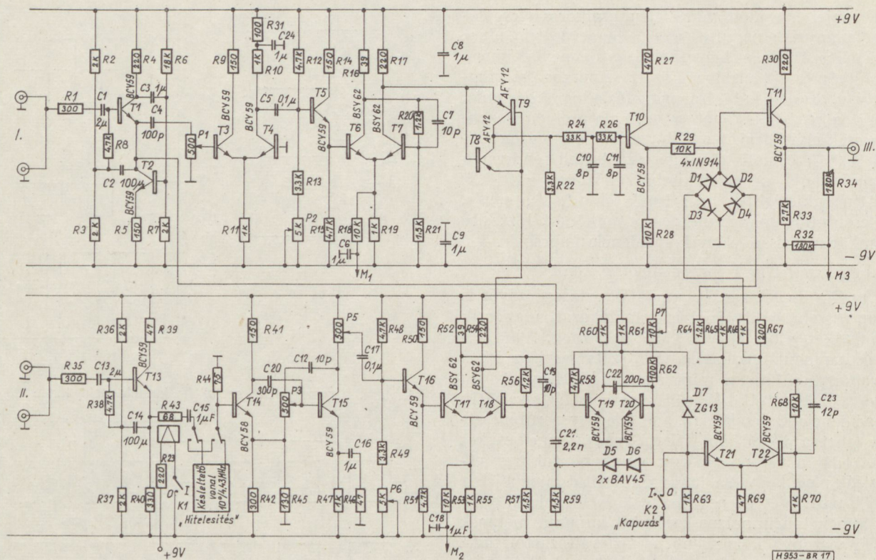
17. ábra. Az EMV-ben kifejlesztett műszer elvi rajza
