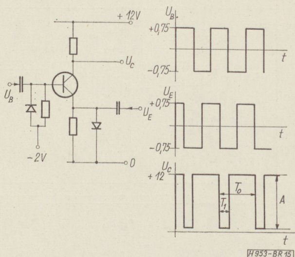
15. ábra. Egyszerű fázisszelektív koincidencia kapcsolás
