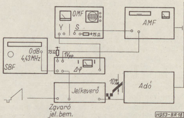
18. ábra. Differenciális fázishiba mérési összeállítás
