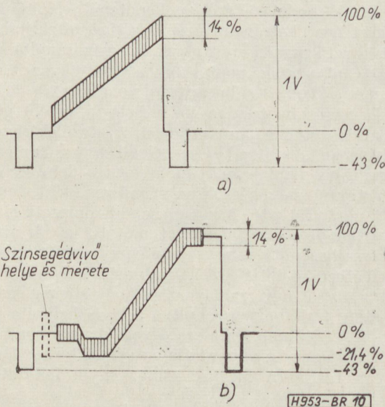
10. ábra. Differenciális fázisméréshez alkalmazott mérőjelek
