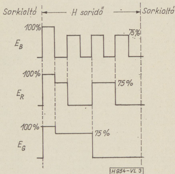
3. ábra. Elektronikus színsávgenerátor 75% telítettségű alapjelei
