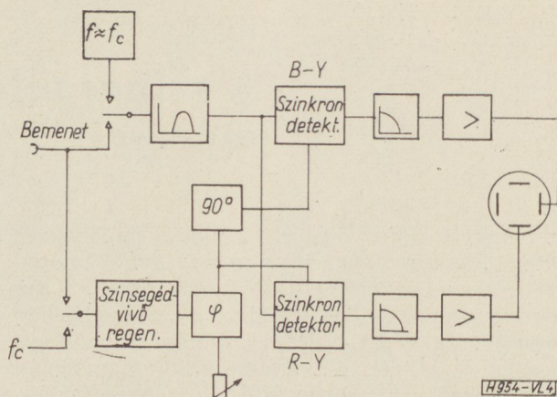
4. ábra. Vektorszóp kapcsolási vázlata
