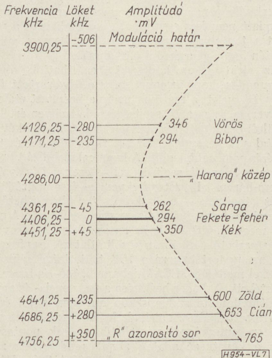
7. ábra. SECAM-színjel jellemzői D'_R sornál 75% telítettségű színsáv közvetítésekor
