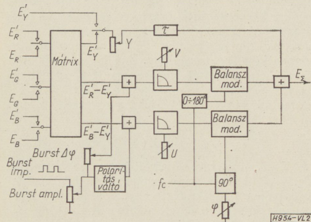
2. ábra. PAL-kódor kapcsolási vázlata
