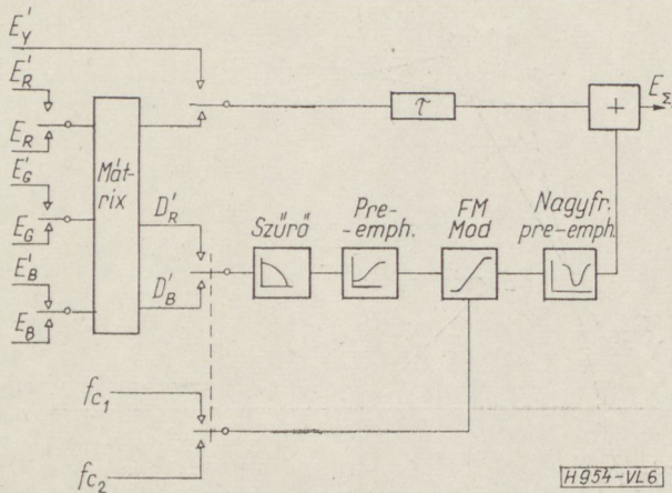
6. ábra. SECAM-kóder vázlatos felépítése
