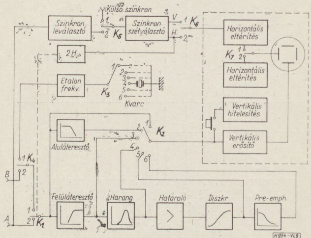
9. ábra. Szekamszkóp vázlatos felépítése
