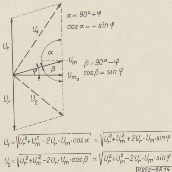
14. ábra. A kimenő feszültség vektordiagramja a 13. ábra szerinti diszkriminátornál
