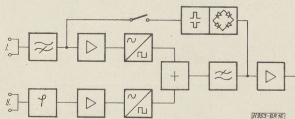
16. ábra. Az Elektromechanikai Vállalatnál kifejlesztett differenciális fázismérő blokkvázlata
