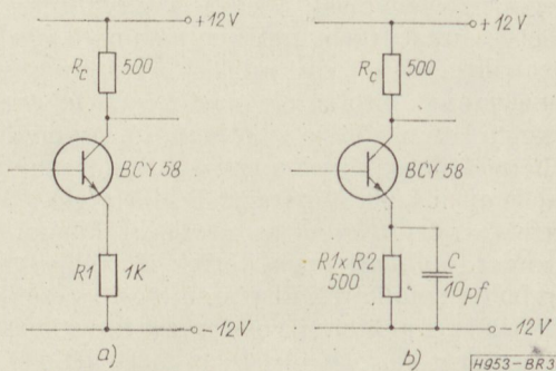
3. ábra. A korrektor fokozat emitter körének alakulása: a) fekete szintnél; b) fehér szintnél
