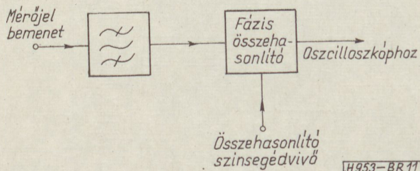
11. ábra. A differenciális fázishiba mérésére alkalmas műszerek elvi felépítése
