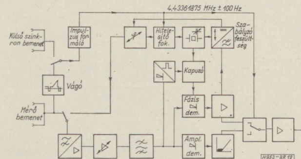
12. ábra. Rohde—Schwarz gyártmányú PVF-műszer blokk-vázlata
