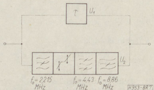
7. ábra. Sávszűrős differenciális fáziskorrektor blokkvázlata
