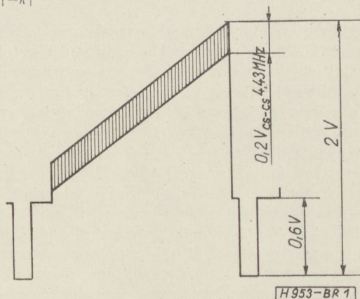
1. ábra. Korrektor bemenőjel
