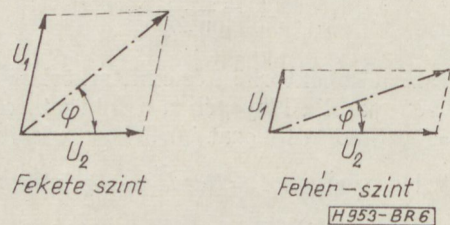
6. ábra. Az 5. ábra szerinti korrektor kimenőjelének alakulása fekete, illetve fehér szintnél
