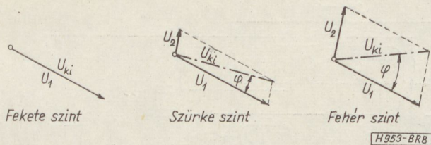
8. ábra. A 7. ábra szerinti korrektor kimenőjelének alakulása különböző szinteknél
