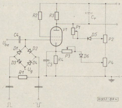
4. ábra. Egycsatornás differenciális fáziskorrektor
