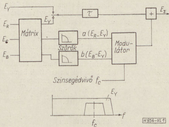
1. ábra. Kompatibilis színes jelformálás vázlata
