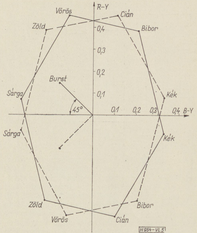
5. ábra. 75% telítettségű színsávjelek PAL vektorábrája
