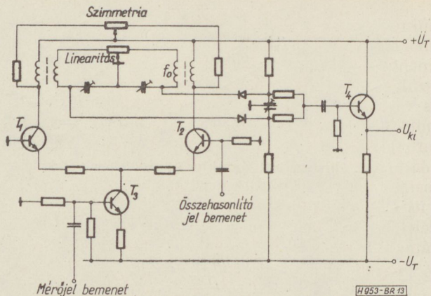
13. ábra. A PVF műszerben alkalmazott fázis diszkriminátor elvi vázlata
