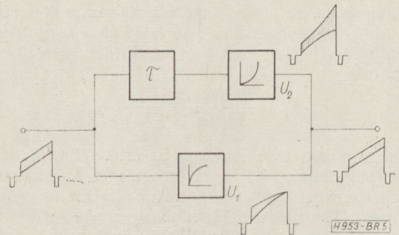
5. ábra. Fázistolós differenciális fáziskorrektor blokkvázlata
