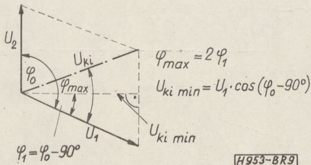
9. ábra. A 7. ábra szerinti korrektor fázisszögeinek számítása
