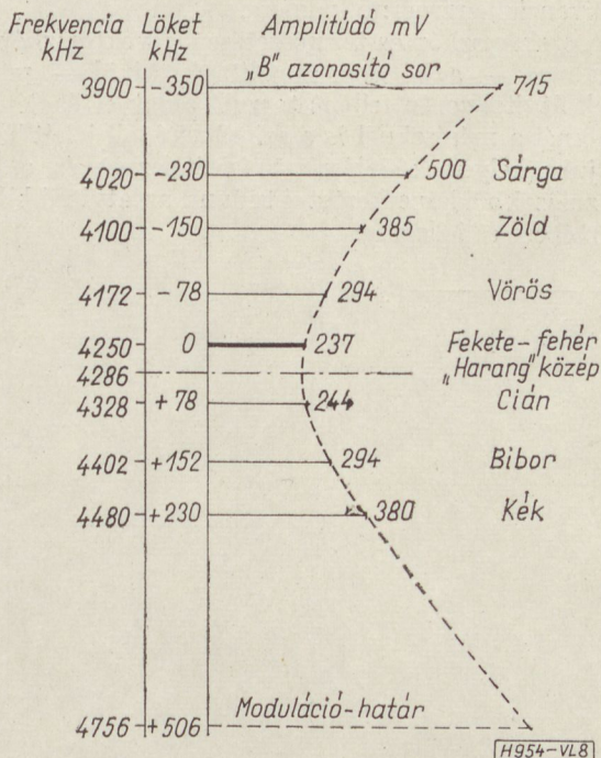
8. ábra. SECAM-színjel jellemzői D'_B sornál 75% telítettségű színsáv közvetítésekor
