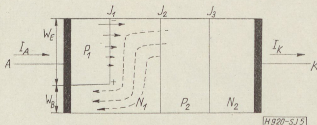
5. ábra. Rövidrezárt emitterű négyrétegű dióda felépítése
