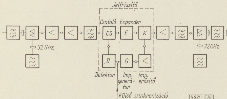
6. ábra. Vonali ismétlőerősítő
