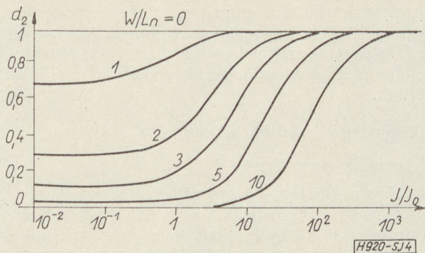
4. ábra. \alpha_2 a normalizált áram függvényében
