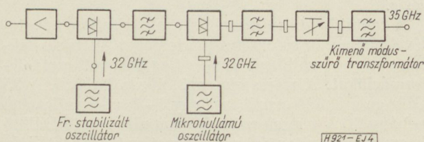
4. ábra. Adóoldali végberendezés
