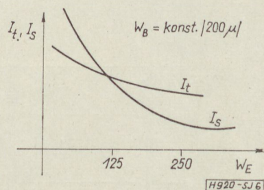
6. ábra. Kapcsoló- és tartóáram az emitterszélesség függvényében
