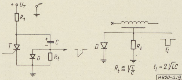
9. ábra. Impulzus generátor
