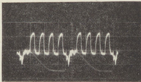
Kék vezérlés: kék rác-katód jel Függőleges lépték: 50 V/osztás a)
