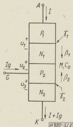
2. ábra. A vezérelt négyrétegű kapcsoló felépítése
