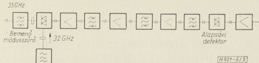
5. ábra. Vevőoldali végberendezés
