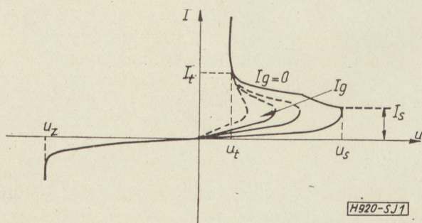
1. ábra. A négyrétegű kapcsoló karakterisztikája
