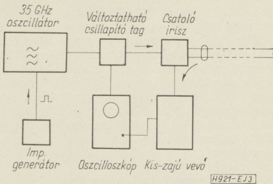
3. ábra. Csillapításmérés reflektált impulzusokkal
