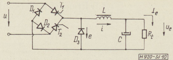
10. ábra. Egyenirányító kapcsolás tirisztorral
