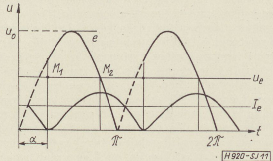
11. ábra. A 10. ábra kapcsolásához tartozó hullámformák
