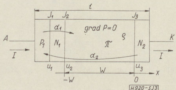
3. ábra. A PN \pi N kapcsoló felépítése
