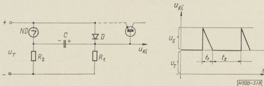
8. ábra. Impulzus generátor
