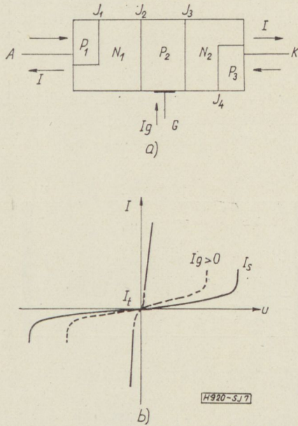
7. ábra. Ötrétegű kapcsoló és karakterisztikája
