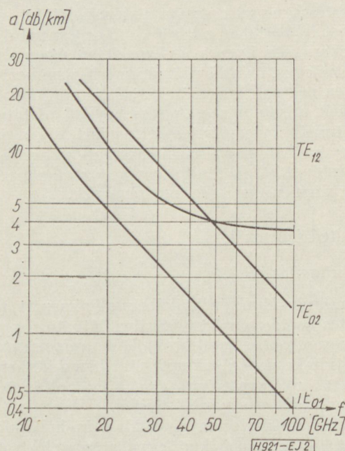
2. ábra. Körkeresztmetszetű hullámvezető csillapításmenete
