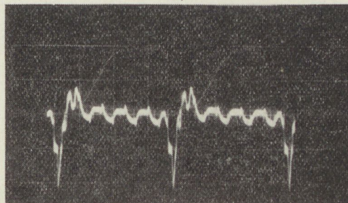
Kék vezérlés: zöld rác-katód jel Függőleges lépték: 20 V/osztás c)
