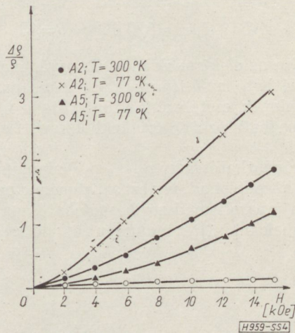
4. ábra. A mágneses ellenállás-változás térfüggése az n típusú A2 és p típusú A5 minták esetében 77 K° és 300 K° hőmérsékletnél. 300 K°-nál mindkét minta sajátvezető
