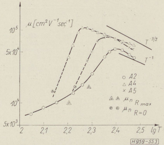
3. ábra. Az elektronmozgékonyosság hőmérsékletfüggése az n típusú A2 és p típusú A4 és A5 mintákban. Eltérő módon jelöltük az A4 és A5 mintákra az R_{\text{max}} -ból (3) alapján számított b felhasználásával kapott mozgékonyságokat (háromszög), valamint az R=0 -ból (7) alapján számított b felhasználásával kapottakat (kör)
