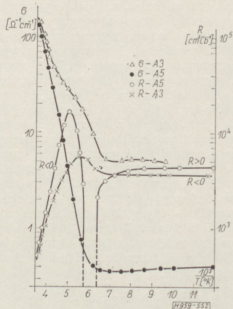
2. ábra. Az n típusú A3 és p típusú A5 minta vezetőképessége és Hall állandójának hőmérsékletfüggése 77 K° és 300 K° hőmérsékleti tartományban
