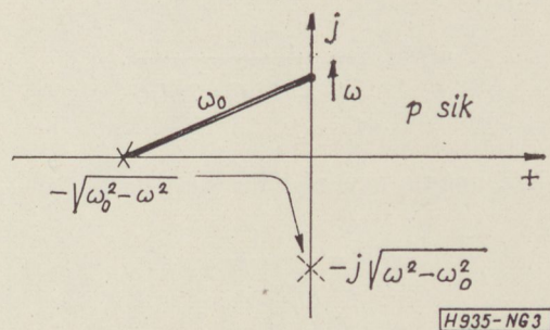
3. ábra. F(p) pólusmozgása
