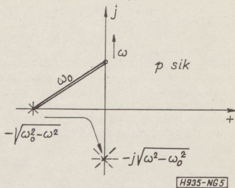
5. ábra. \psi(p) pólusmozgása
