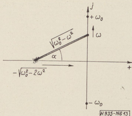
13. ábra. \psi(p) pólusmozgása
