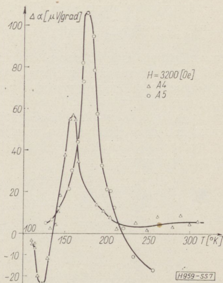
7. ábra. A longitudinális Nernst—Ettingshausen-effektus hőmérsékletfüggése 110 K° és 300 K° közötti hőmérsékleti tartományban 3200 Oe télerősségű mágneses térben
