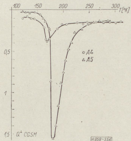
6. ábra. A transzverzális Nernst—Ettingshausen-együttható hőmérsékletfüggése a p típusú A4 és A5 mintákon 3200 Oe télerősségű mágneses térben
