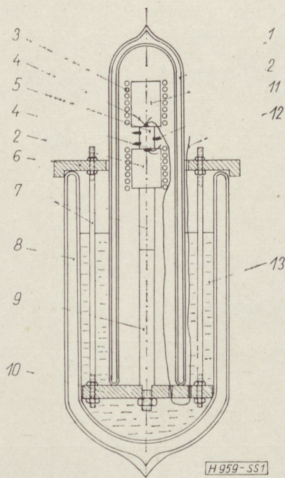
1. ábra. A Seebeck- és Nernst – Ettingshausen-jelenségek vizsgálatához használt hűtőberendezés: 1. felső Dewar-edény; 2. vörösréz tuskó; 3. fűtőtest; 4. termoelem; 5. minta; 6. plexi tartólemez; 7. sárgaréz rúd, hőhid; 8. külső, alsó Dewar-edény; 9. vörösréz tartórúd; 10. plexi alaplap; 11. kontaktus kivezetéssel; 12. kivezető vörösréz huzal; 13. folyékony nitrogén
