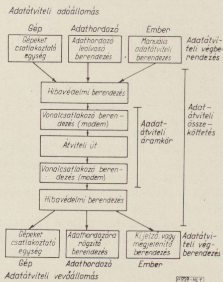
1. ábra. Az adatátvitel felépítése
