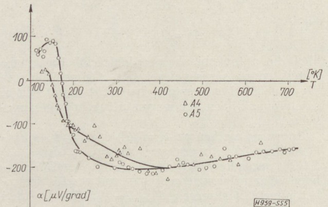
5. ábra. A termofeszültség hőmérsékletfüggése a p típusú A4 és A5 mintákban
