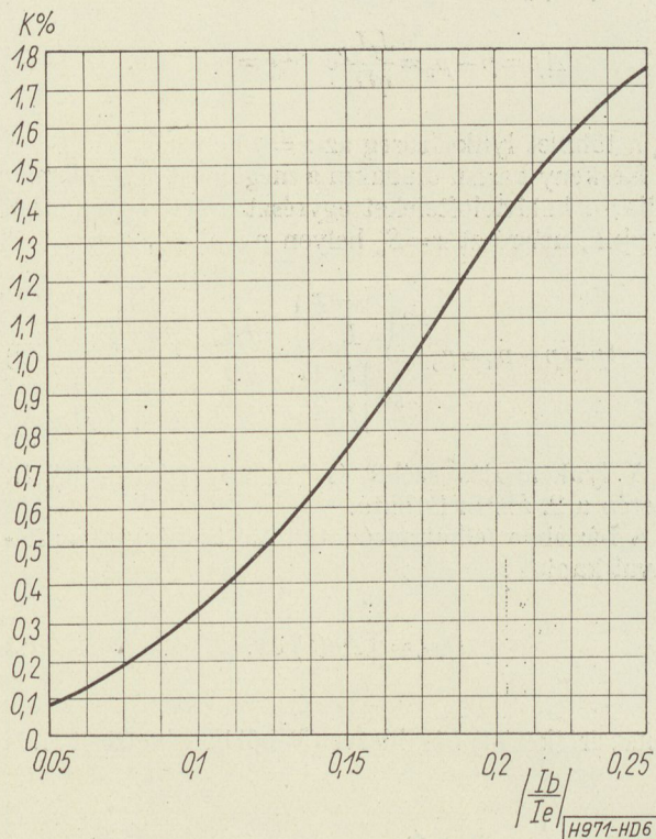
6. ábra. A négydiódás szabályozóáramkör okozta harmonikus torzítási tényező a diódán átfolyó váltakozó áram és szabályozó egyenáram viszonyának függvényében
