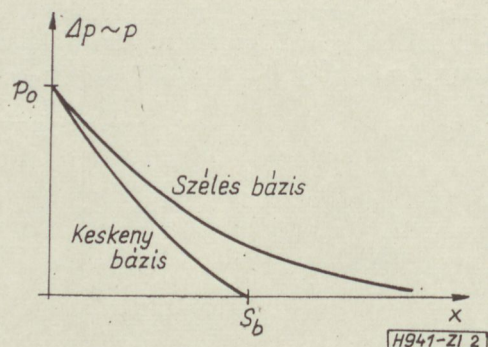
2. ábra. Lyukeloszlás a bázisban statikus esetben
