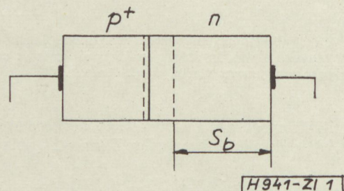
1. ábra. A p^+ - n dióda elvi felépítése
