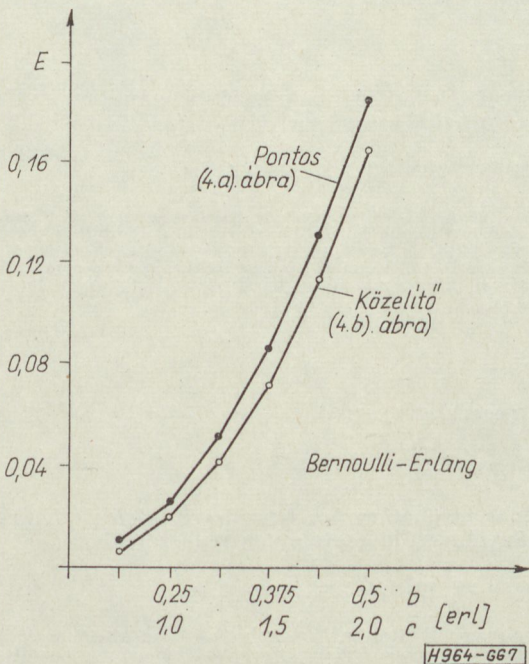
7. ábra. A pontos és a közelítő számítás összehasonlítása. A B mezőben Bernoulli-, a C mezőben Erlang-eloszlás van
