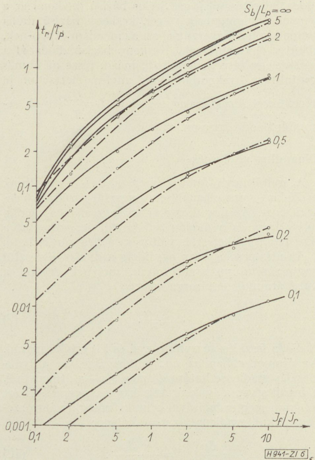
6. ábra. A pontos és a közelítő számításból adódó kikapcsolási idők különböző S_b/L_p és J_f/J_r viszonyok esetén. A pontos értékeket a folyamatos, a közelítő értékeket a szaggatott vonalak ábrázolják. Ha a közelítő értékekből adódó t_r értéket még egy kb. 1,25-ös faktoral megszorozzuk, az ábra tanúsága szerint még jobb egyezést kapunk
