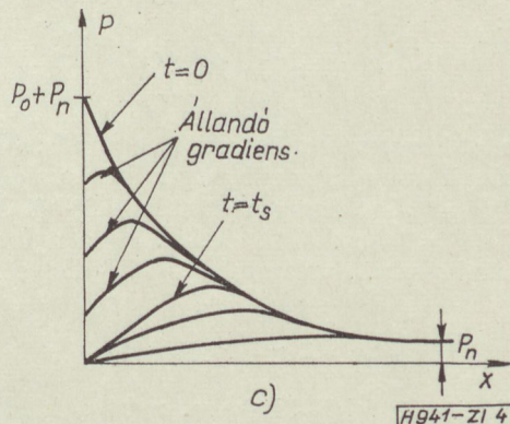
4. ábra. A kikapcsolás folyamata. a — áramalak a kikapcsolás-kor, a közelítő áramforma pont-vonallal bejelölve; b — a diódán levő feszültség alakulása a kikapcsolás folyamán; c — a bázisban levő lyuksűrűség alakulása a kikapcsolás különböző pillanataiban. A telítési idő végéhez tartozó lyukeloszlást ( t=t_s ) külön bejelöltük
