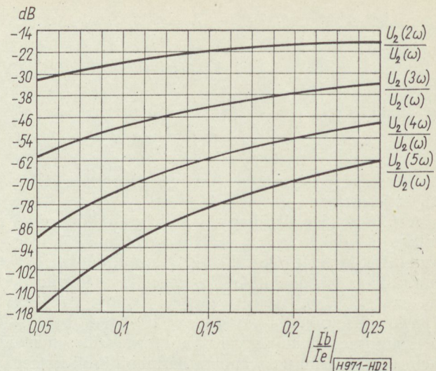
2. ábra. Az egydiódás szabályozóáramkörben keletkező felharmonikusok csillapítása az alapharmonikusra vonatkoztatva, a diódán átfolyó váltakozó áram és szabályozó egyenáram viszonyának függvényében
