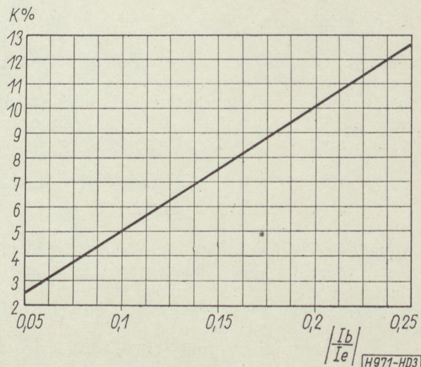
3. ábra. Az egydiódás szabályozóáramkör okozta harmonikus torzítási tényező a diódán átfolyó váltakozó áram és szabályozó egyenáram viszonyának függvényében
