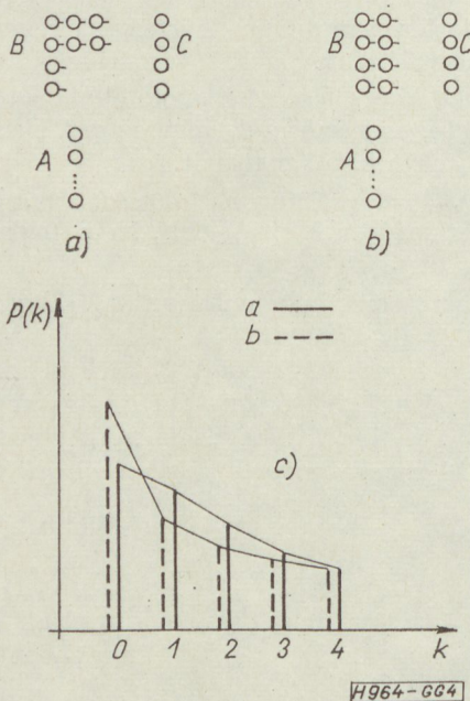
4. ábra. C) Foglalt sorok előfordulásának gyakorisága, figyelembe véve a foglalt elemek összes lehetséges elhelyezkedését
