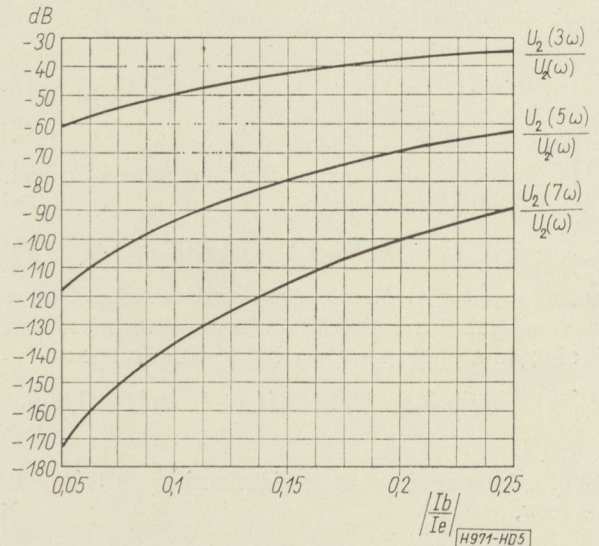
5. ábra. A négydiódás szabályozóáramkörben keletkező felharmonikusok csillapítása az alapharmonikusra vonatkoztatva, a diódán átfolyó váltakozó áram és szabályzó egyen-áram viszonyának függvényében
