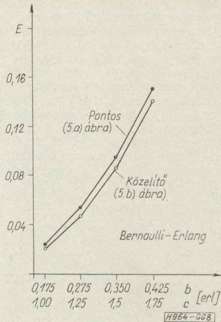
8. ábra. A pontos és a közelítő számítás összehasonlítása. A B mezőben Bernoulli-, a C mezőben Erlang-eloszlás van. A b tengelyen a beosztás nem léptékhelyes
