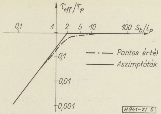
5. ábra. Az effektív élettartam alakulása a bázis normált szélességének a függvényében
