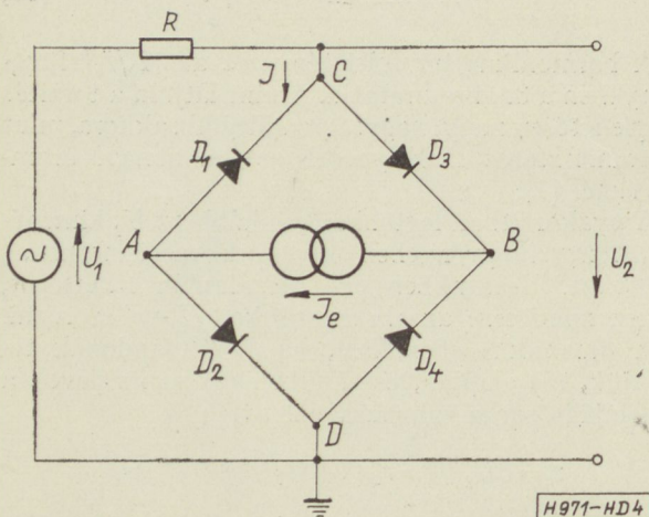
4. ábra. A négydiódás szabályozóáramkör
