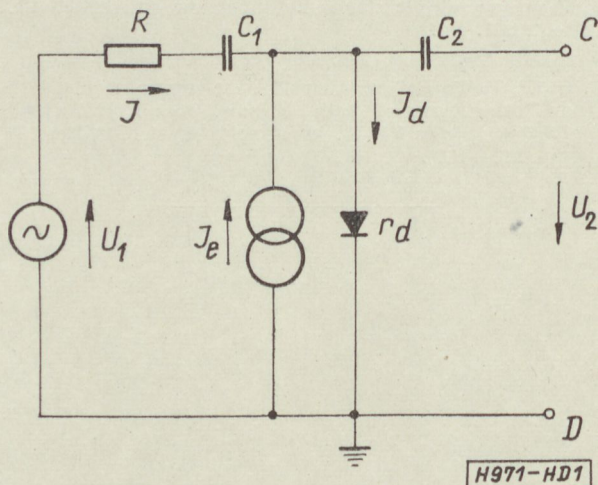
1. ábra. Egydiódás szabályozóáramkör
