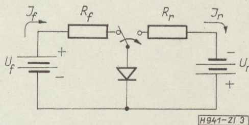
3. ábra. A kapcsoló áramkör elvi vázlata
