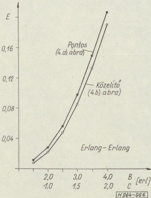
6. ábra. A pontos és a közelítő számítás összehasonlítása, a B és C mezőben egyaránt Erlang-eloszlás van
