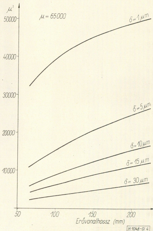
4. ábra. Nagypermeabilitású anyag magpermeabilitásának változása a légréssel
