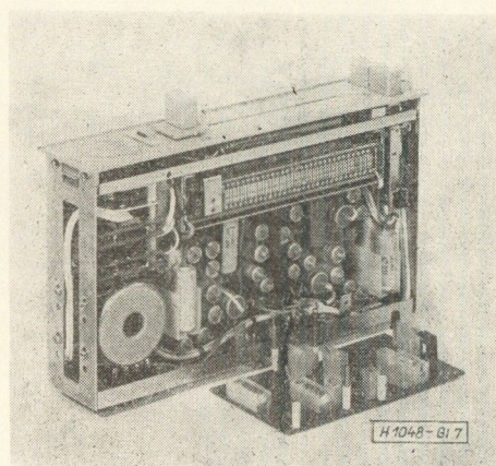
7. ábra. BEAG-erősítő betétegység toroidtranszformátorral
