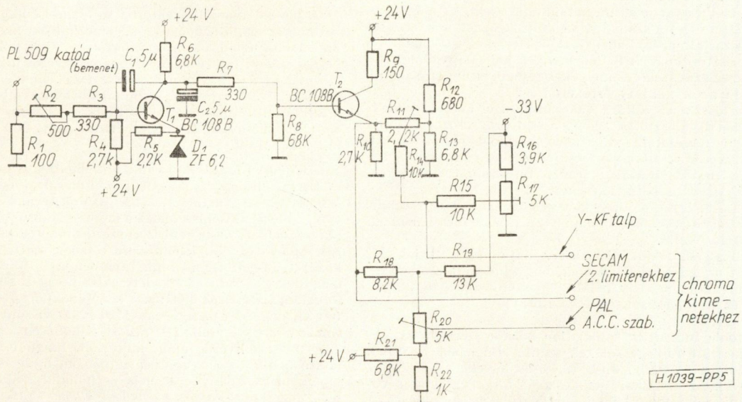
5. ábra. A korlátozó kapcsolási rajza
