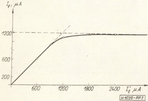
3. ábra. Szabályozási karakterisztika
