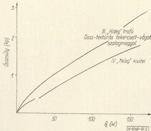
2. ábra. A transzformátor hőmérsékletének hatása a transzformátor súlyára
