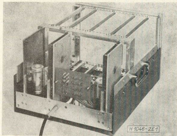
1. ábra. 12/18as műszer vázszerkezet beépített tápegységgel
