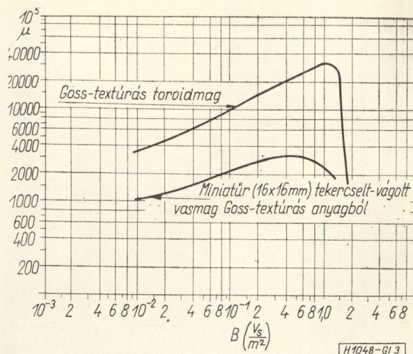
3. ábra. A légrés „nyíró-hatása” kis méretek esetén
