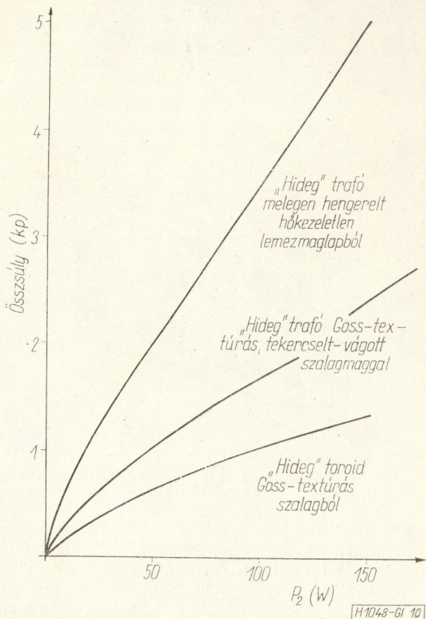
10. ábra. Lemezmaglappos, tekercselt-vágott vasmagos- és toroidmagú transzformátorok súlyadatai
