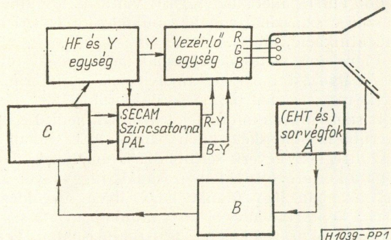
1. ábra. A korlátozó blokk sémája
