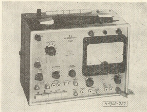
2. ábra. Színes tv Transistest Secam egységgel
