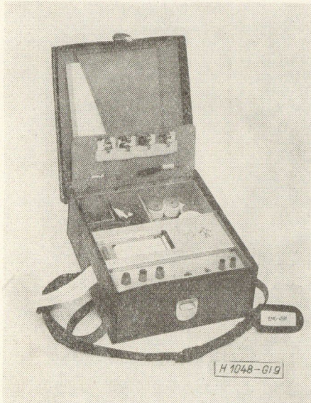
9. ábra. EMG hordozható elektrokardiográf 4,8 kg összsúllyal
