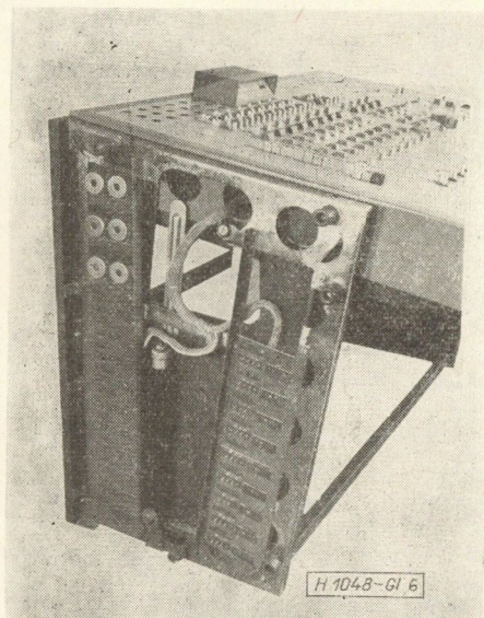
6. ábra. BEAG-gyártmányú tranzisztoros stúdióasztal toroid-illesztőtranszformátorokkal
