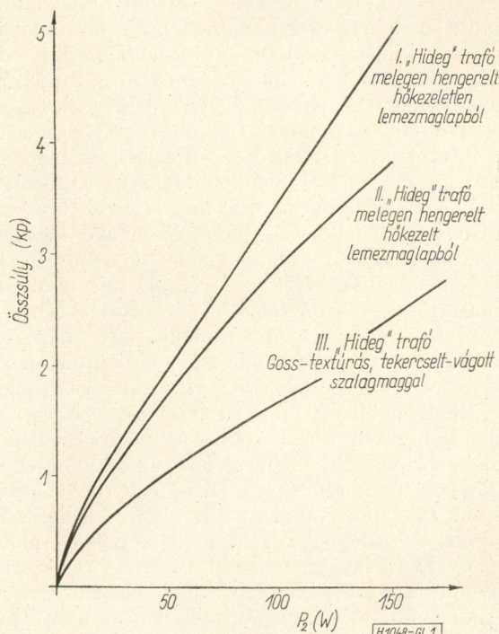
1. ábra. A súlycsökkentés mértéke Goss-textúras magok alkalmazásával
