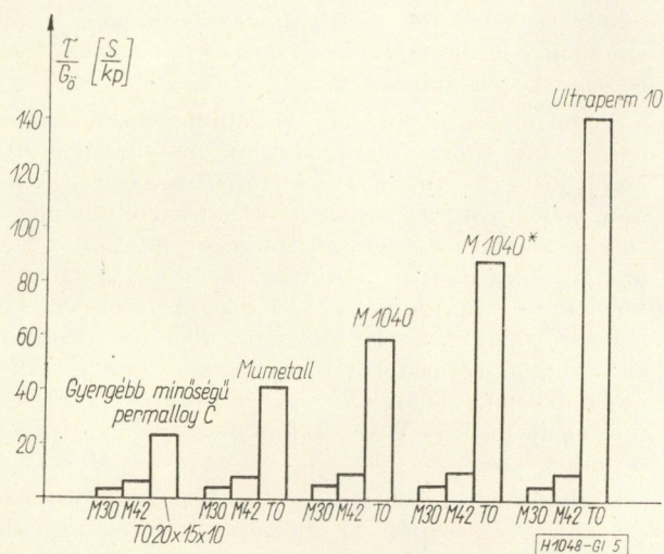
5. ábra. Különböző típusú vasmagok súlyegységre eső idő-állandói
