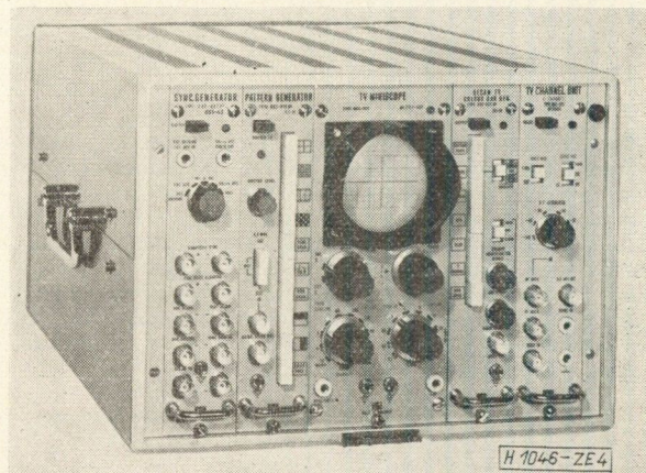
4. ábra. Színes tv Komplex generátor
