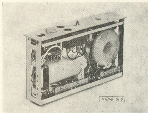
8. ábra. BEAG tápegység 60 W hasznos teljesítményű toroidtranszformátorral
