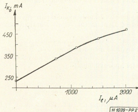
2. ábra. Érzékelő karakterisztika
