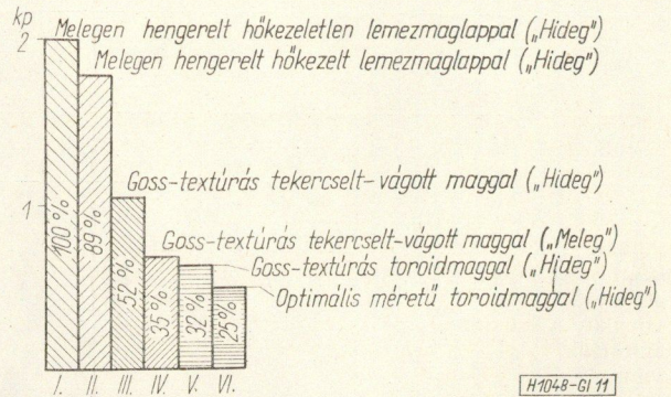
11. ábra. Különböző típusú vasmagokkal kialakított 50 W hasznos teljesítményű transzformátorok súlyviszonyai
