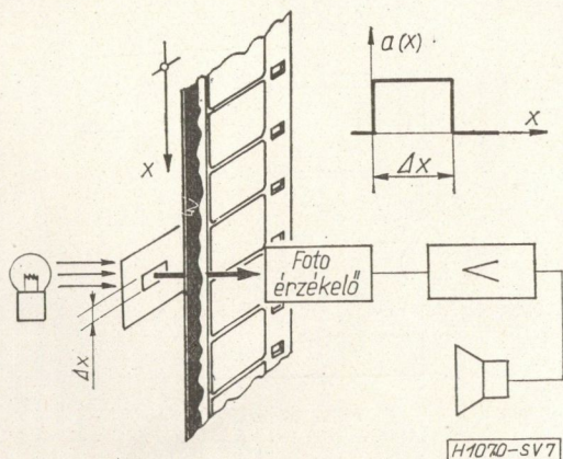
7. ábra. Az optikai hangrögzítés résfüggvény-problémája
