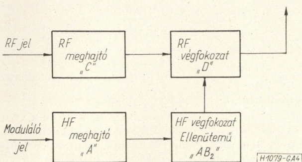
4. ábra. „D”-osztályú rádiófrekvenciás résszel, klasszikus ellenütemű AB_2 -osztályú modulátorral rendelkező adó modellje
