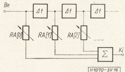
16. ábra. Reciprok ablakot megvalósító korrektor
