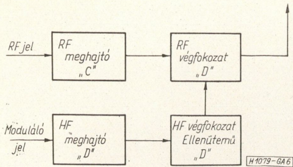
6. ábra. A legjobb teljes hatásfokot biztosító adó blokk-sémája. „D”-osztályú rádiófrekvenciás és ellenütemű „D”-osztályú hangfrekvenciás rész
