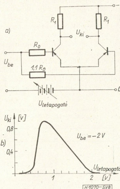
8. ábra. a) egyszerű amplitúdósűrűség-mérő, b) a letapogató ablak
