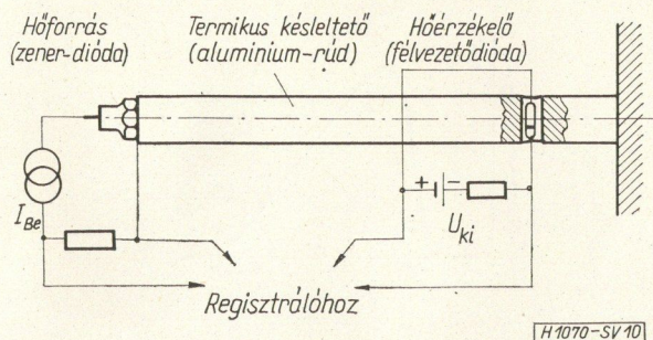
10. ábra. Termikus késleltetővonal vázlata
