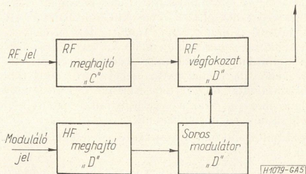
5. ábra. „D”-osztályú rádiófrekvenciás résszel soros „D”-osztályú modulátorú adó blokkismája
