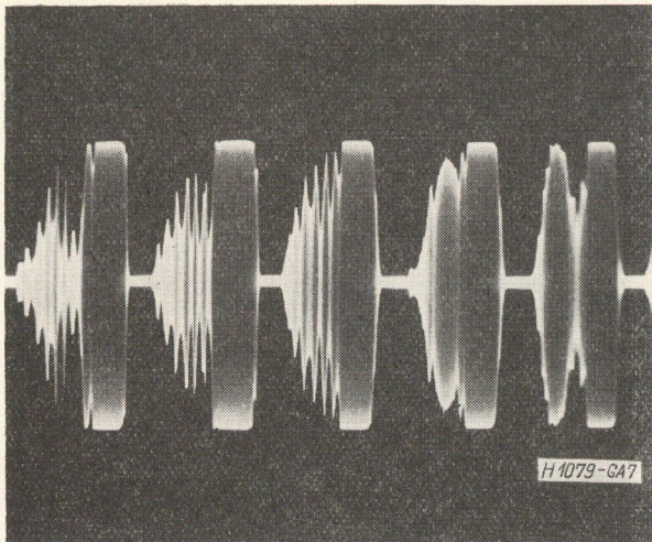
7. ábra. A 3. ábrán látható modulált adó által kisugárzott rádiófrekvenciás jel burkolója trapézmoduláció esetén.
