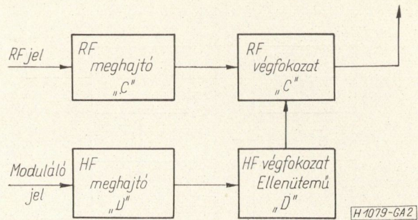
2. ábra. Klasszikus felépítésű rádiófrekvenciás résszel ellenütemű „D”-osztályú modulátorral rendelkező adó blokkismája
