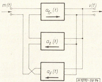
14. ábra. Reciprok súlyfüggvényt megvalósító hálózat
