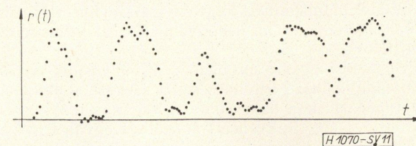
11. ábra. A termikus késleltetővonal v(t) gerjesztése, m(t) kimeneti függvénye és az r(t) javított kimeneti függvény
