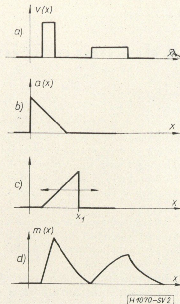
2. ábra. a) valódi függvény, b) ablakfüggvény, c) letapogatás ablak az x_1 pozícióban, d) mért függvény
