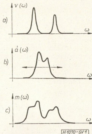
1. ábra. a) valódi spektrum, b) az analizátor átvitele, c) mért spektrum
