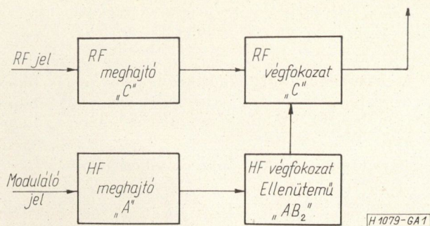
1. ábra. Klasszikus felépítésű adó blokkismája
