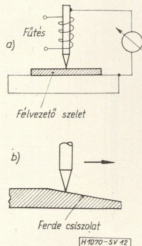
12. ábra. Fajlagos ellenállás melegtűs mérése
