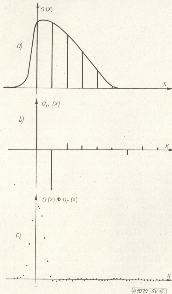
15. ábra. a) ablakfüggvény és közelítése Dirac-deltákkal, b) közelítő reciprok ablakfüggvény, c) ablak és közelítő reciprok ablak konvolúciója
