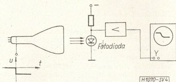
4. ábra. Utánvilágítási függvény mérése
