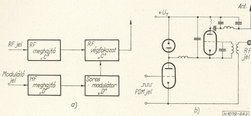
3. ábra. A GATES cég által forgalmazott adó modellje. Klasszikus rádiófrekvenciás rész soros „D”-osztályú modulátor
