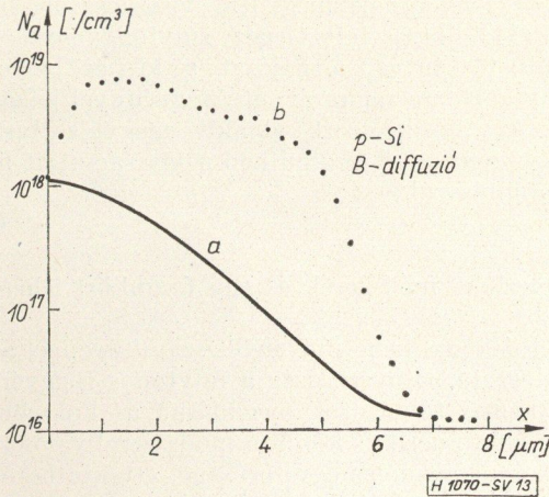
13. ábra. Szennyezés-koncentráció a mélység függvényében: a) közvetlen mérési eredmények, b) dekonvolúcióval javított eredmények
