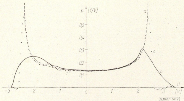
9. ábra. Színusz hullám amplitúdóspektruma: a) ideális sűrűségfüggvény, b) mért függvény, c) dekonvolúcióval javított eredmény
