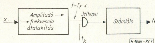
7. ábra. A/D konverzió amplitúdó-frekvencia átalakítással
