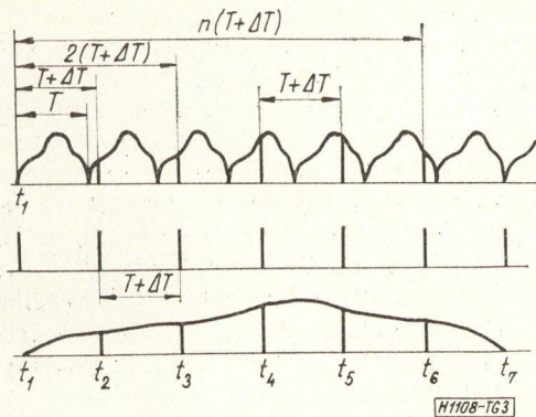
3. ábra. Jelátalakítás stroboskopikus módszerrel
