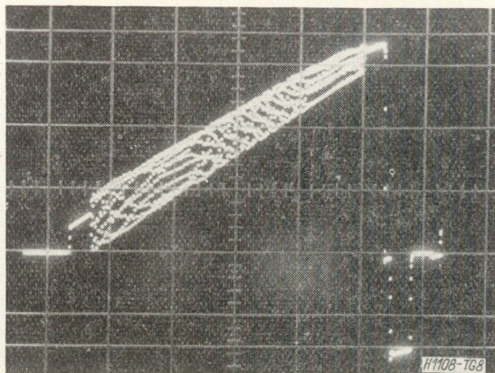
8. ábra. Linearitásmérő jelet tartalmazó átalakított vizsgáló-sor. Az 1,2 MHz frekvenciájú szuperponált szinuszjelből a mintavétel a fáziskötés hiánya miatt véletlenszerűen történt
