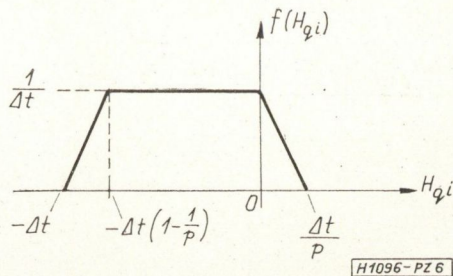
6. ábra. Az 5. ábra szerinti időintervallum kvantálás hibájának sűrűségfüggvénye (trapéz-eloszlás)
