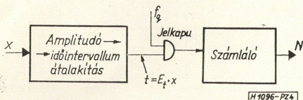
4. ábra. A/D konverzió időintervallum kvantálással
