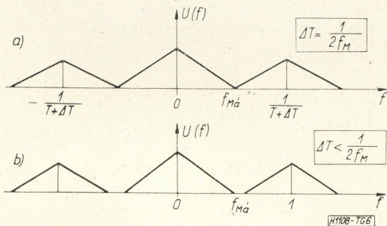
6. ábra. Az átalakított jel spektruma
