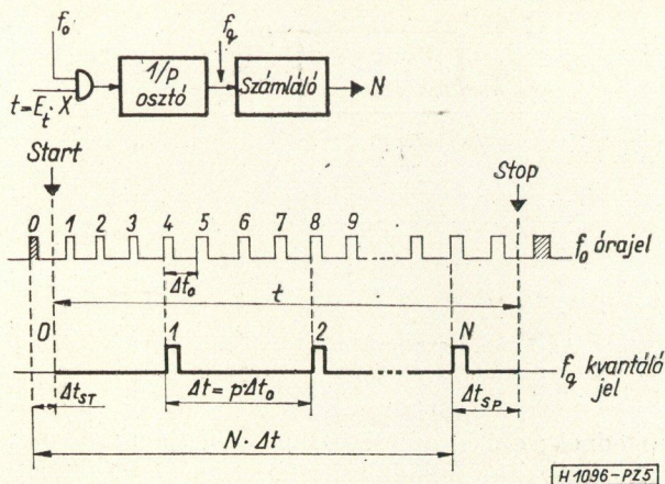
5. ábra. Időintervallum kvantálás kapuzás utáni osztással ( p=4 )
