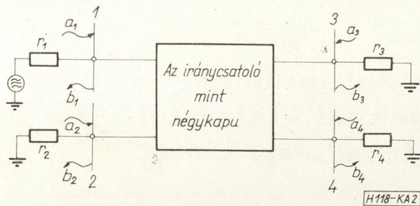
2. ábra. Az iránycsatoló mint négykapu áramkör, 1 — a bemenő kapu; 2 — csatolt kapu; 3 — az átviteli kapu; 4 — izolált kapu
