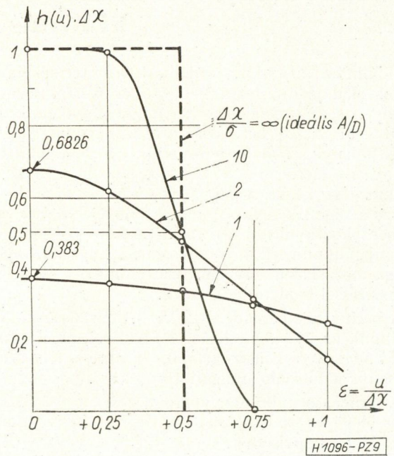
9. ábra. Nem-ideális A/D konverter hibájának (u) normalizált sűrűségfüggvénye
