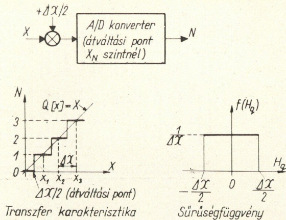
1. ábra. A/D konverter optimális kvantálási hibával ( +\Delta X/2 eltolással)
