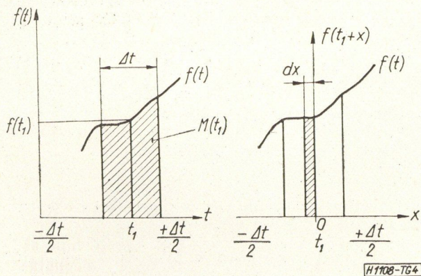
4. ábra. A mintavétel hibájának számításához
