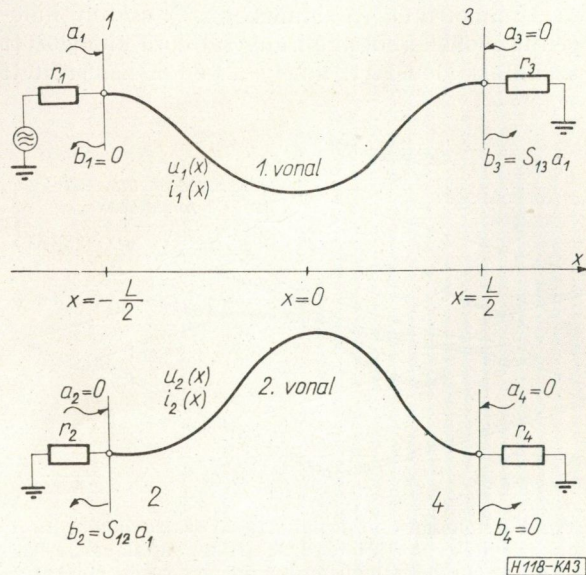
3. ábra. Csatlott inhomogén szalagvonalak
