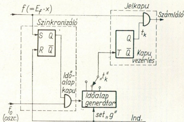
8. ábra. „Szinkronizált” jelkapu nyitás a kvantálási hiba csökkentésére (digitális frekvenciamérés)
