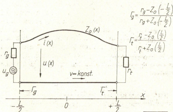
5. ábra. Inhomogén vonal analíziséhez
