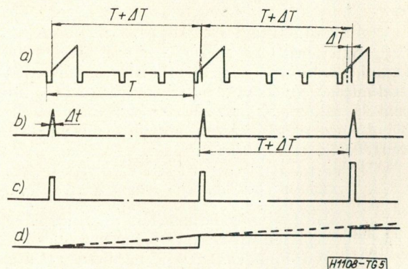
5. ábra. Vizsgálósor átalakítása
