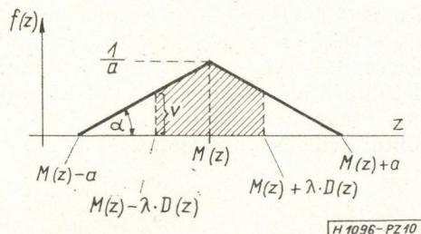
10. ábra. Simpson eloszlás
