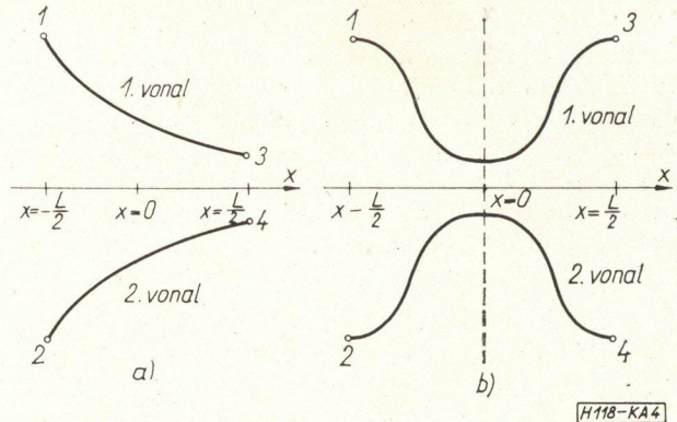
4. ábra. Aszimmetrikus és kétszeresen szimmetrikus iránycsatoló, a — az aszimmetrikus és b — a kétszeresen szimmetrikus iránycsatoló vázlata
