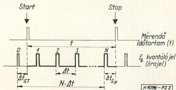
2. ábra. Időintervallum kvantálás
