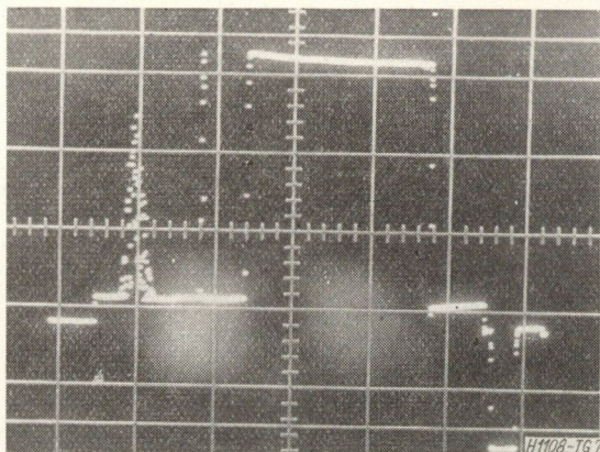
7. ábra. Stroboszkopikus mintavétellel átalakított vizsgáló-sor. A vizsgáló-sor 2T és 20T impulzust és sorfrekvenciás négyszög-jelet tartalmaz. Időlépték: 5 sec/cm, feszültséglépték: 0,2 V/cm
