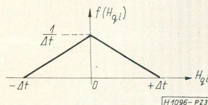
3. ábra. A 2. ábra szerinti időintervallum kvantálás hibájának sűrűségfüggvénye (Simpson eloszlás)
