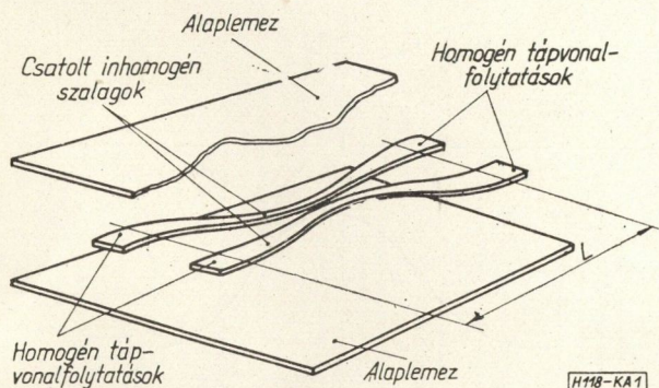
1. ábra. Folytonosan csatolt inhomogén szalagvonalas iránycsatoló felépítése. A kitöltő dielektrikum általában szilárd közeg, ezt az ábrából az egyszerűbb rajzolás végett elhagytuk.
