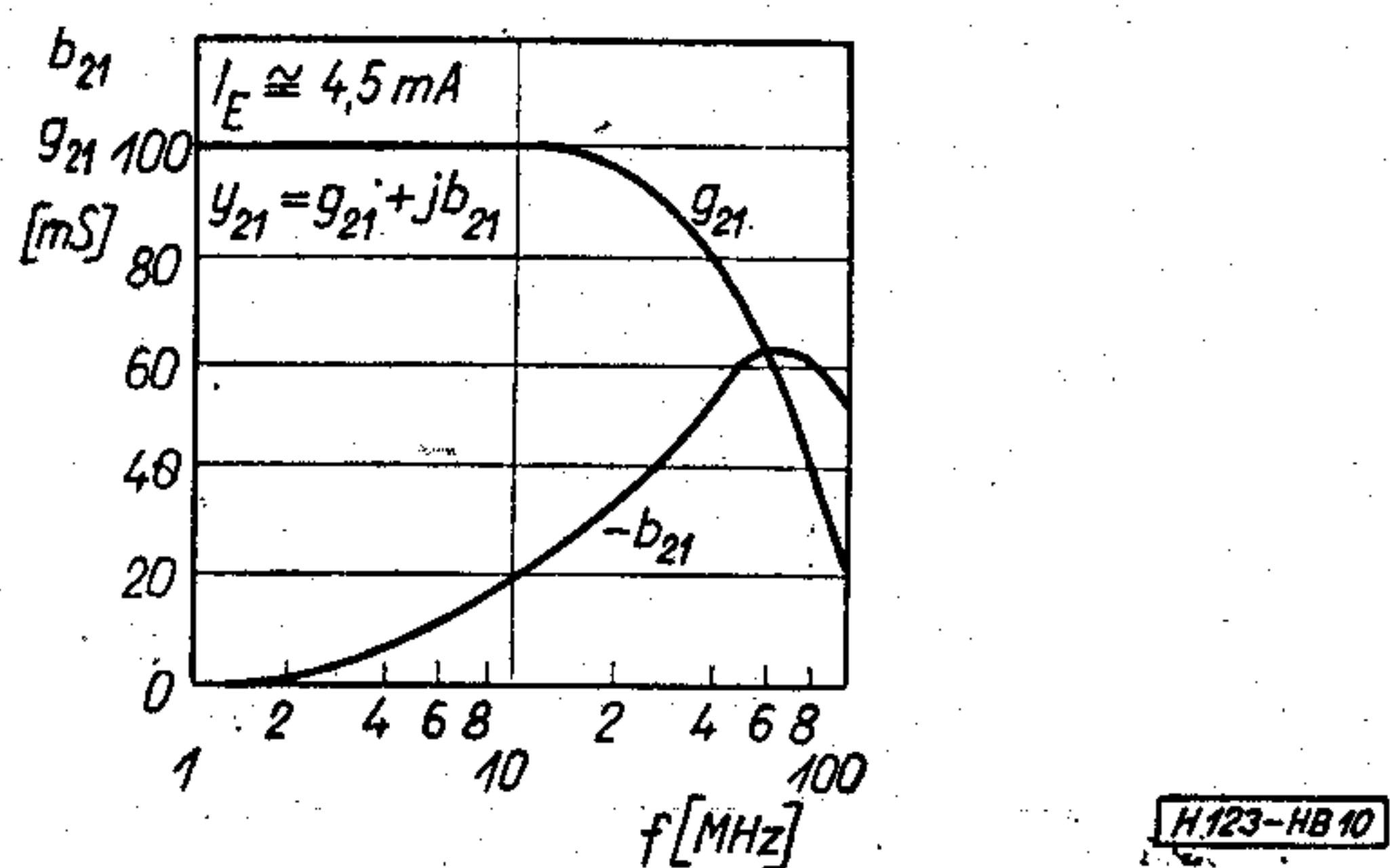
10. ábra. CA 3028A kaszkód üzemi vezetésparaméterei
