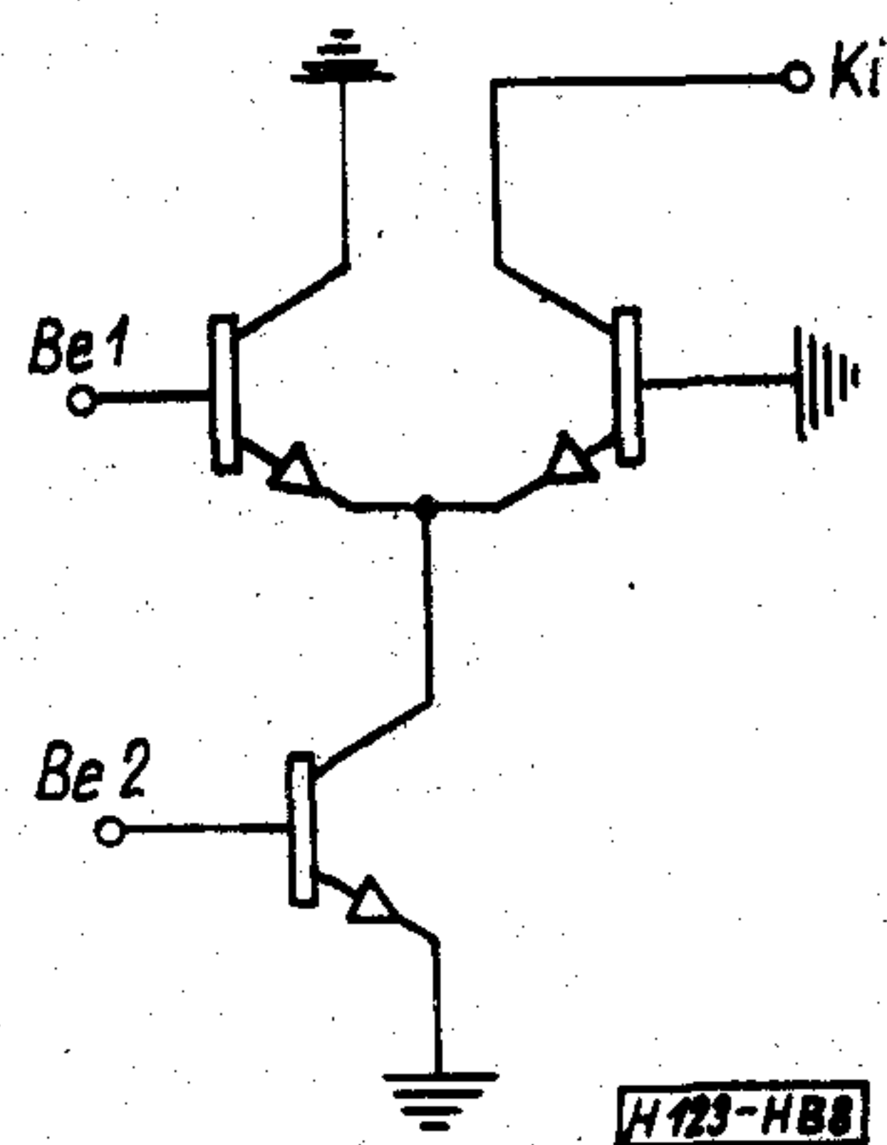
8. ábra. Kettős vezérlésű erősítőfokozat
