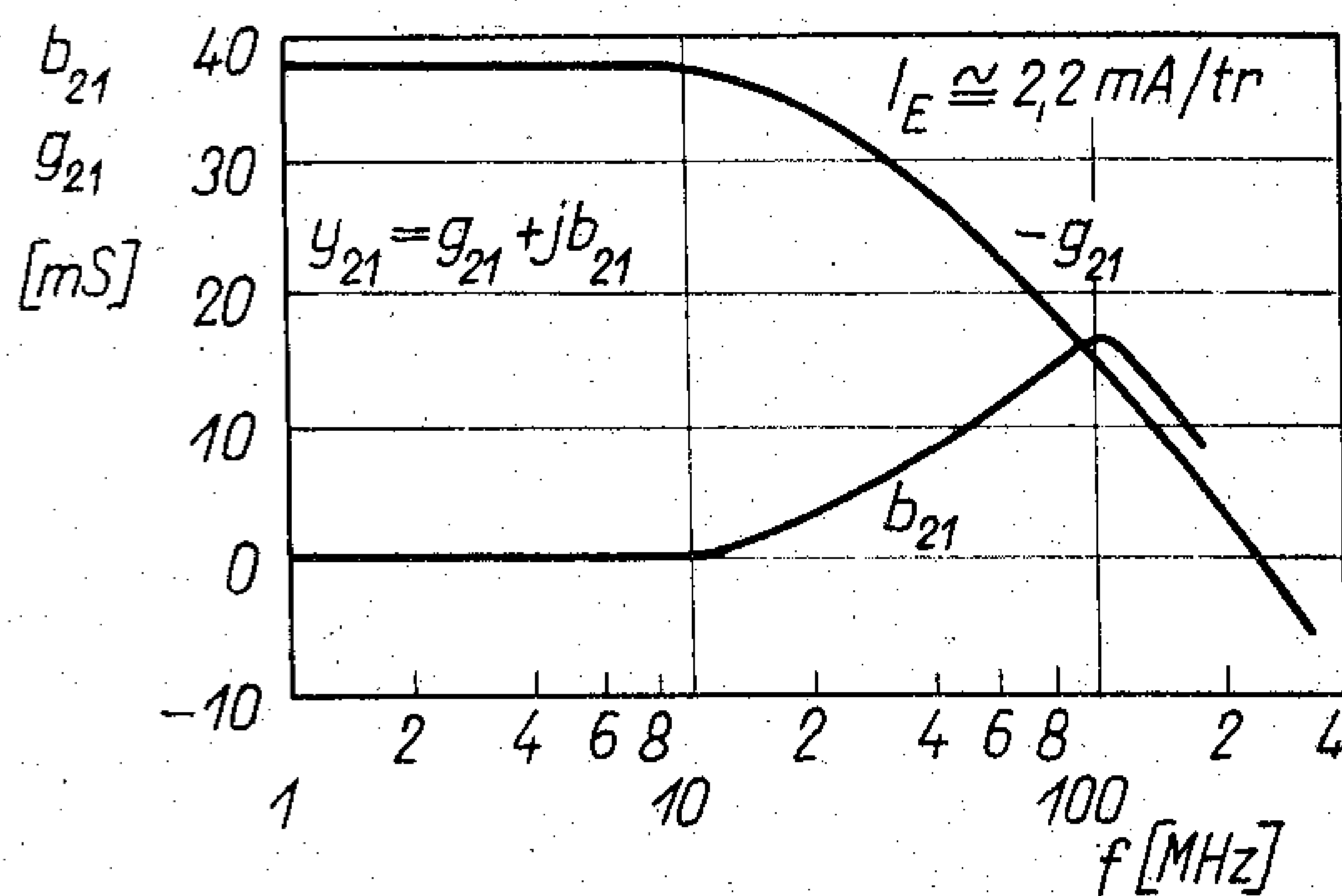
9. ábra. CA 3028A differenciálerősítő üzemi vezetésparaméterei
