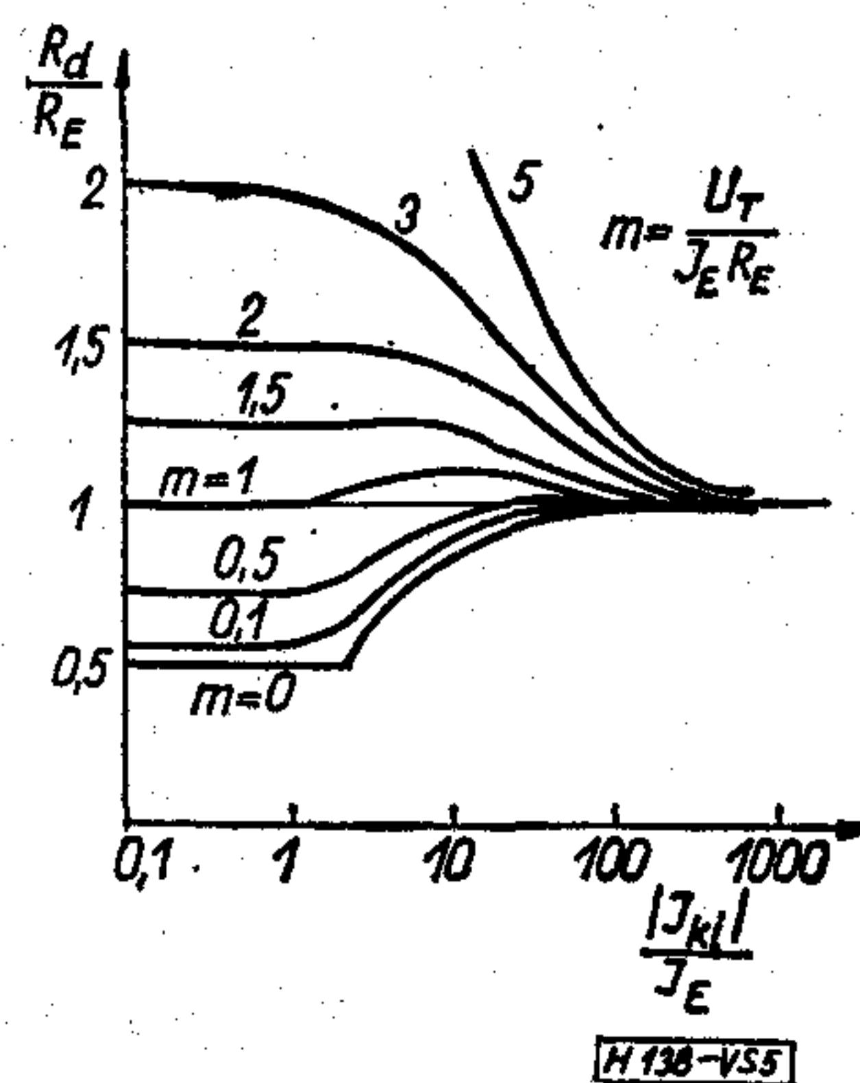
5. ábra. Az R_d ellenállás változása a kivezérés függvényében
