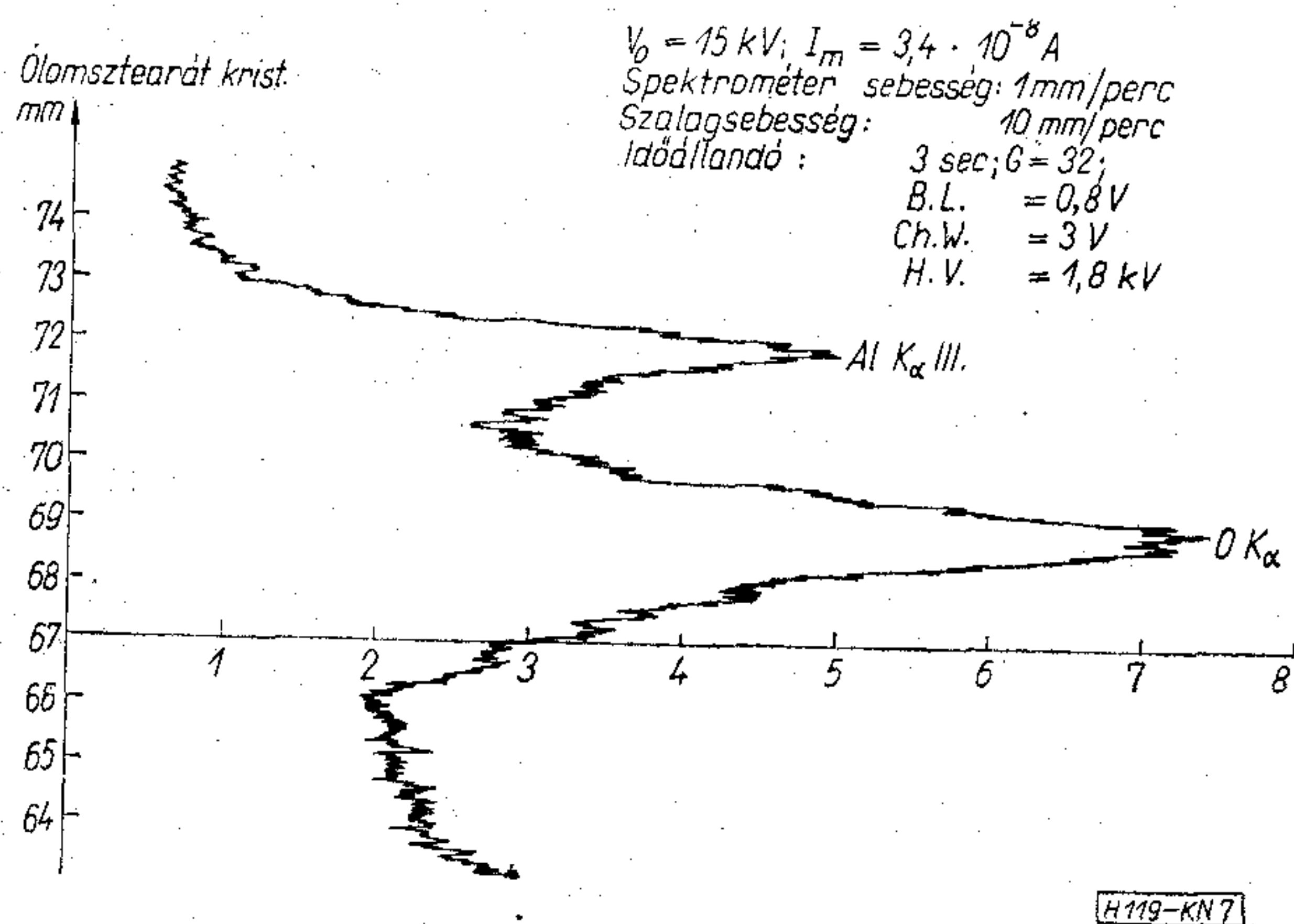
4. ábra. Oxidálódott alumíniumkontaktus röntgenspektrumában az OK_{\alpha} csúcsa és az AlK_{\alpha} harmadrendű csúcsa
