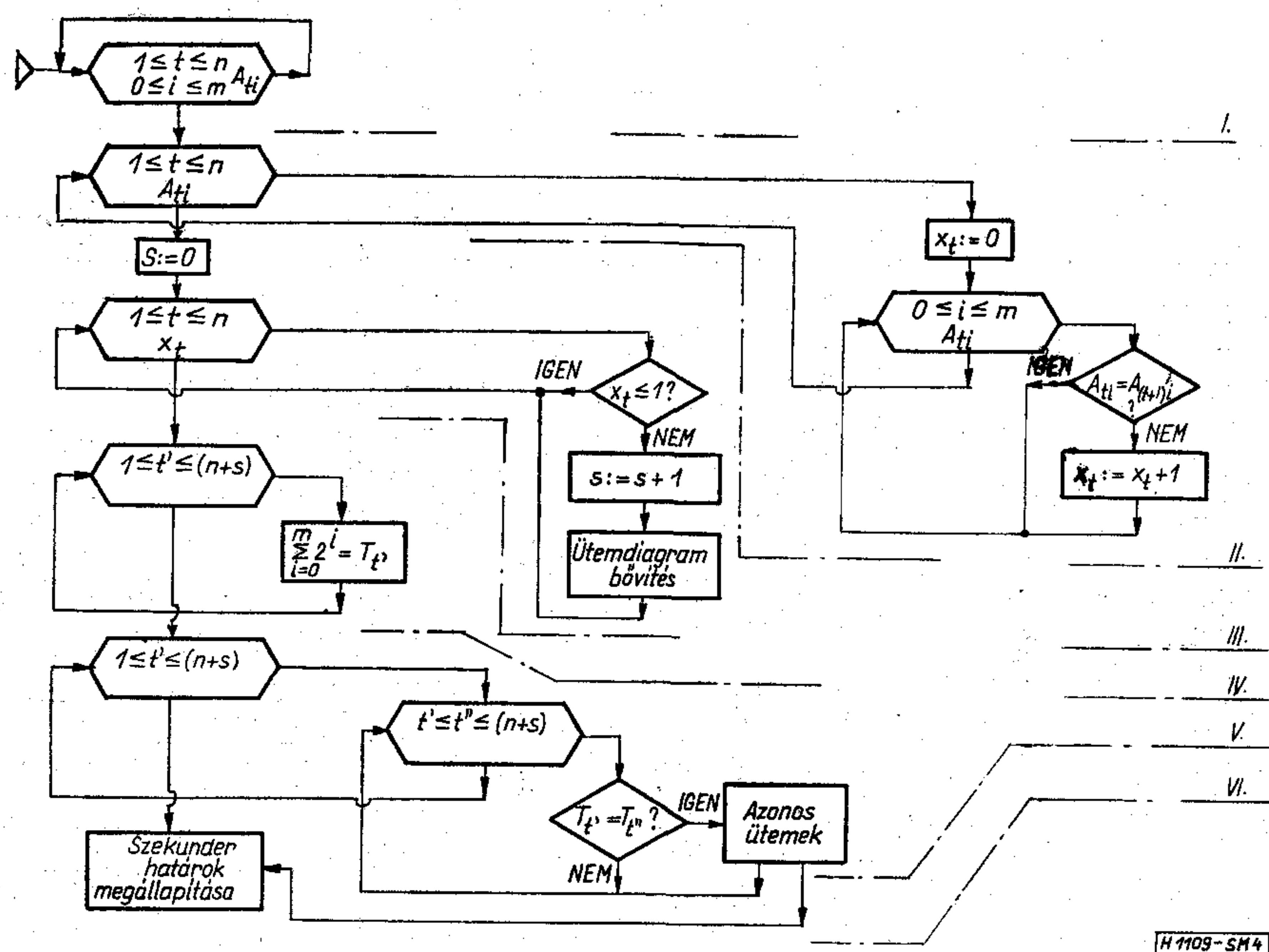
4. ábra. Tömbvázlat
