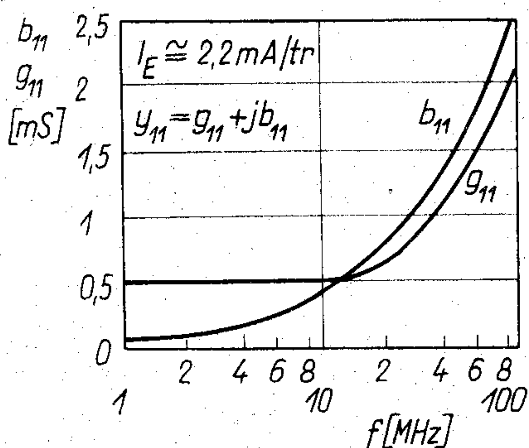
9. ábra. CA 3028A differenciálerősítő üzemi vezetésparaméterei
