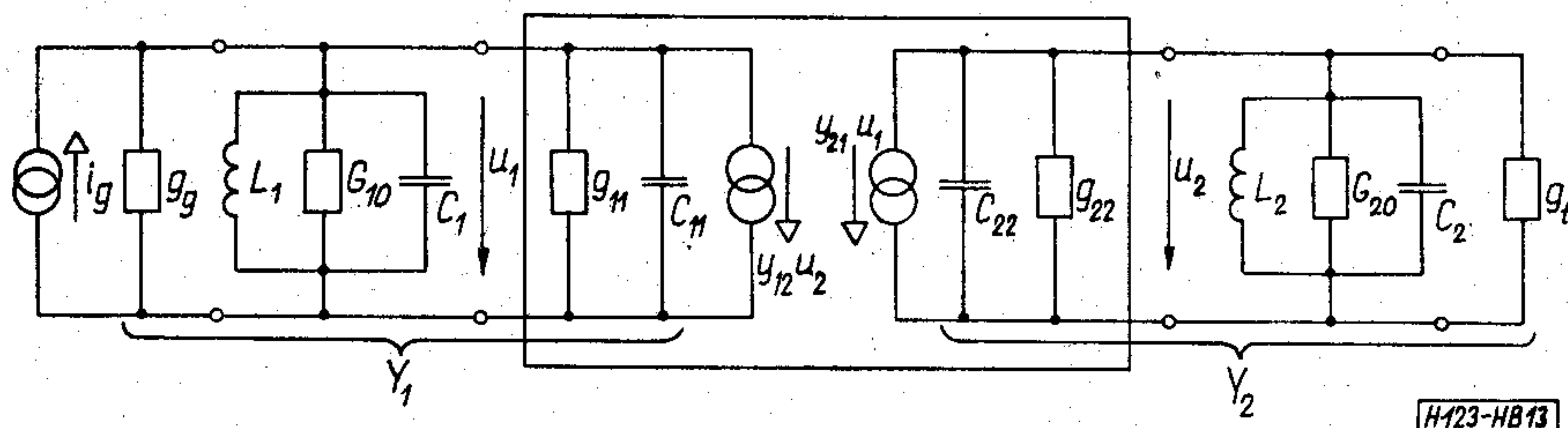
13. ábra. A teljesítményerősítés számításához
