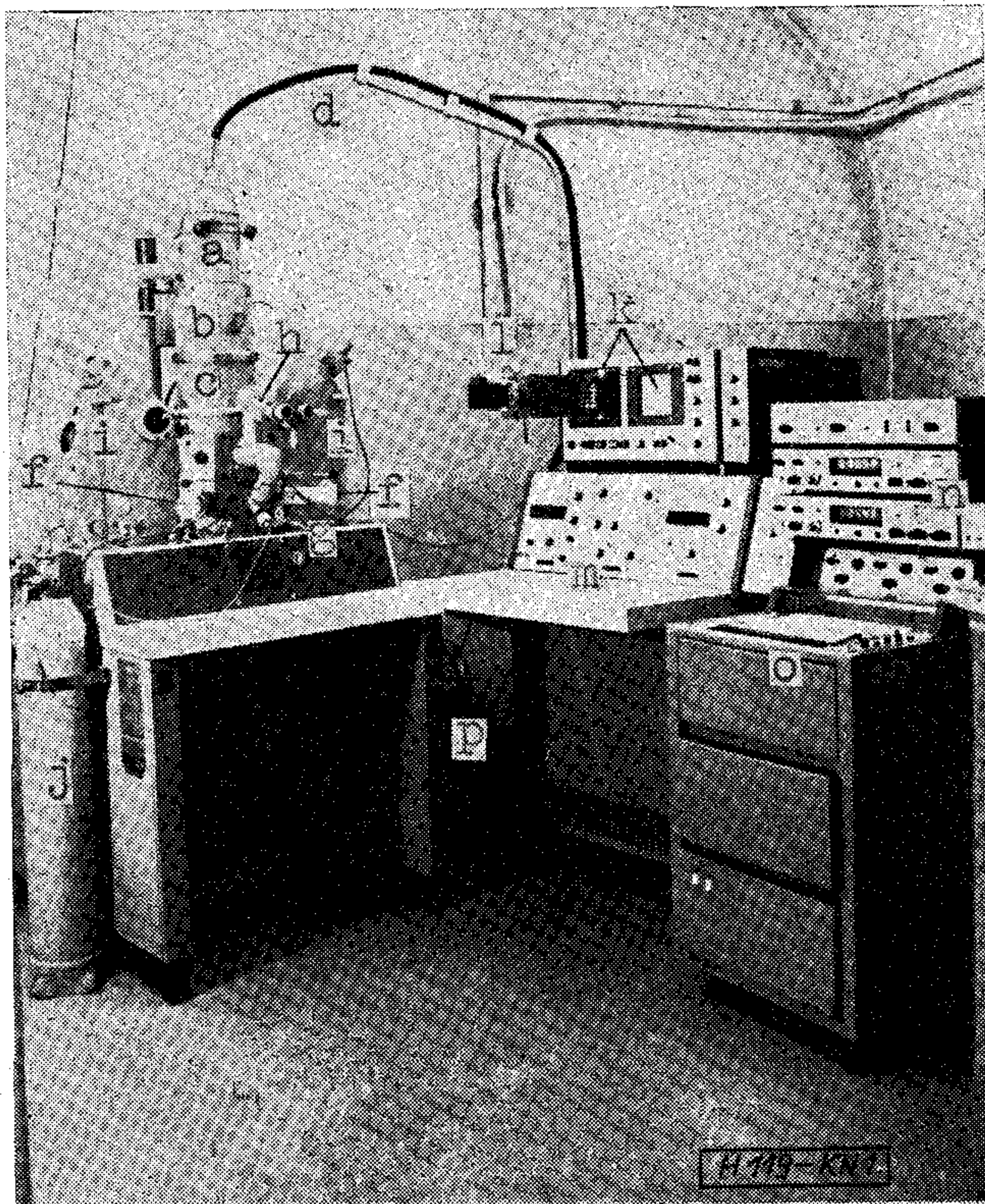
1. ábra. a) Elektronágyú — b) kondenzor — c) objektív — d) nagyfeszültségű kábel — f) vízszintes mintamozgató orsók — g) függőleges irányú mintamozgató csavar — h) mikroszkóp — i) röntgenspektrométerek — j) a proporcionális számláló gázpalackja — k) képernyők — l) fényképezőfeltét fényképezőgéppel — m) az elektronoptikai rendszer kezelőasztala — n) impulzuselemző és -számláló rendszerek — o) regisztráló — p) rotációs vákuumszivattyú
