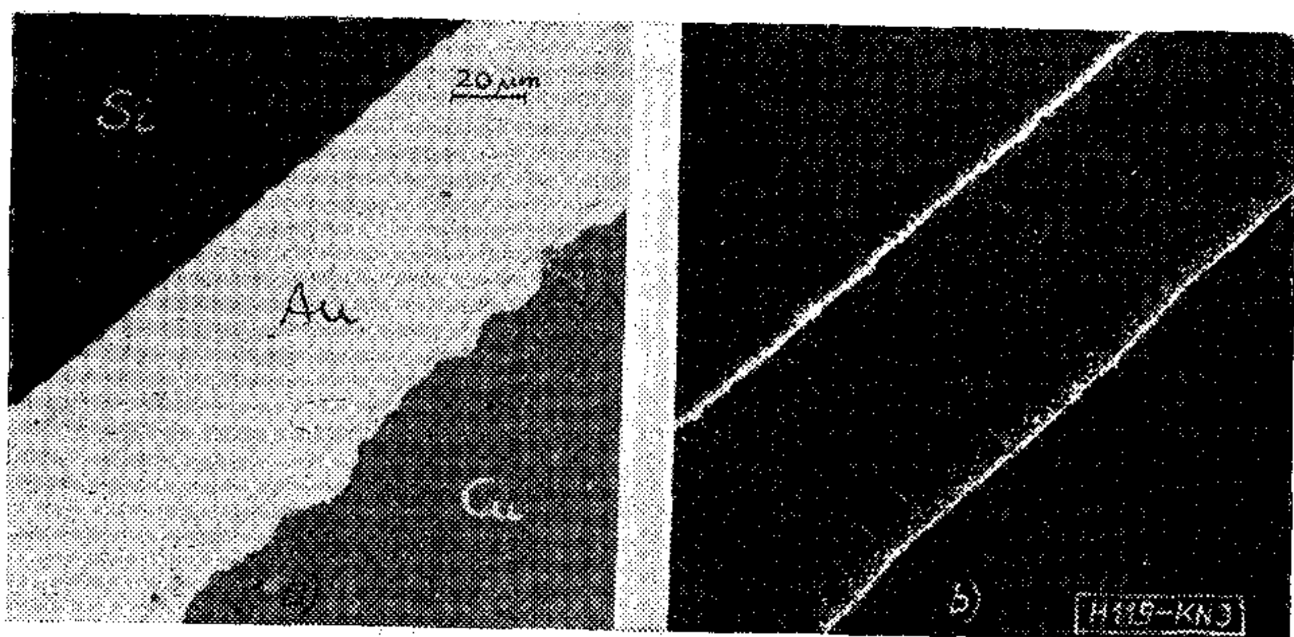
3. ábra. Félvezető eszköz kontaktusának keresztmetszete. a) Kompozíció — b) Ni K_{\alpha} kép. A szilíciumlapka és az aranyréteg között, továbbá az arany a réztuskó felé eső szélénél vékony nikkelréteg helyezkedik el
