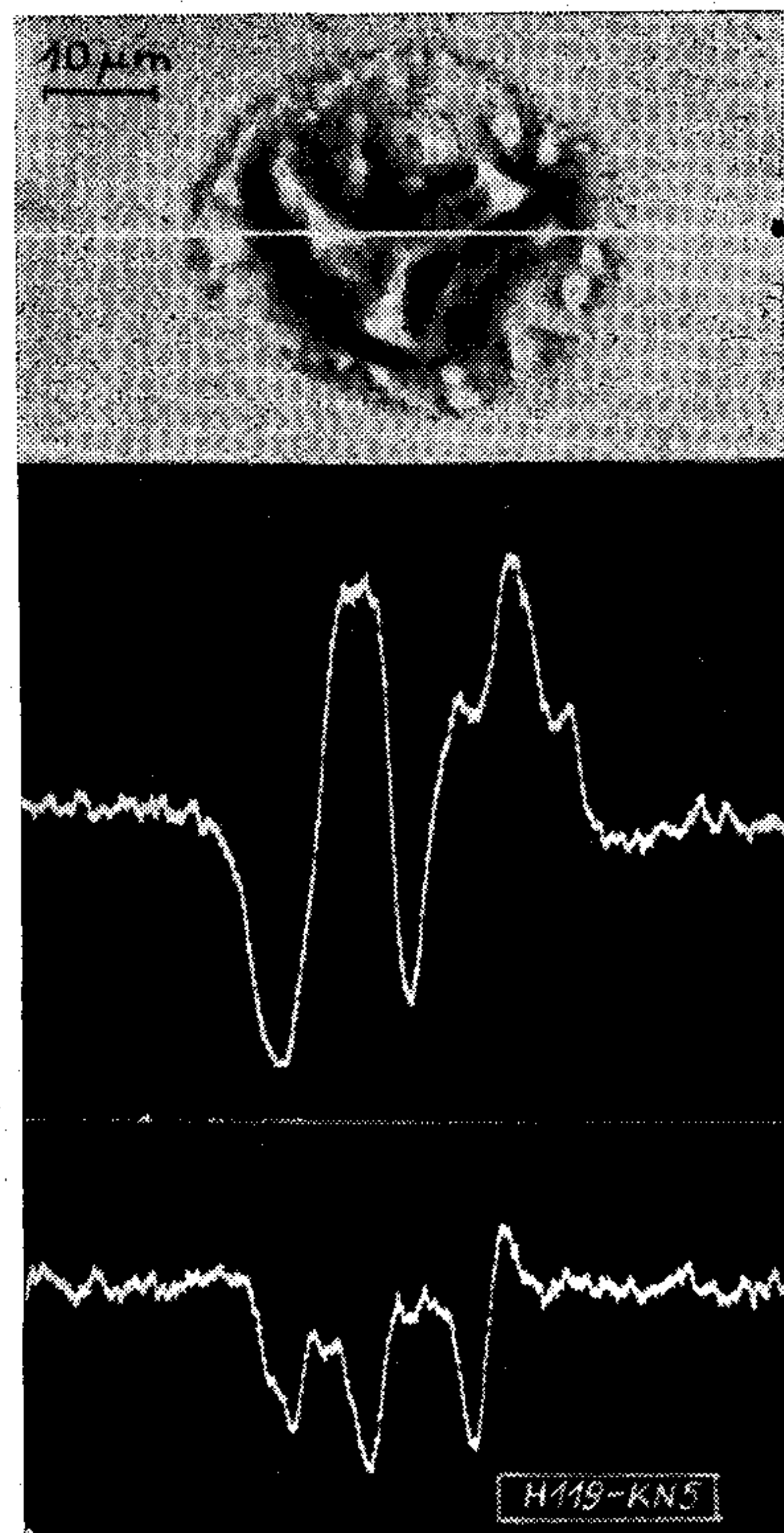
6. ábra. Al-tartalmú alakzat. Fönt: kompozíció és elemzési vonal. Középen: az Al eloszlása az elemzési vonal mentén. Lent: a háttér az elemzési vonal mentén. Az alakzat kívül nincs alumínium, ott csak az egyenletes háttér látszik. Az alakzat felületi domborzata helyenként leárnyékolja mind az \text{Al K}_\alpha sugárzását, mind a háttérét.
