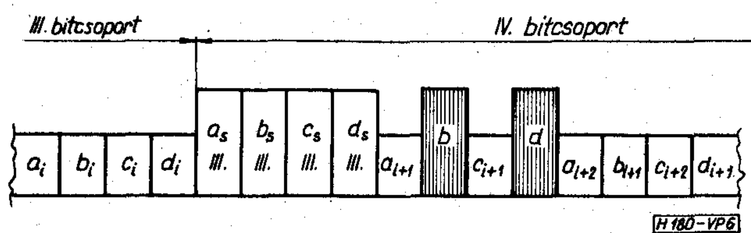
6. ábra. A szekunder multiplex vonali jel keretszerkezetének egy részlete. Az a és c primer jelek esetében pillanatnyilag nem történt stuffbeavatkozás, a b és d primer jelek esetében viszont történt
