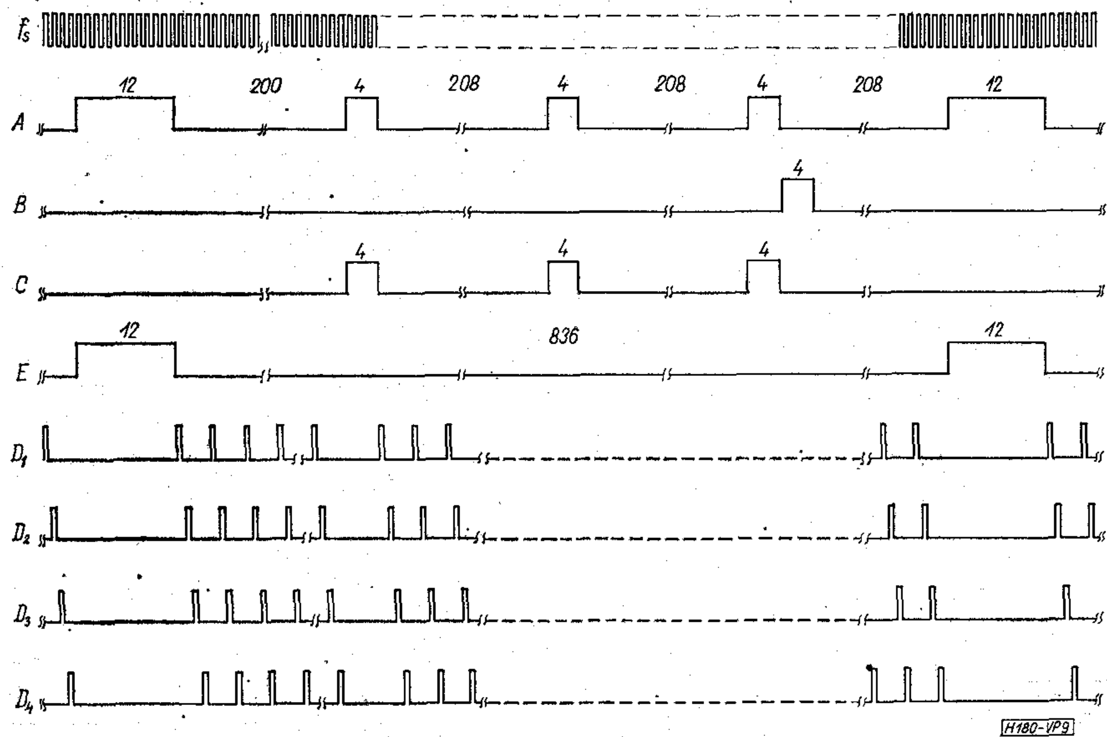
9. ábra. A szekunder digitális multiplex adó- és vevőoldalán fellépő főbb jelalak időrend szerinti ábrázolása. f_s = szekunder órajel, A = a szekunderkeret megszervezését szolgáló jelek, B = a stuffingbeavatkozás lehetséges pillanatait kijelölő jel, C = a stuffingjelzés időpillanatait kijelölő jel, D_i = a rugalmas tárolóból való kiolvasás (adóoldalon) és a rugalmas tárolóba való beírás (vevőoldalon) időpontjait meghatározó jelek, E = a keretszinkronszavak helyét kijelölő jel
