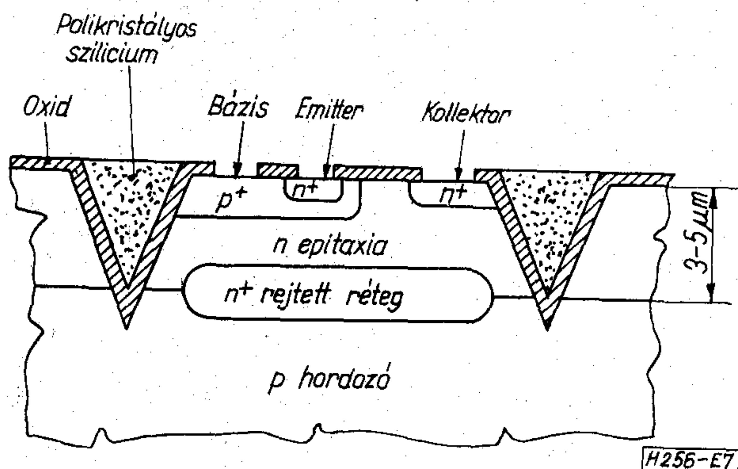
7. ábra. VIP vagy polyplanár technológiával kialakított tranzistor szerkezete
