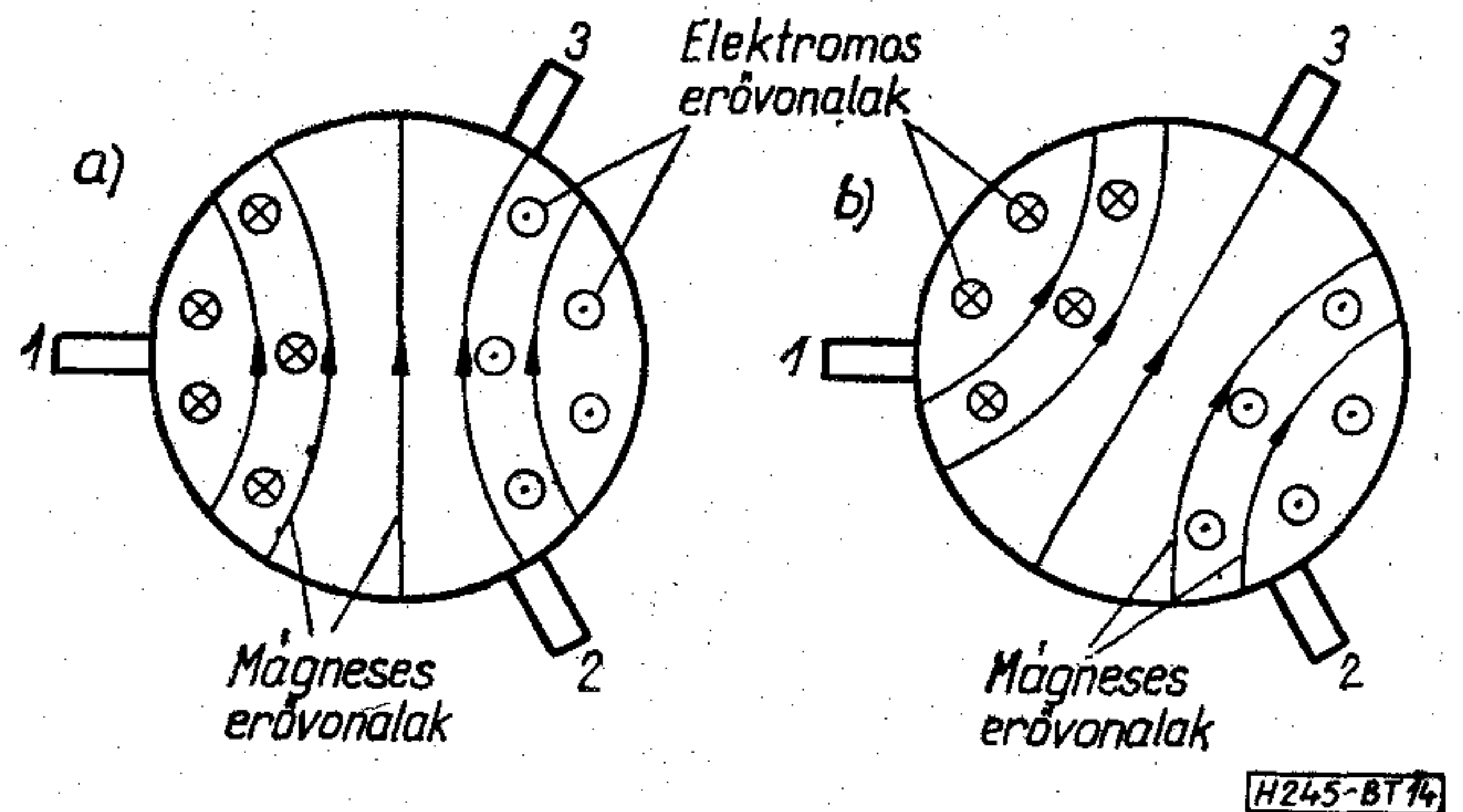
14. ábra. Tárcsarezonátor alpmódusának erővonalképe: a) polarizáló mágneses tér nélkül, b) polarizáló mágneses tér jelenlétében
