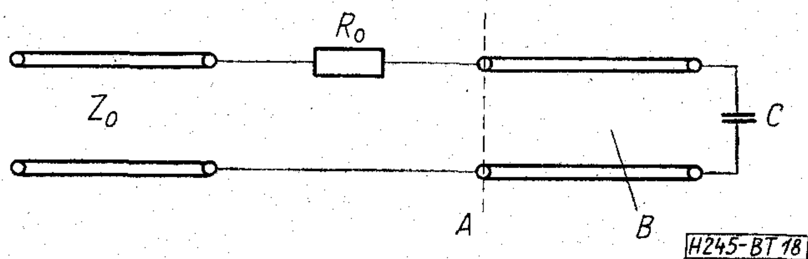
18. ábra. Illesztett lezáró helyettesítő kapcsolása
