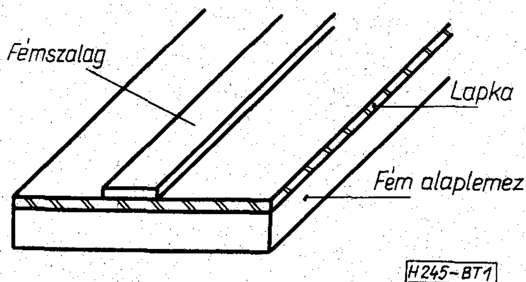
1. ábra. Mikroszalag-tápvonal vázlatos rajza
