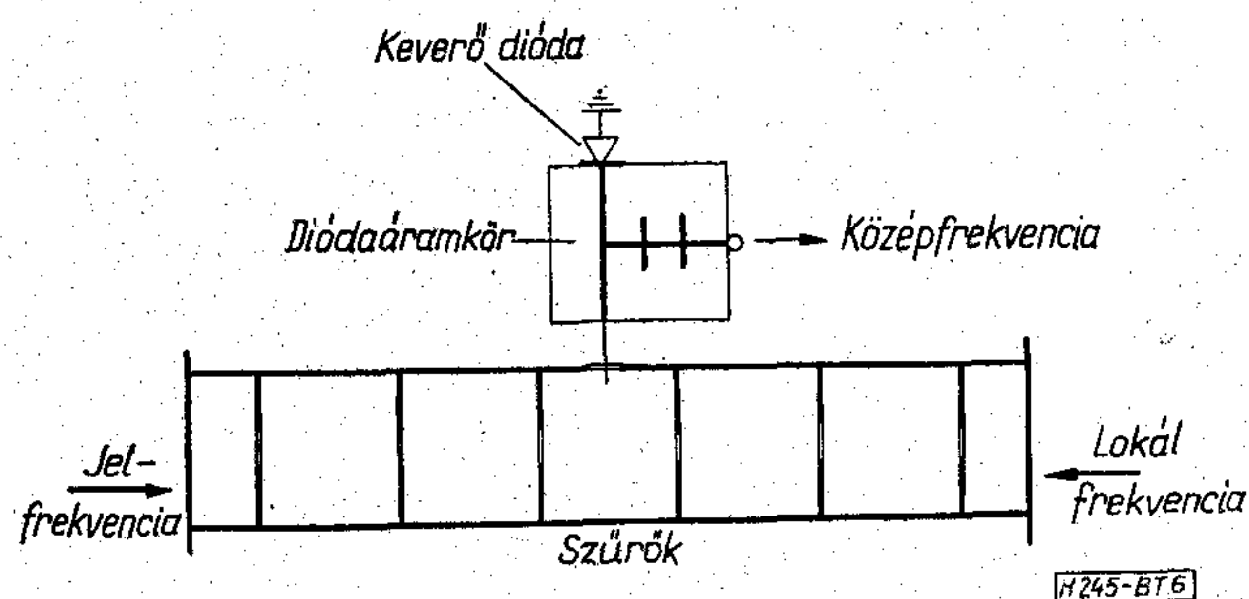
6. ábra. Vevőkeverő vázlatos rajza
