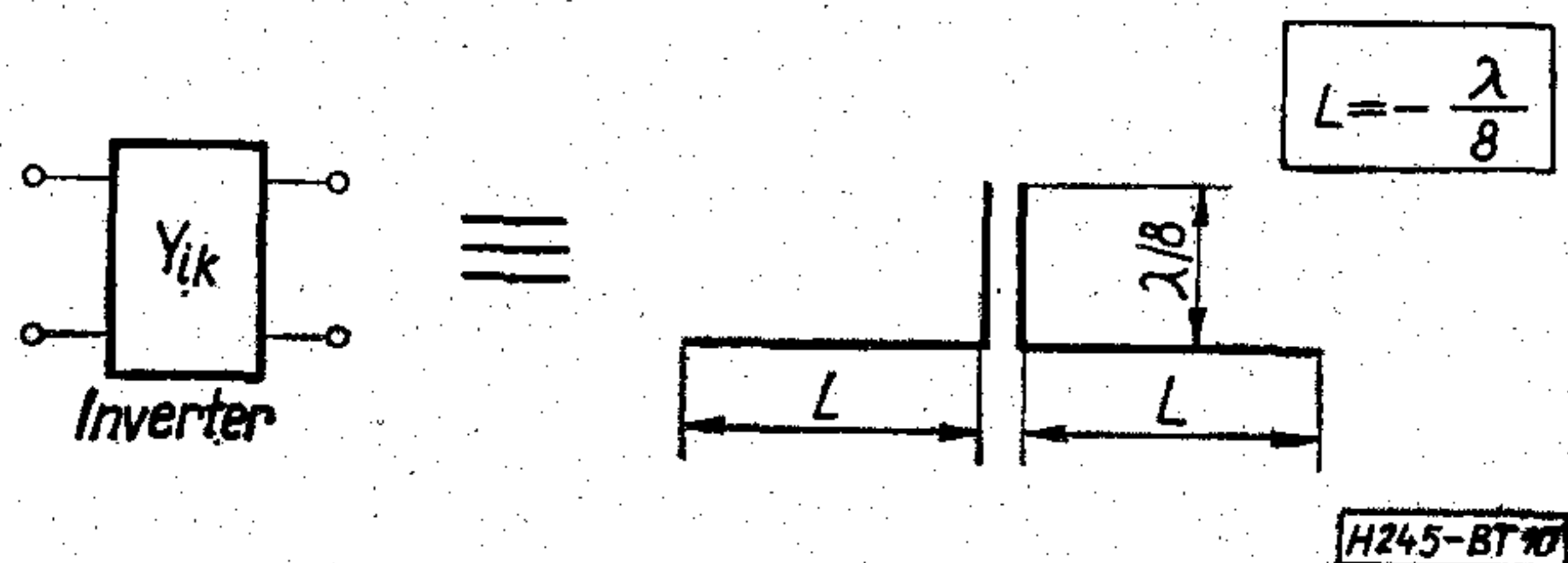
10. ábra. Inverter megvalósítása
