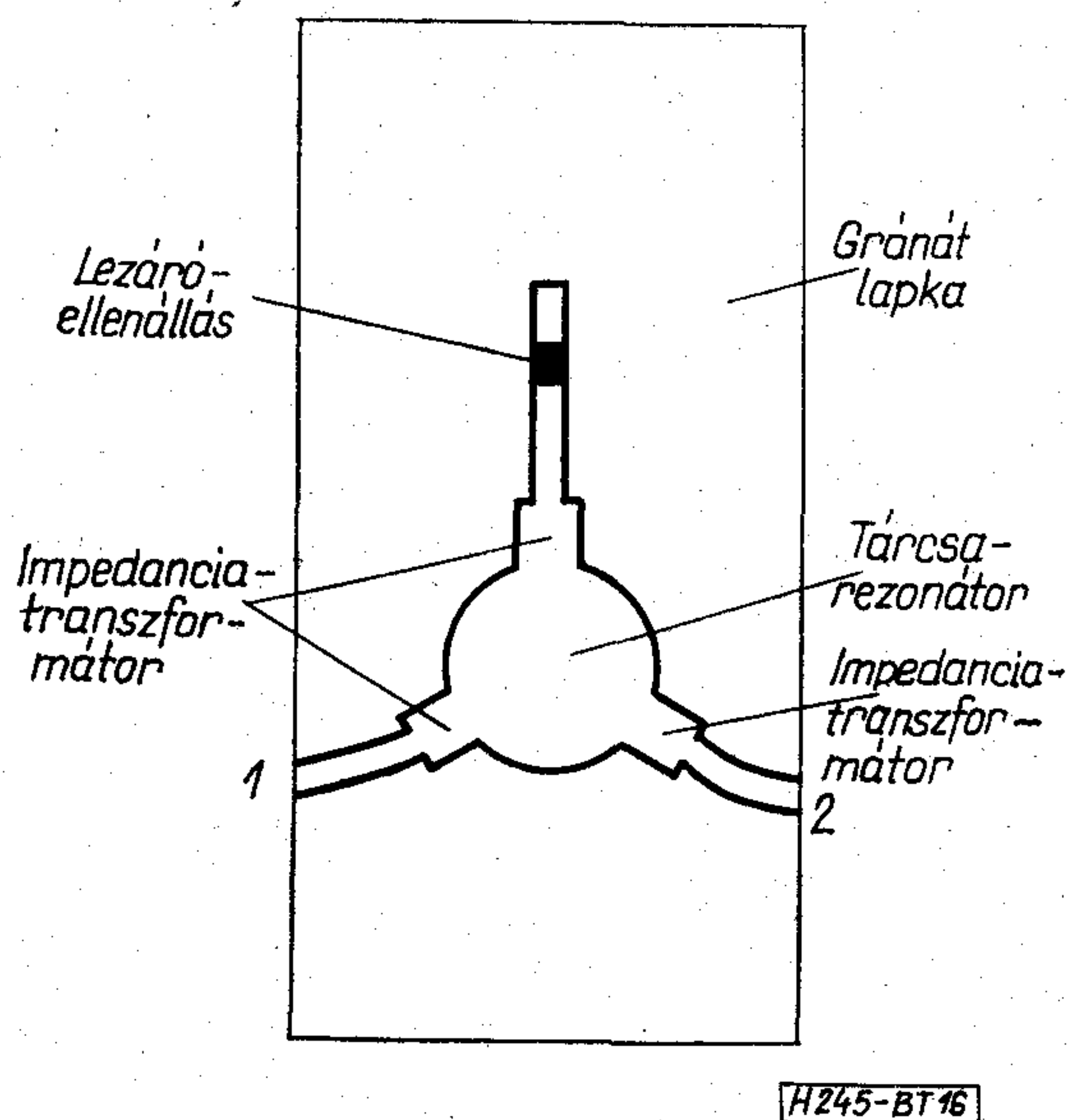
16. ábra. Szélessávú izolátor áramköri elrendezése
