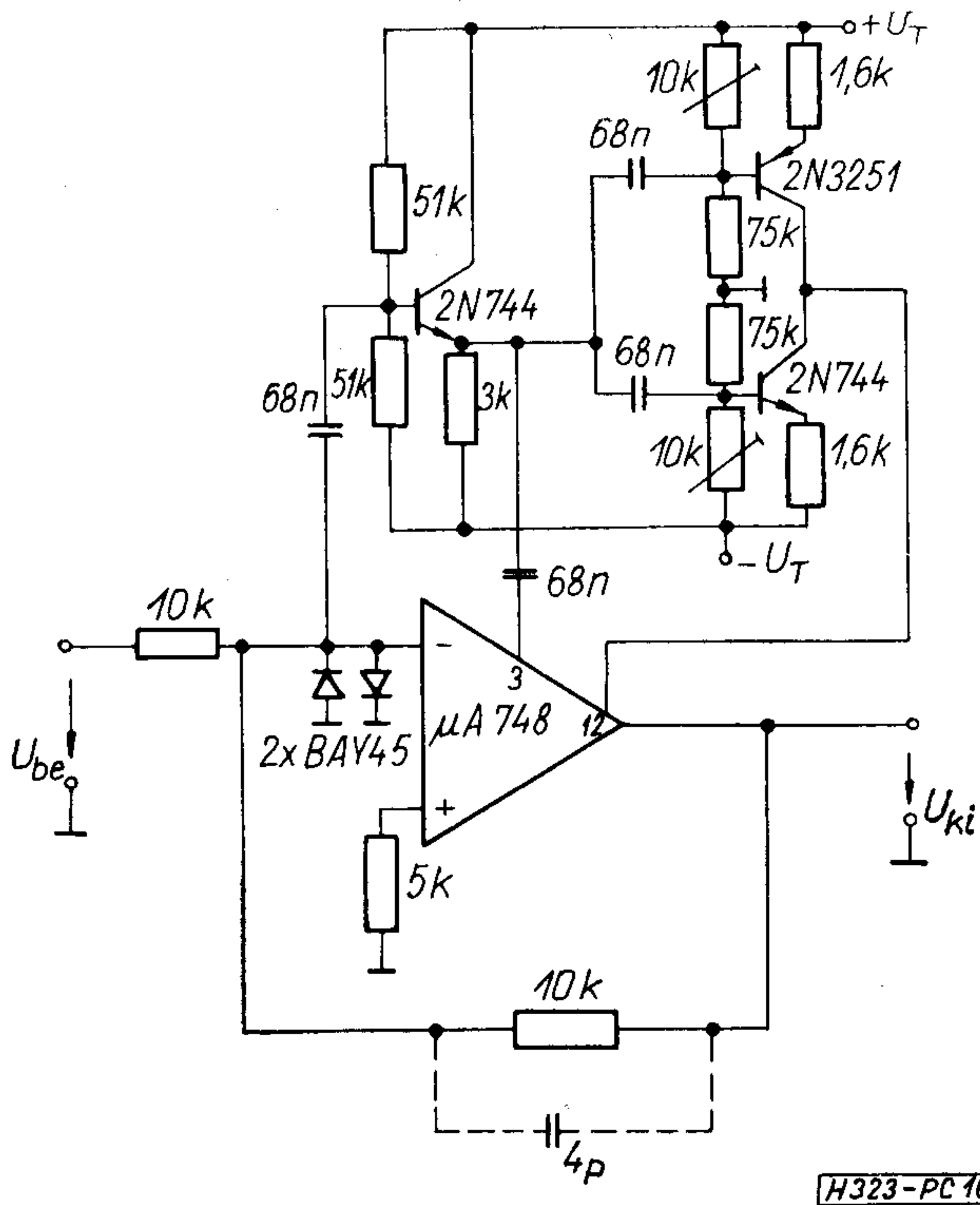
16a ábra. Kettős előrecsatolásos kompenzálás elválasztó erősítővel (feszültség- és áramösszegezés elvén)
