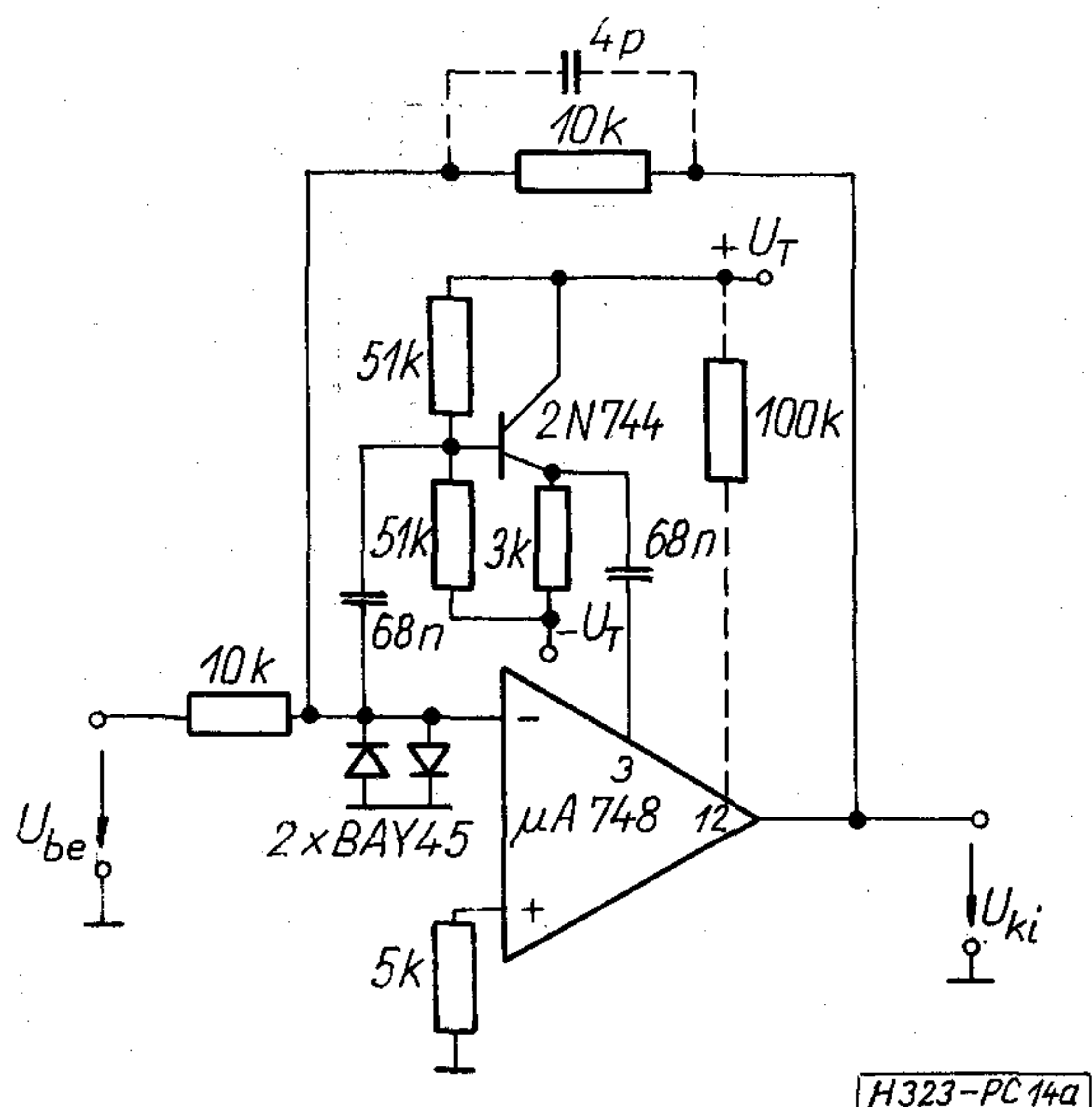
14a ábra. Előreccsatolós kompenzáls elválasztó erősítővel
