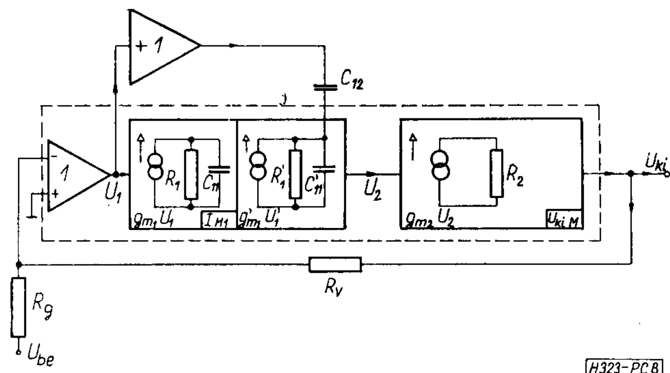
8. ábra. Előreccsatolás a rendszer kimenetére
