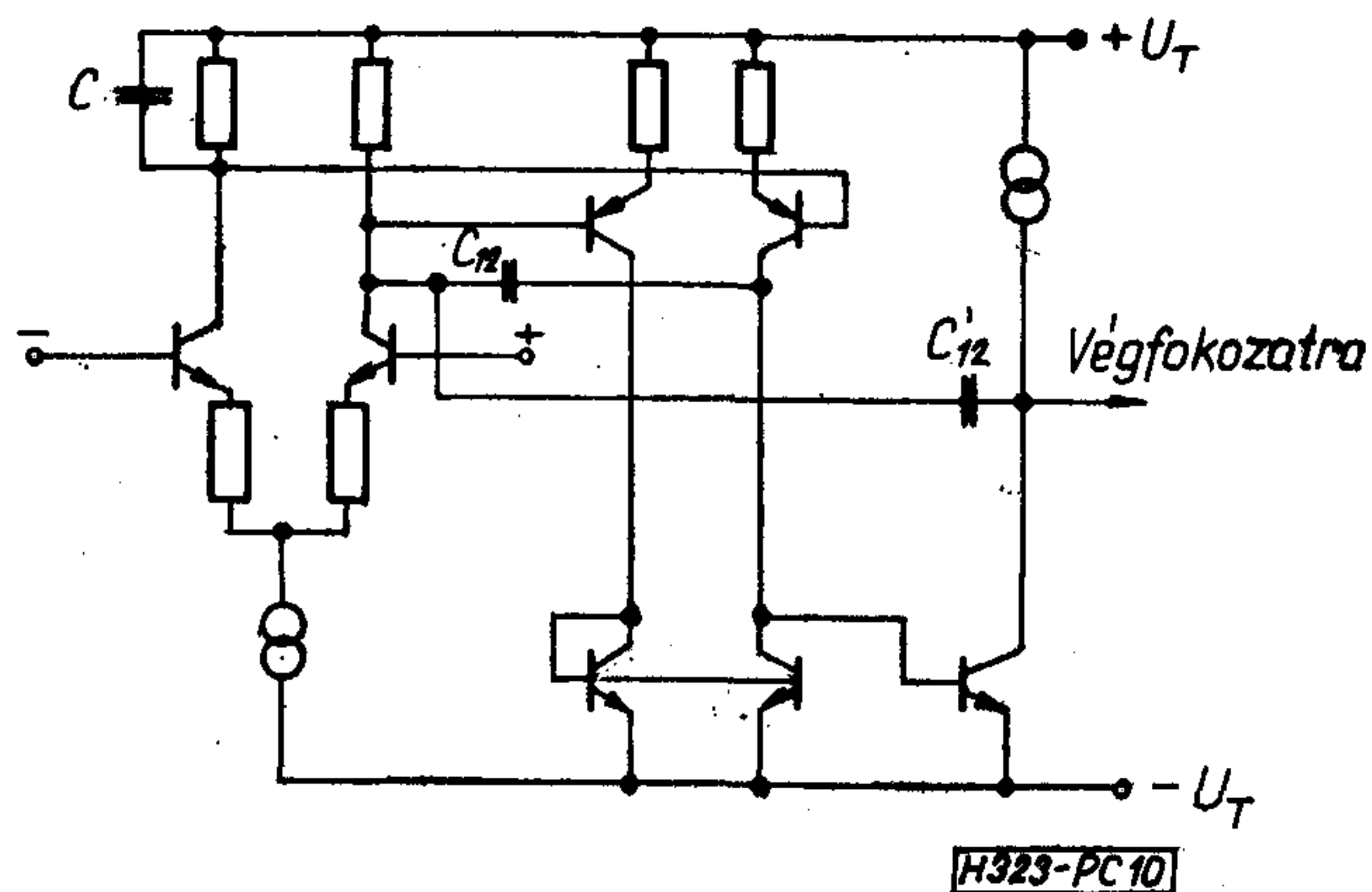
10. ábra. Előrecsatolásos kompenzálás integrált áramkörön belül (LM 318)
