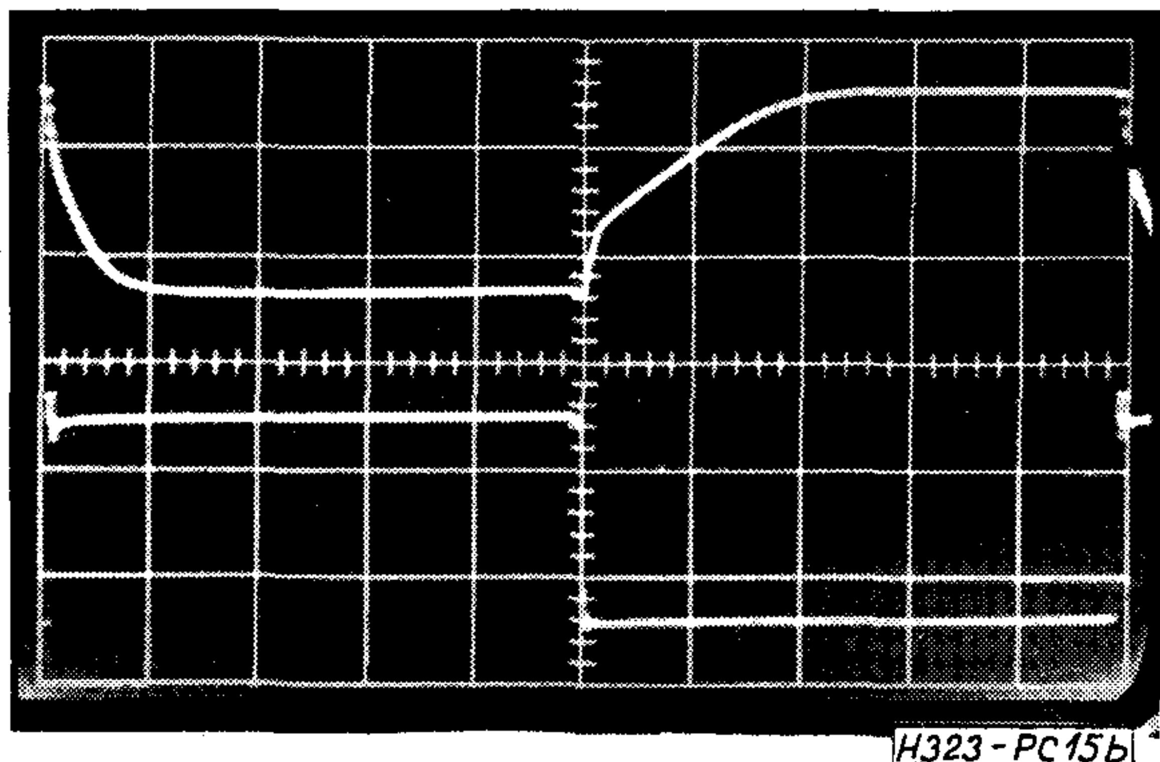
15b ábra. Függőleges eltérítés: 5 V/cm, vízszintes eltérítés: 0,5 \mu s/cm
