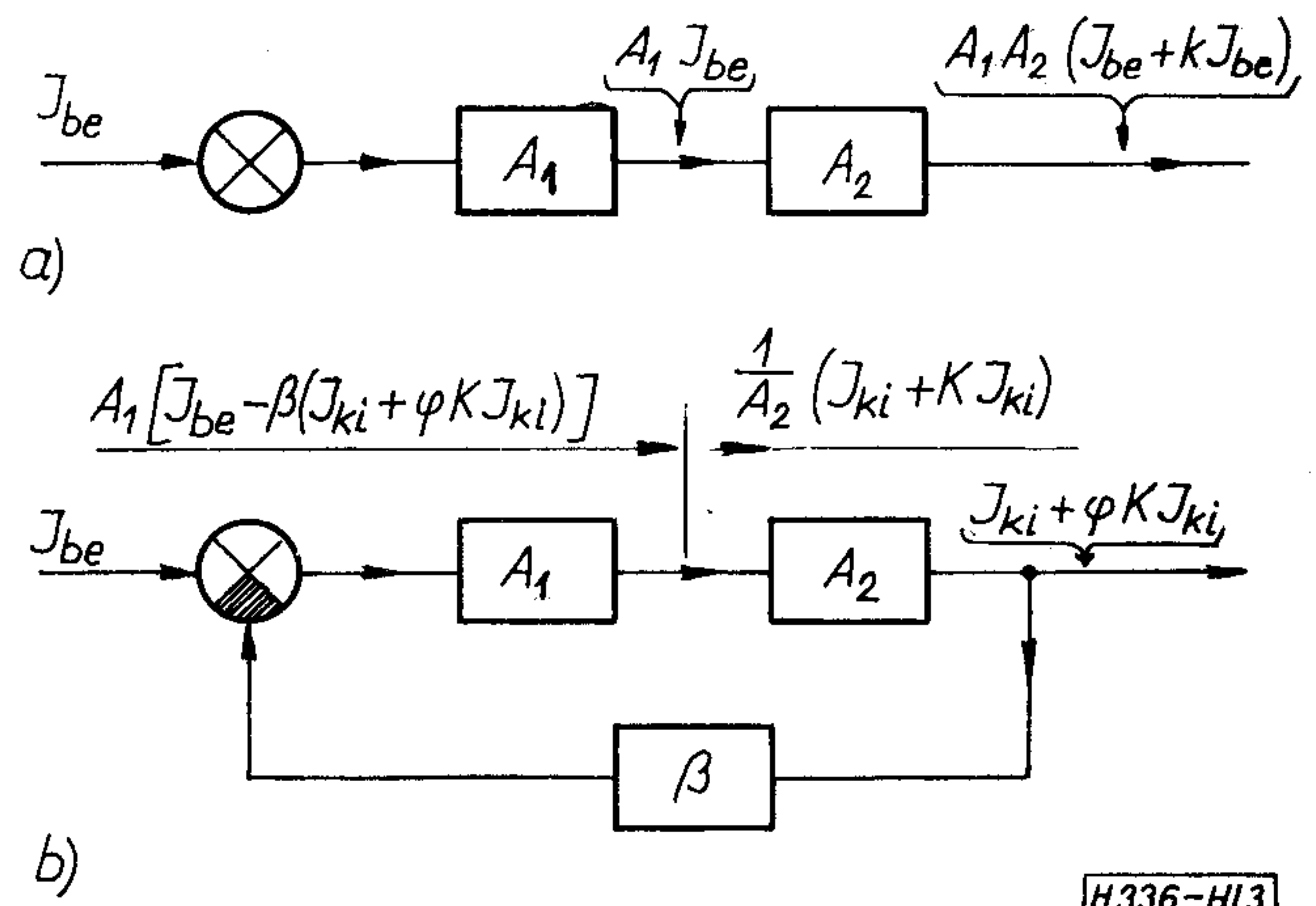
3. ábra. Visszacsatolatlan (a) és negatív visszacsatolt (b) rendszer jelátvitel
