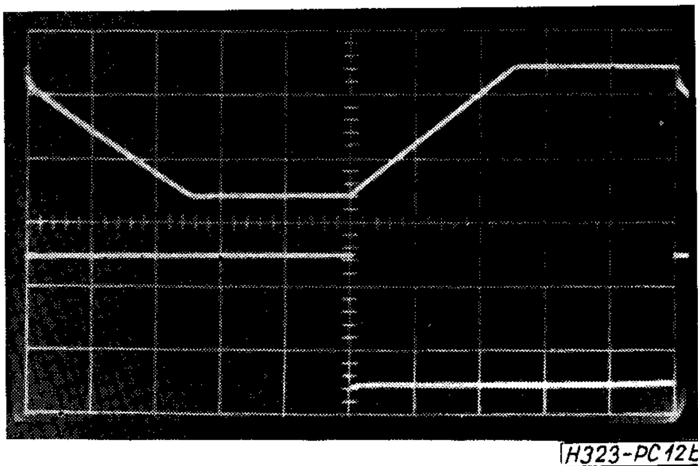
12b ábra. Függőleges eltérítés: 5V/cm, vízszintes eltérítés: 10 μs/cm
