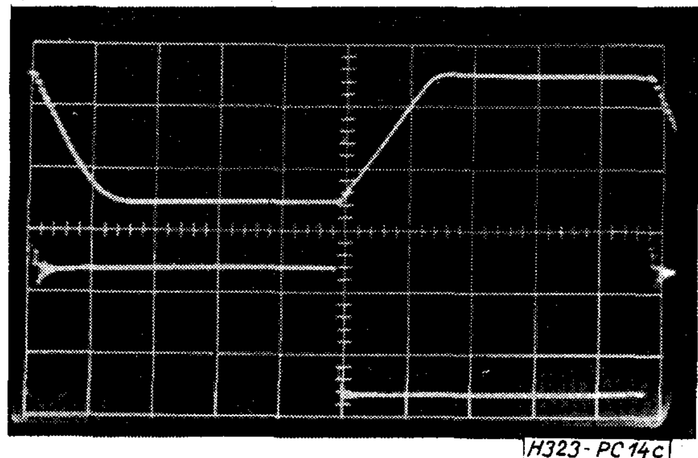
14c ábra. Függőleges eltérítés: 5 V/cm, vízszintes eltérítés: 0,2 \mu s/cm
