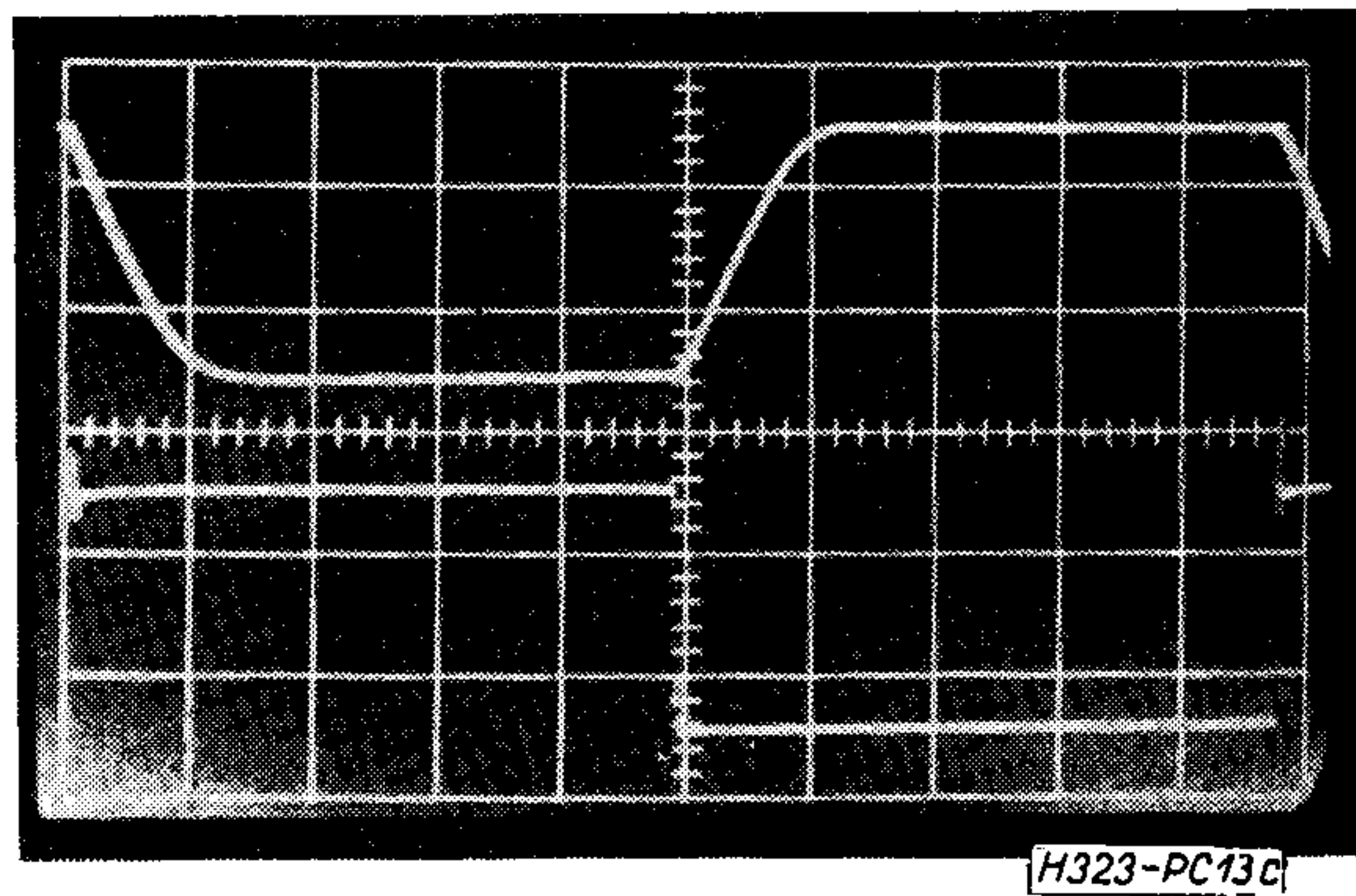
13c ábra. Függőleges eltérítés: 5 V/cm, vízszintes eltérítés: 0,5 μs/cm
