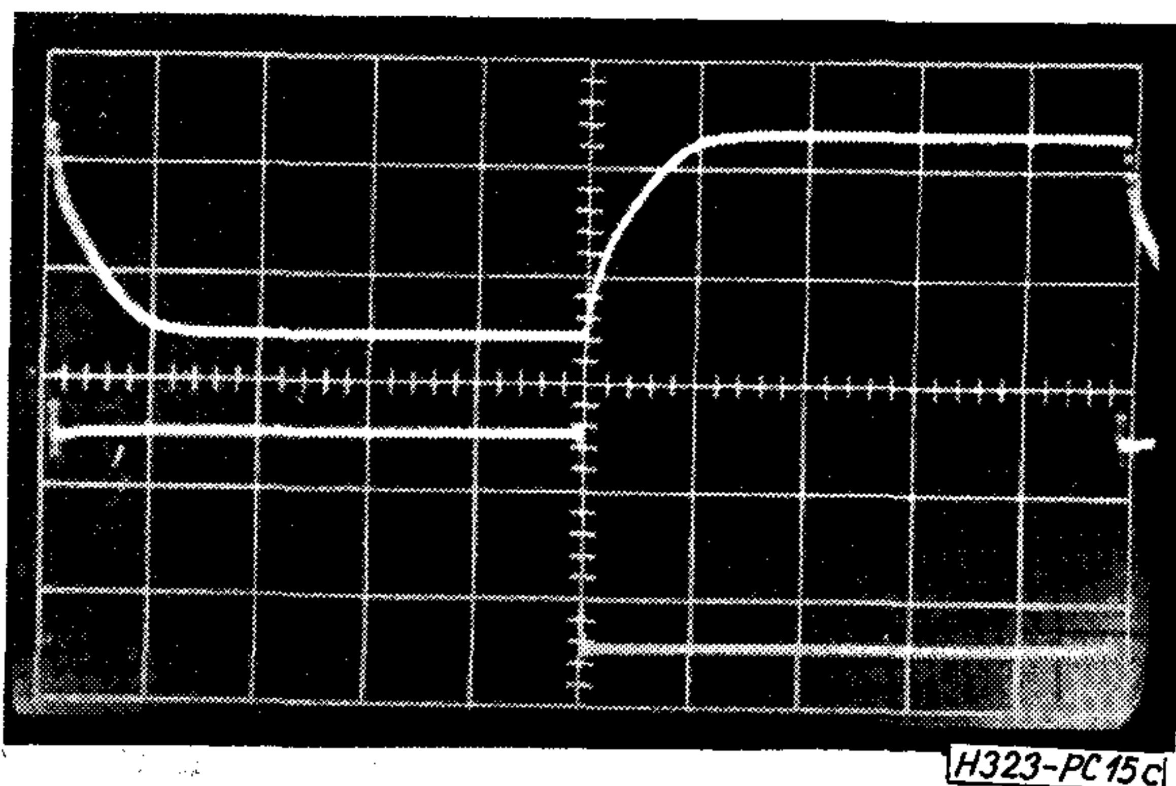
15c ábra. Függőleges eltérítés: 5 V/cm, vízszintes eltérítés: 0,5 \mu s/cm
