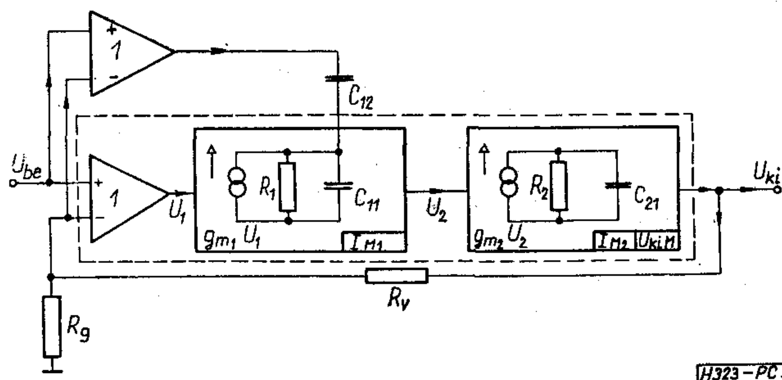
9. ábra. Pozitív erősítésű erősítő előrecsatolásos kompenzálásának elvi vázlata
