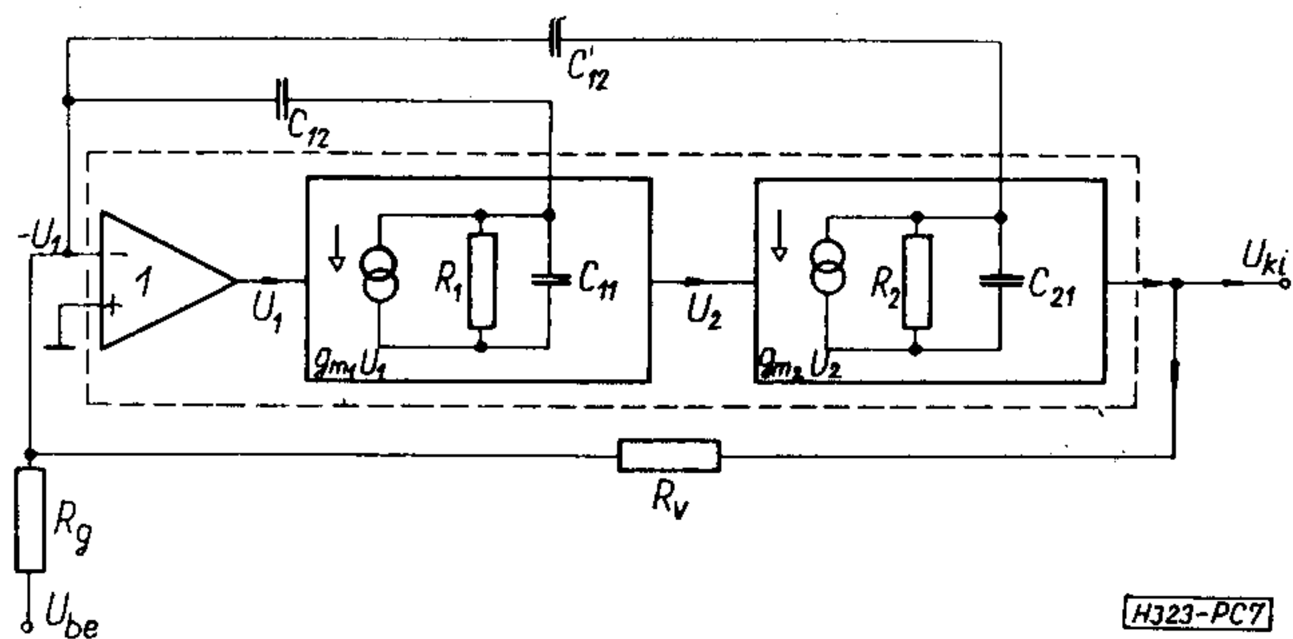
7. ábra. Előreccsatolás kompenzálás elválasztó erősítő nélkül
