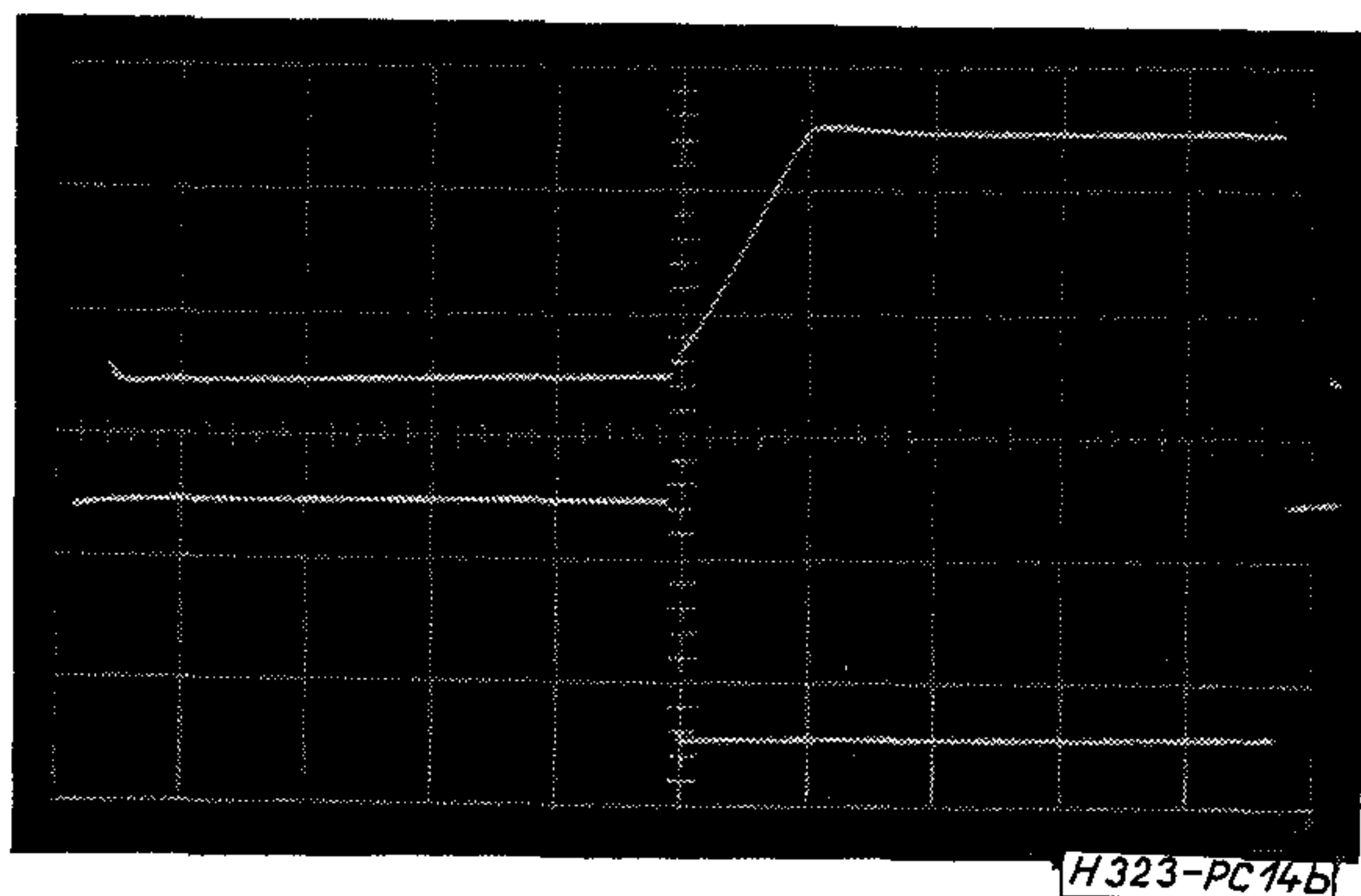
14b ábra. Függőleges eltérítés: 5 V/cm, vízszintes eltérítés: 0,5 \mu s/cm
