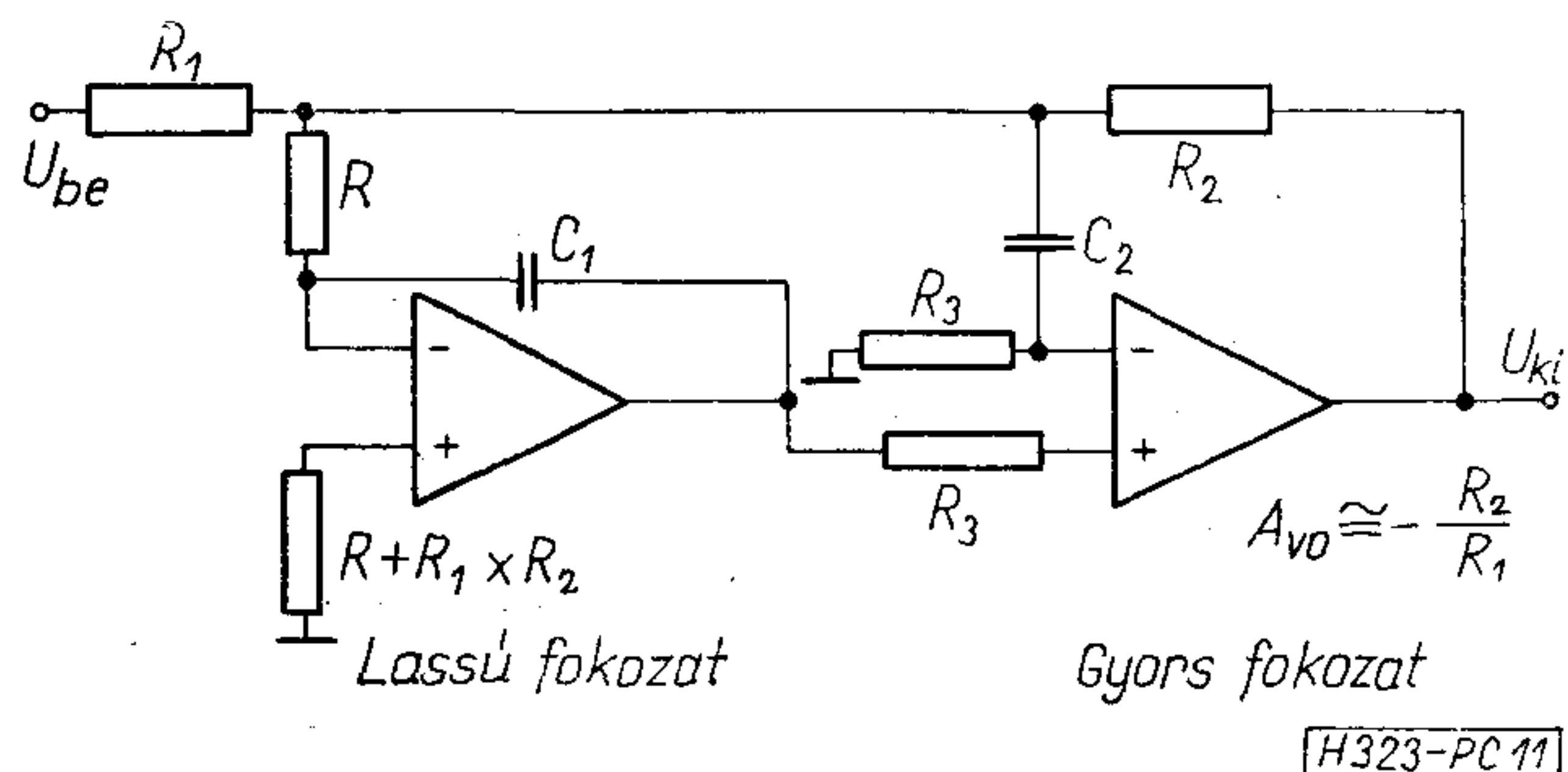
11. ábra. Több műveleti erősítőt felhasználó előrecsatolásos kompenzálás (példa a gyors és pontos fázisfordító fokozatra)
