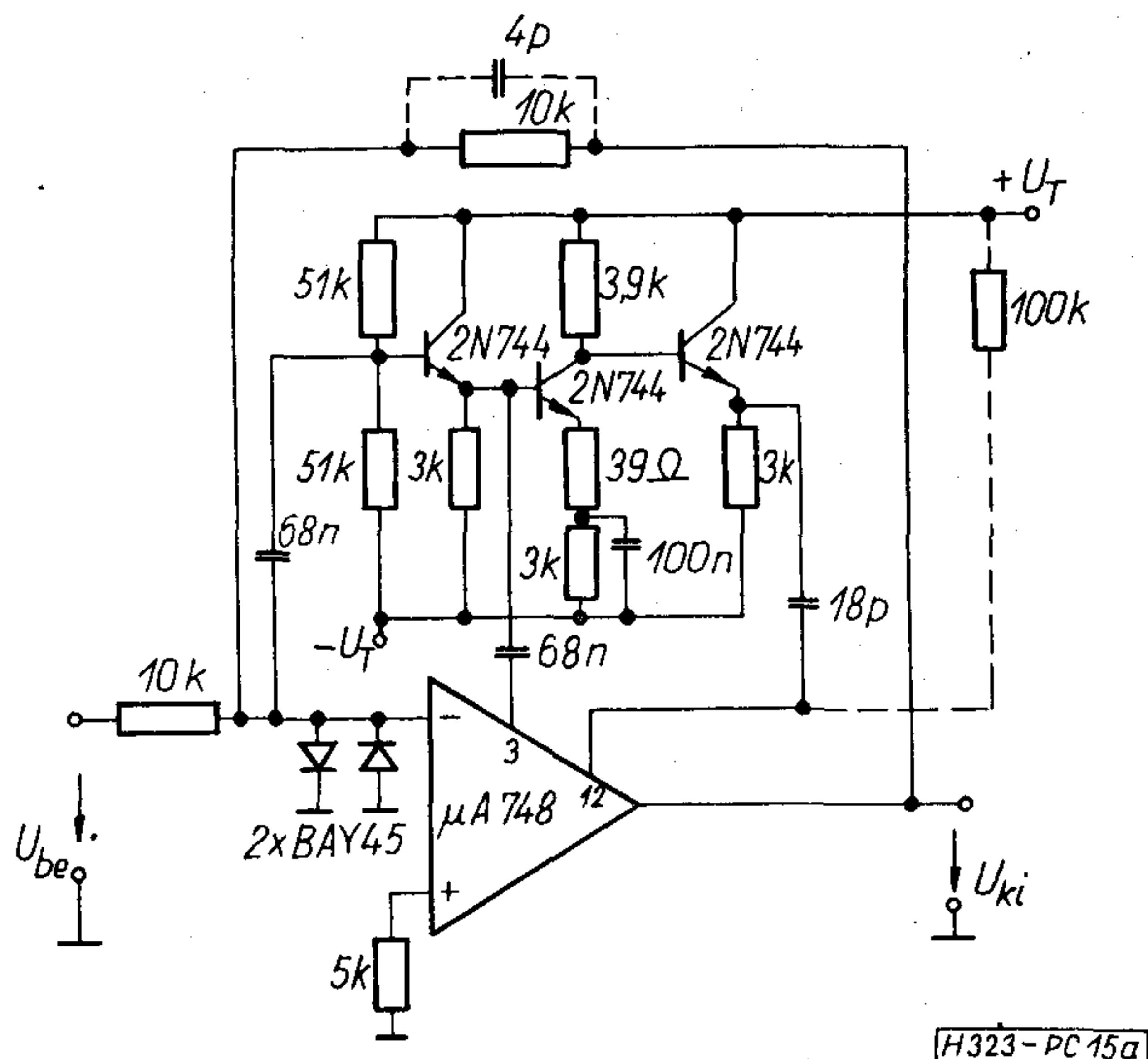
15a ábra. Kettős előreccsatolás elválasztó erősítővel (feszültségösszezés elvén)
