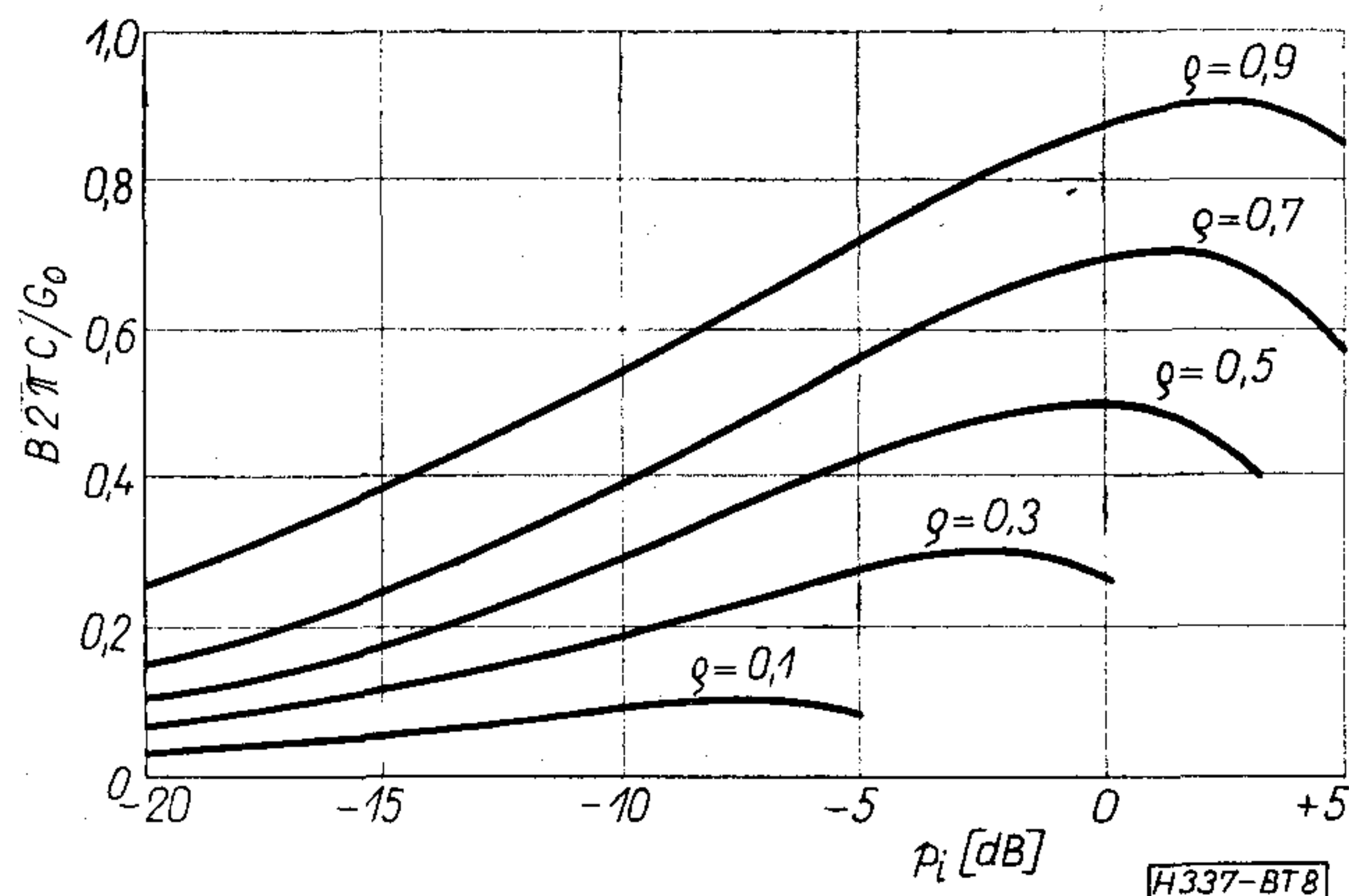
8. ábra. A vezérlési sávval arányos B2\pi C/G_0 mennyiség a bemenő teljesítmény függvényében, a görbék paramétere a terhelési tényező
