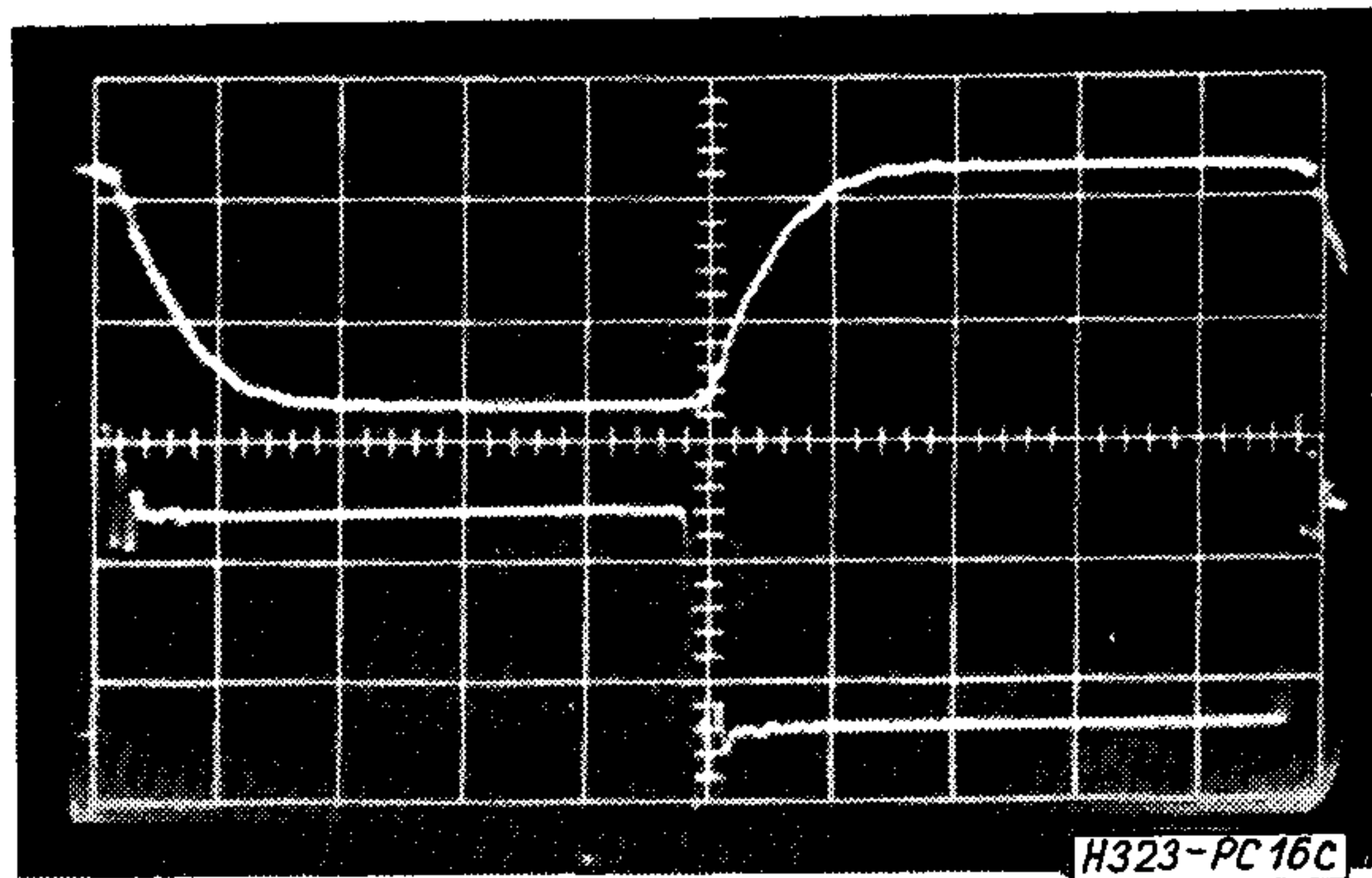
16c ábra. Függőleges eltérés 0,5 V/cm, vízszintes eltérés: 0,1 μs/cm
