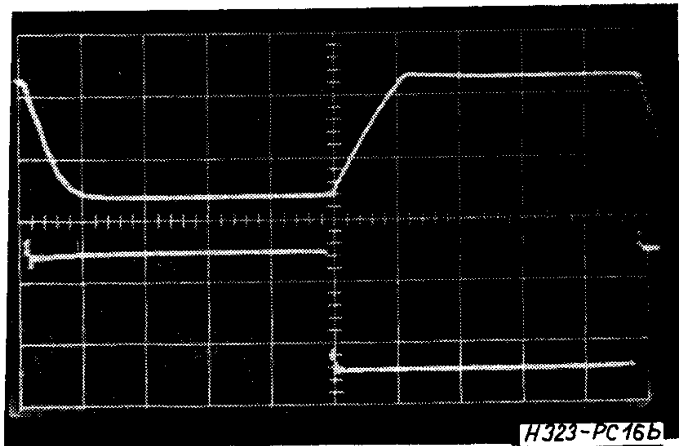
16b ábra. Függőleges eltérés: 5 V/cm, vízszintes eltérés: 0,2 μs/cm
