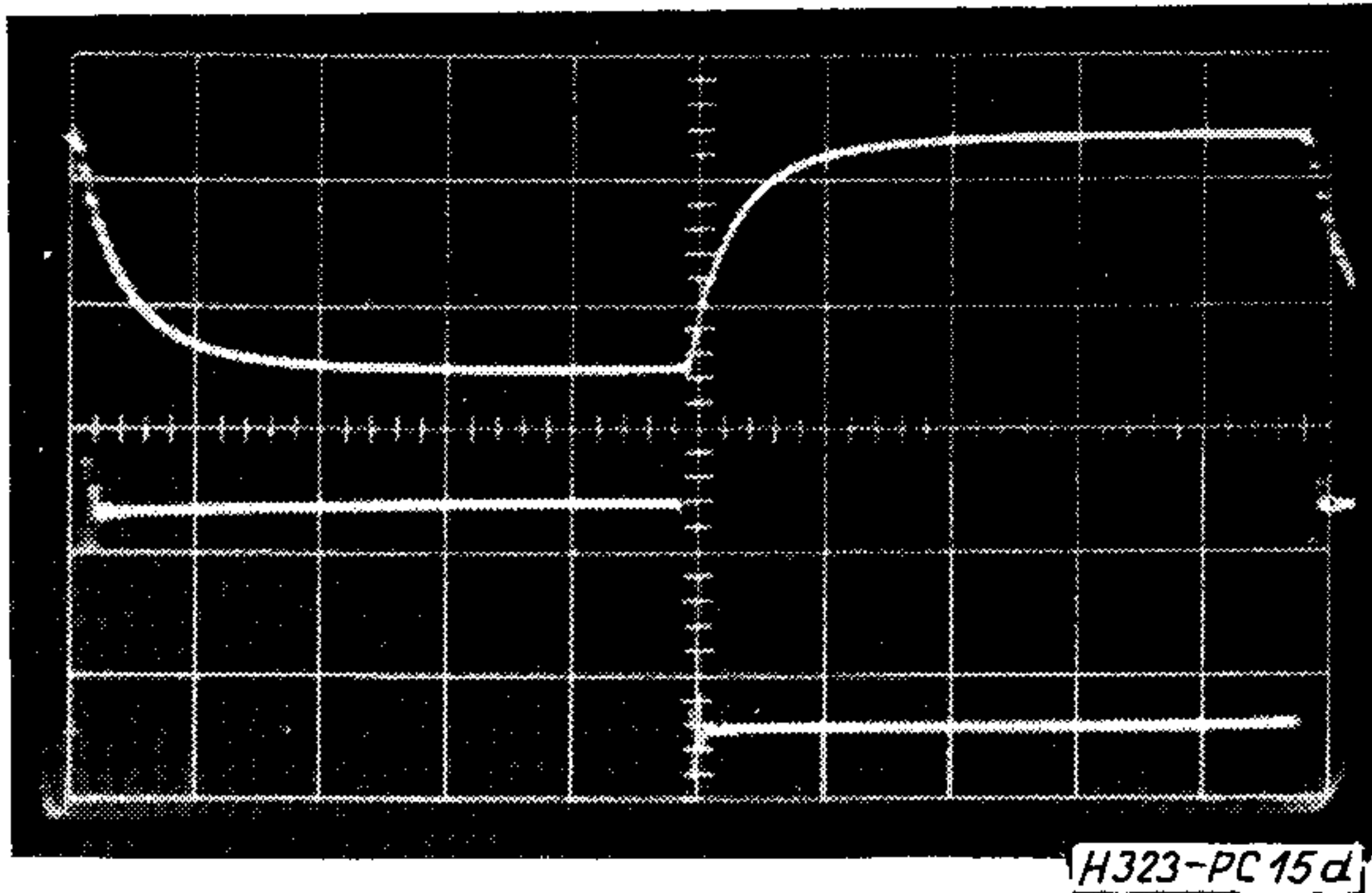
15d ábra. Függőleges eltérés: 0,5 V/cm, vízszintes eltérés: 0,2 μs/cm
