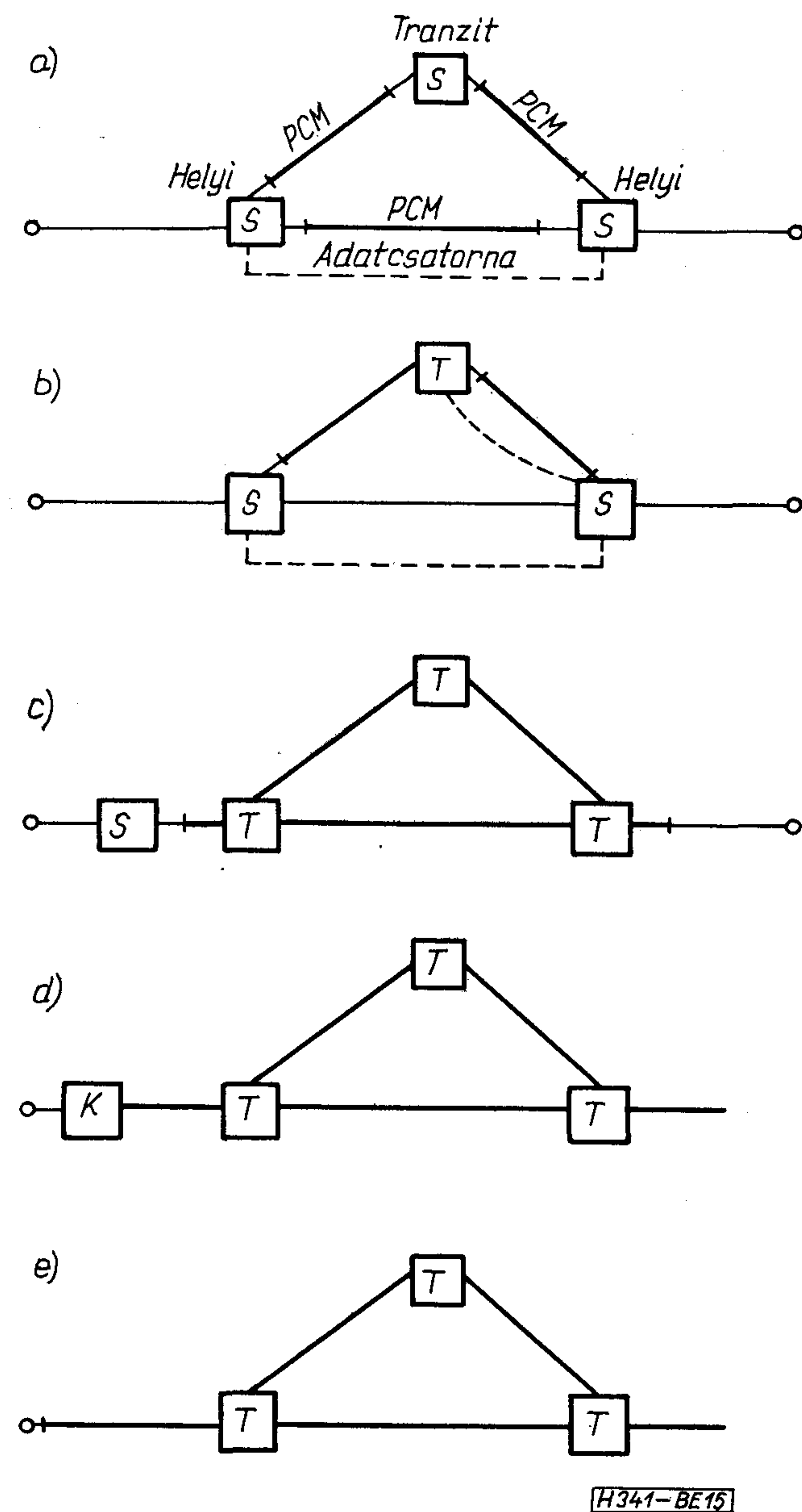
15. ábra. A PCM kapcsolástechnika fokozatos bevezetése
