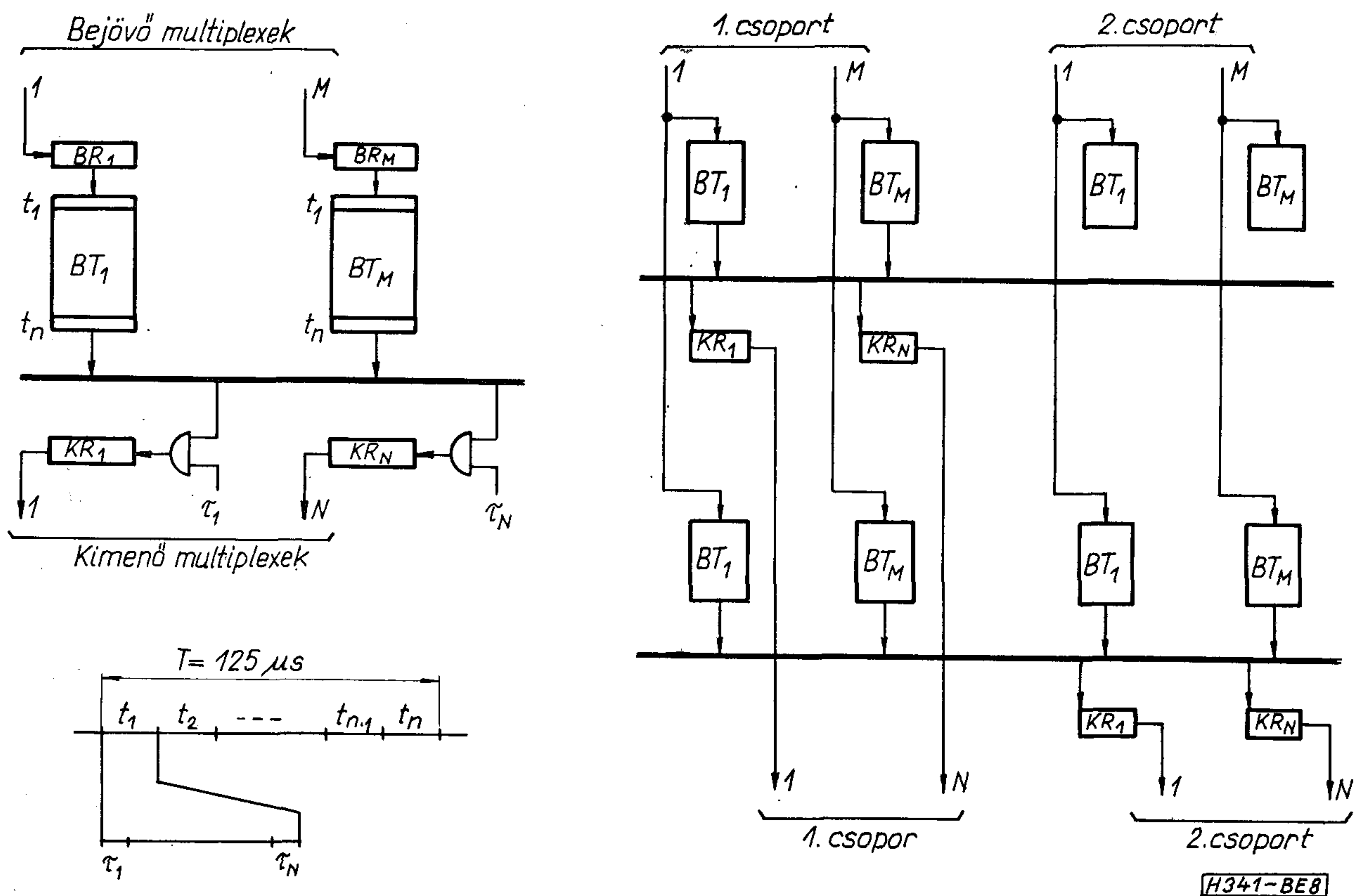
8. ábra. Egyirányú ideális PCM kapcsoló, beszédjeltárral
