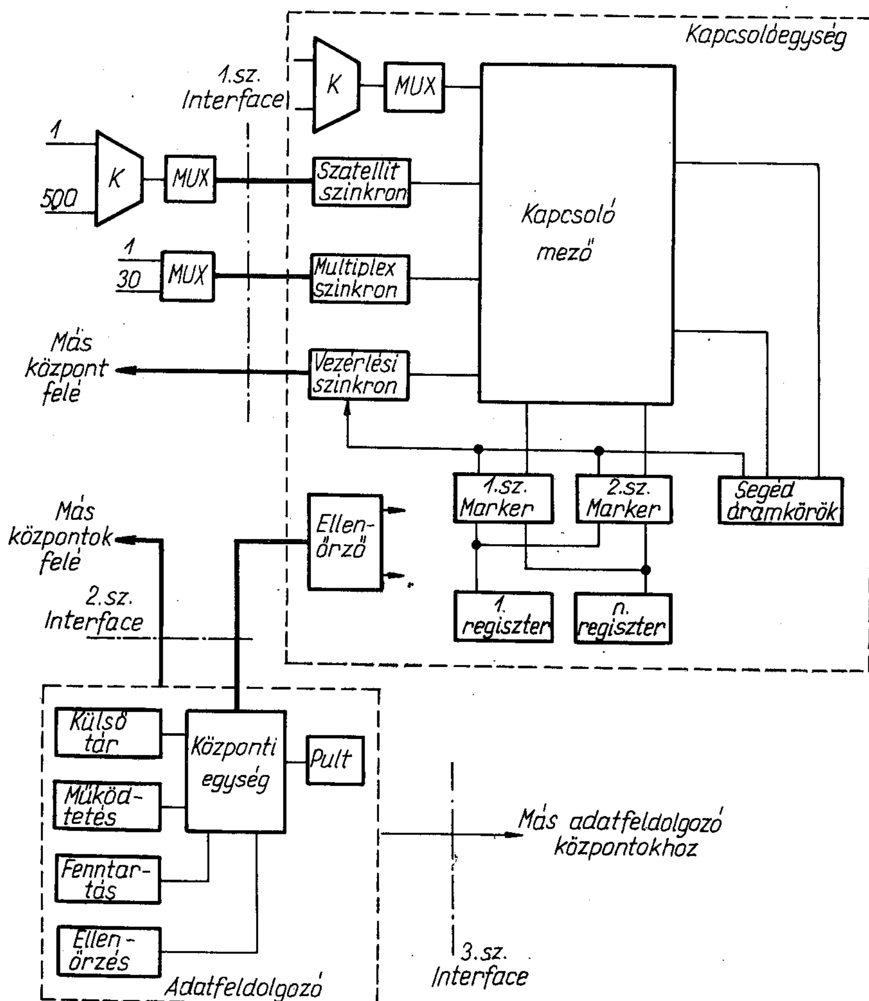
13. ábra. Az E10 rendszer blokkvázlata
