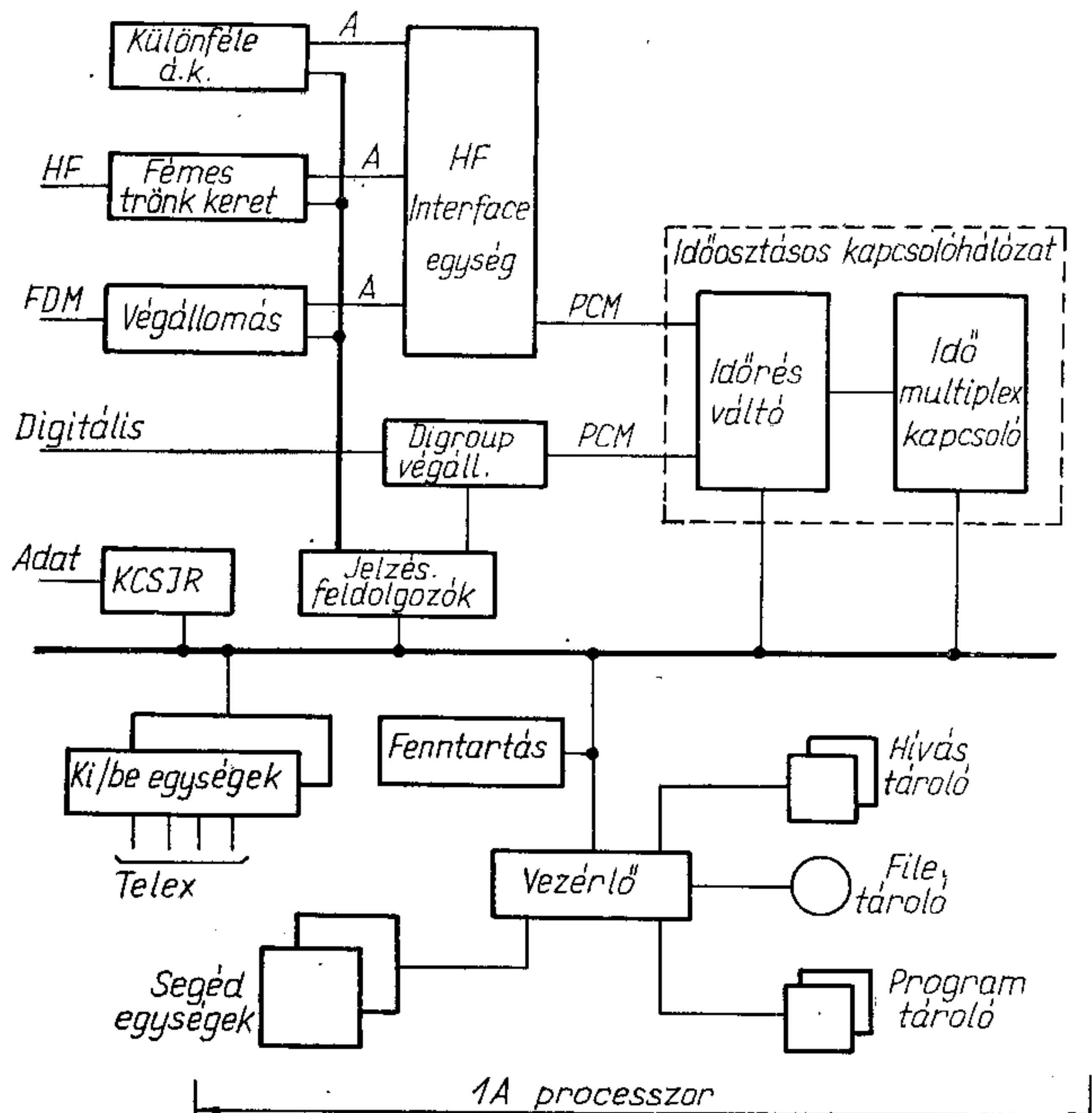
14. ábra. A No. 4., ESS elektronikus kapcsolórendszer felépítése
