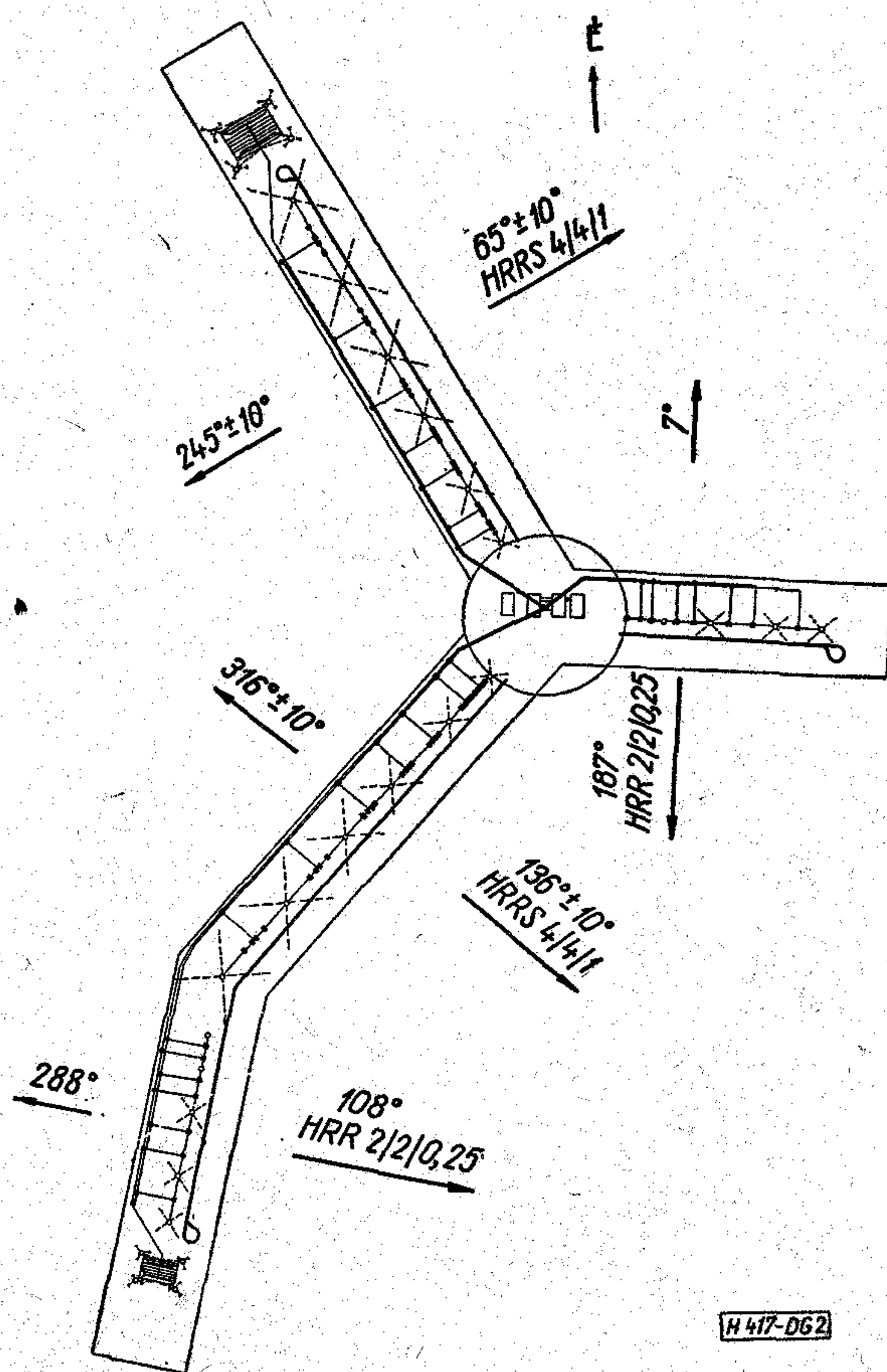
2. ábra. Jászberényi rövidhullámú adóállomás rendszertechnikai terve
