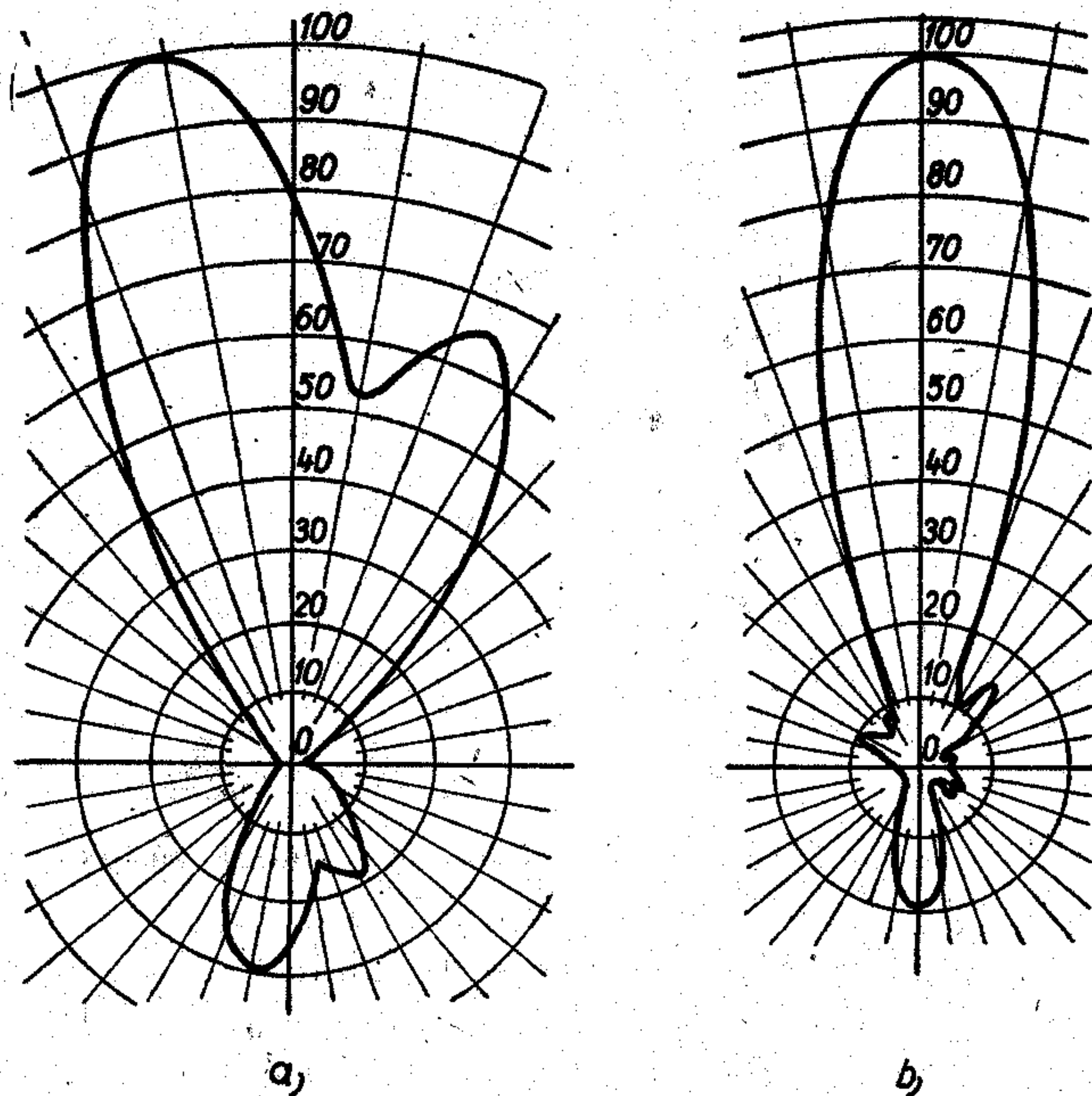
6. ábra. a) HRRS 4/4/1 típusú antennarendszer vízszintes iránykarakteristikája modellmérések alapján b) HRRS 4/4/1 típusú antennarendszer vízszintes iránykarakteristikája balra billentett esetben, modellmérések alapján
