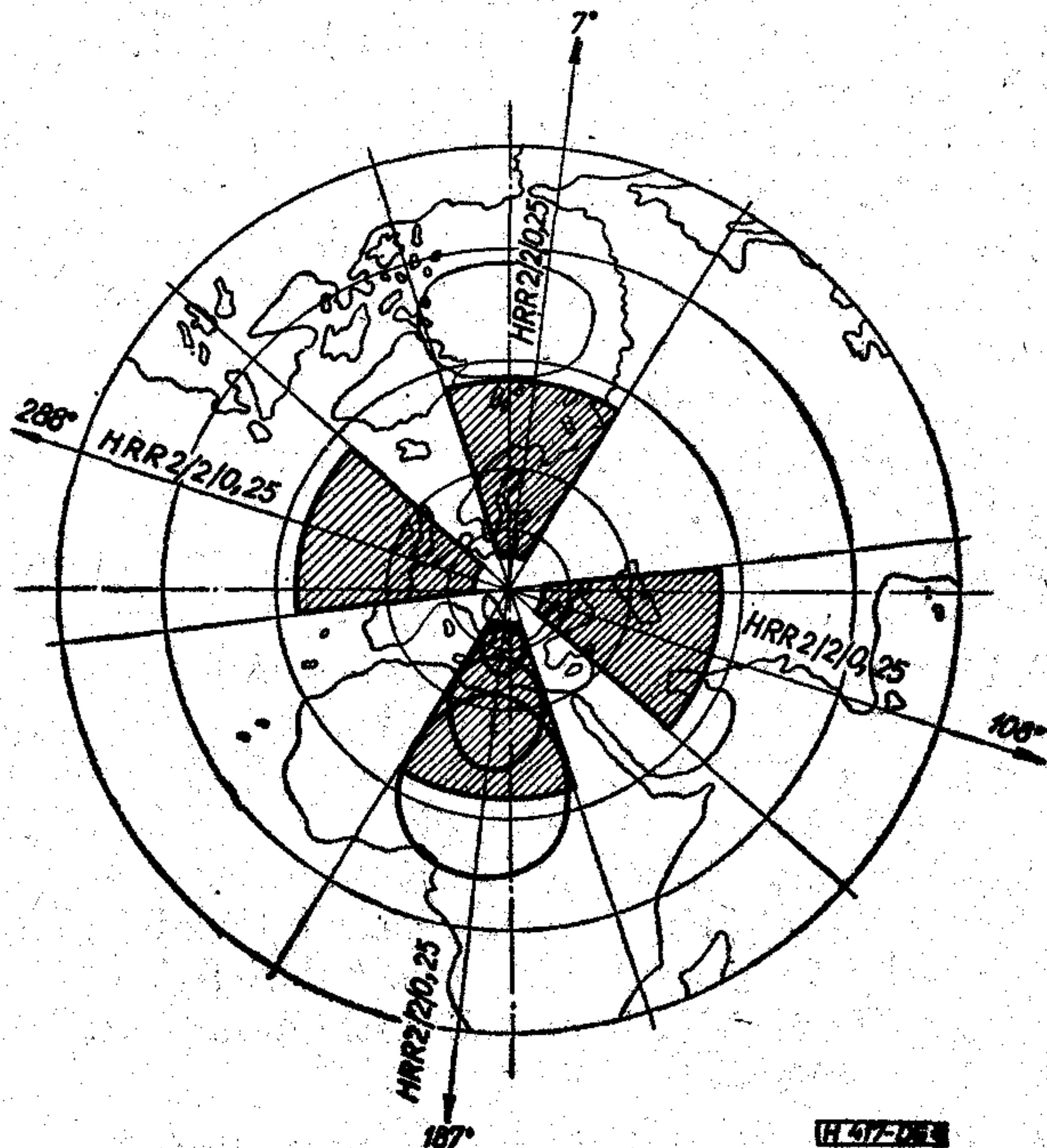
4. ábra. HRR 2/2/0,5 antennarendszer hatáskörzete
