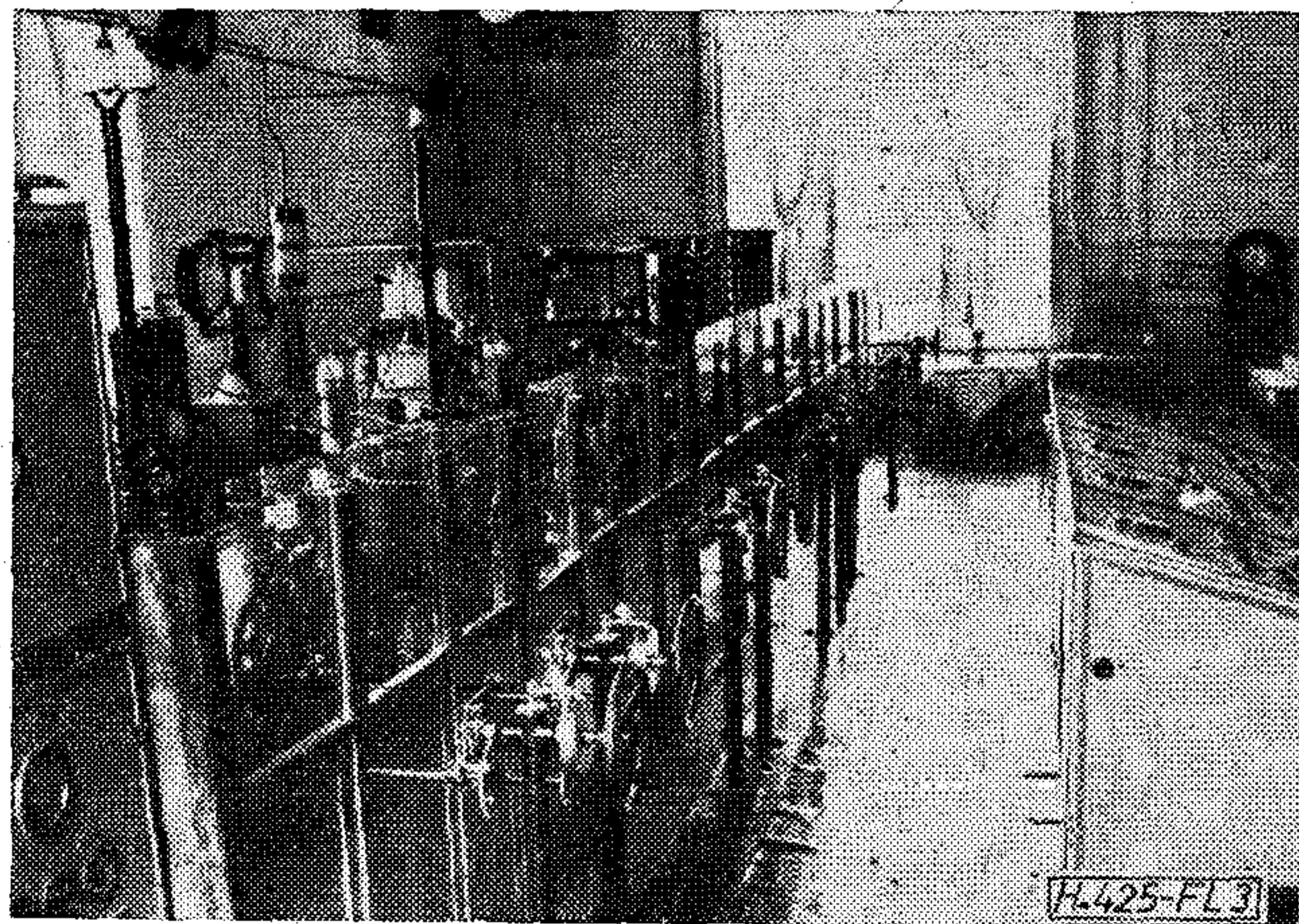
3. ábra. A lakihegyi 20/50 kW-os középhullámú adóberendezés
