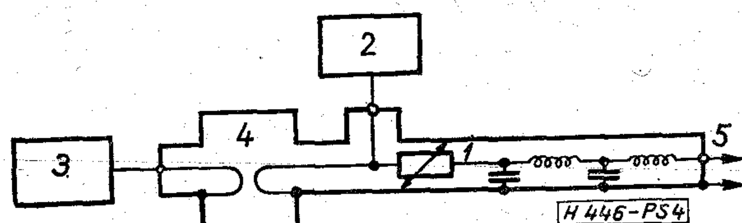
4. ábra. Egytermisztoros, bolométeres feszültségmérő kapcsolási vázlata. 1. termisztor, 2. vizsgálandó feszültségmérő, 3. generátor, 4. csatoló hurok, 5. ellenállásmérő hídhoz
