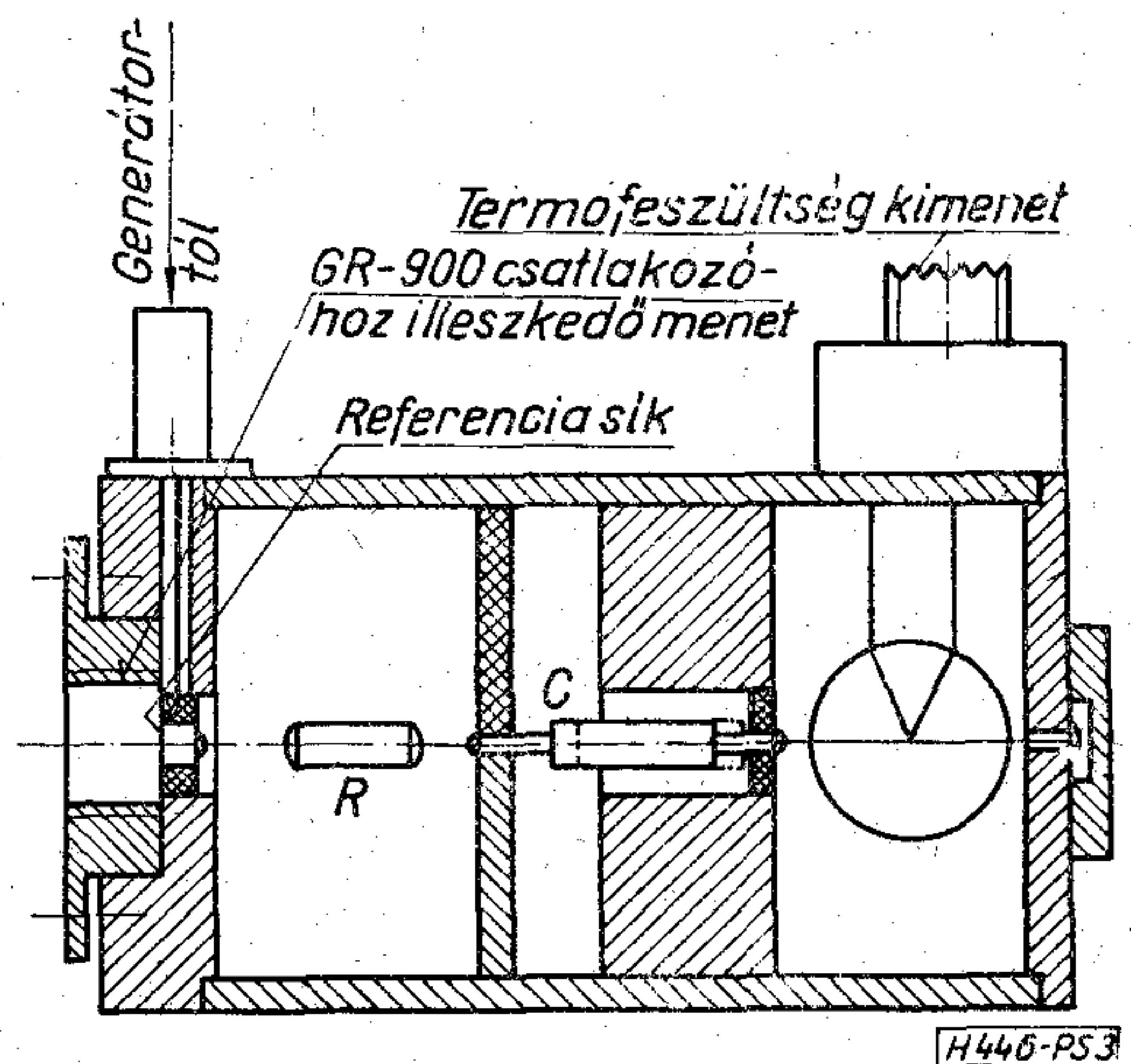
3. ábra. Nagyfrekvenciás egyen-váltakozó átvivő
