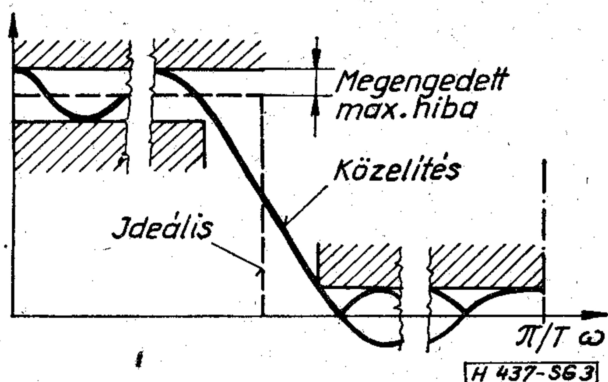
3. ábra. Frekvenciatartománybeli követelmény és egyenletes közelítése
