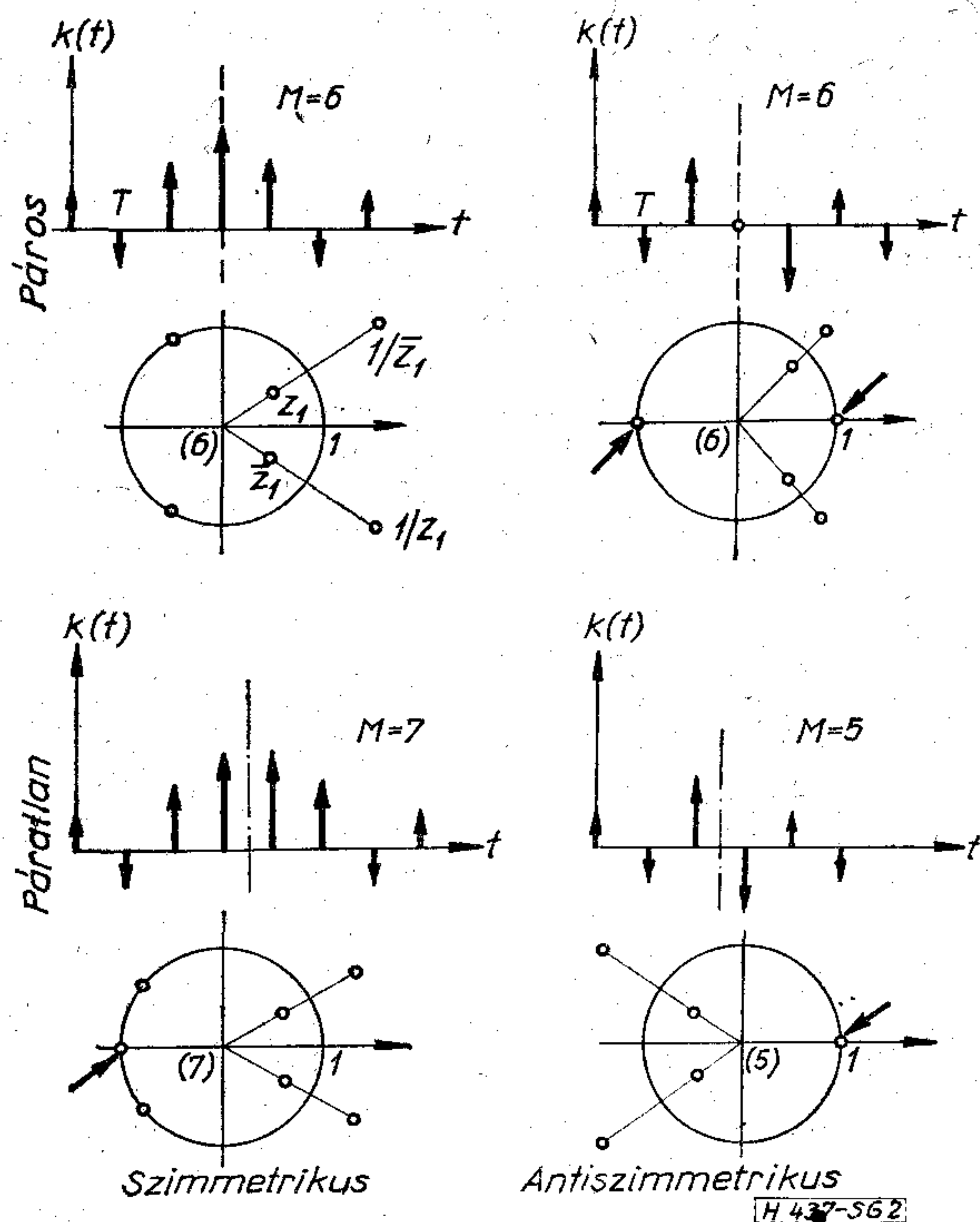
2. ábra. Lineárisfázisú FIR szűrők négy esete. Súlyfüggvény és zérus-pólus elrendezés a struktúrából adódó zérusok megjelölésével
