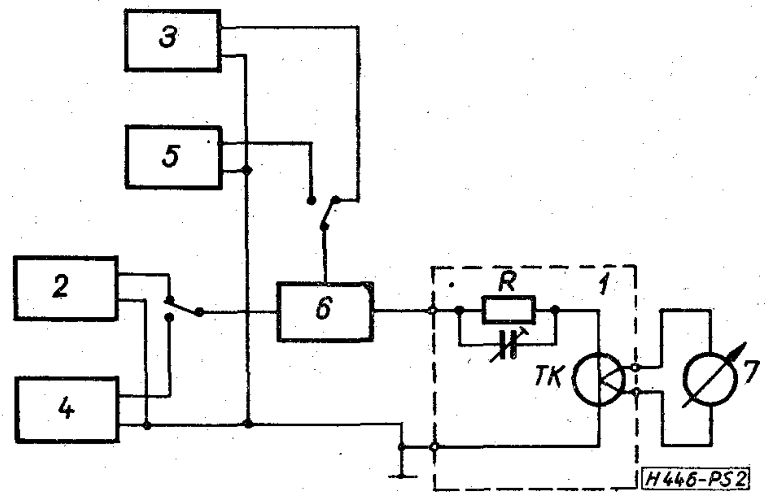
2. ábra. Váltakozó feszültségű voltmérő vizsgálata termokeresztes átvivővel. 1. termokeresztes átvivő, 2. vizsgálandó voltmérő, 3. váltakozó feszültségű generátor, 4. egyenfeszültségű voltmérő, 5. egyenfeszültség-forrás, 6. I-elágazás, 7. galvanométer
