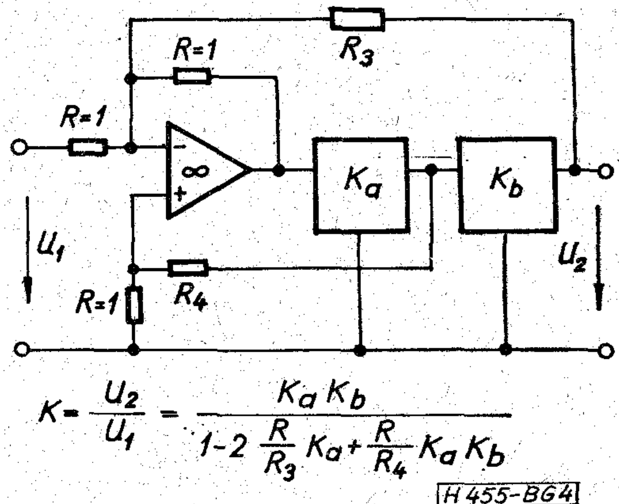
4. ábra. PRB kapcsolás. Az áramköri elemek értéke:
