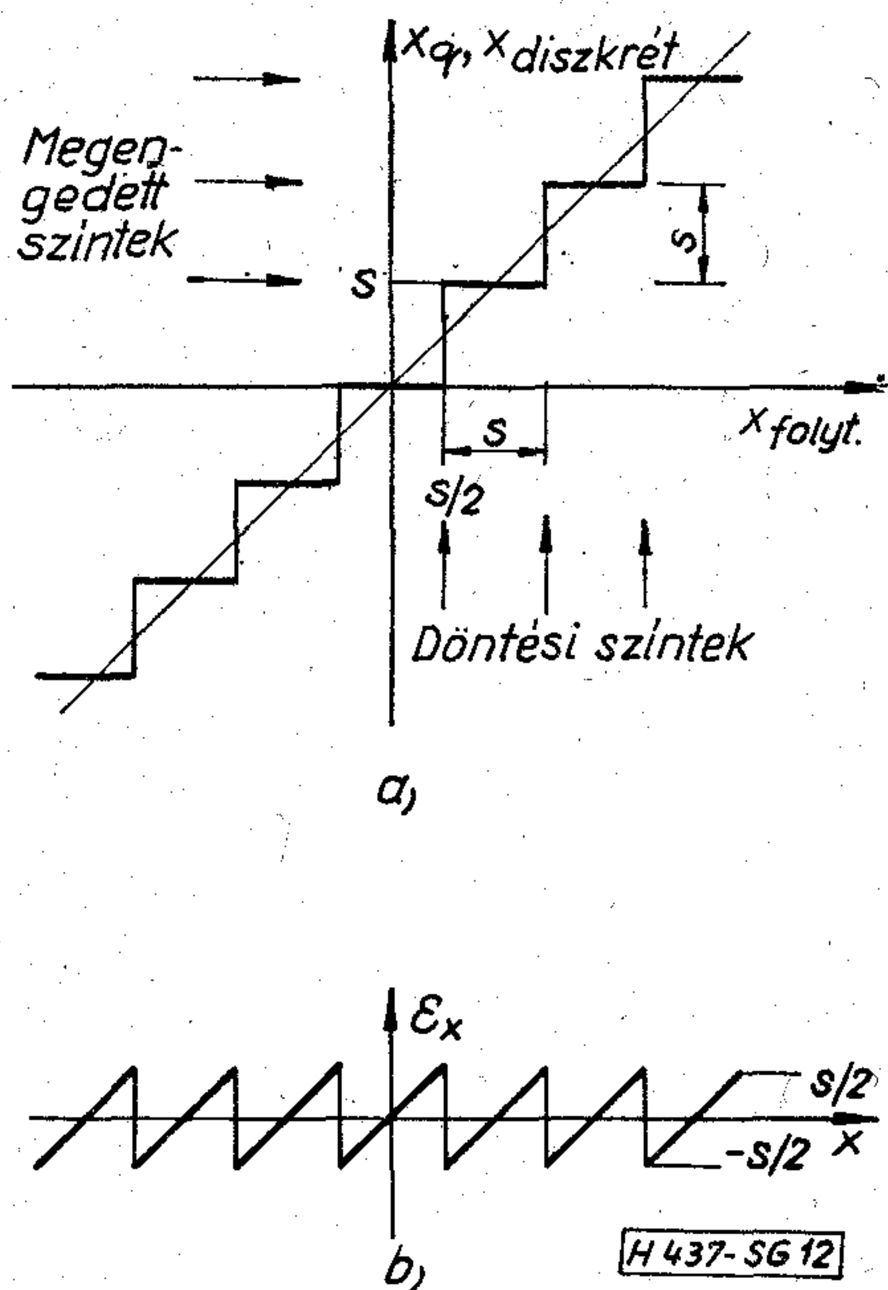
12. ábra. Kvantálási karakterisztika (a) és a kerekítés hibája (b)
