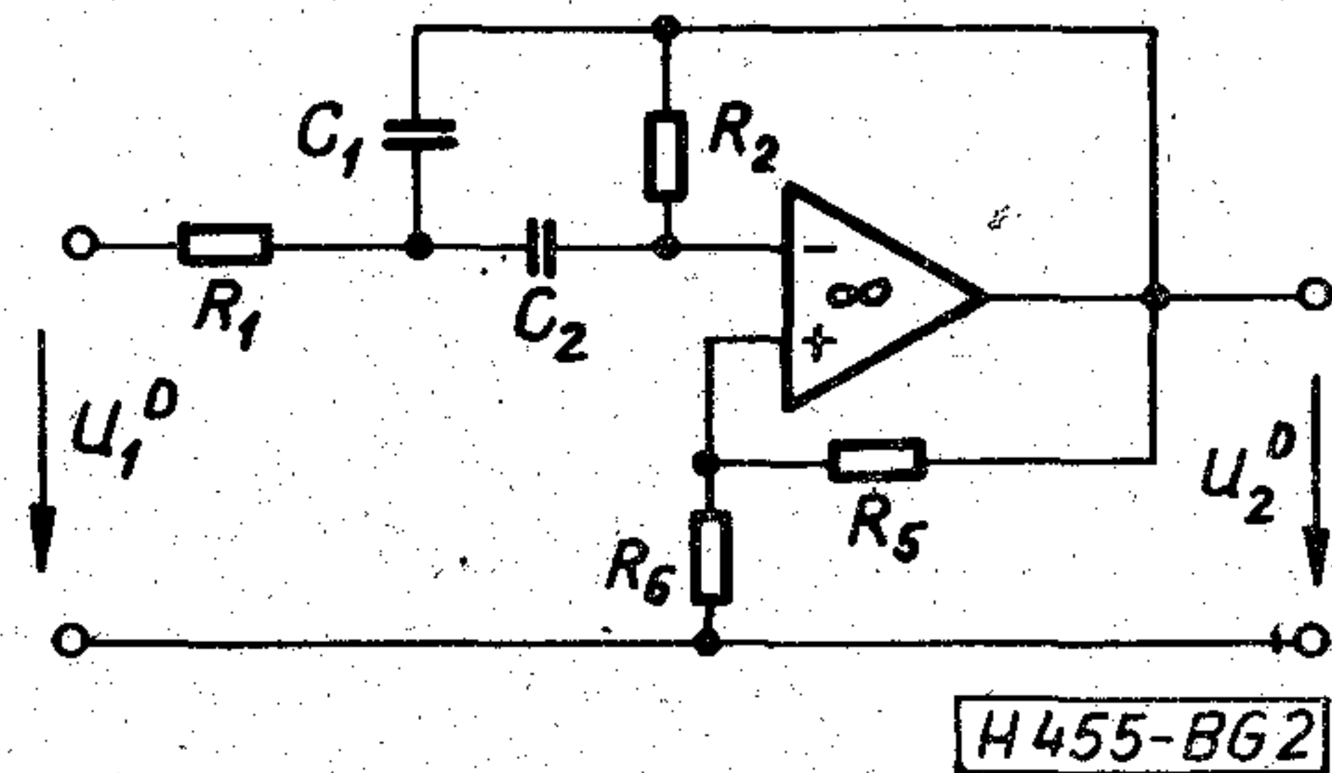
2. ábra. Deliyannis-féle sávszűrő alaptag
