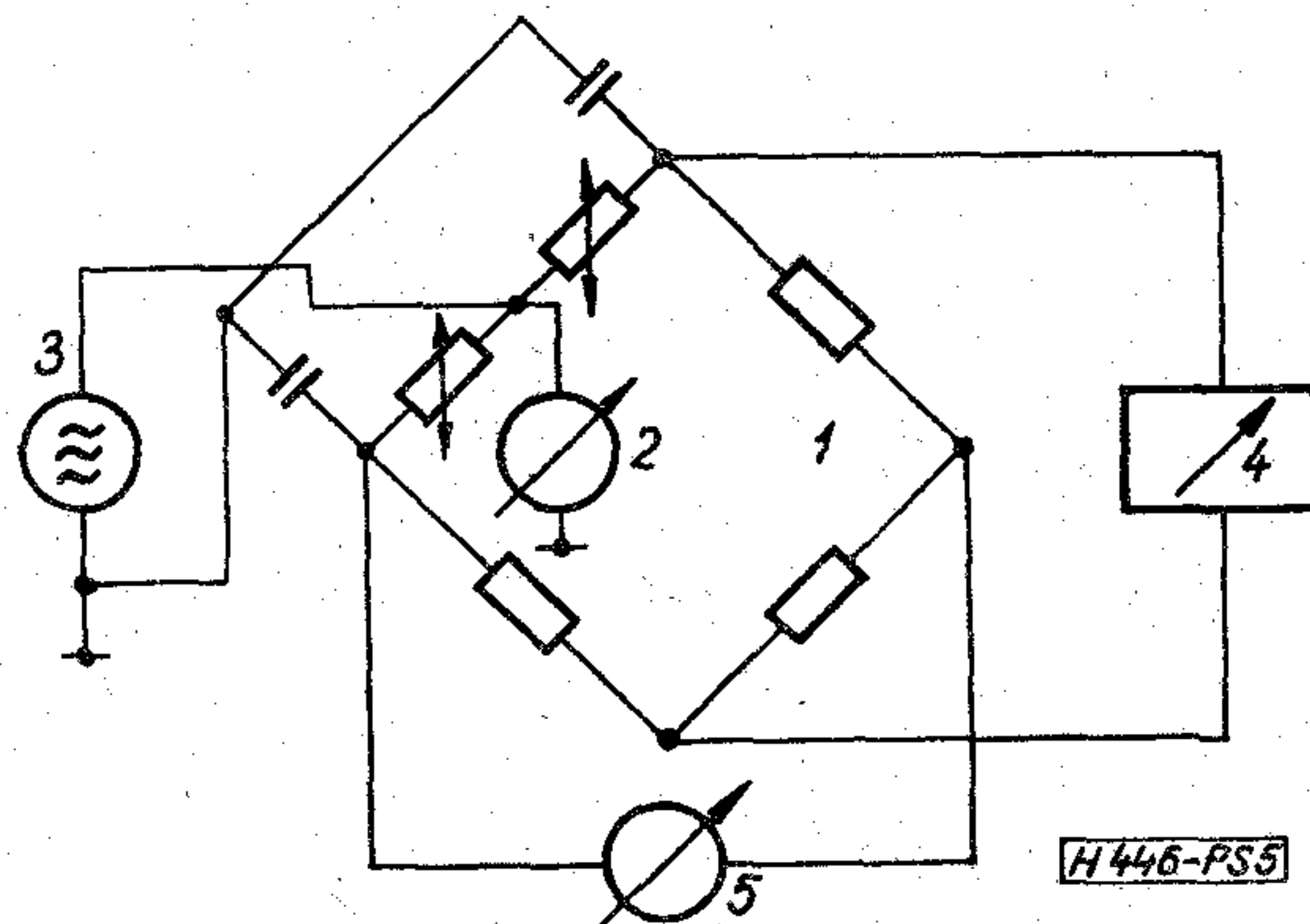
5. ábra. Kéttermisztoros, bolométeres feszültségmérő. 1. bolométer-híd, 2. vizsgálandó voltmérő, 4. változtatható egyenfeszültség-forrás, 5. nullindikátor
