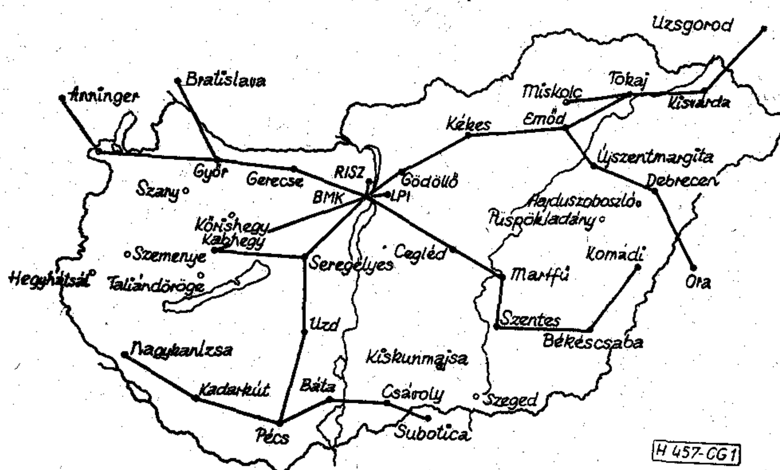
1. ábra. Az ország jelenlegi mikrohullámú gerinchálózatának nyomvonalrajza
