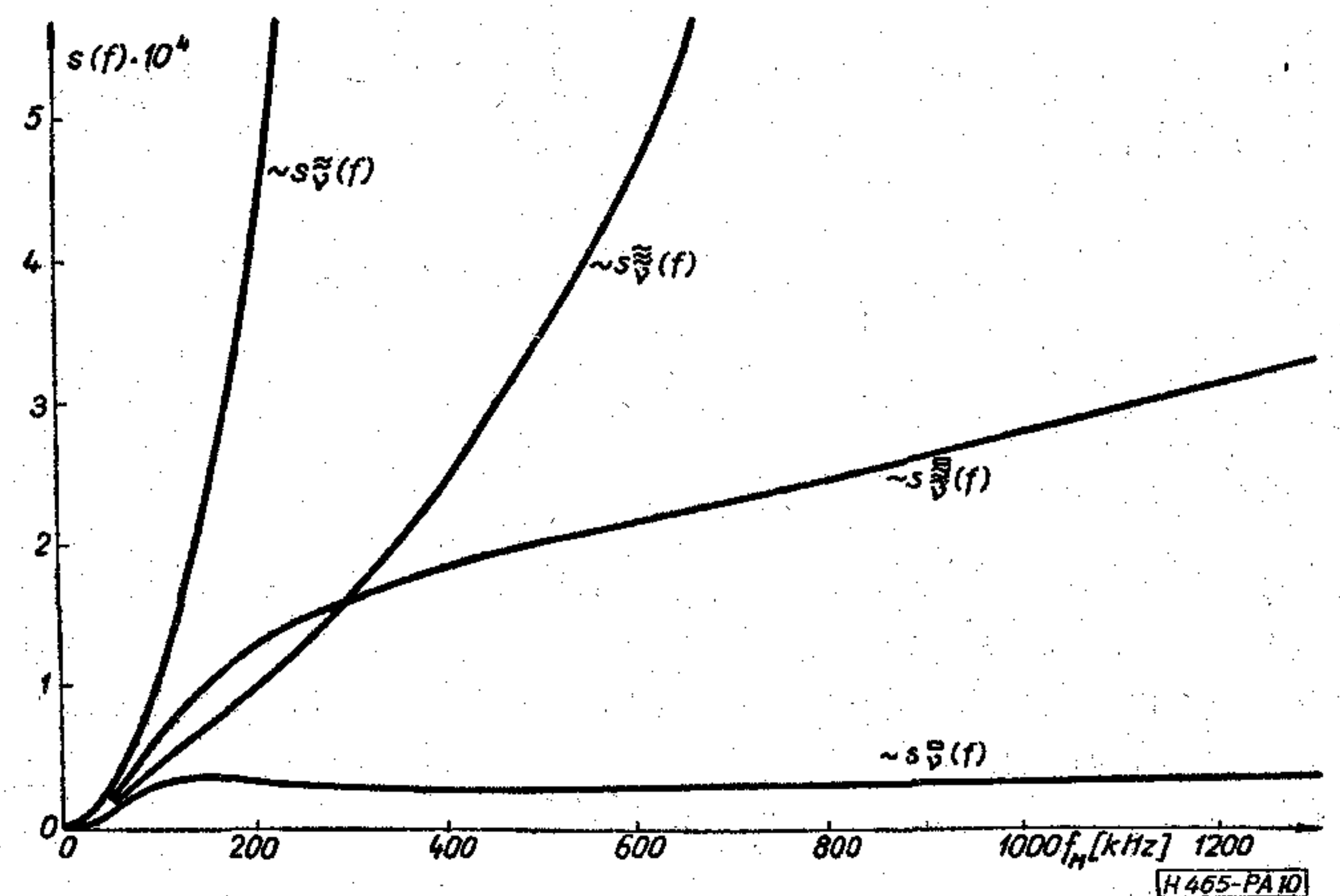
10. ábra. A jel—zaj viszony javulás számításánál fellépő spektrális sűrűségek
