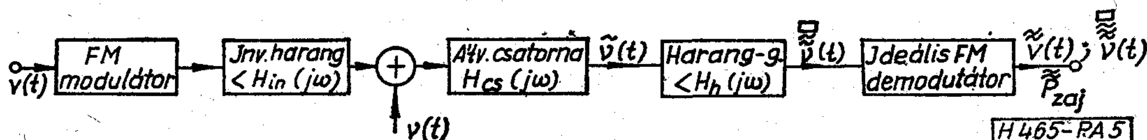
5. ábra. SECAM rendszerű jelátvitel egyszerűsített tömbvázlata, ha csak nagyfrekvenciás előkiemelést és utóelnyomást tételezünk fel
