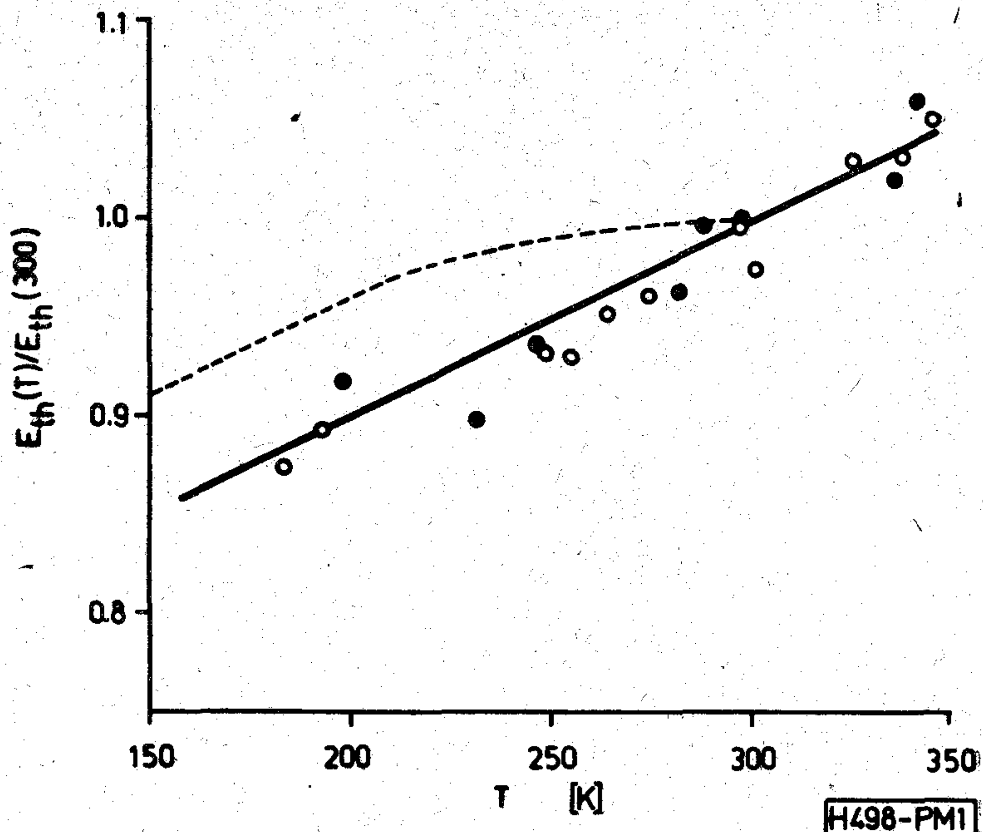
1. ábra. A küszöbfeszültség relatív értéke a hőmérséklet függvényében. ○, ● — két diódán mért értékek, szaggatott vonal — a [8]-ben közölt planáris Gunn-diódán mért E_{th}(T)/E_{th}(300\text{ K}) értékek
