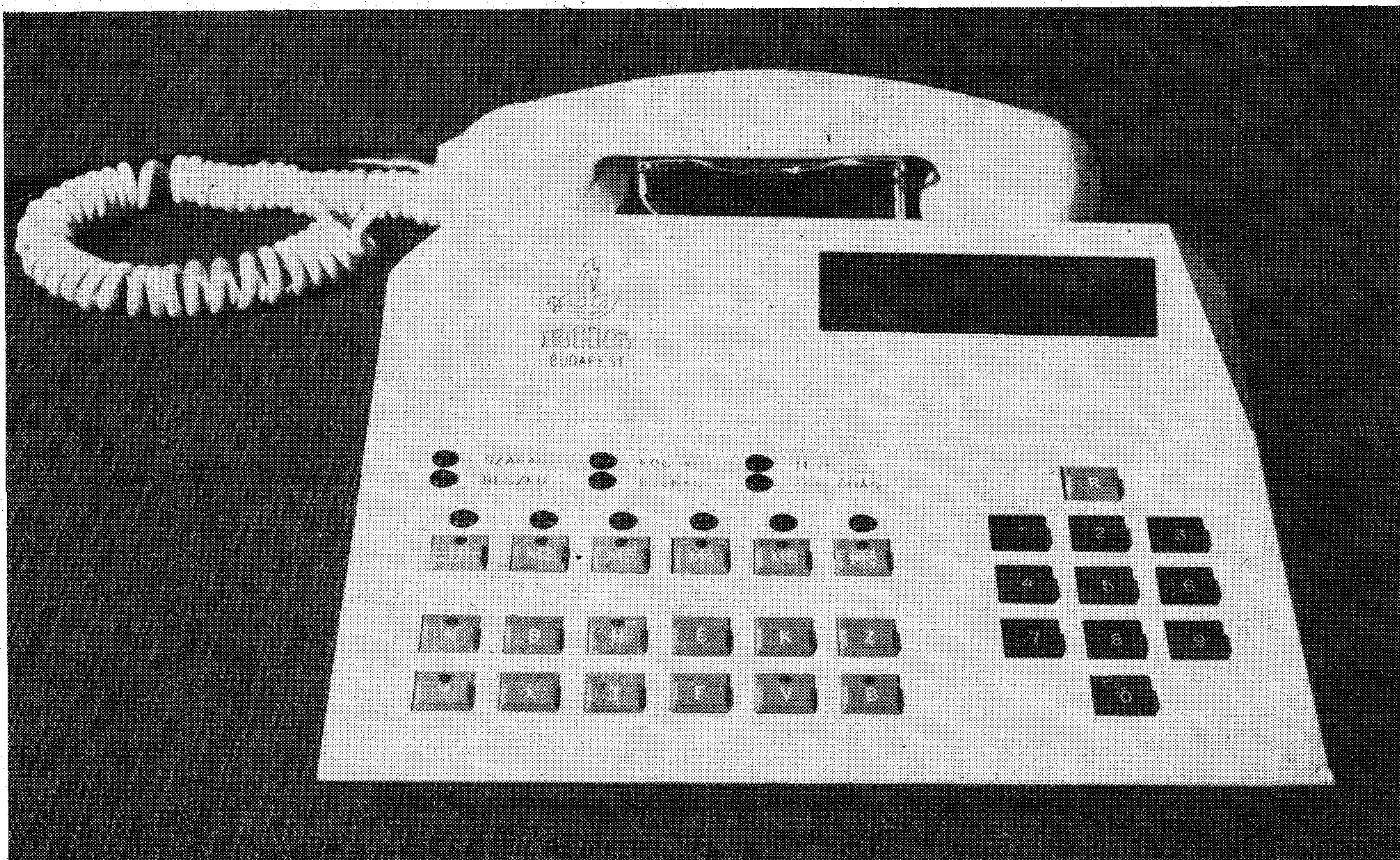
2. ábra. Újvonalú kezelőkészlet a QA 96 típusú alközpontozóhoz
