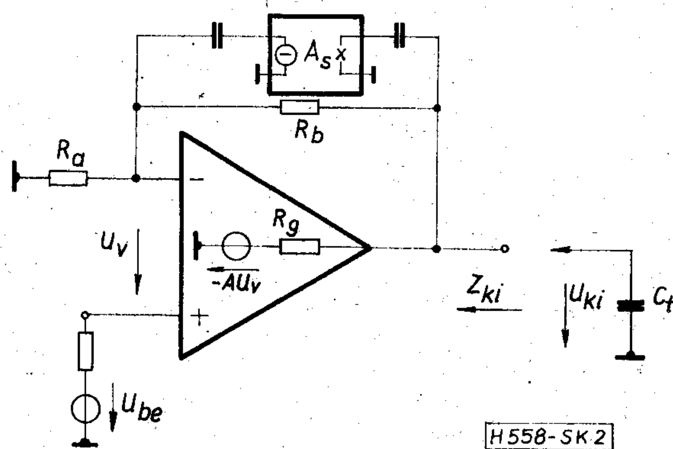
2. ábra. A visszacsatolás célszerű módszere kapacitív terhelésnél
