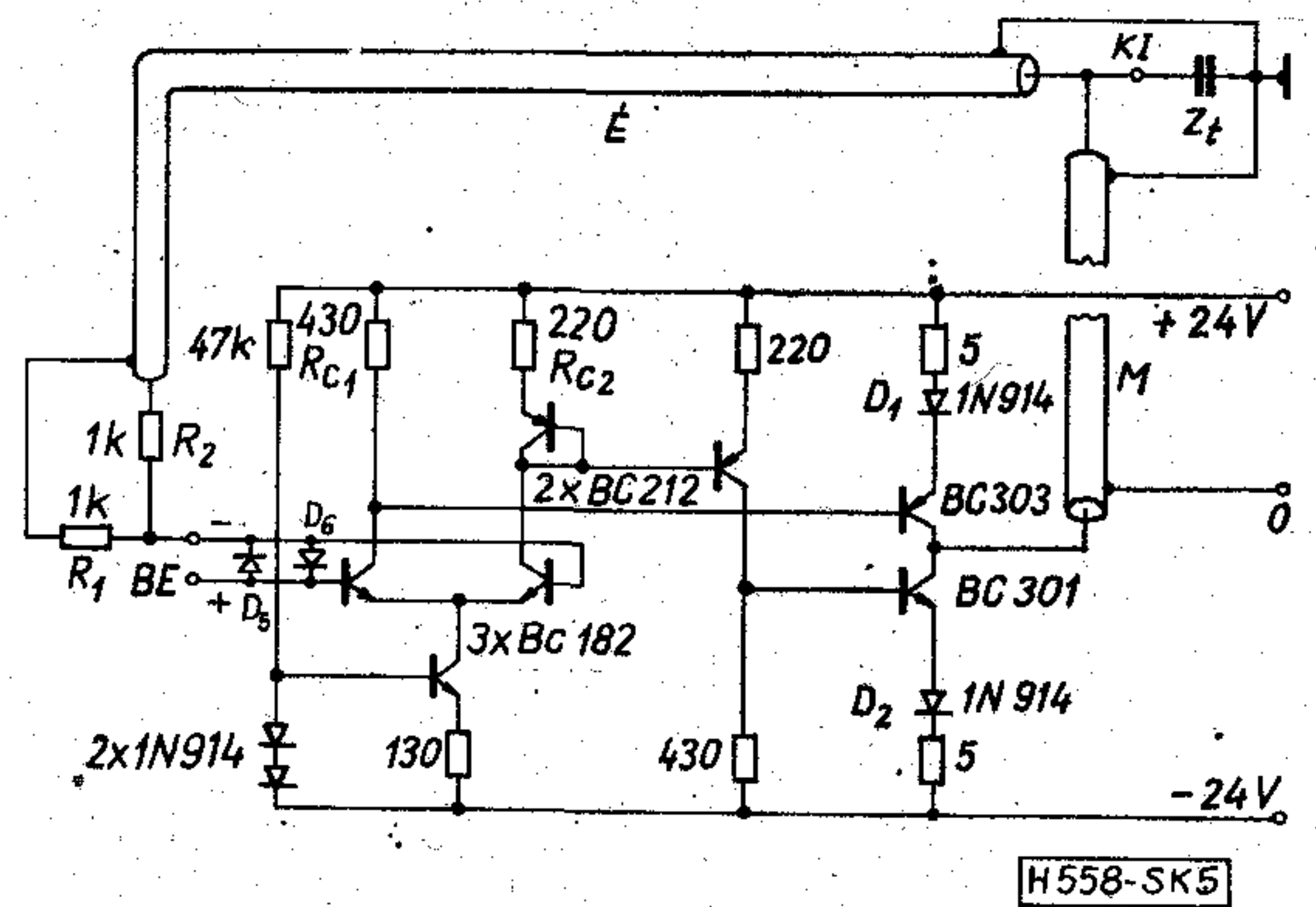
5. ábra. A végfokozat kapcsolási rajza
