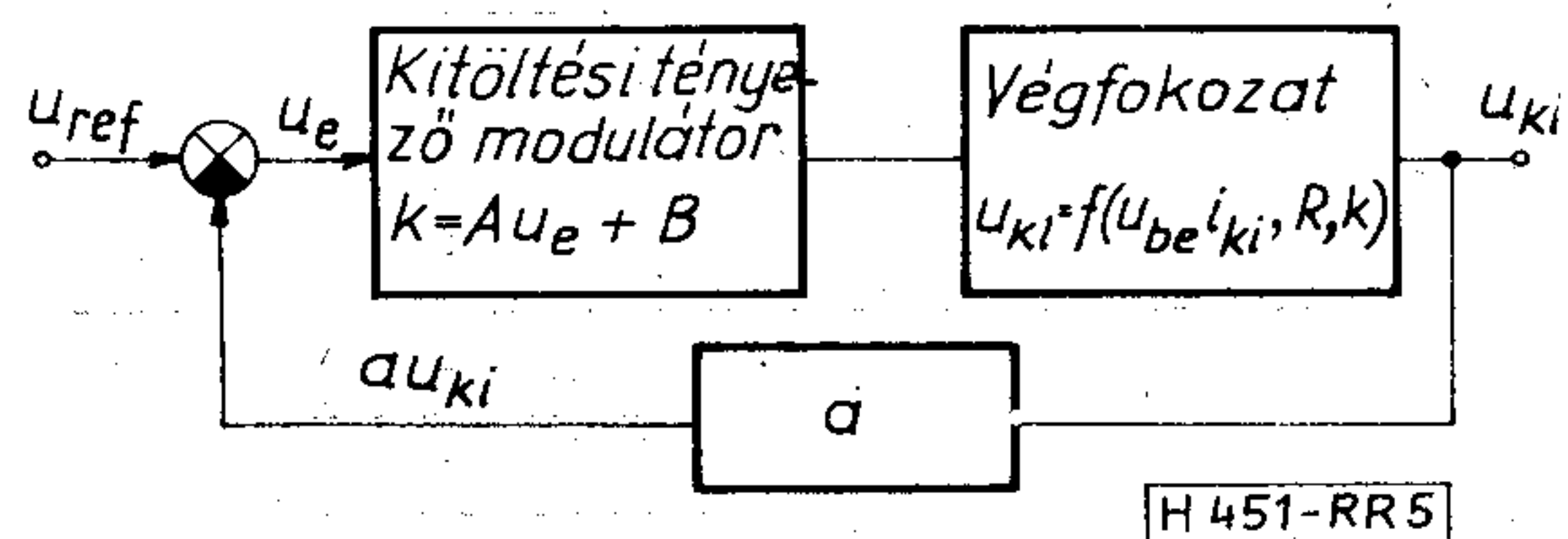
5. ábra. Nagyjelű visszacsatolt modell
