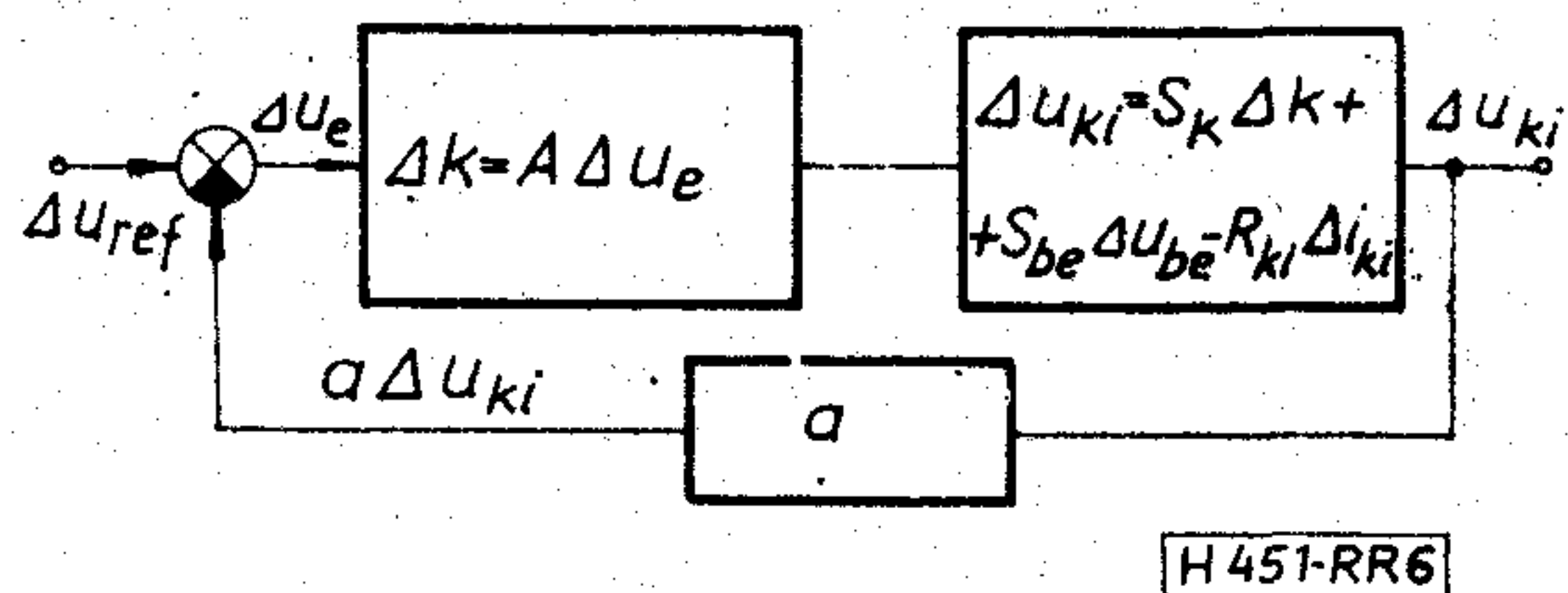
6. ábra. Kisjelű (linearizált) visszacsatolt modell
