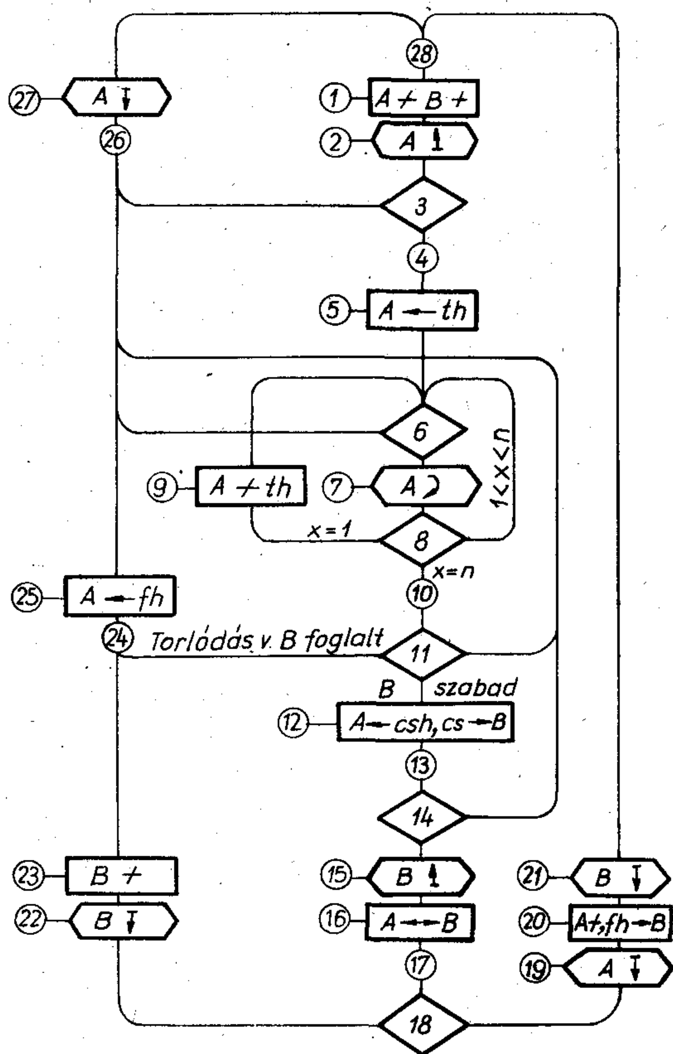
2. ábra. Egyszerű központ folyamatábrája, csak rendes kezelés esetén beadott bemenő jelekkel
