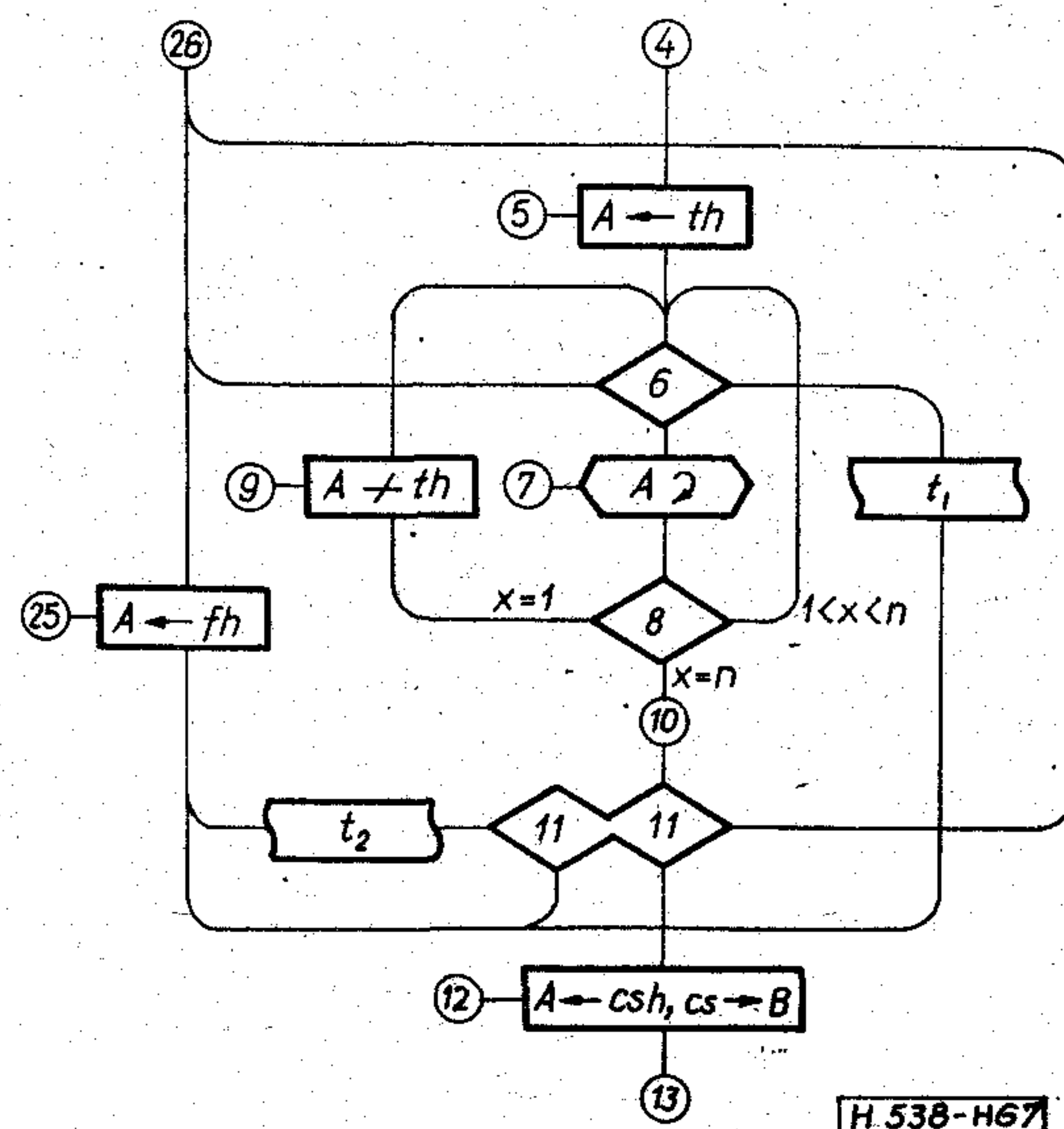
7. ábra. Tárcsázás és választás időzítése:
