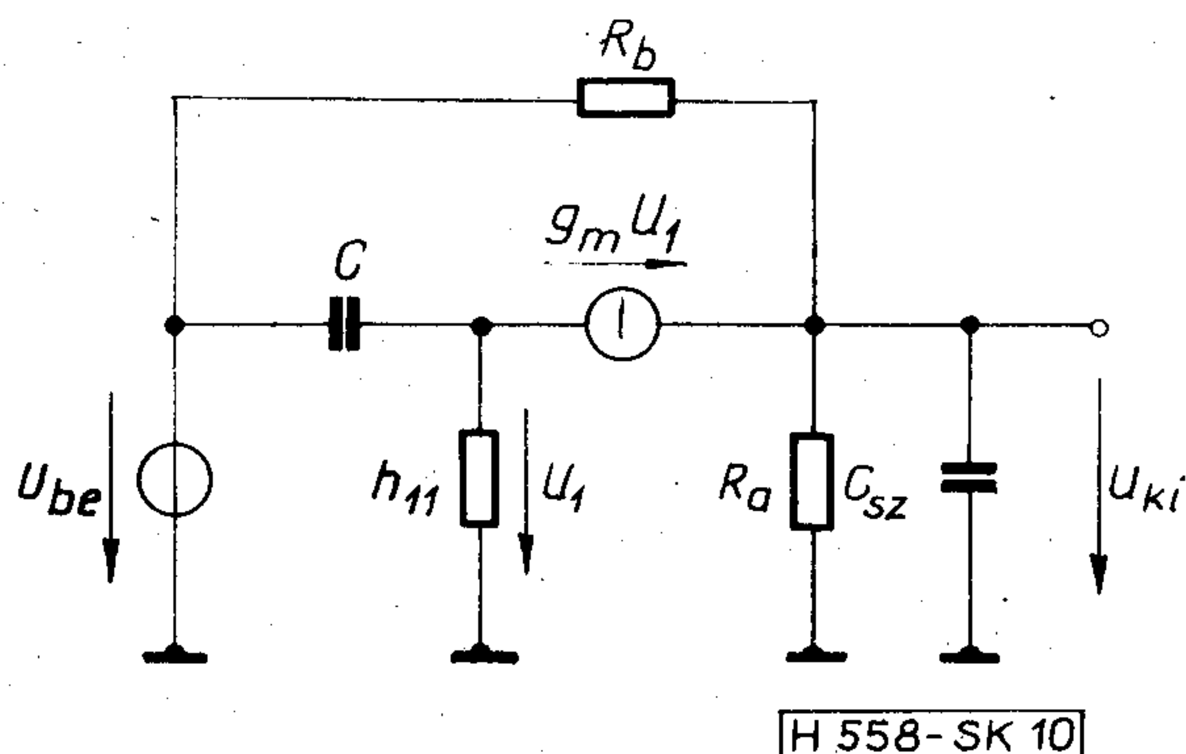
10. ábra. A visszacsatoló áramkör helyettesítő képe
