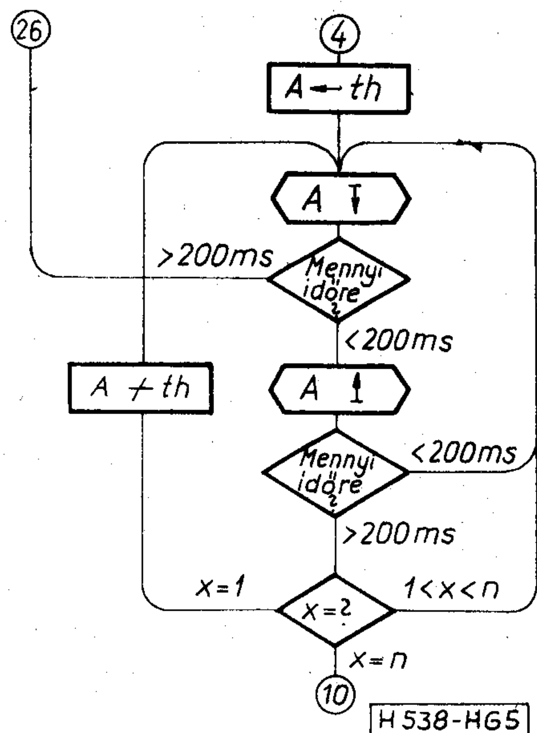
5. ábra. Tárcsázás folyamatábrája áramkörü szinten
