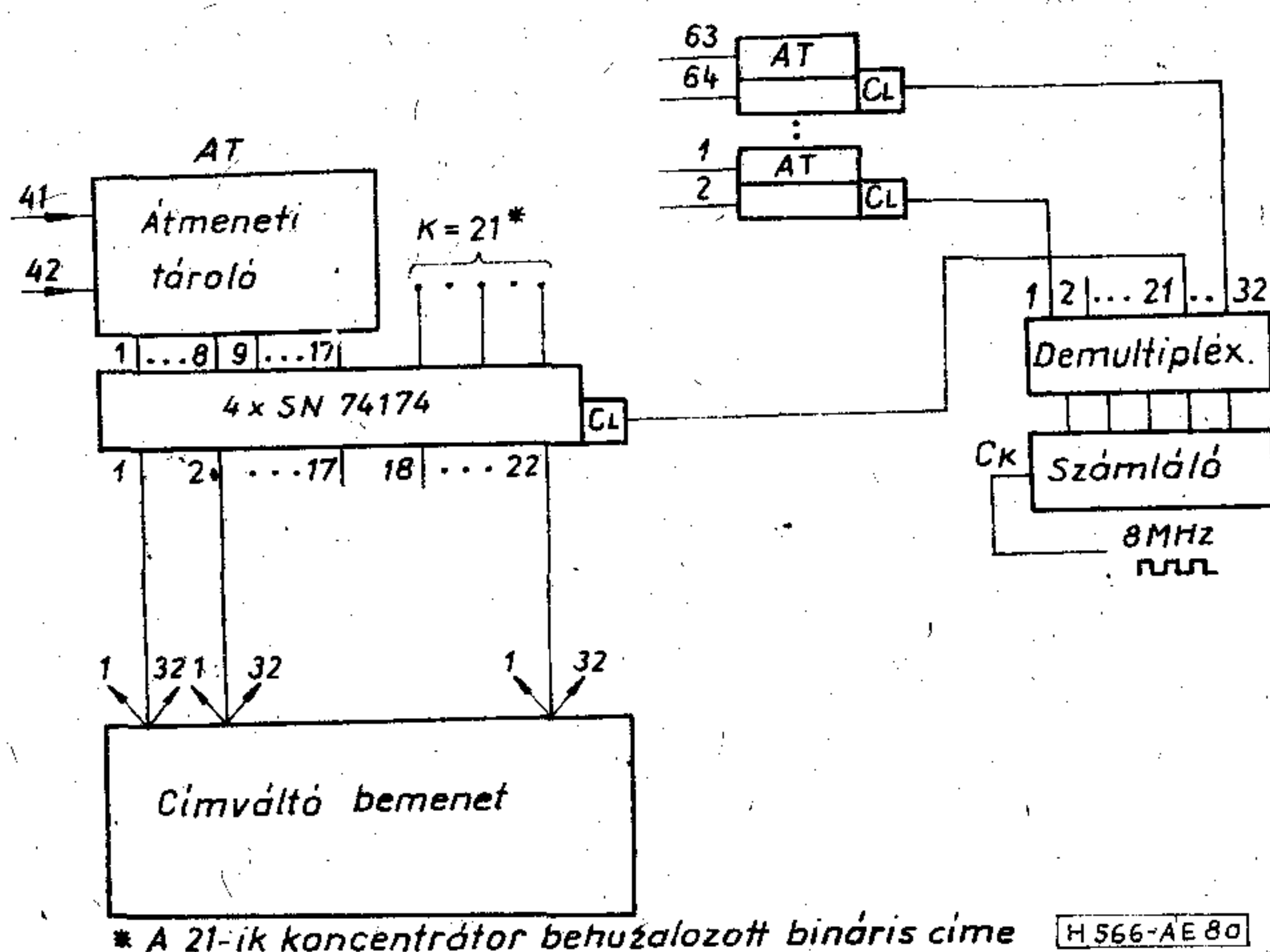
8a ábra. A-egység bemenet (részlet). Feltételezzük, hogy egy koncentrátorból 2 láncon 29 időrsben jönnek a 17 bites AKS kódok. Ezek a 3/B1 ábra szerinti módon, egymás után léptethetők ki a kódváltó keretre. Legyen a koncentrátor pl. K = 21 .
