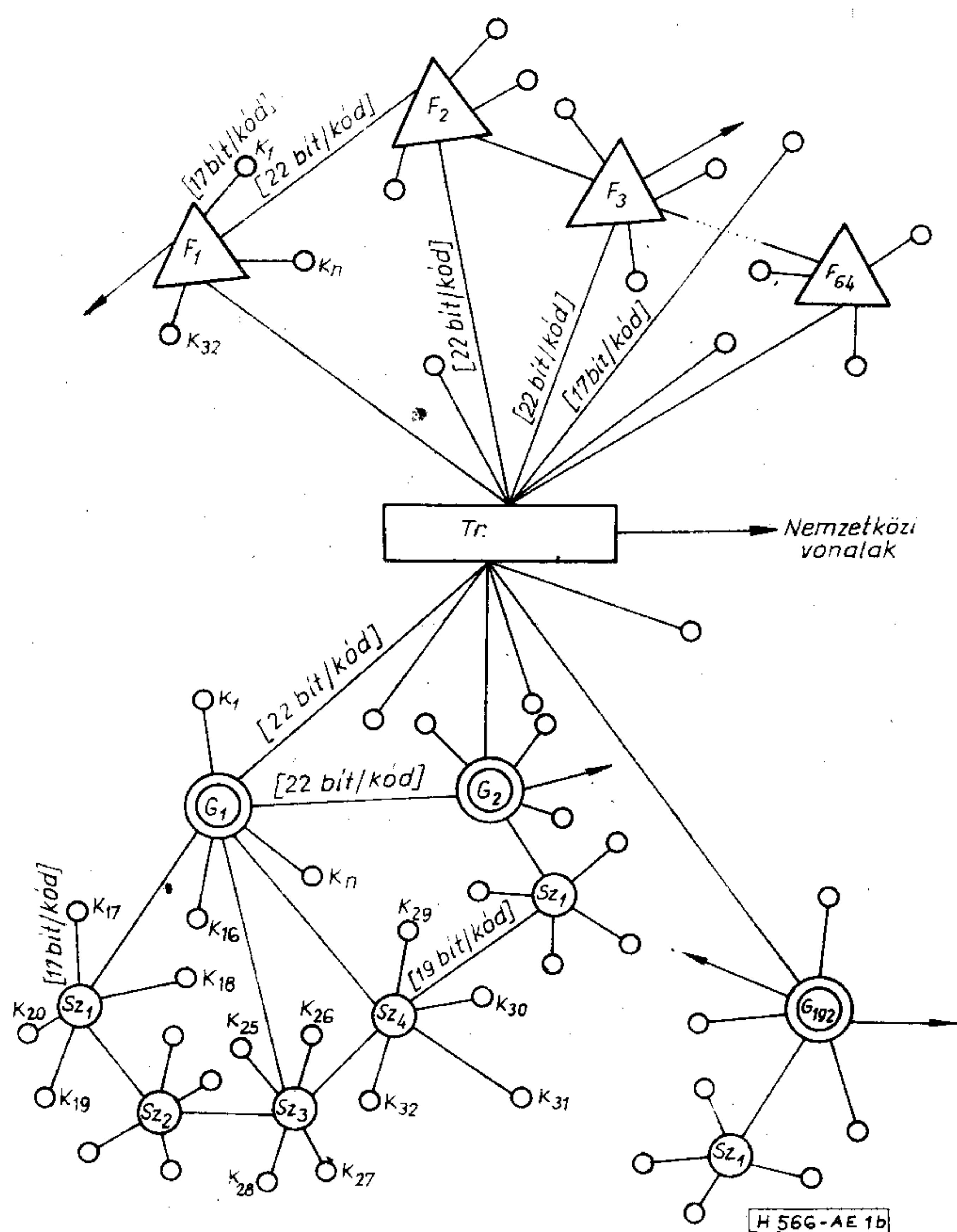
1b ábra. A 4 millió vonalas országos hálózat: 1 db trónkközpont Tr, 64 db 16 000 vonalas főközpont F, 192 db 16 000 vonalas gócközpont G, melyben 768 db 2000 vonalas szektorközpont Sz és 8192 db 512 vonalas koncentrátor K van
