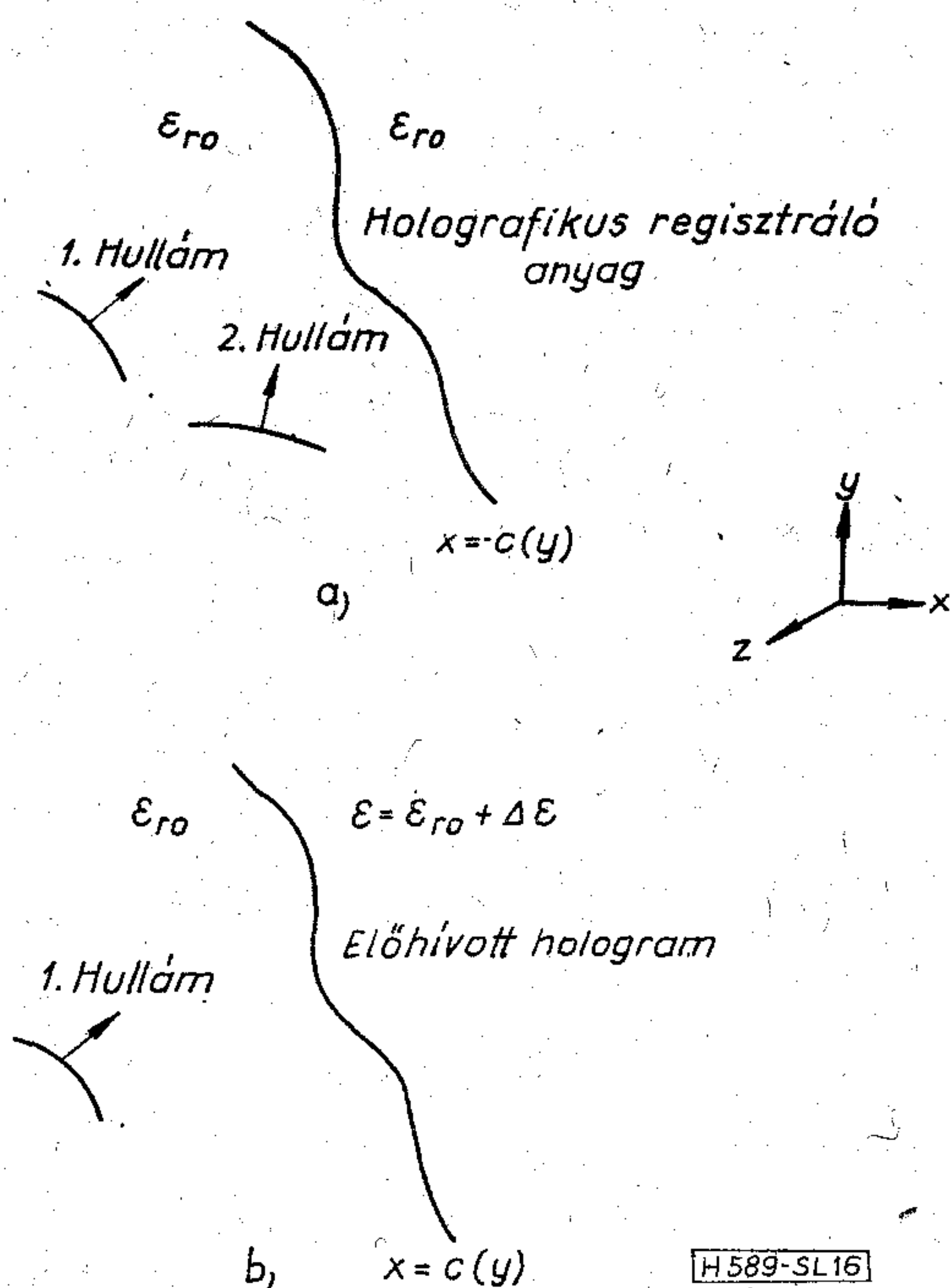
16. ábra. a) Hologram felvétele két sugár segítségével, b) az előhívott hologram referenciahullámmal való megvilágítása, x = c(y) a holografikus anyagot határoló görbe, ami a legtöbb gyakorlati esetben egy egyenes
