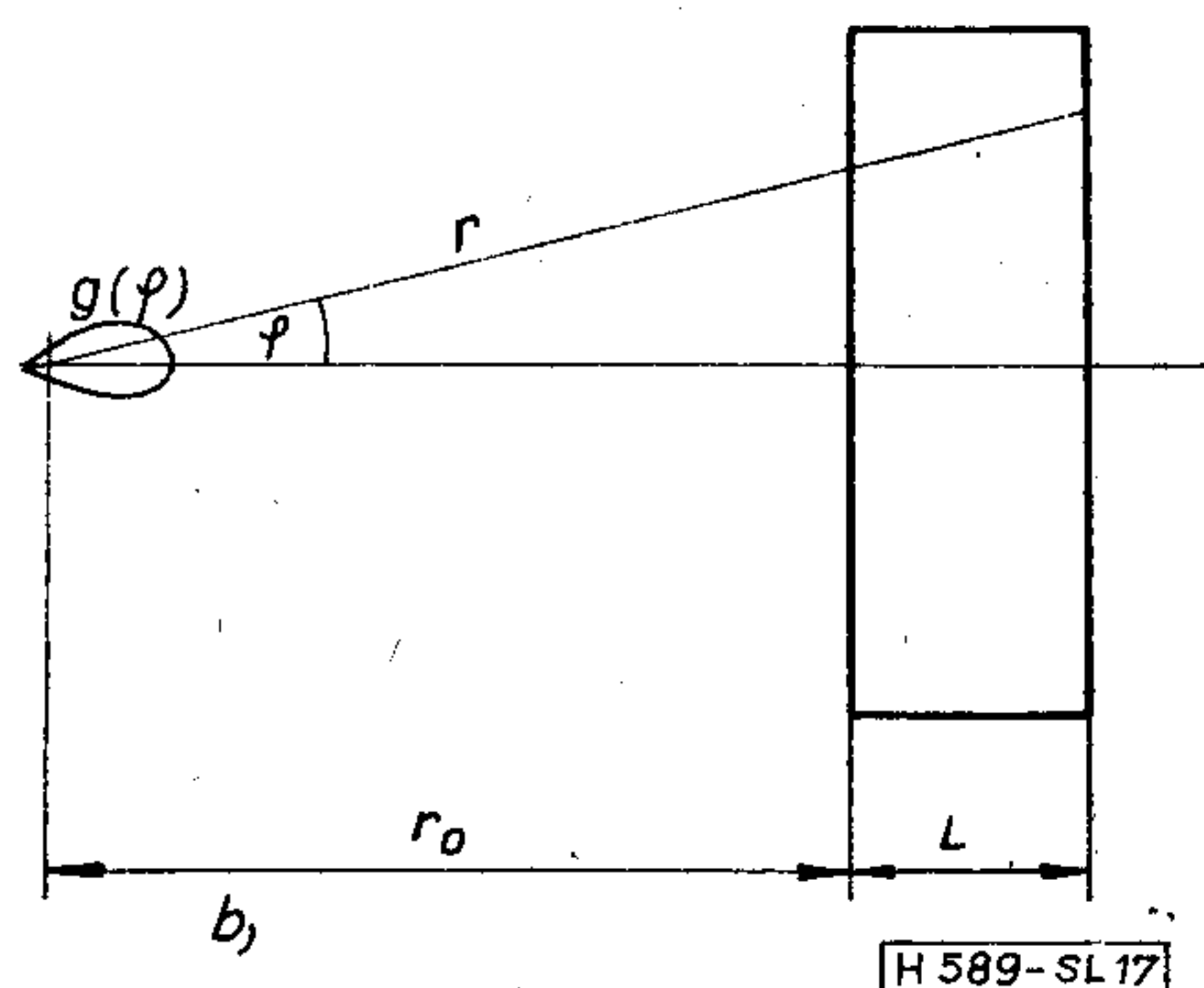
17. ábra. a) Hengeres, b) sík bemenő felületű hologram, amelyek hengerhullámnak síkhullámmá való átalakítására szolgálnak
