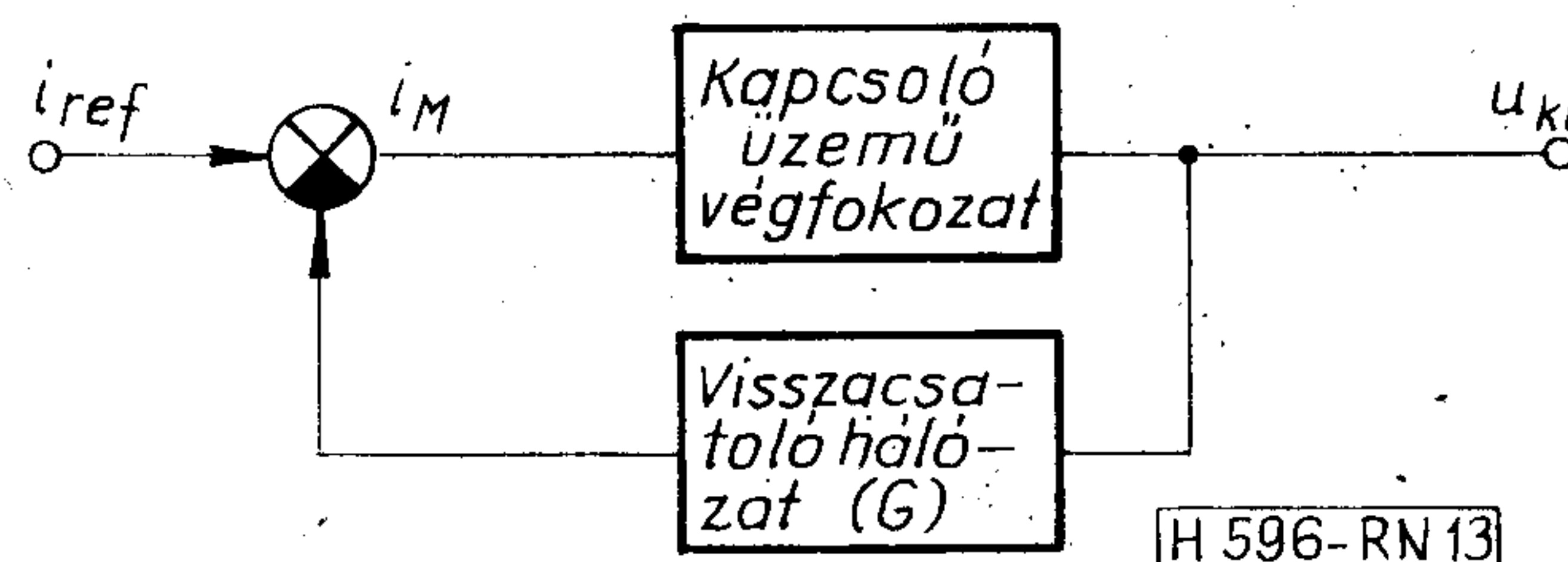
13. ábra. A visszacsatolt áramvezérelt stabilizátor tömbvázlata
