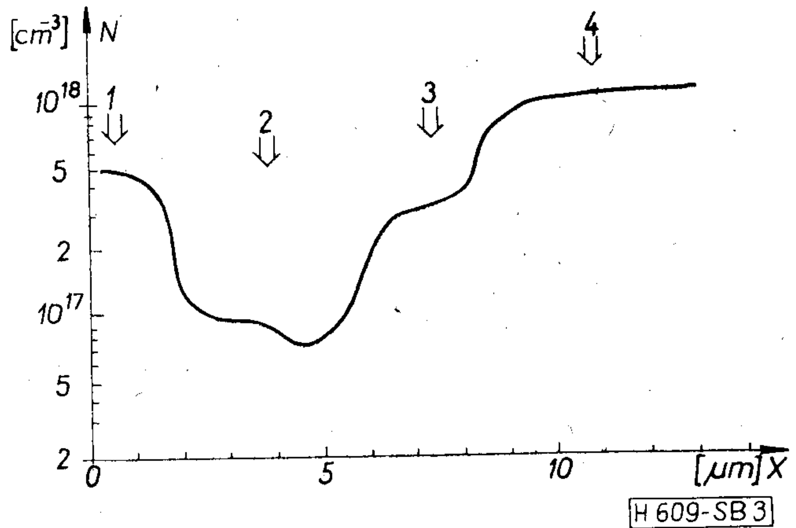
3. ábra. A SZUTA Novoszibirszki Félvezető Intézetében készített GaAs epitaxia profilja. A jelölt szakaszok: 1. n* kontaktálást megkönnyítő fedőréteg; 2. aktív réteg; 3. buffer réteg; 4. hordozó kristály
