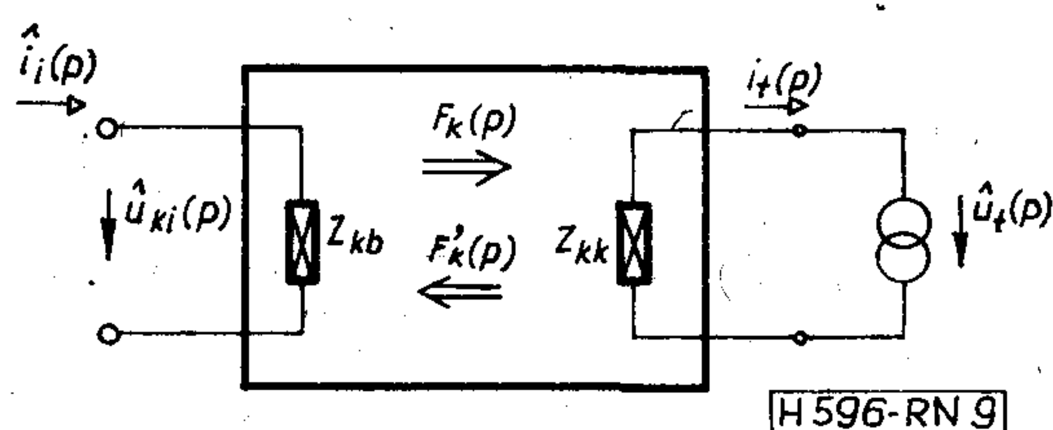
9. ábra. Kimeneti szűrő
