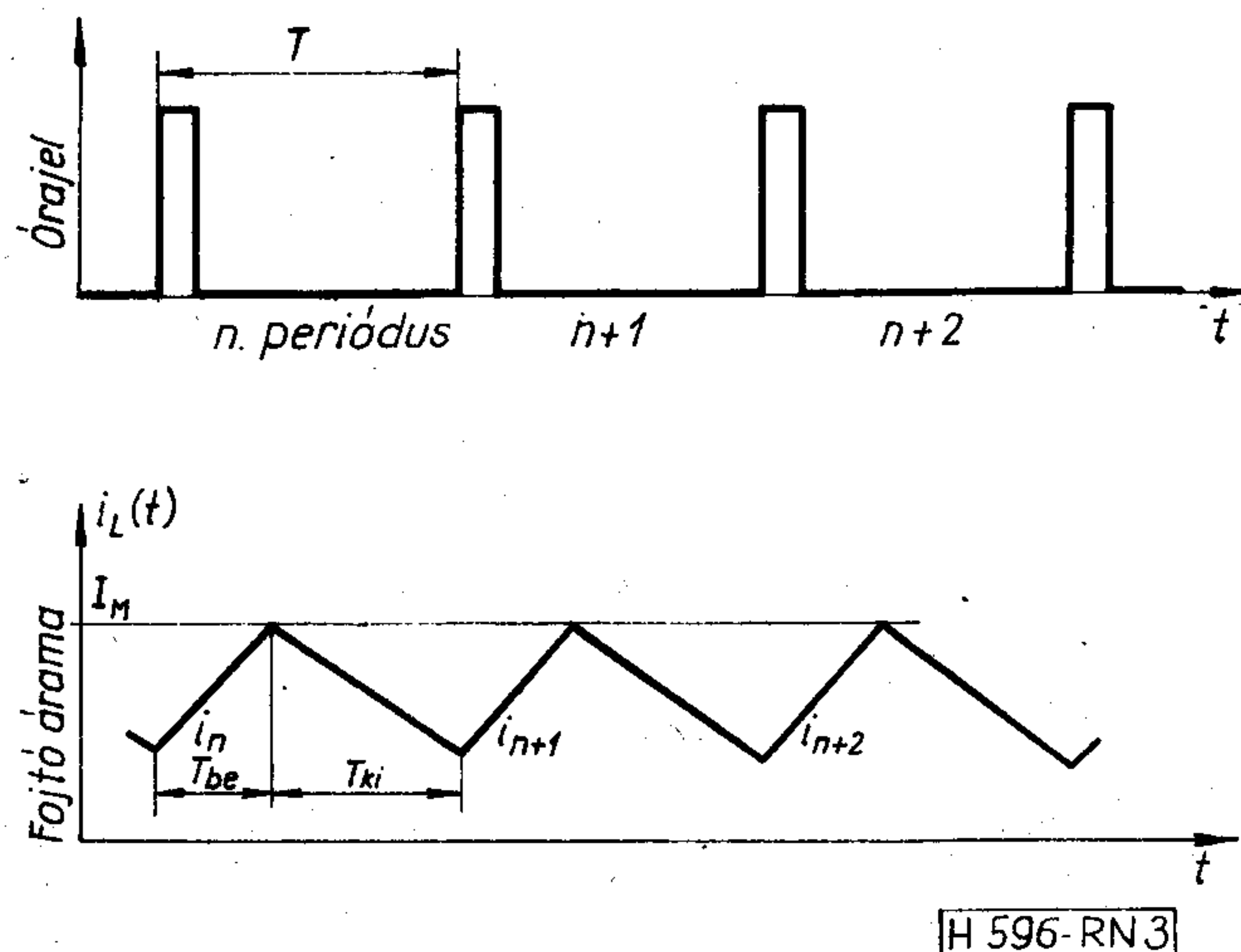
3. ábra. Jelalakok az állandó frekvenciájú működés vizsgálatához
