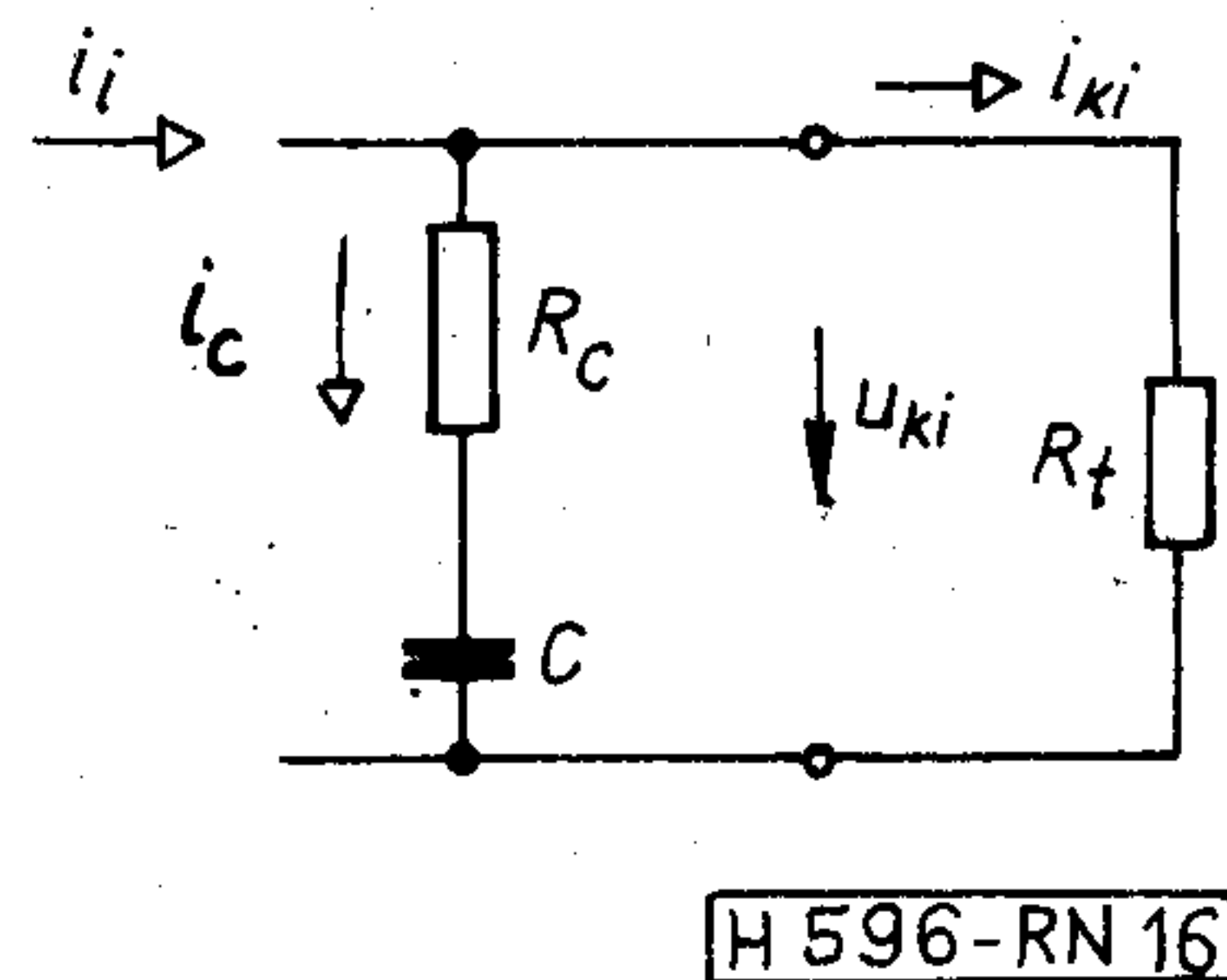
16. ábra. A kimeneti szűrőkondenzátor és a terhelés helyettesítő képe
