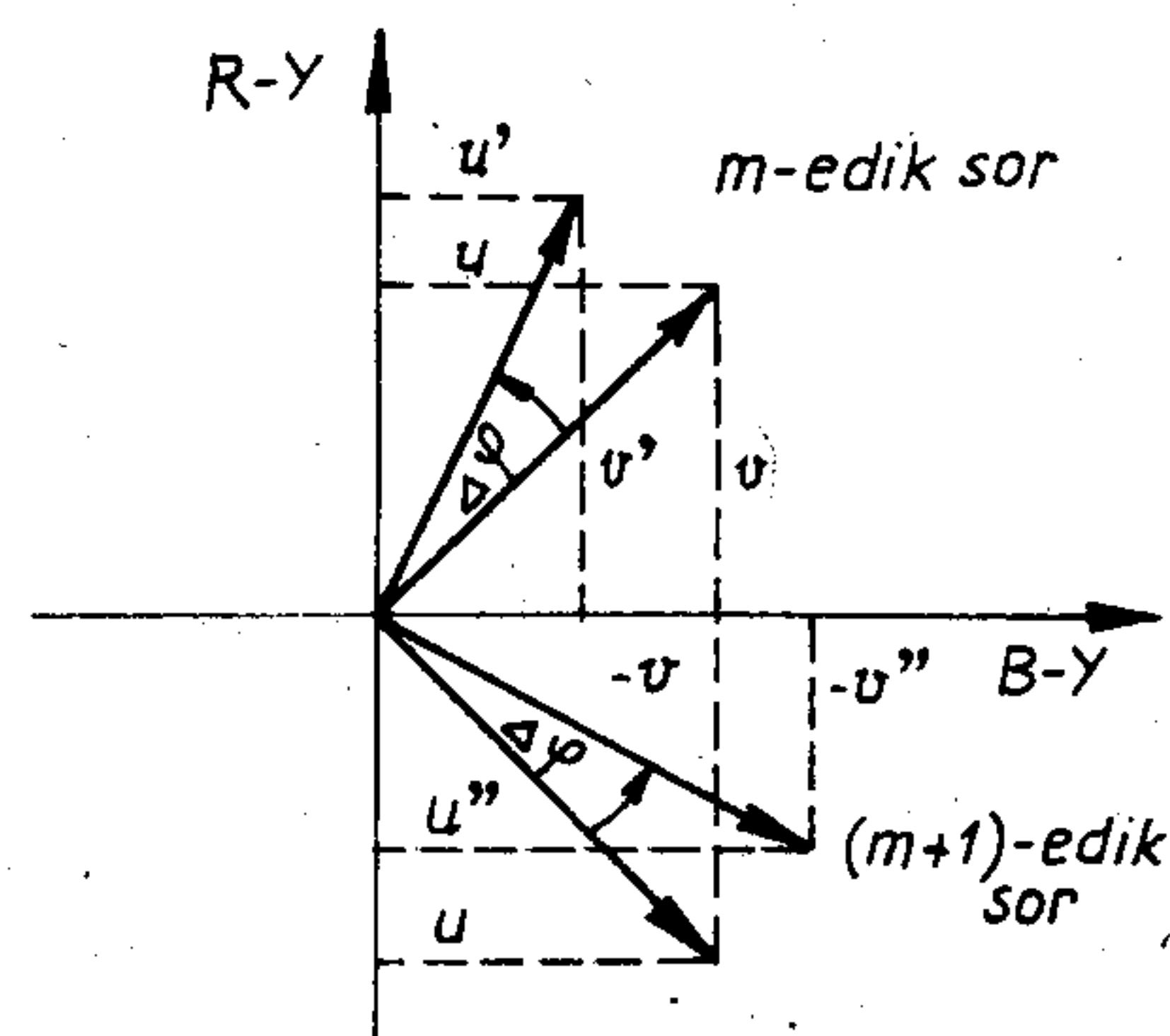
2. ábra. A fázistorzítás hatásának szemléltetése
