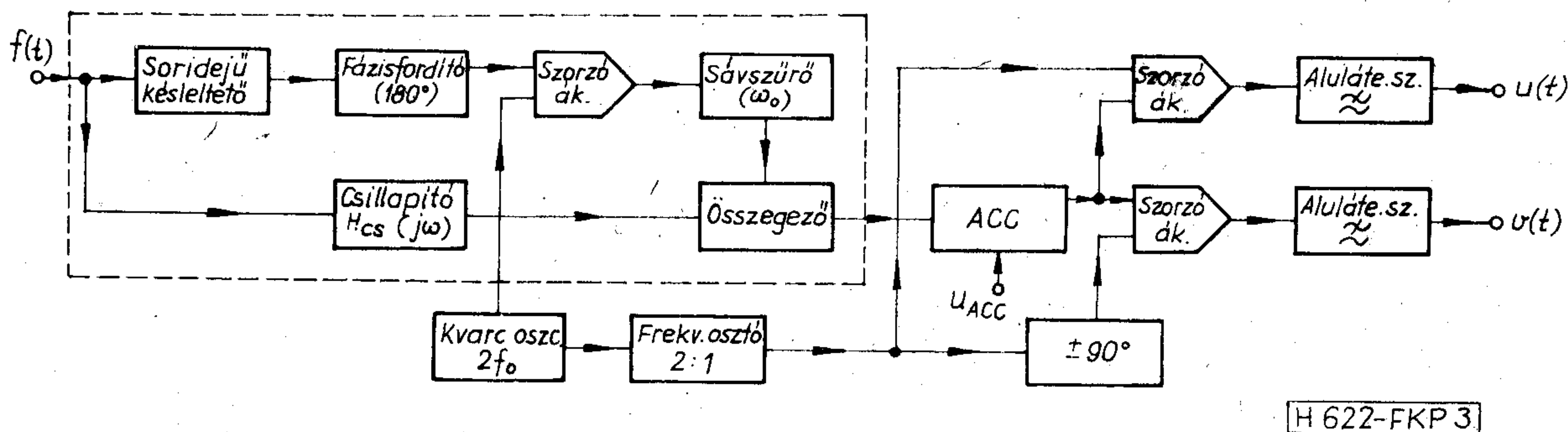
3. ábra. A dekóder tömbvázlata
