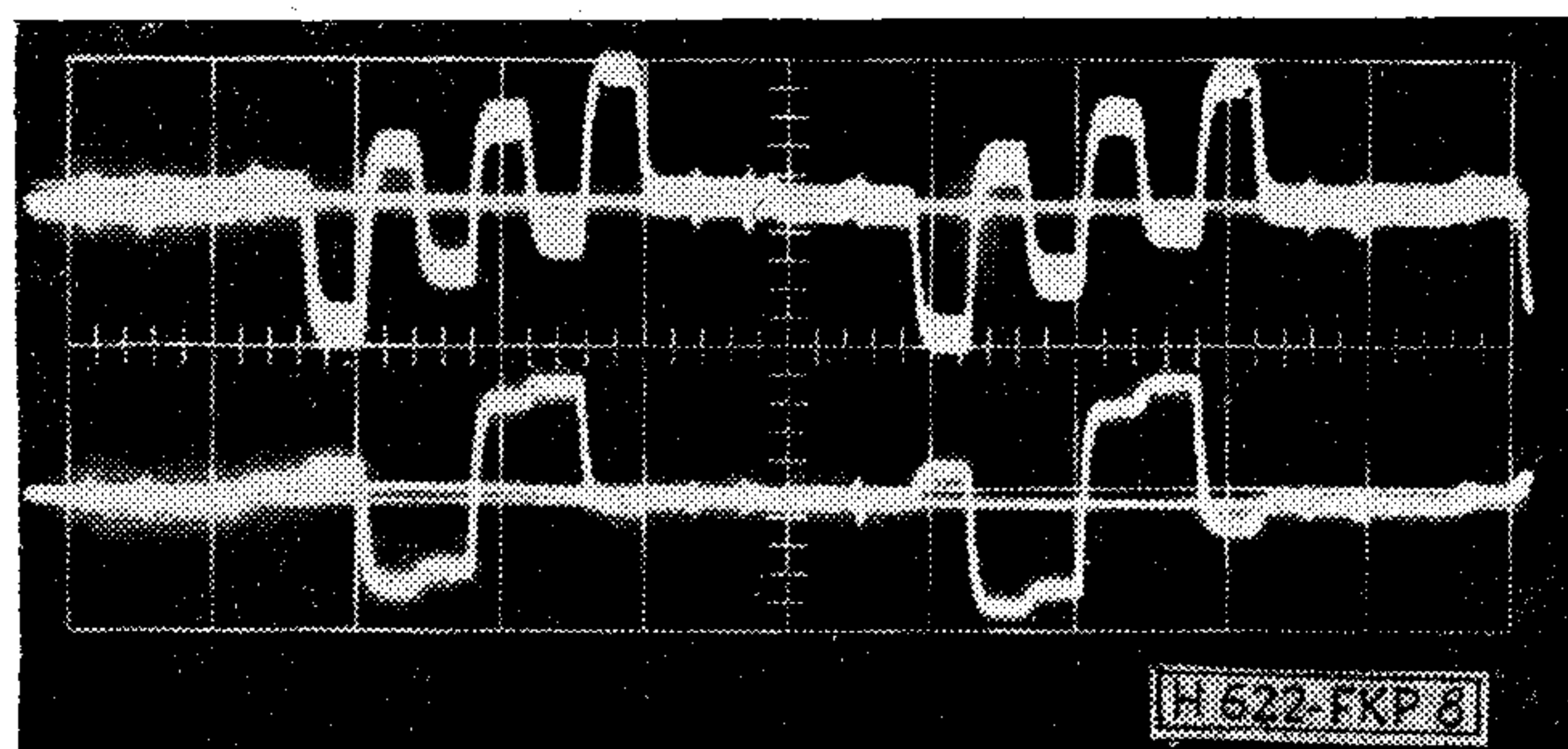
8. ábra. Demodulált B—Y és R—Y jelek idődiagramjai
