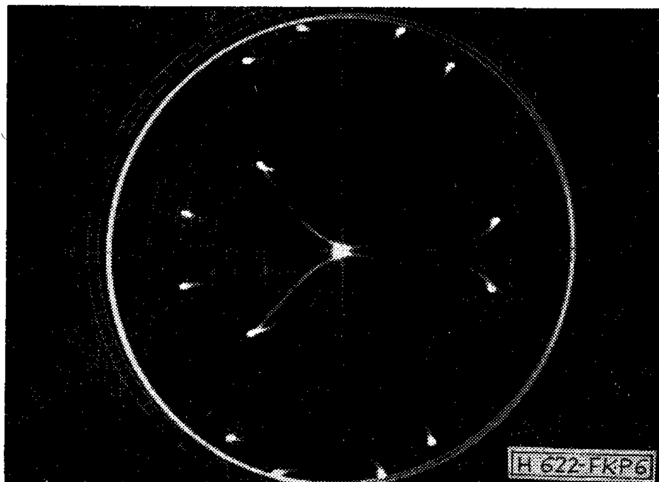
6. ábra. Y-jelről leválasztott PAL jel vektordiagramja
