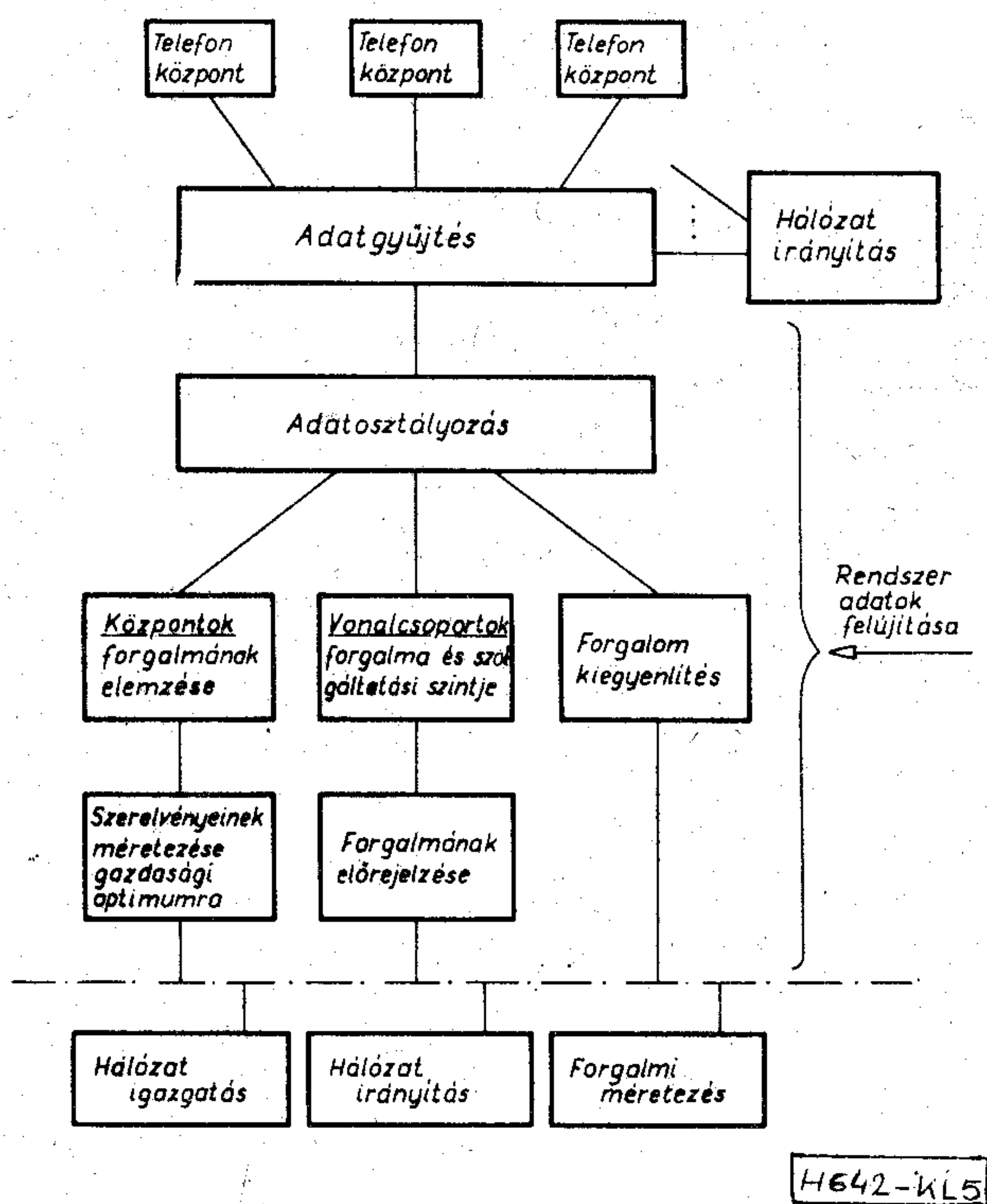
5. ábra. A TNDS rendszer vázlata
