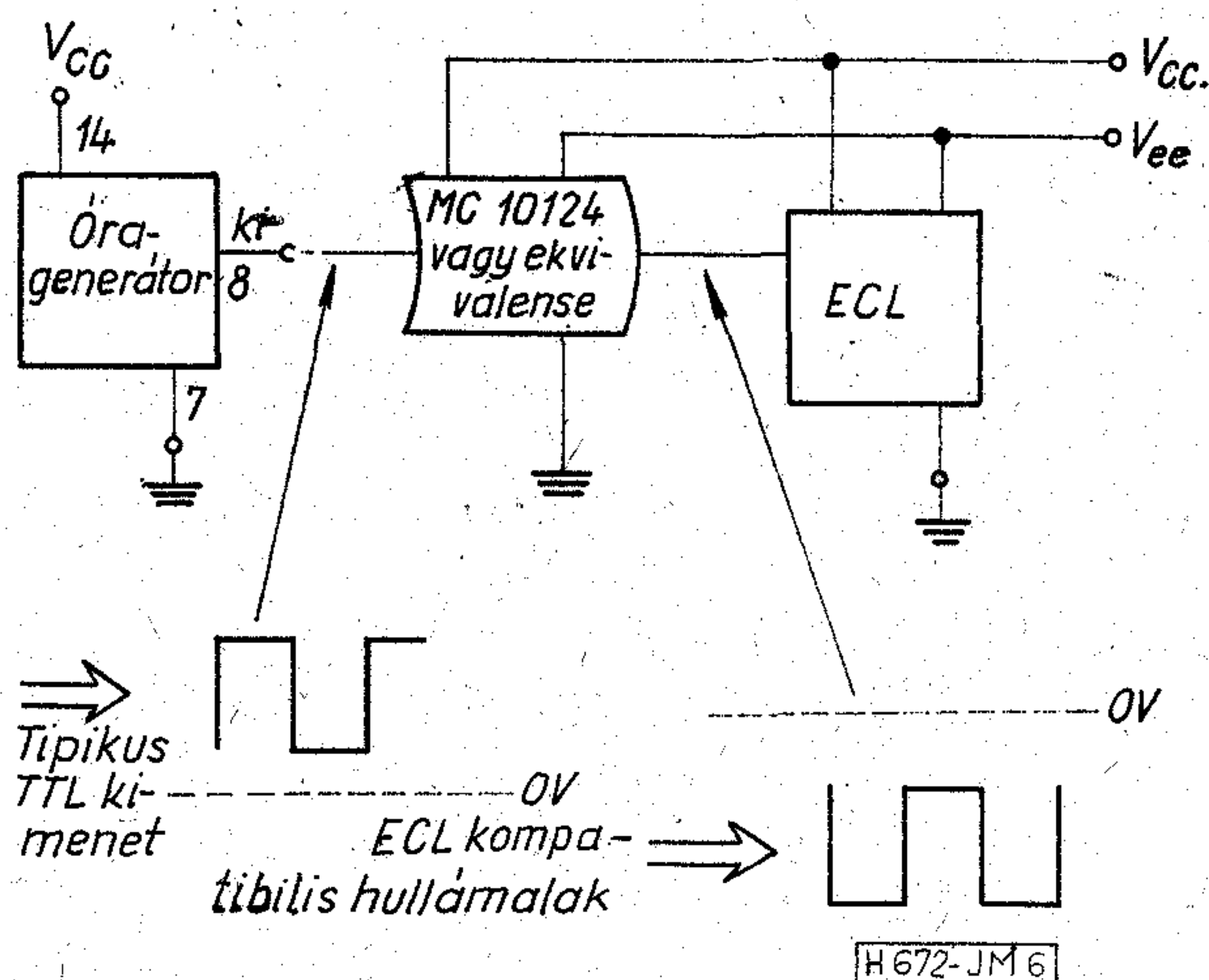
6. ábra. TTL/ECL csatlakozó áramkör
