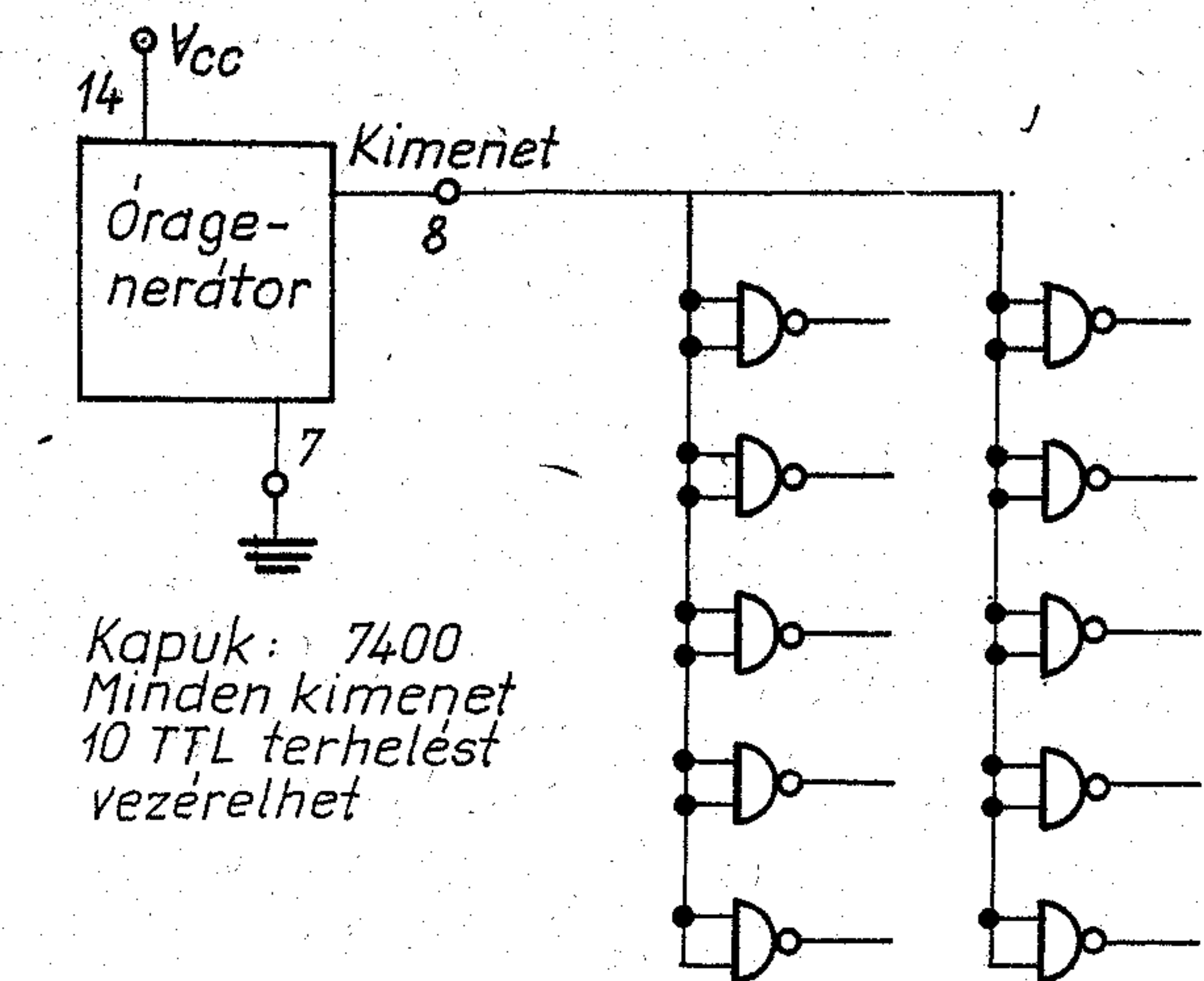
2. ábra. Terhelhetőség
