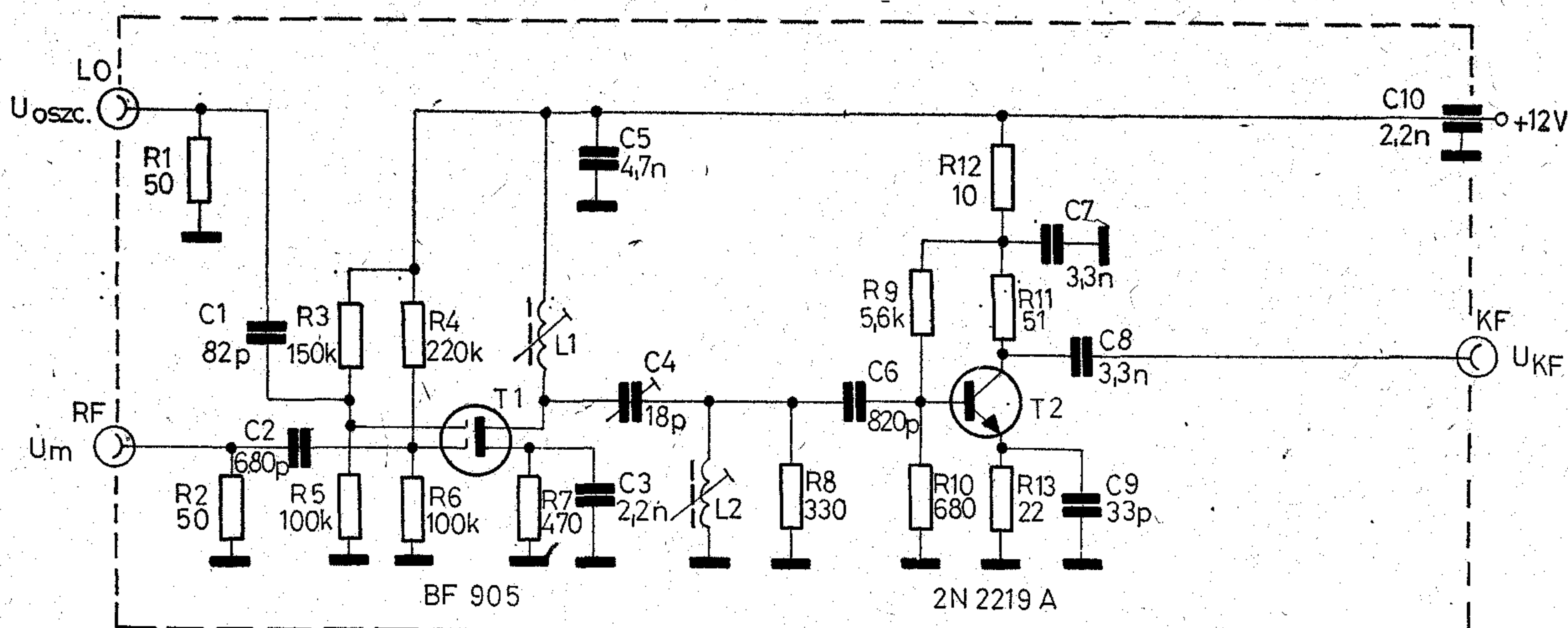
10. ábra. Szélessávú keverőkapcsolás BF 905 típusú dualgate MOSFET-tel
