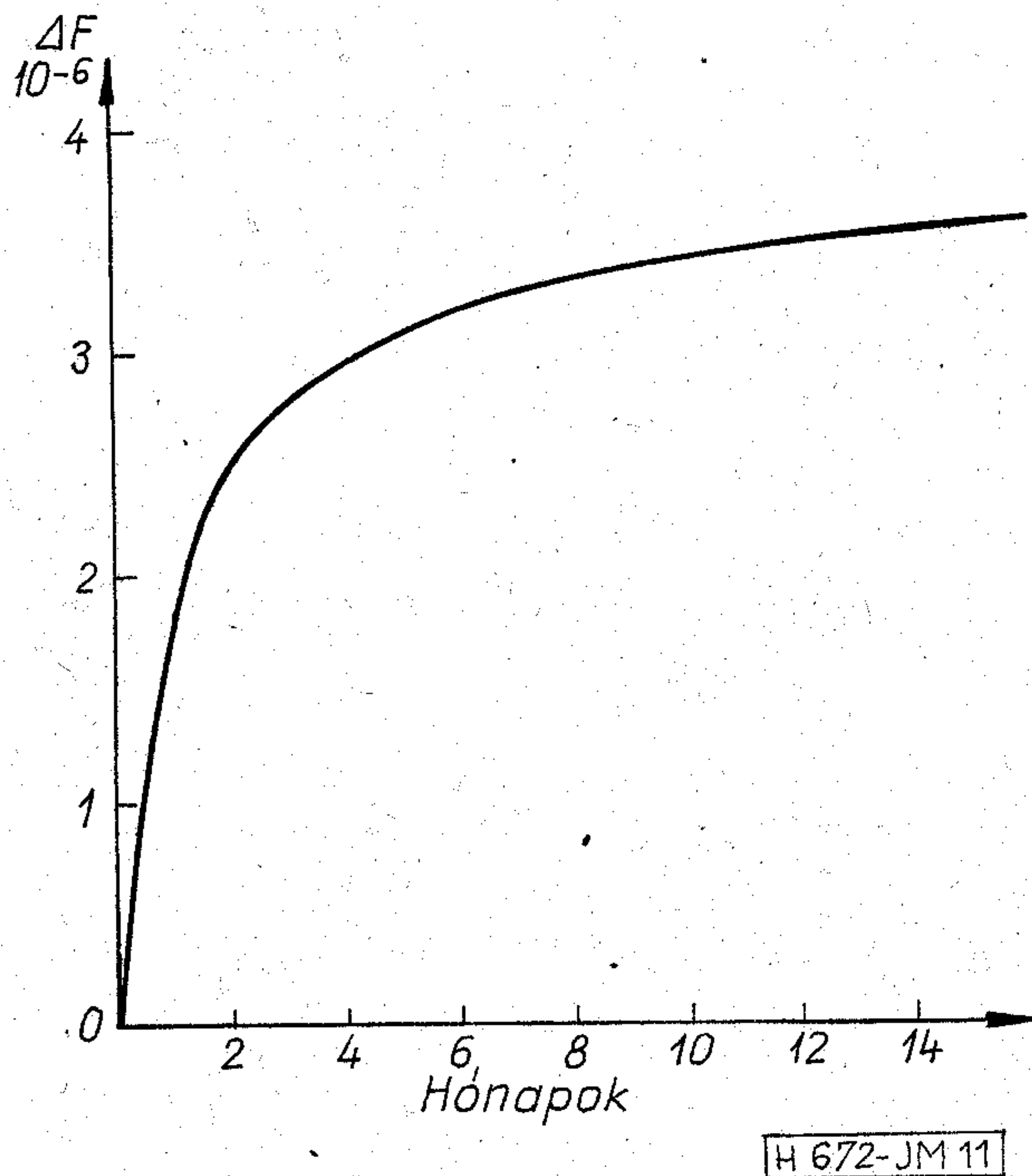
11. ábra. A frekvencia változása az idő függvényében (öregeedés)
