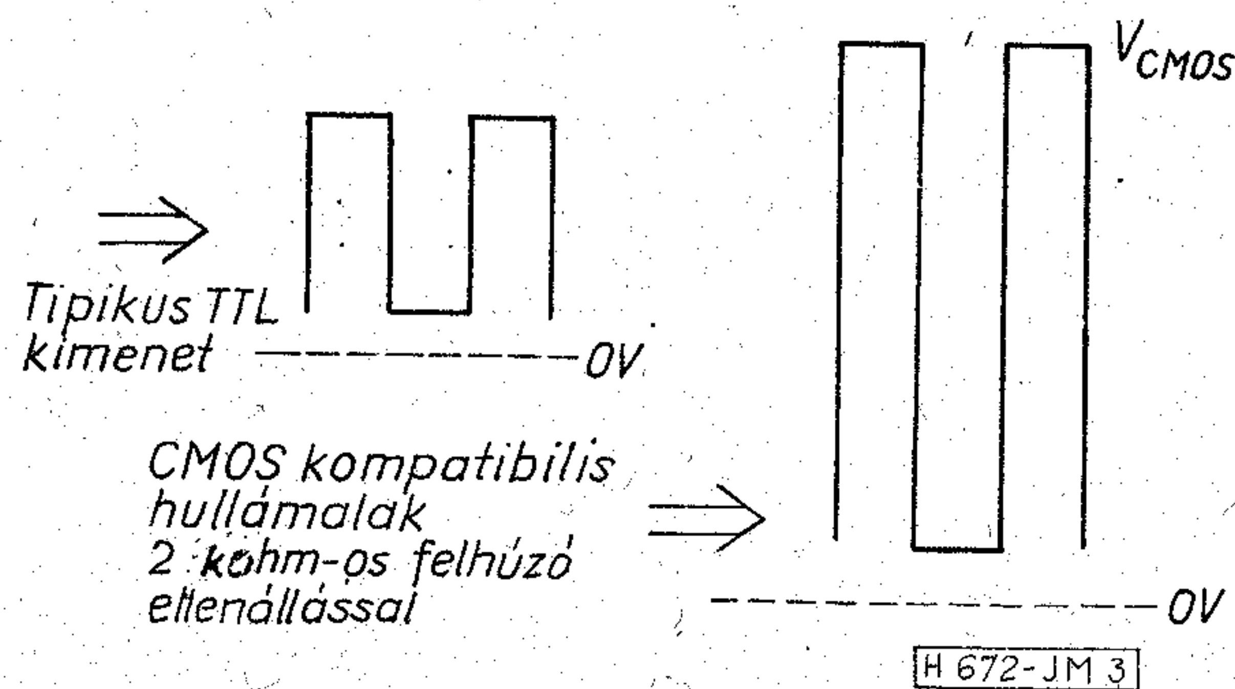
3. ábra. TTL/CMOS csatlakozó áramkör
