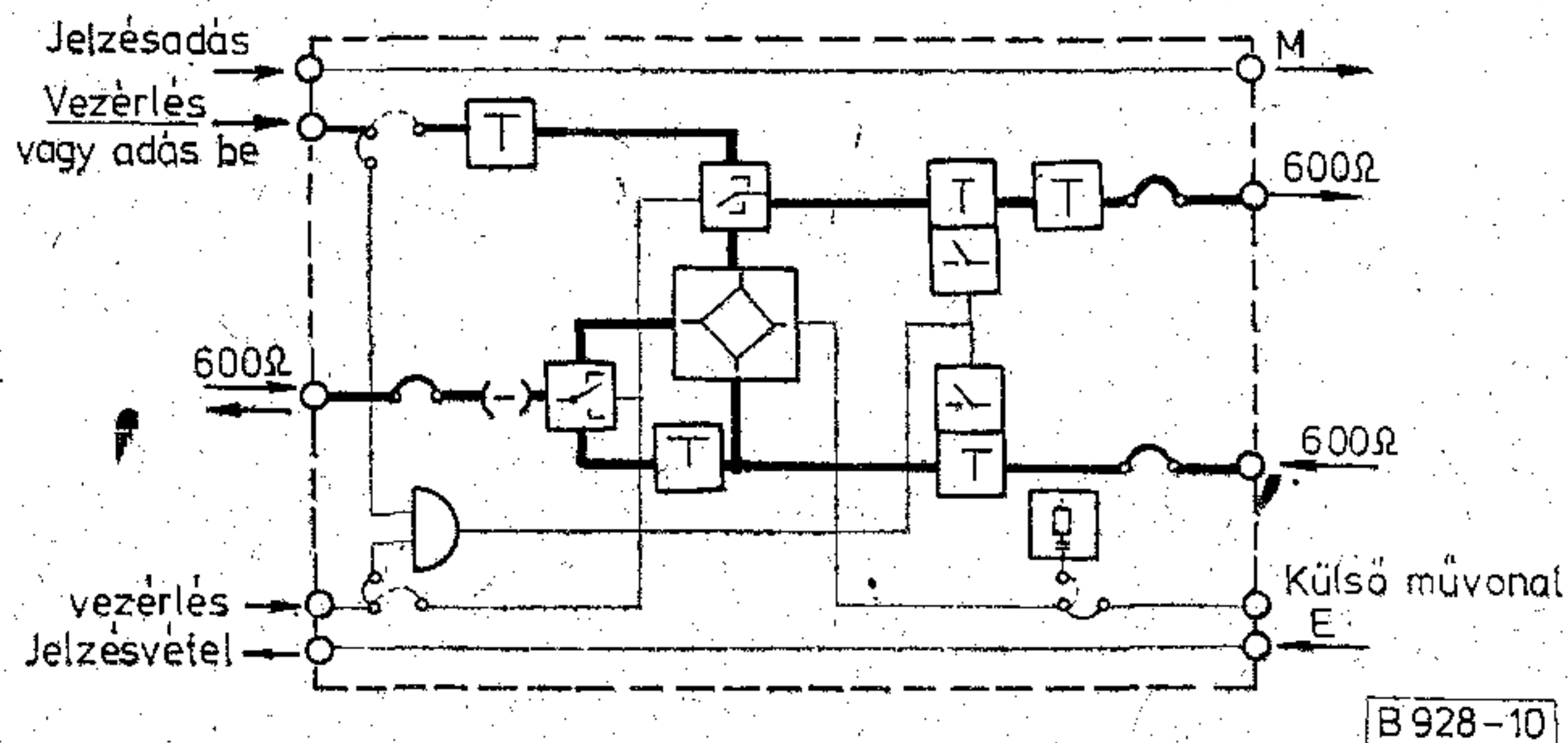
10. ábra. K típusú végződés bloksémája
