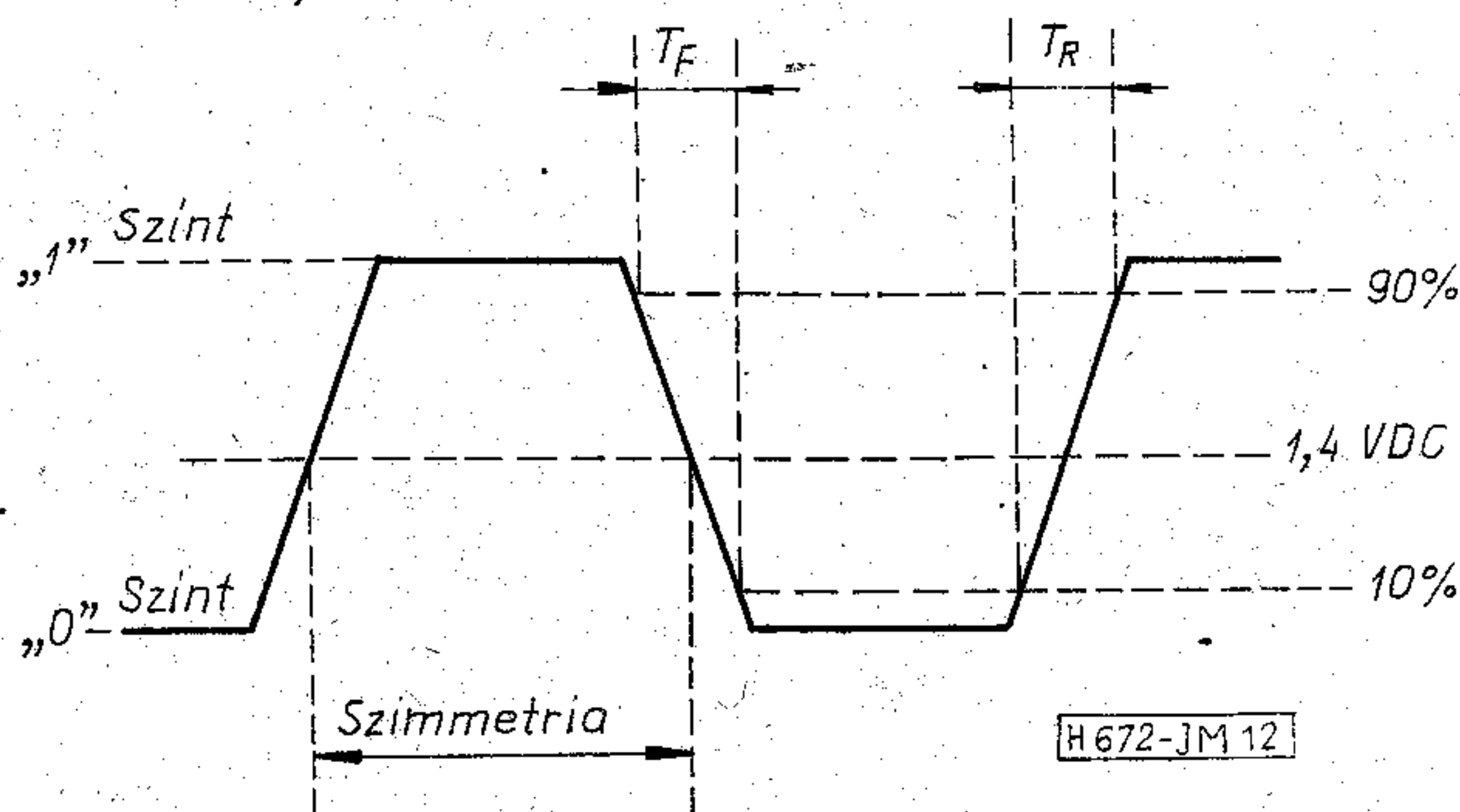
12. ábra. Hullámalak
