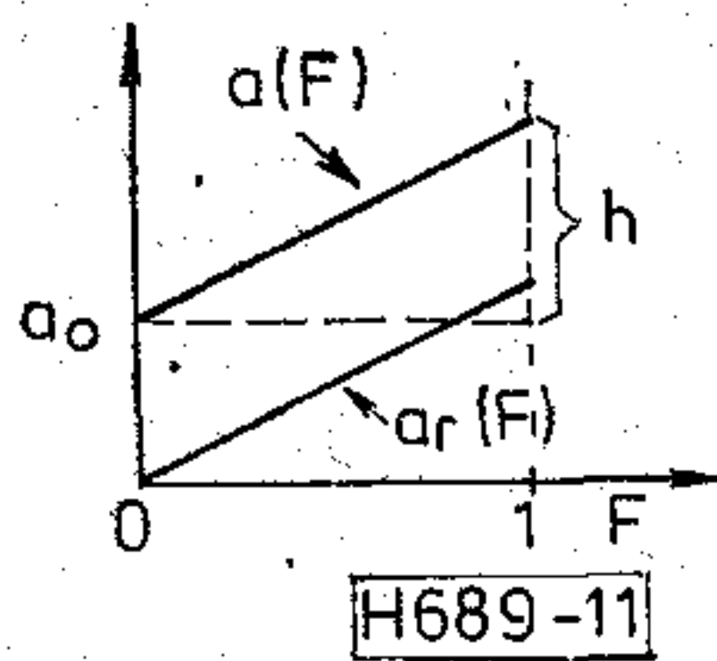
11. ábra. a(F) és a_r(F) lineáris preemfázis esetén
