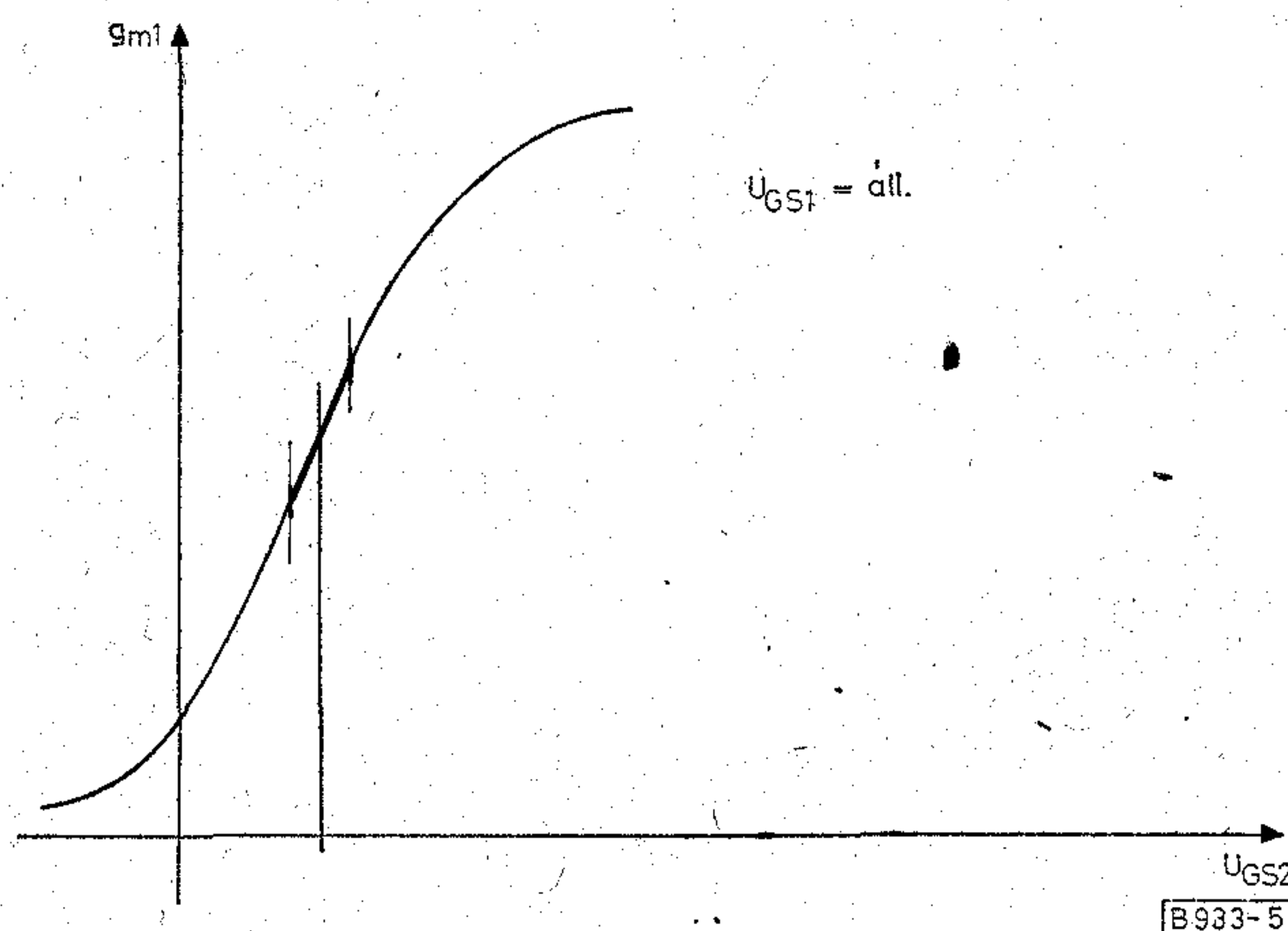
5. ábra. Dual-gate MOSFET g_{m1} = f(U_{GS2}) karakterisztikája
