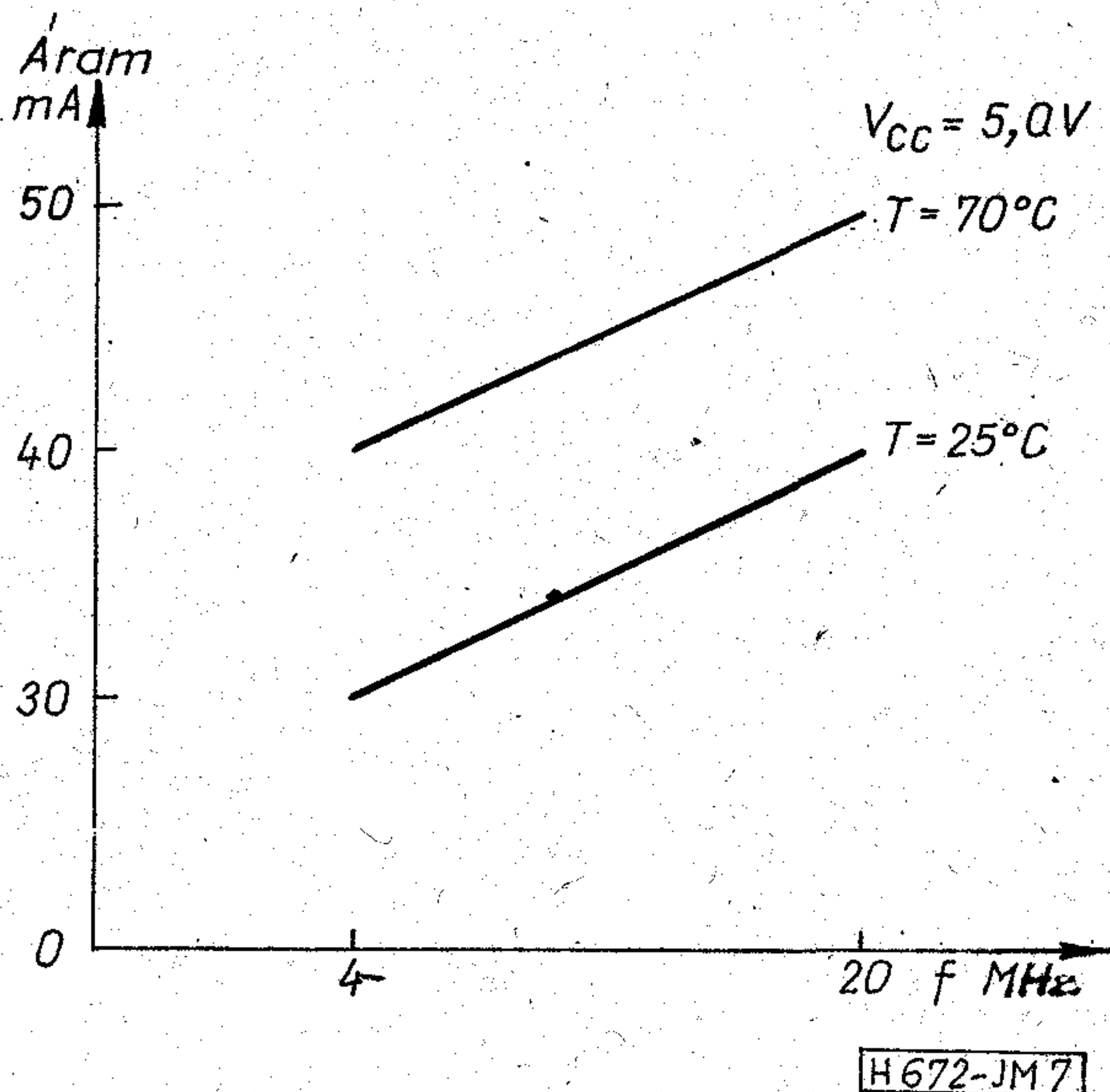
7. ábra. Tipikus áram—frekvencia összefüggés
