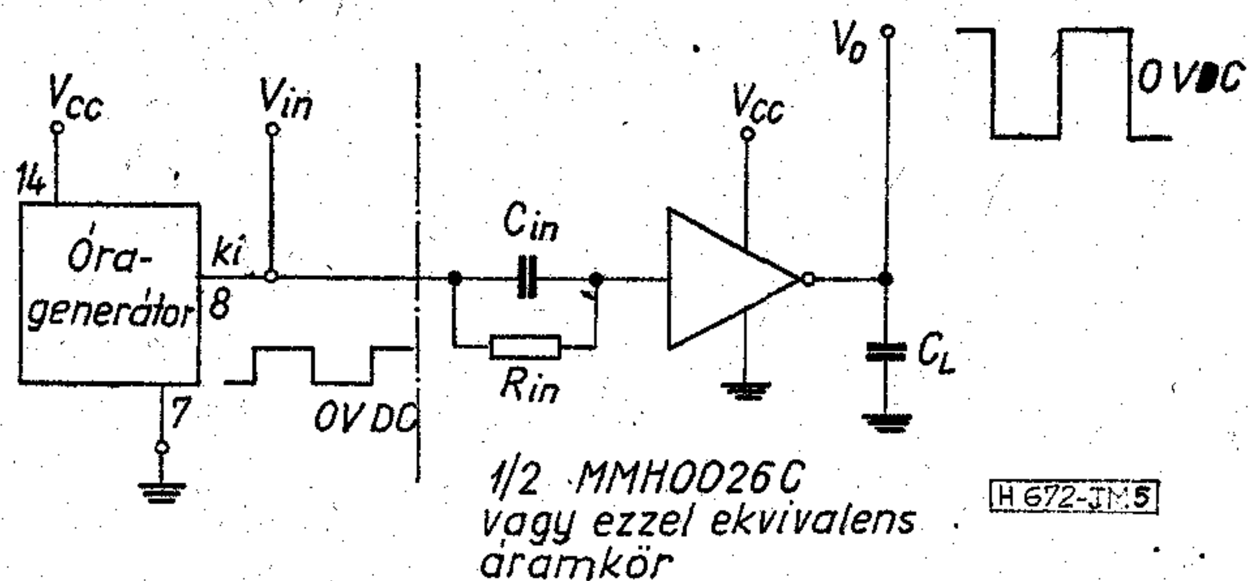
5. ábra. DC csatolású csatlakozó áramkör (egy tápfeszültséggel)
