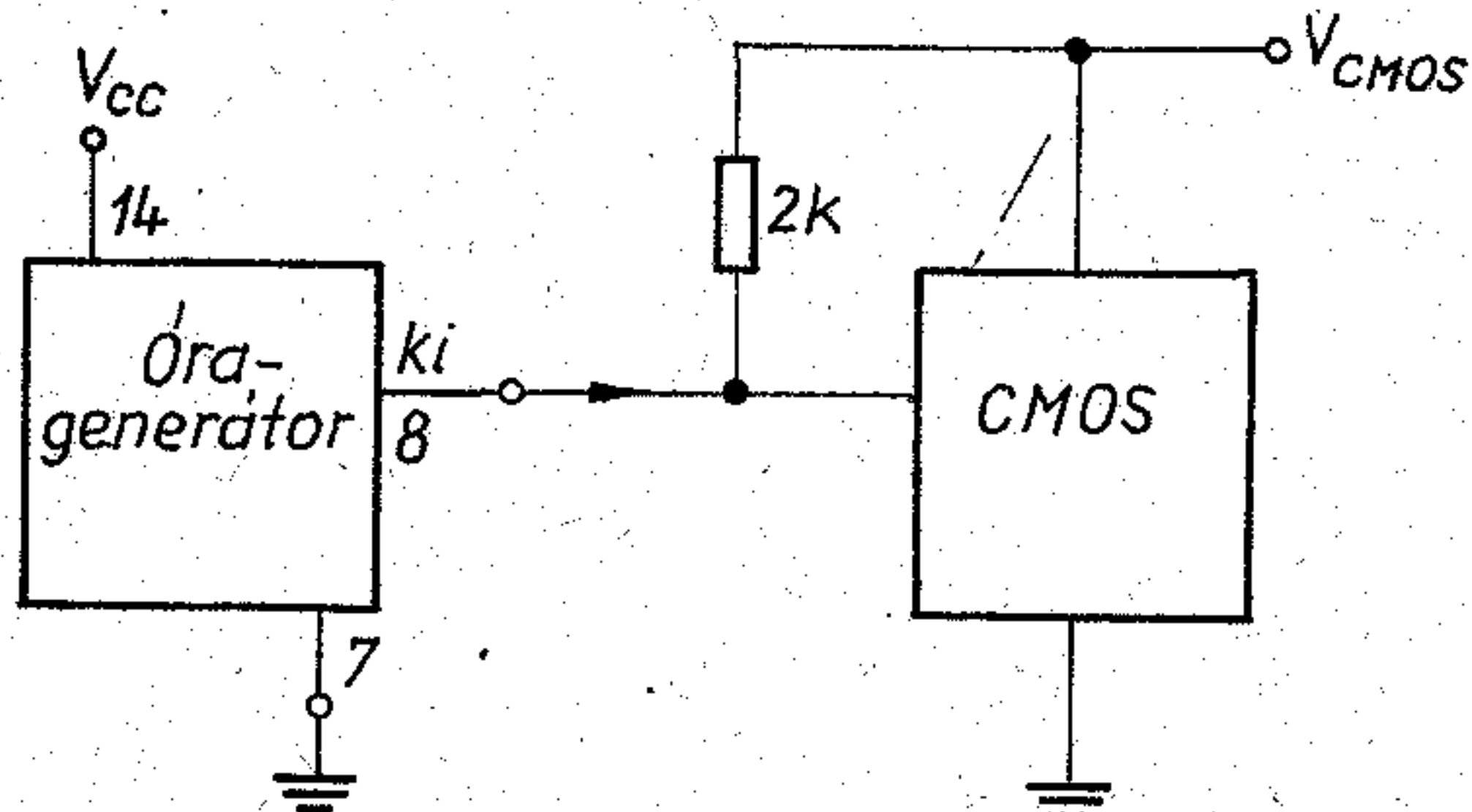
2. ábra. Terhelhetőség
