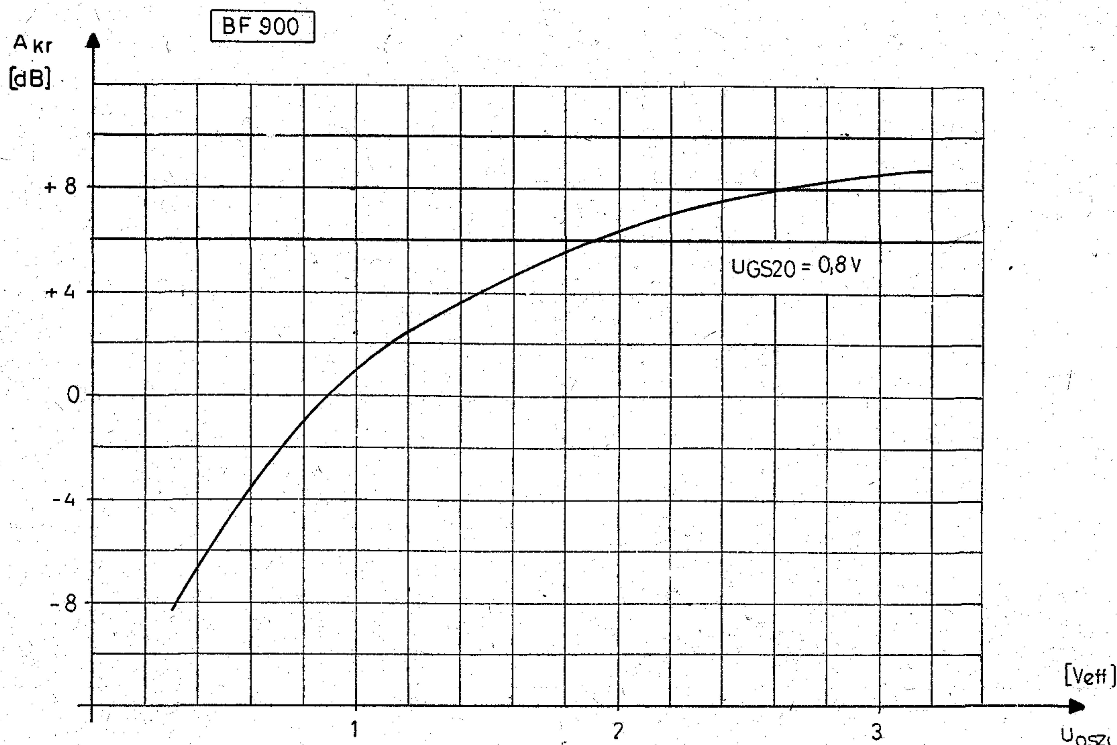
8. ábra. A relatív keverőerősítés az oszcillátorfeszültség függvényében
