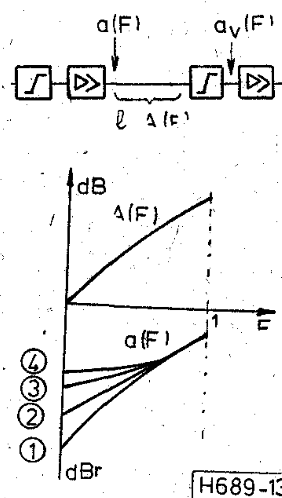
13. ábra. A kábelkarakterisztika és a lehetséges preemfázis-görbék
