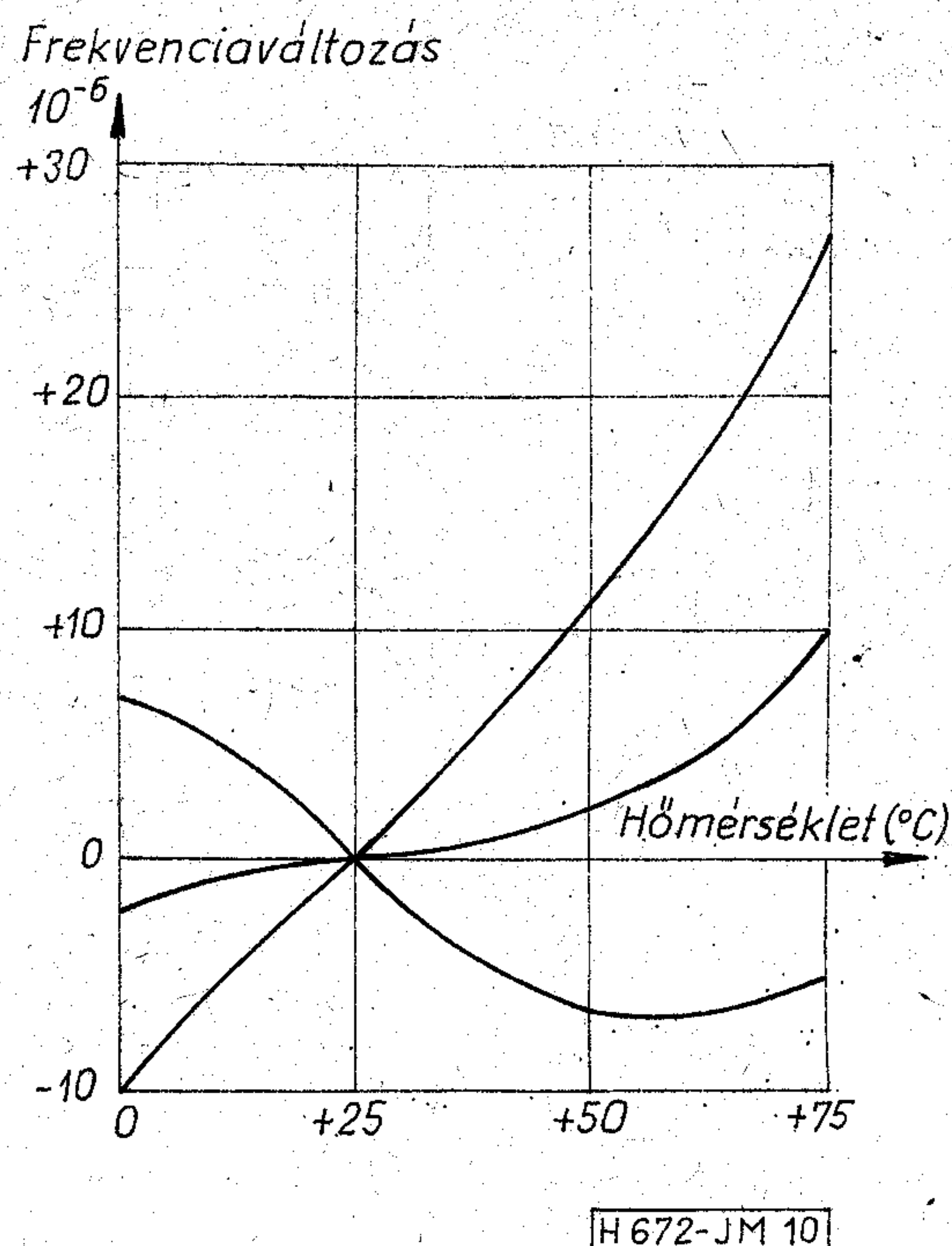
10. ábra. Tipikus hőmérséklet—frekvenciaváltozás karakterisztika
