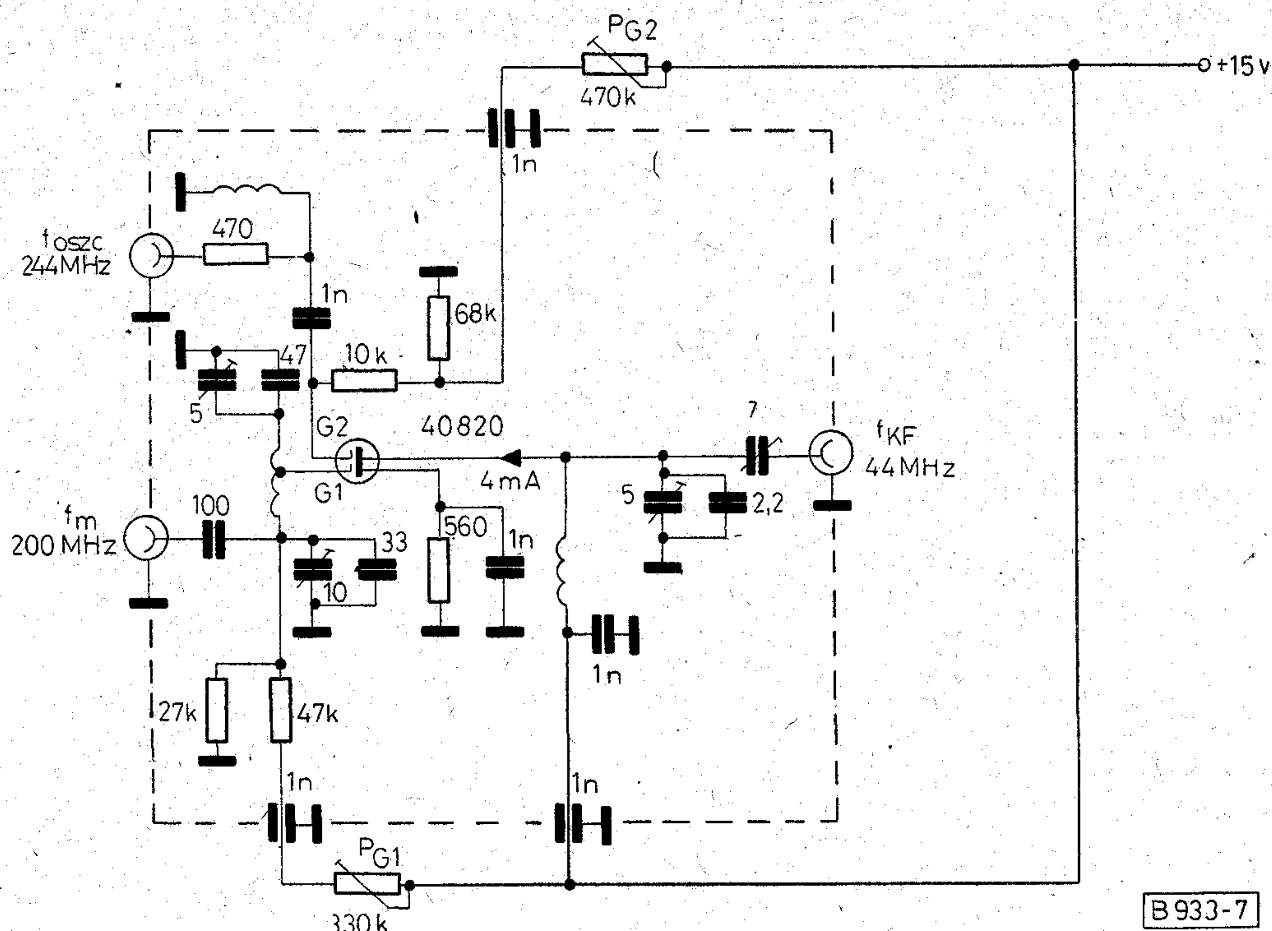
7. ábra. RCA mérőkapcsolás
