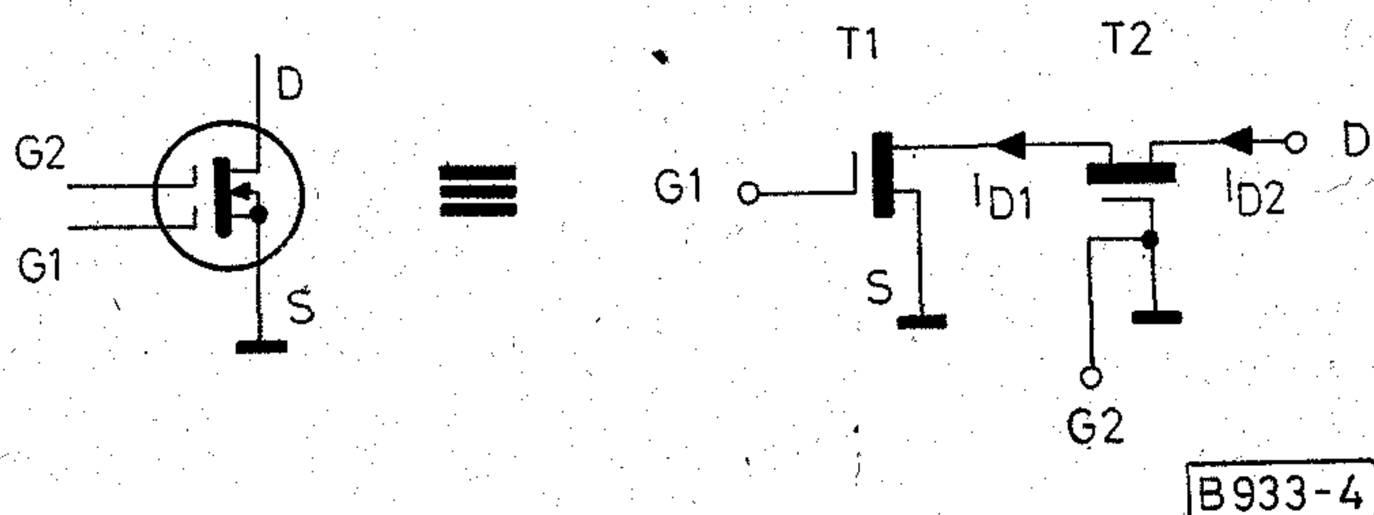
4. ábra. A dual-gate MOSFET elvi rajza
