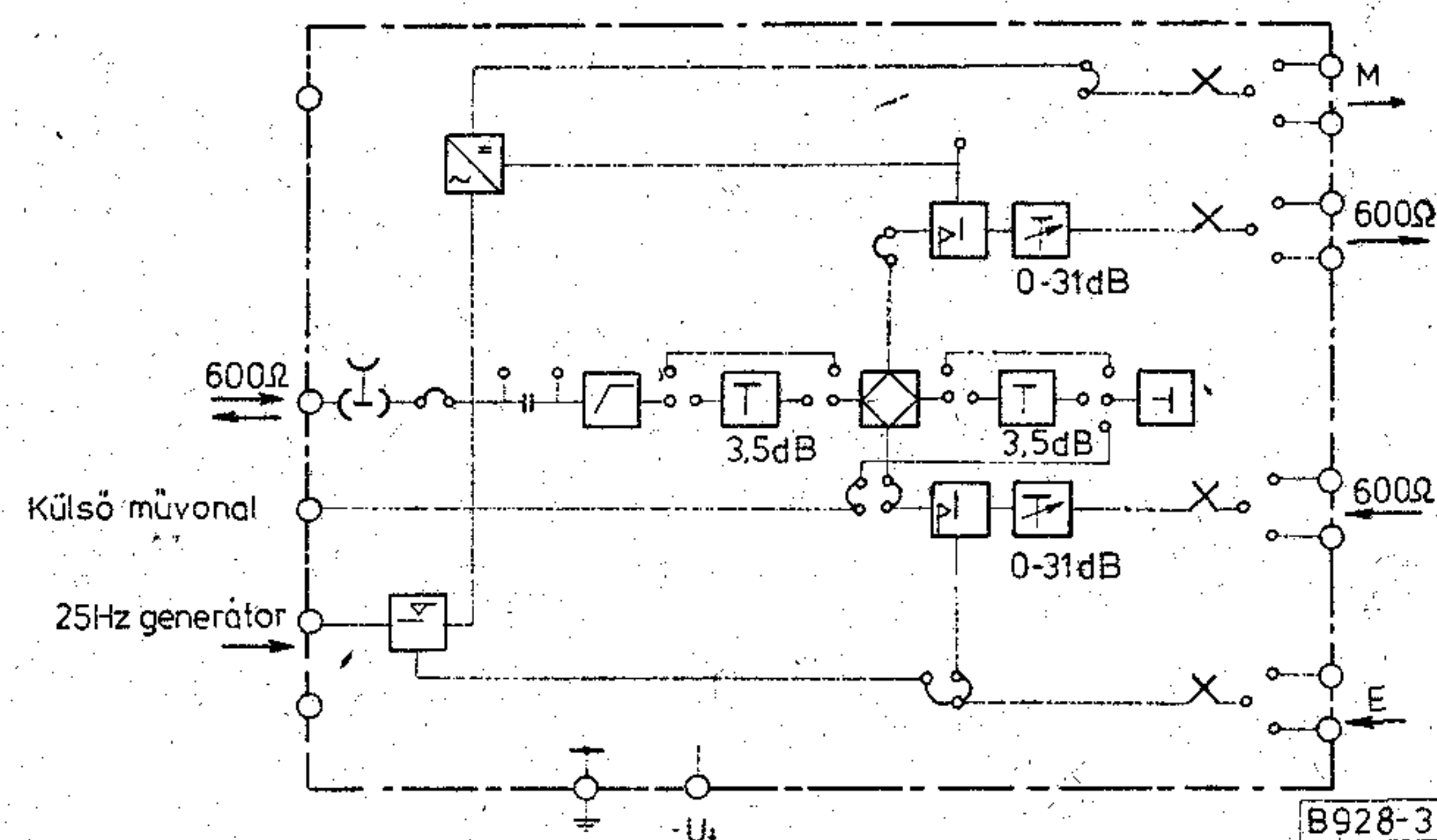
3. ábra. Az 1. üzemmód blokksémája
