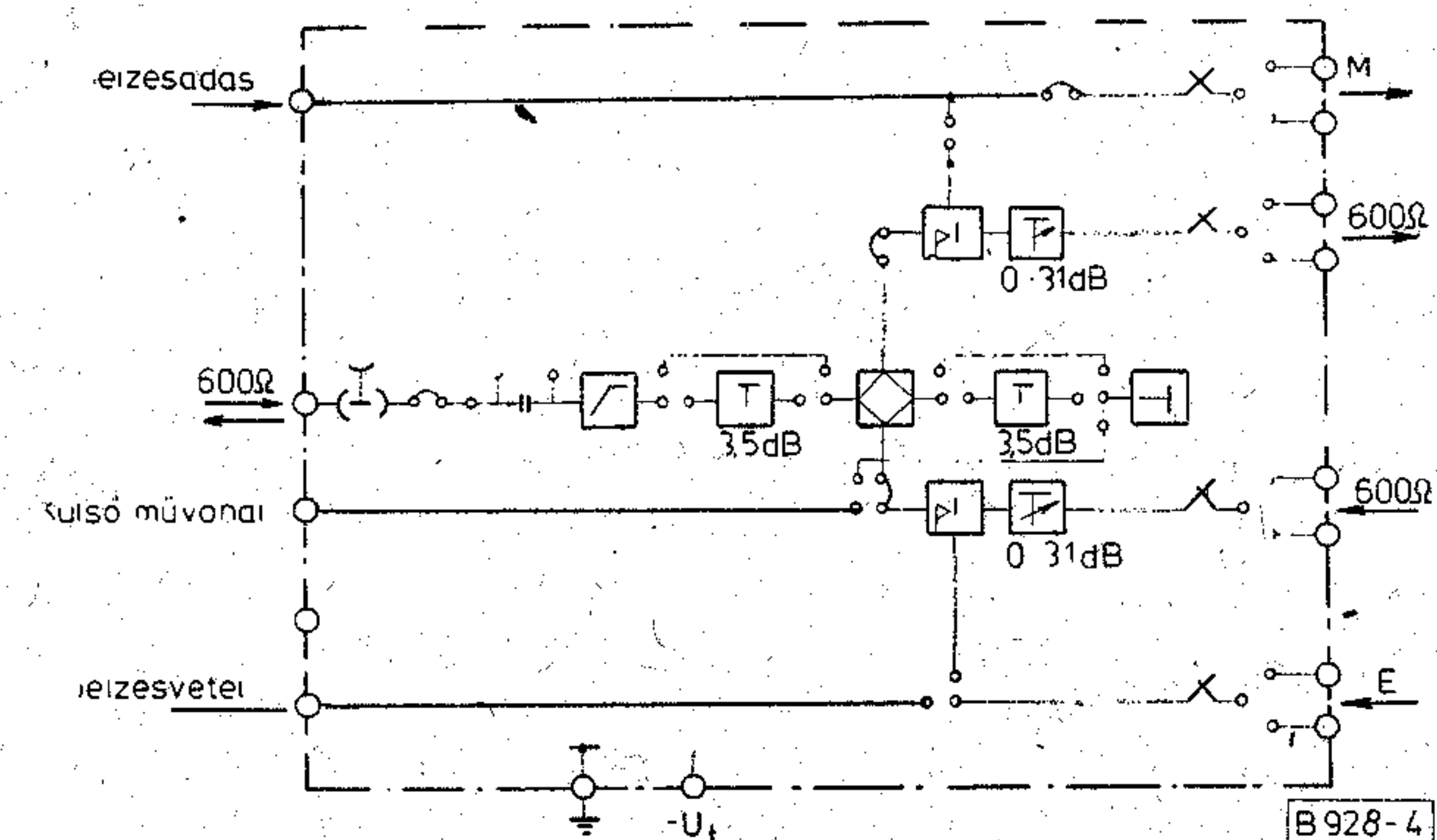
4. ábra. A 2. üzemmód blokksémája
