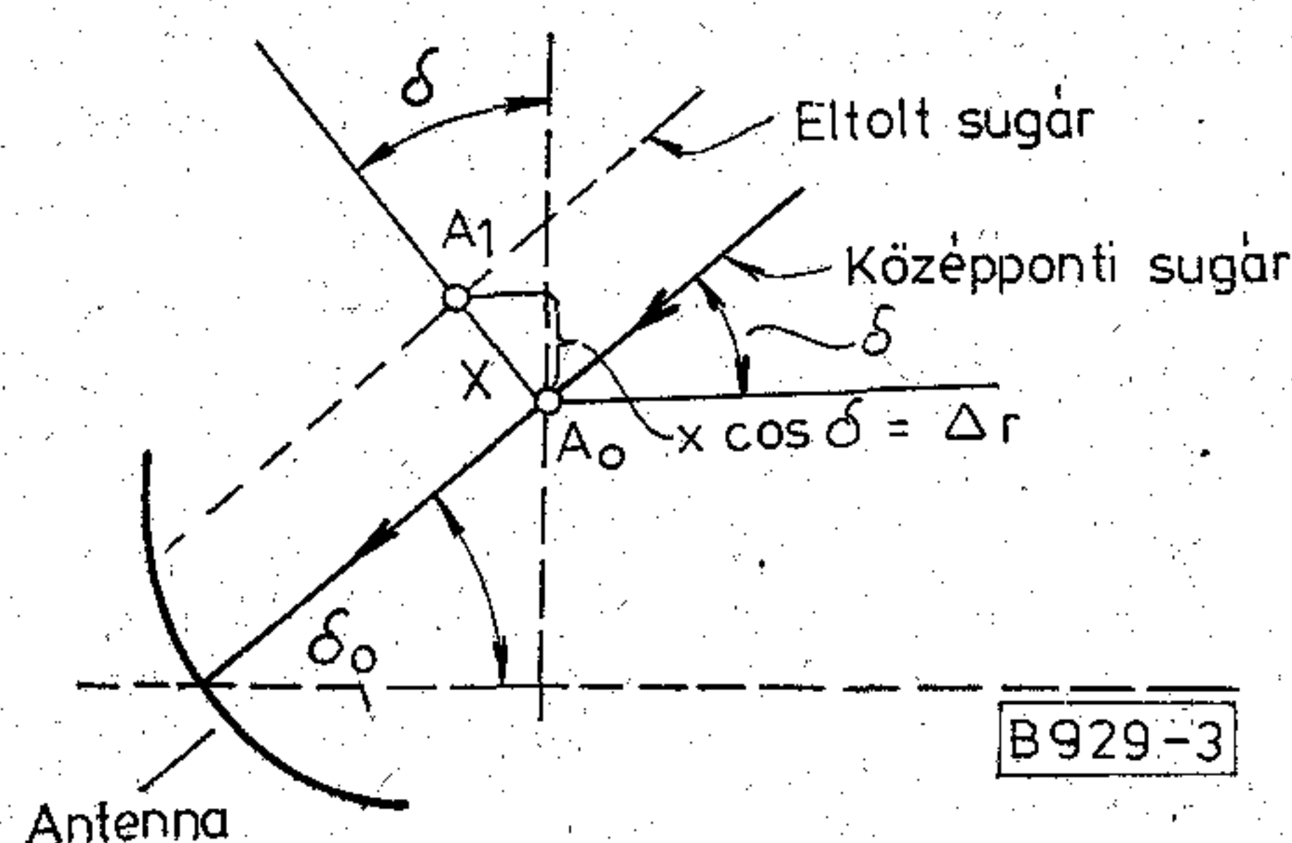
3. ábra. Szcintilláció
