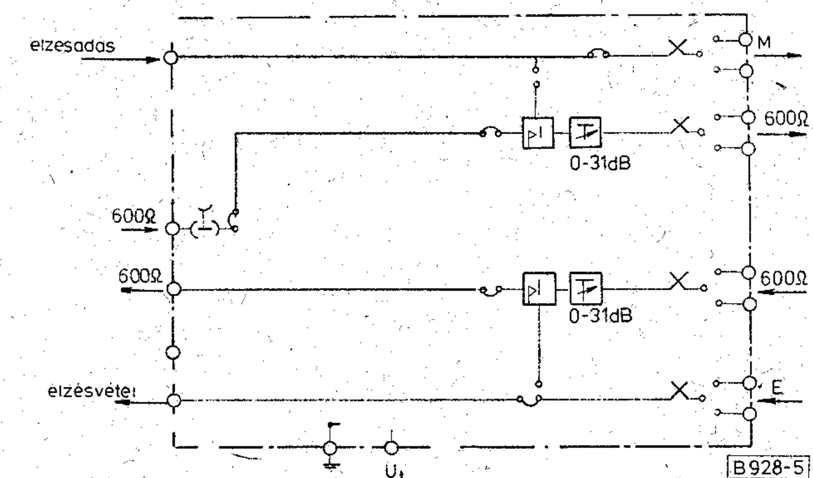
5. ábra. A 3. üzemmód blokksémája
