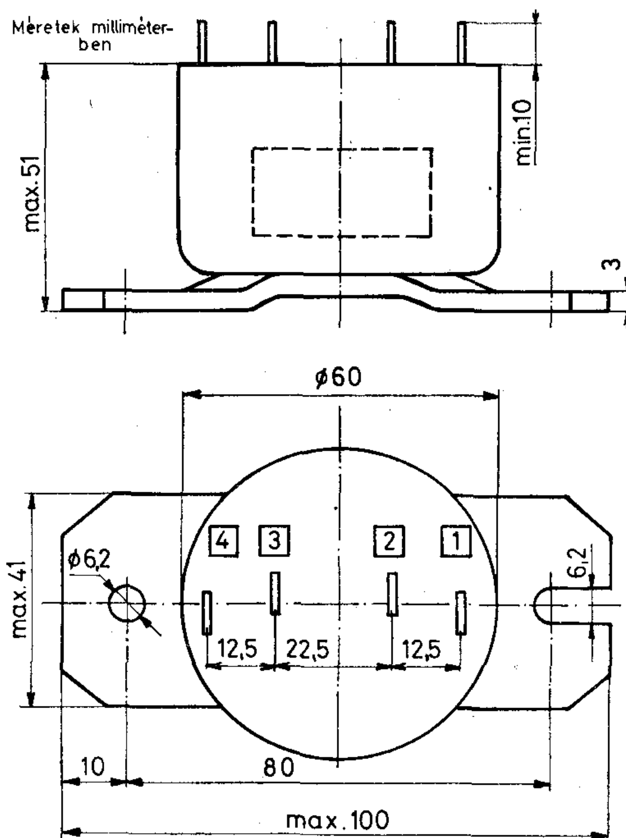
3. ábra. A tokozott egység körvonalrajza
