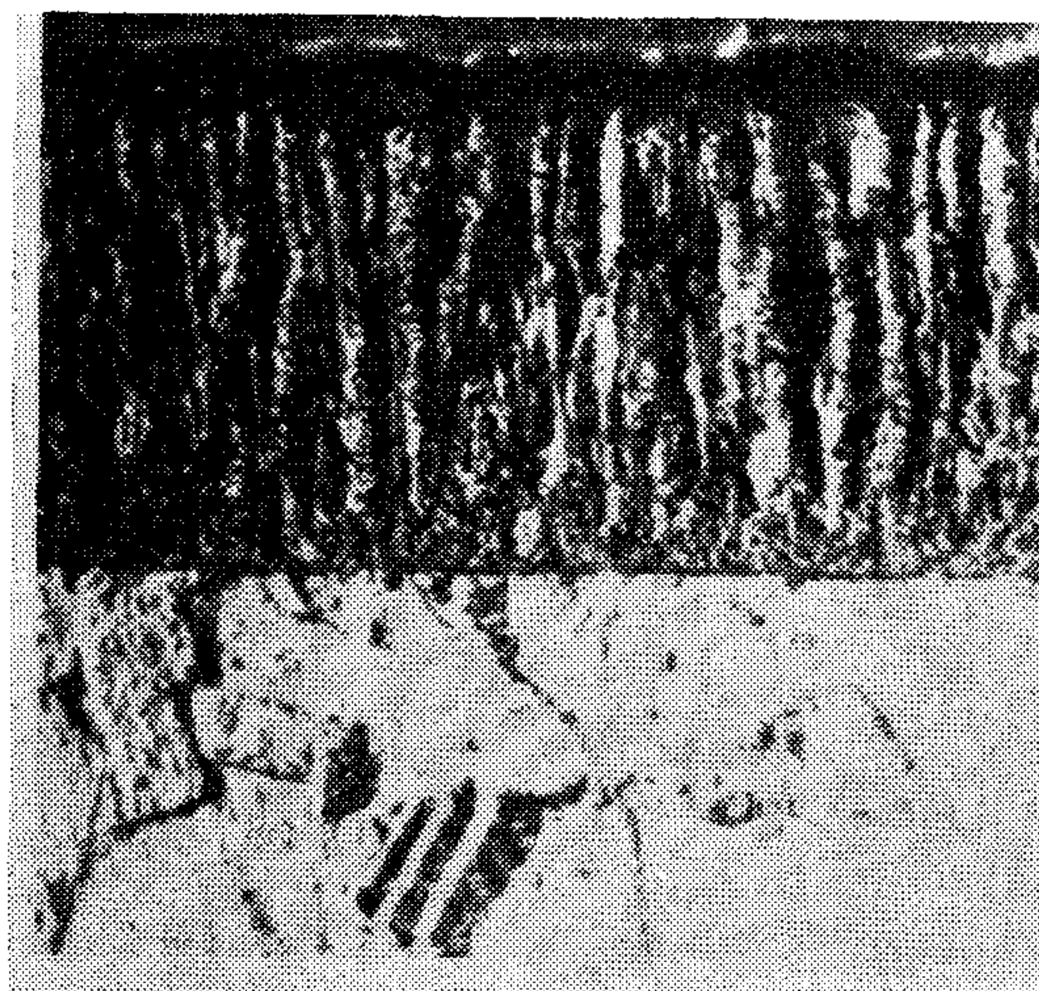
18. ábra. Nitrátos elektrolitból 3 A/dm 2 áramsűrűséggel leválasztott bevonat keresztmetszeti képe
