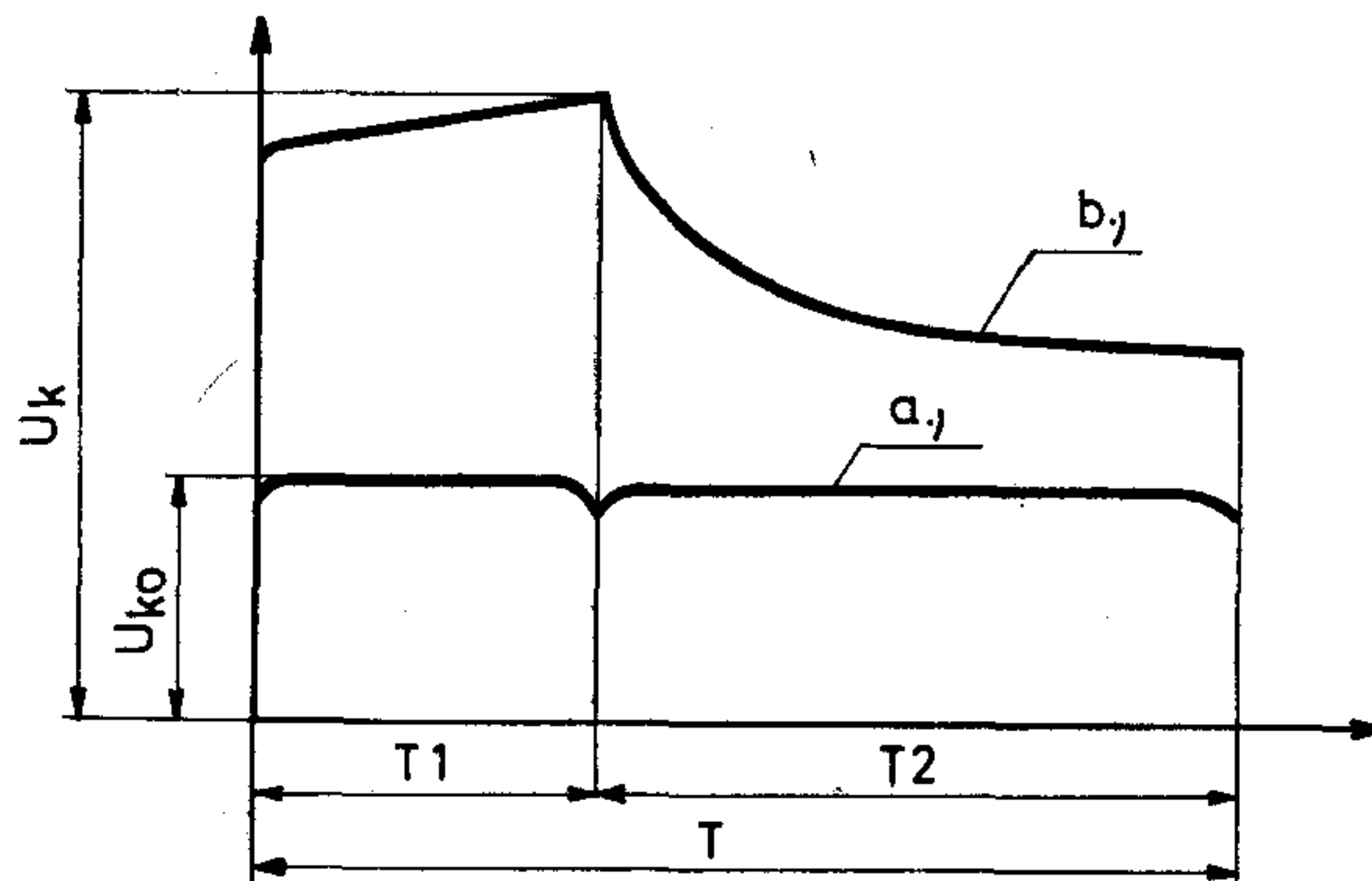
2. ábra. A kimenő feszültség idődiagramja:
