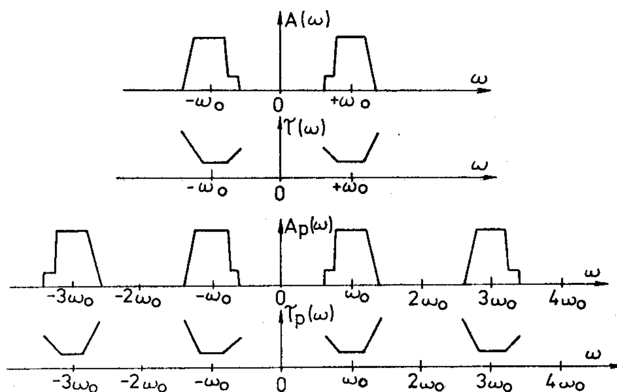
3. ábra. Az átviteli karakterisztika periodikussá tétele
