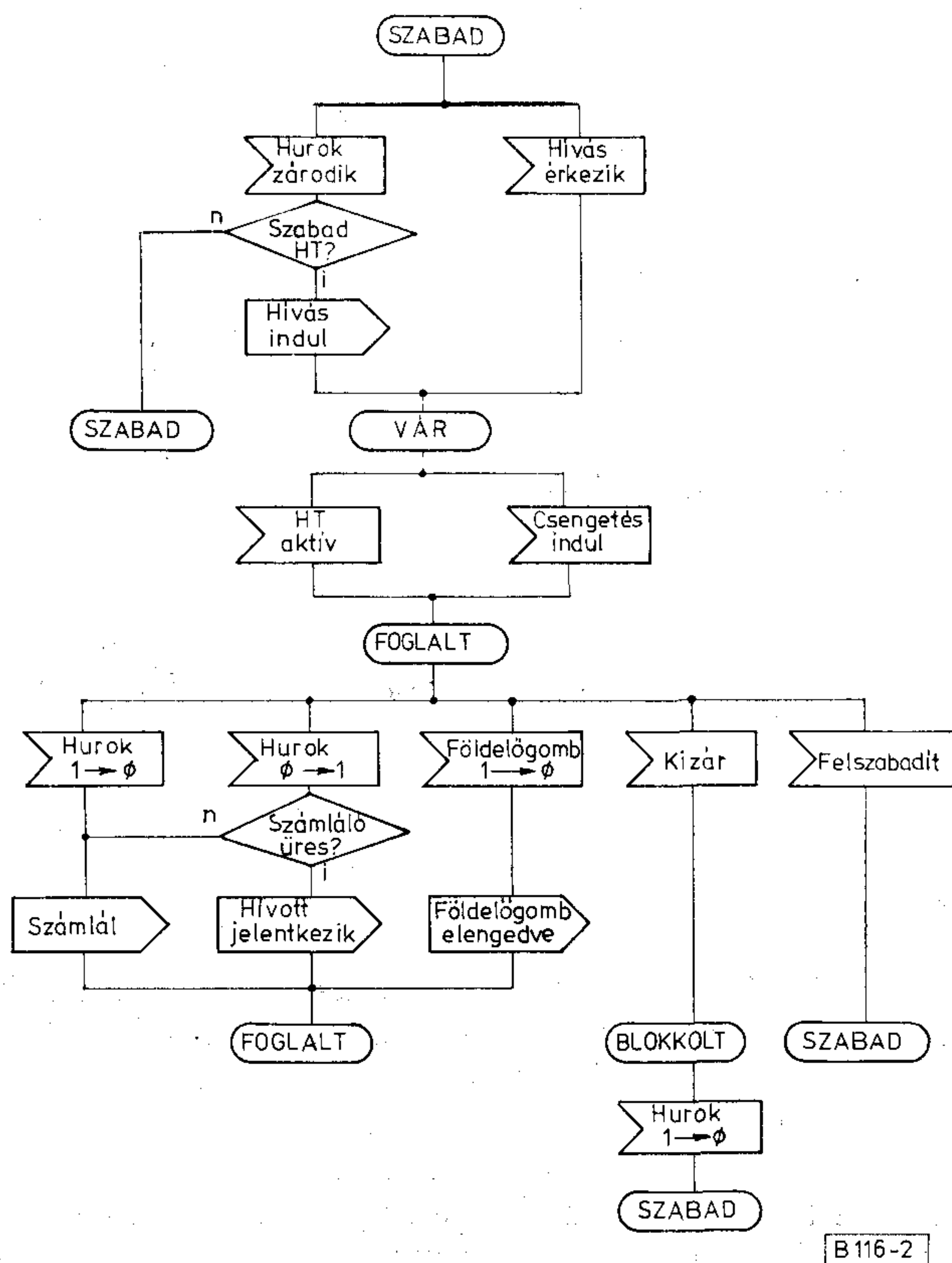
2. ábra. A „vonali” automata
