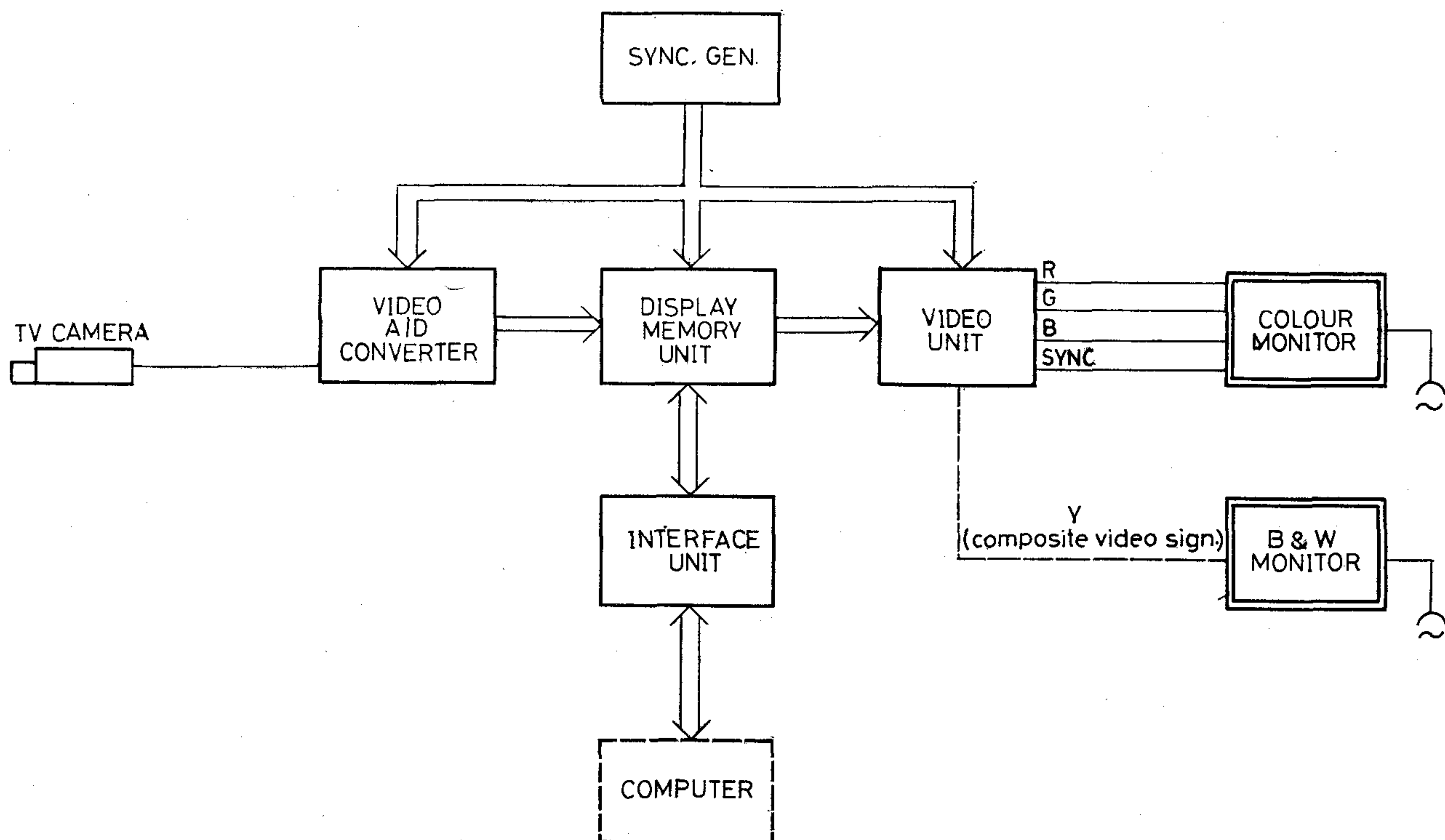
A színes grafikus display (HT 680X—CD) blokkvázlata
