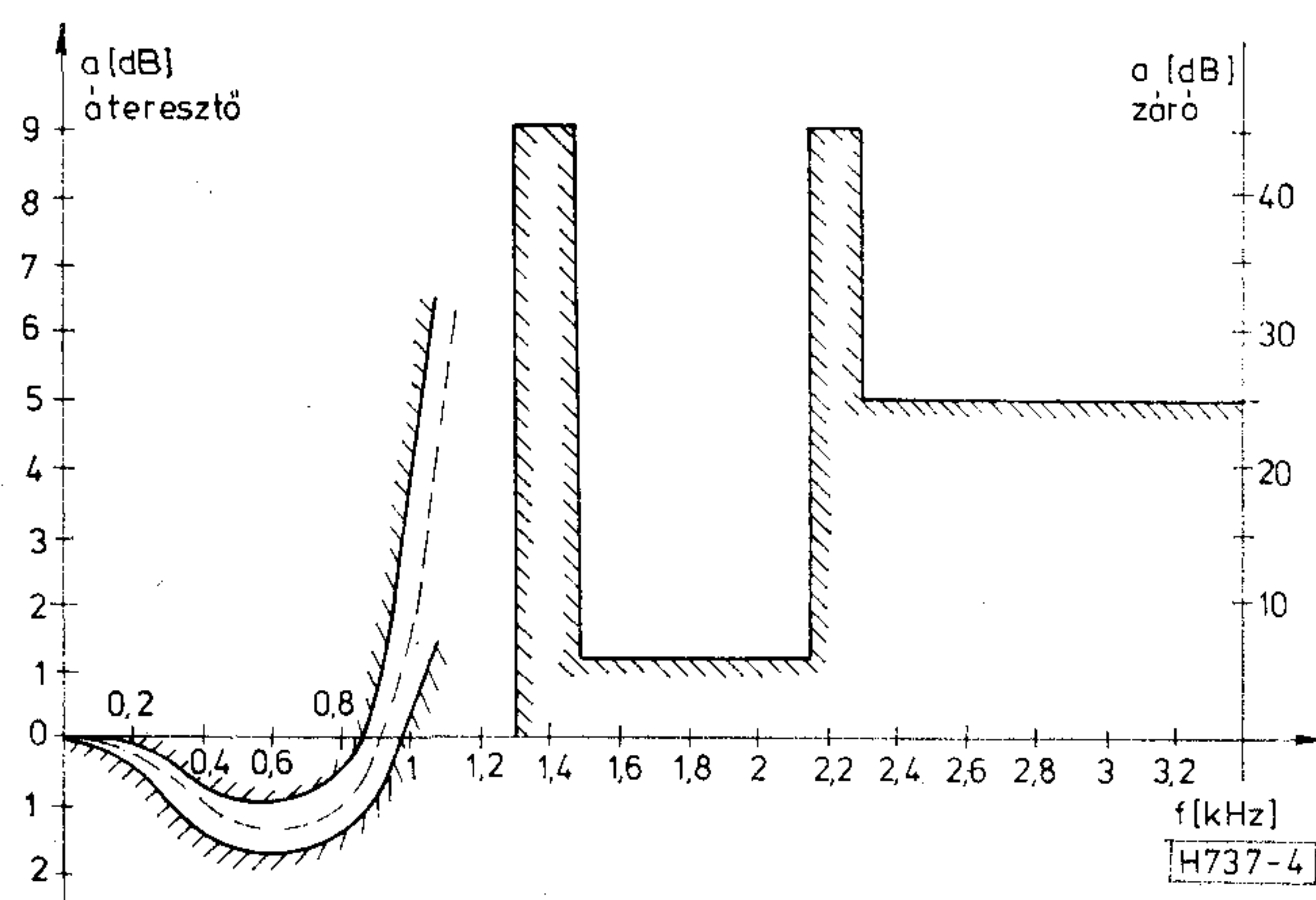
4. ábra. Adószűrő specifikáció 4800 b/s modemhez
