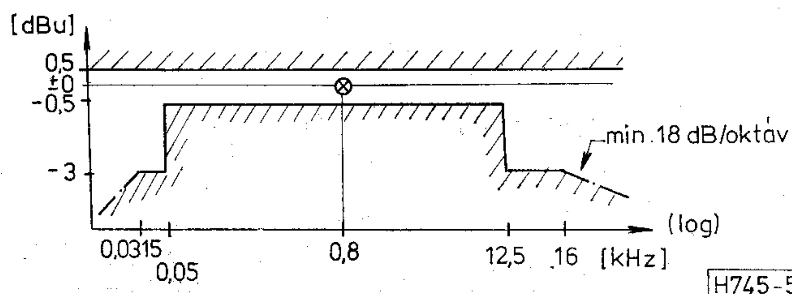
5. ábra. Szélessávú megengedett zajszint-változás a frekvencia függvényében
