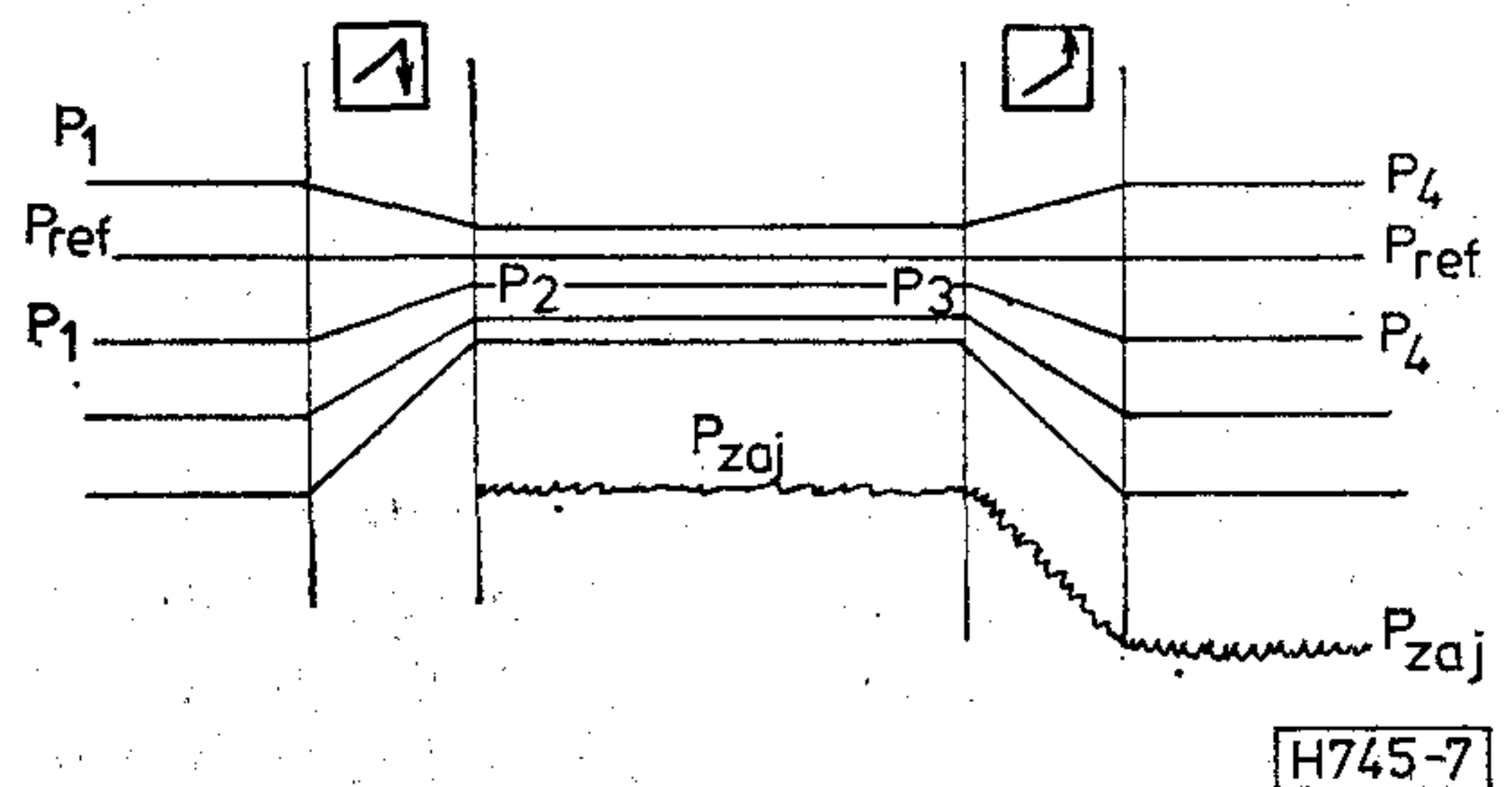
7. ábra. A kompander működési elve
