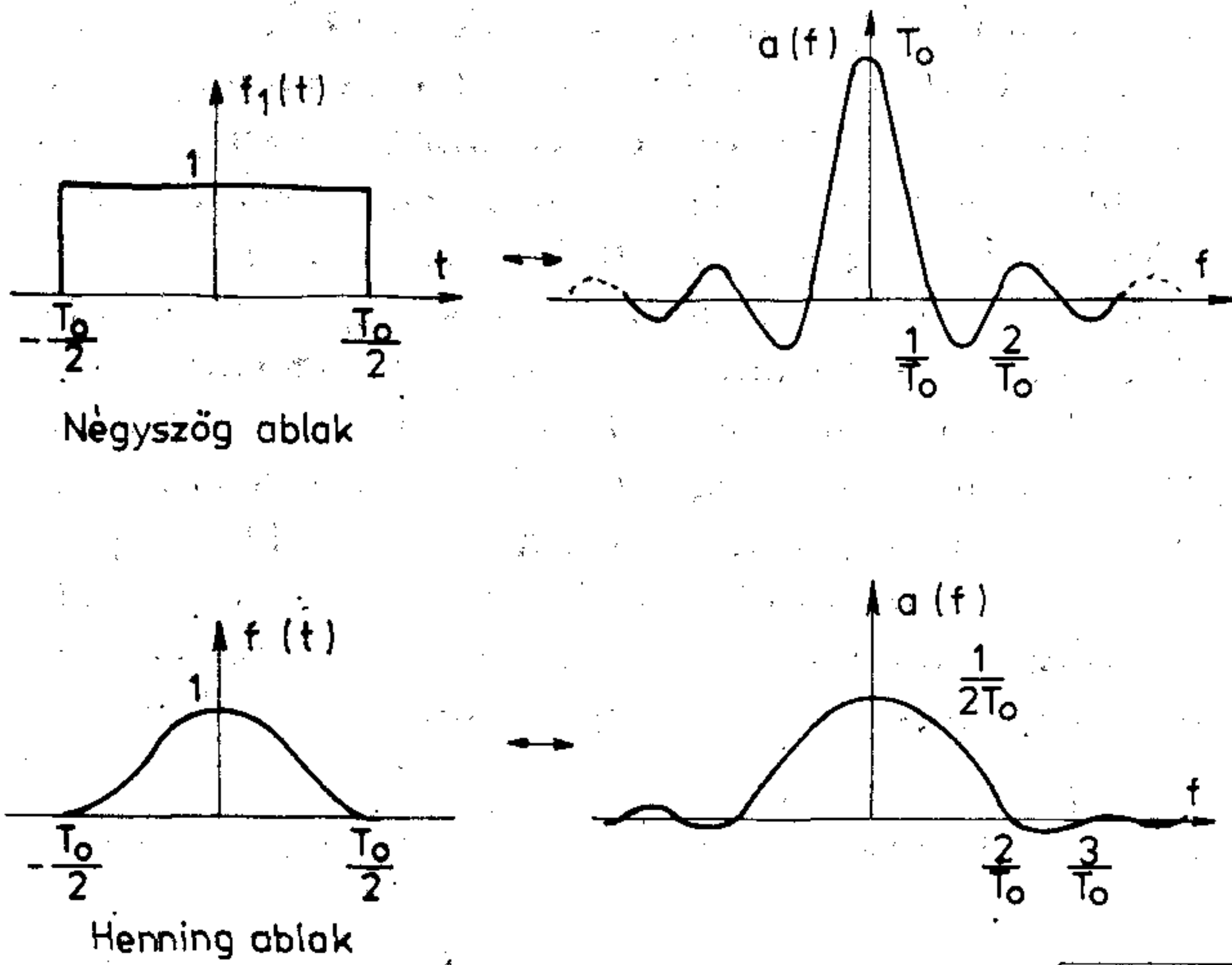
29. ábra. A négyszög és a Hanning ablak és a Fourier-transzformáltjuk
