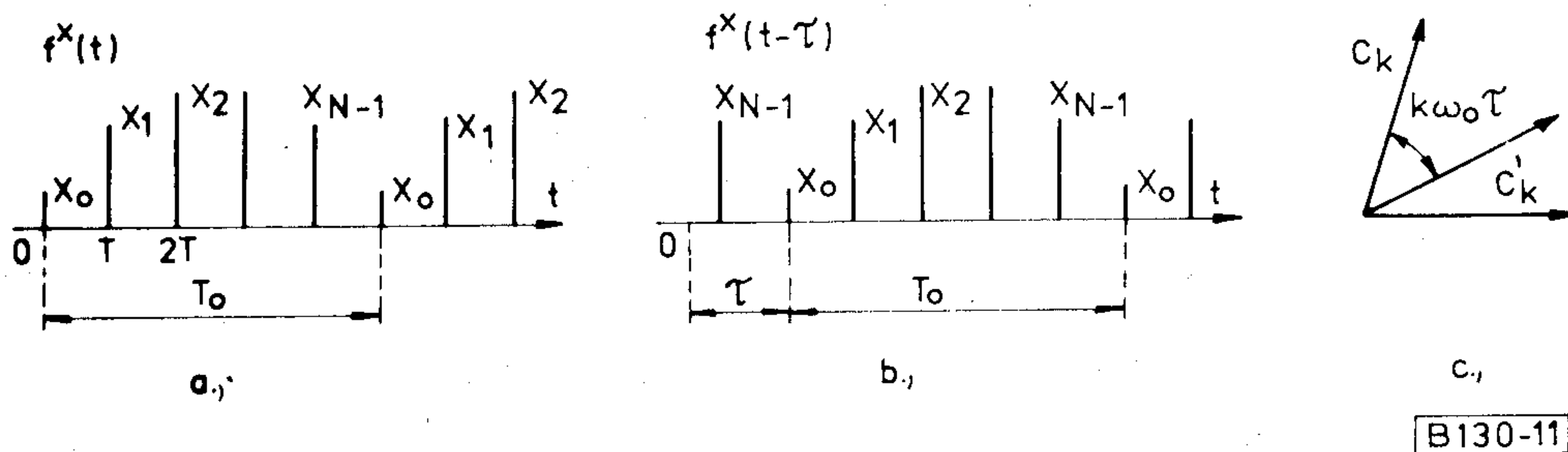
11. ábra. f^*(t) eltolása \tau idővel
