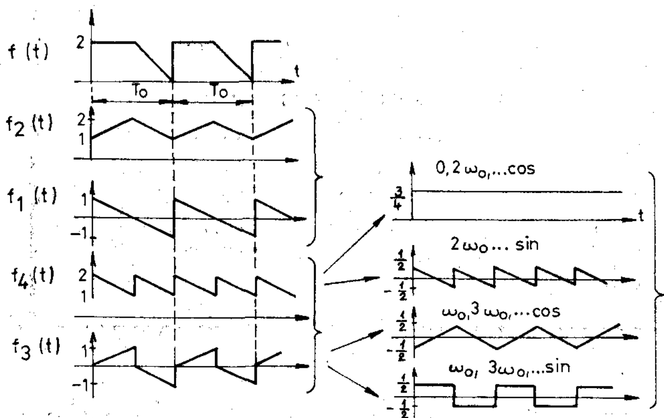
2. ábra. Periodikus függvény felbontása
