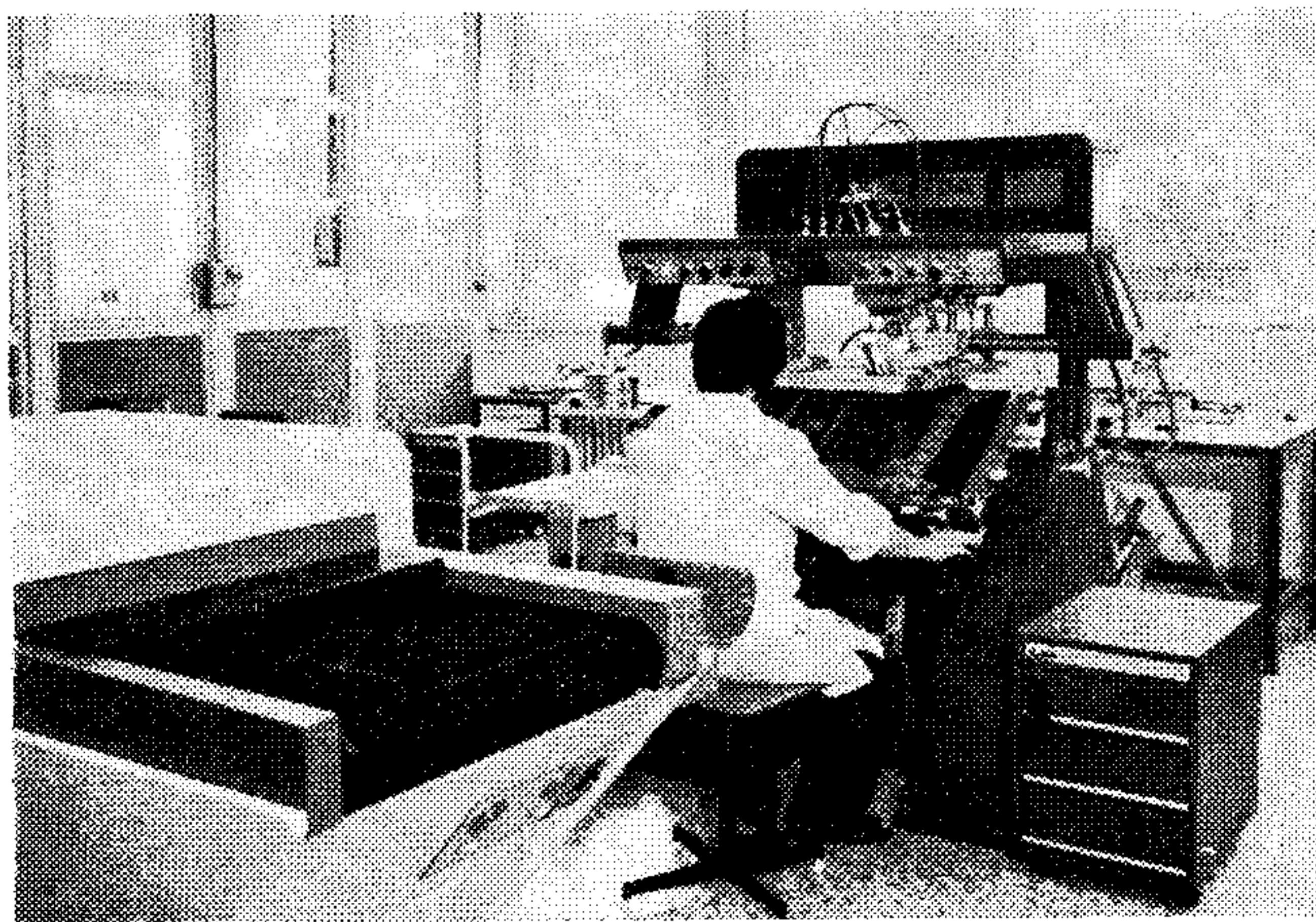
Az előtérben látható a szitafesték-száritó készülék, amely a háttérben elhelyezkedő szitanyomó gépen készülő nyomtatott huzalozású lapokra (3. ábra).
