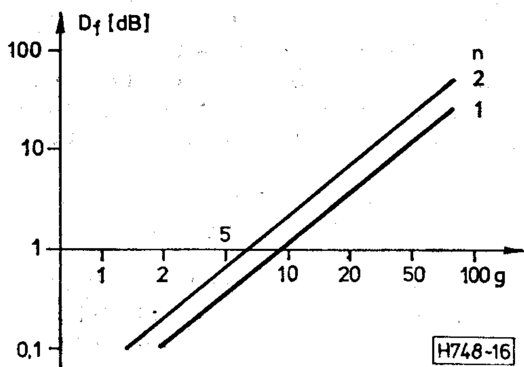
16. ábra. A dinamikatartomány felső határának csökkenése komplex póluspárú szűrő esetén
