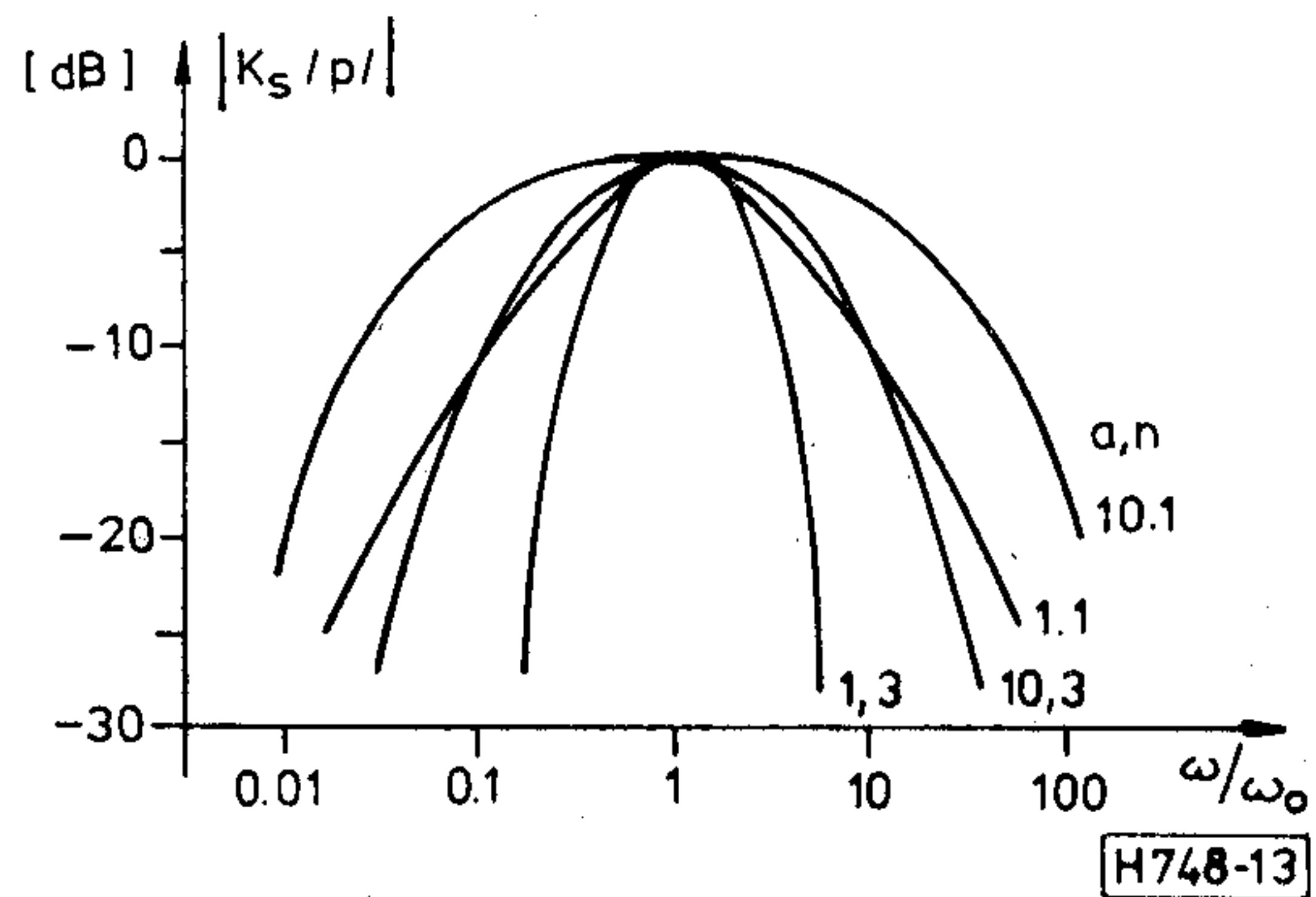
13. ábra. Valós póluspárral kialakított komparátorszűrők átviteli függvénye
