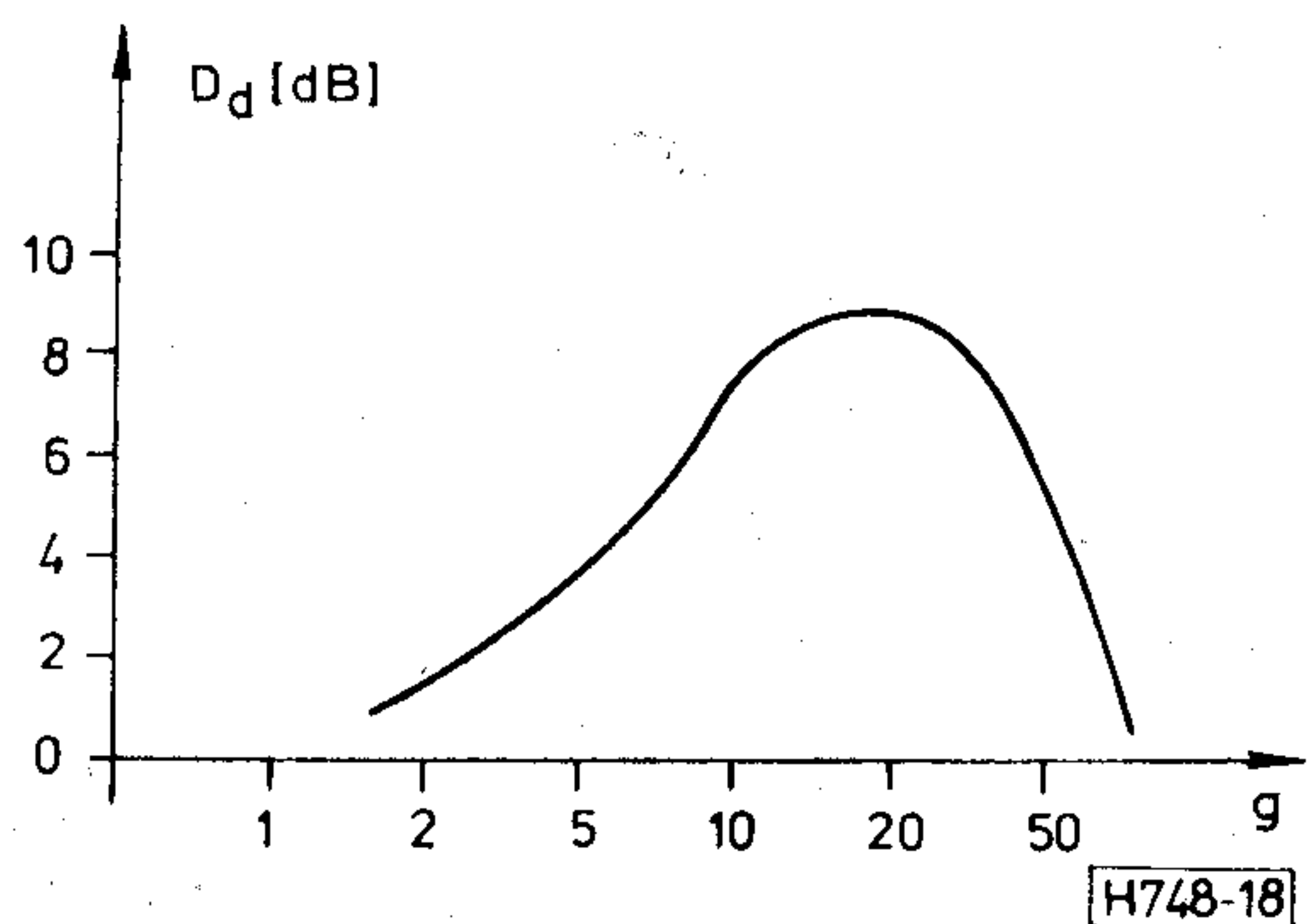
18. ábra. A dinamikatartomány eredő növekedése komplex póluspárok esetén
