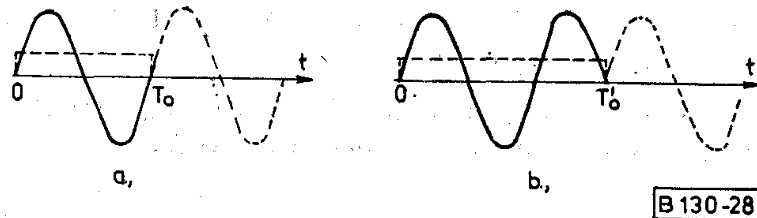
28. ábra. Szinuszos függvényre alkalmazott T_0 és T'_0 = 1,5 T_0 ablak
