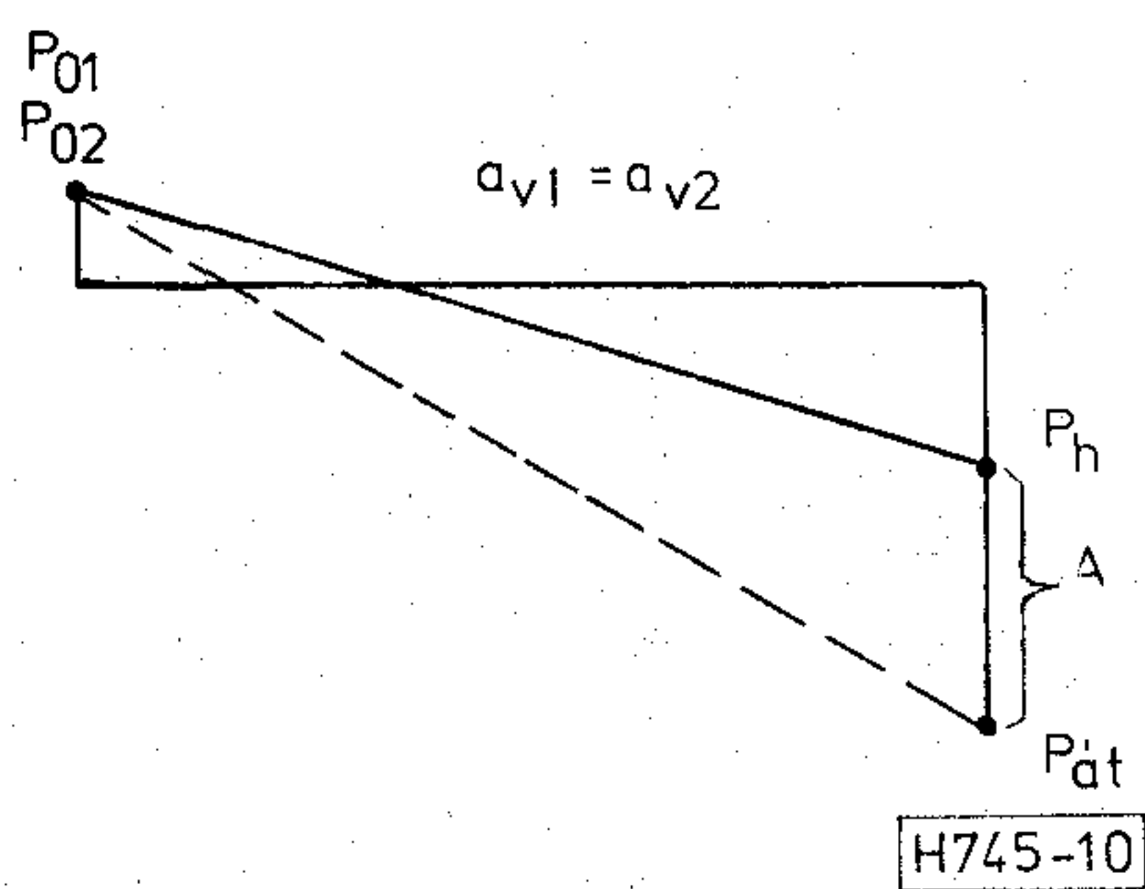
10. ábra. Az áthallási védettség fogalma
