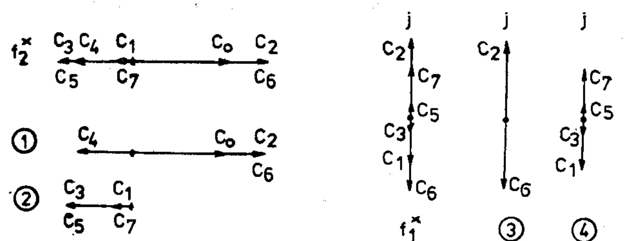
24. ábra. A 23. ábra szerinti impulzusfüggvény felbontása
