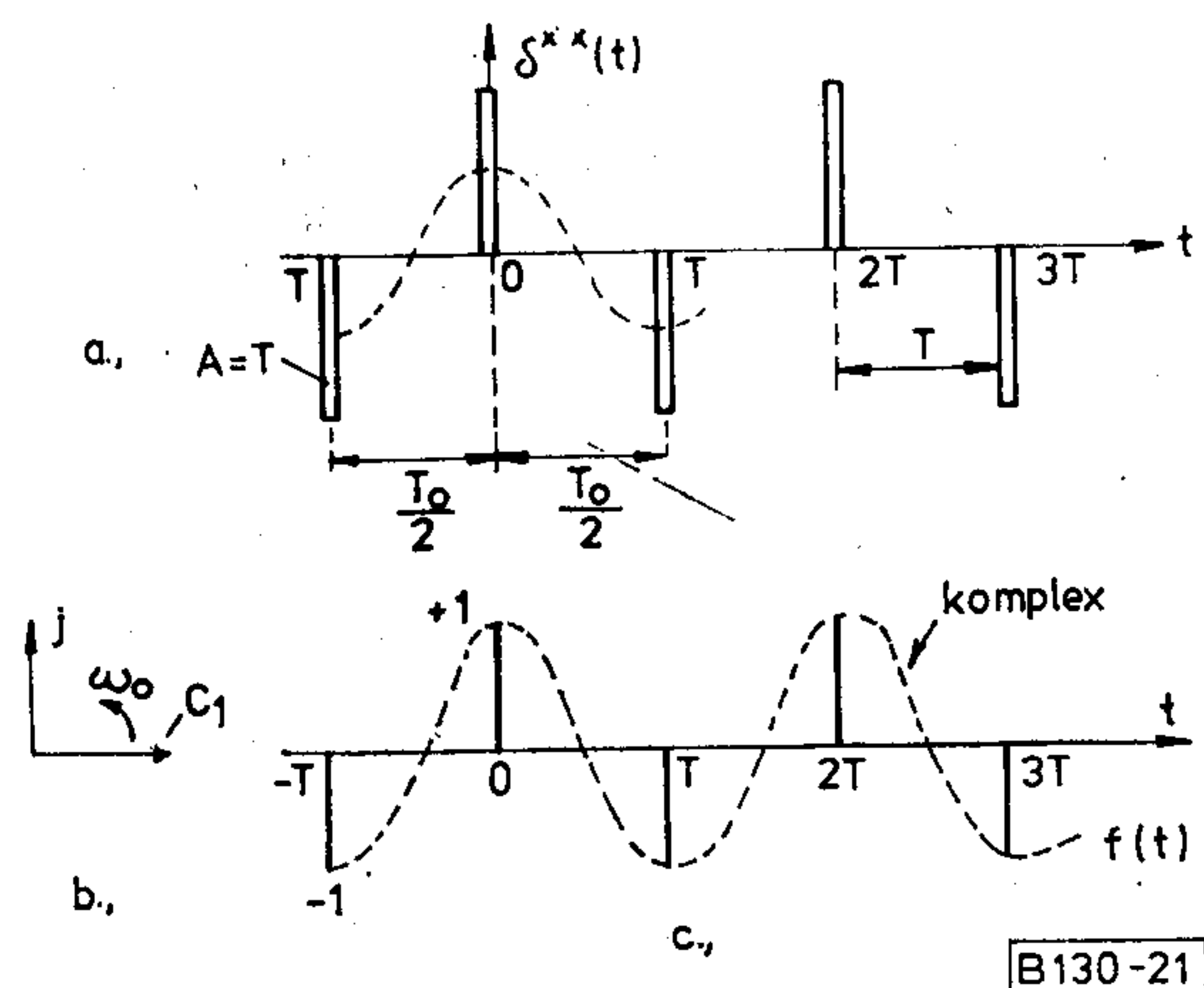
21. ábra. A váltott polaritású mintavételező függvény, \delta^{**}(t)
