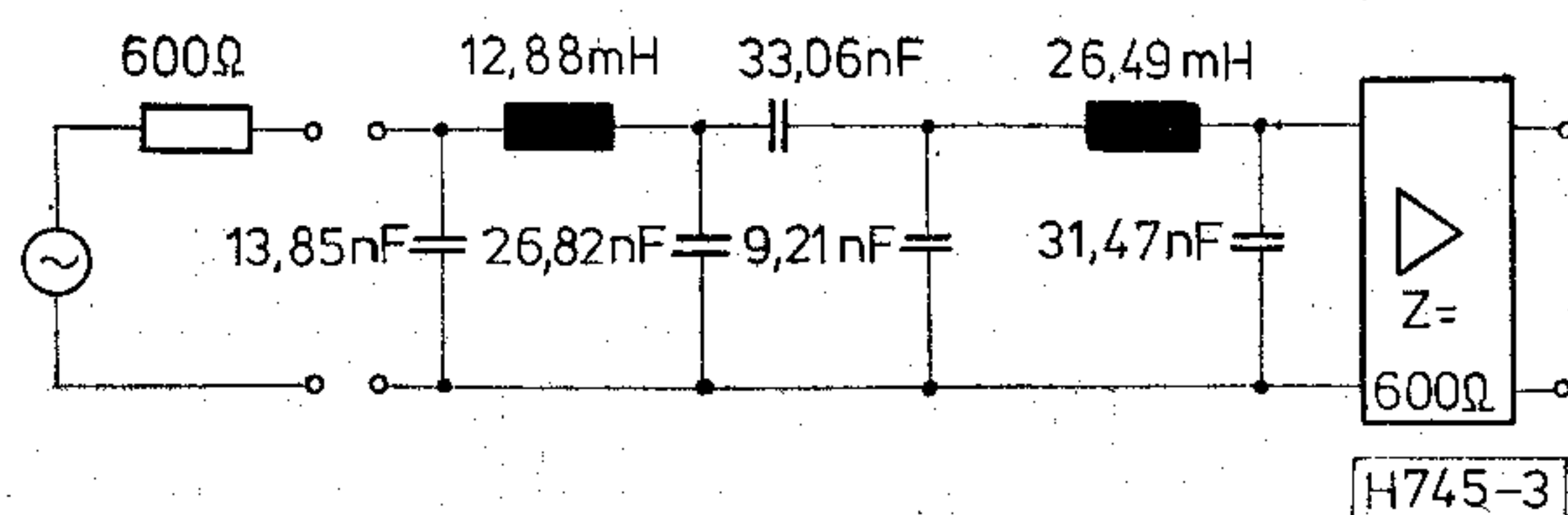
3. ábra. Elektromos négypólus a súlyozógörbe meghatározásához
