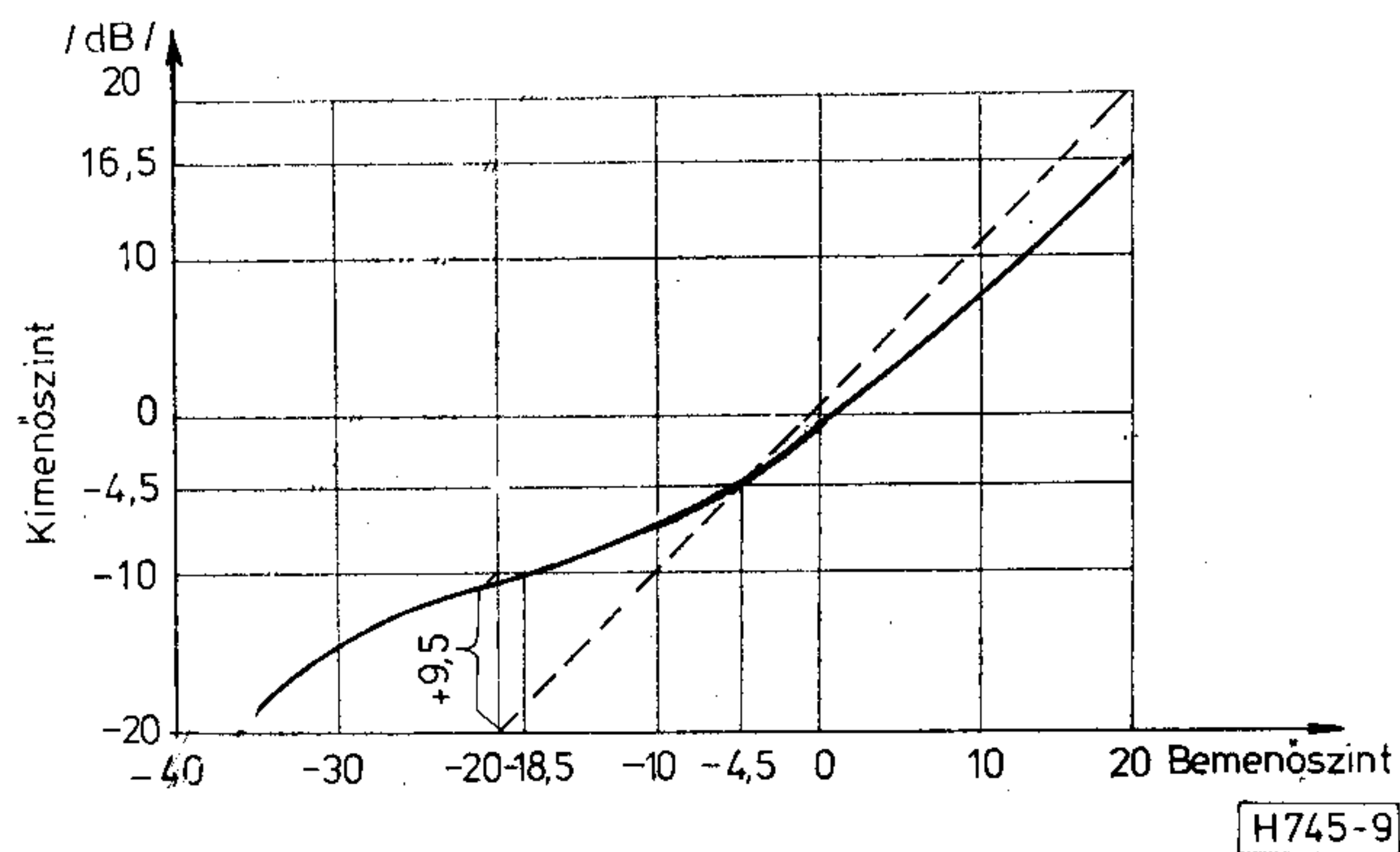
9. ábra. A CCITT által ajánlott kompresszor-karakterisztika
