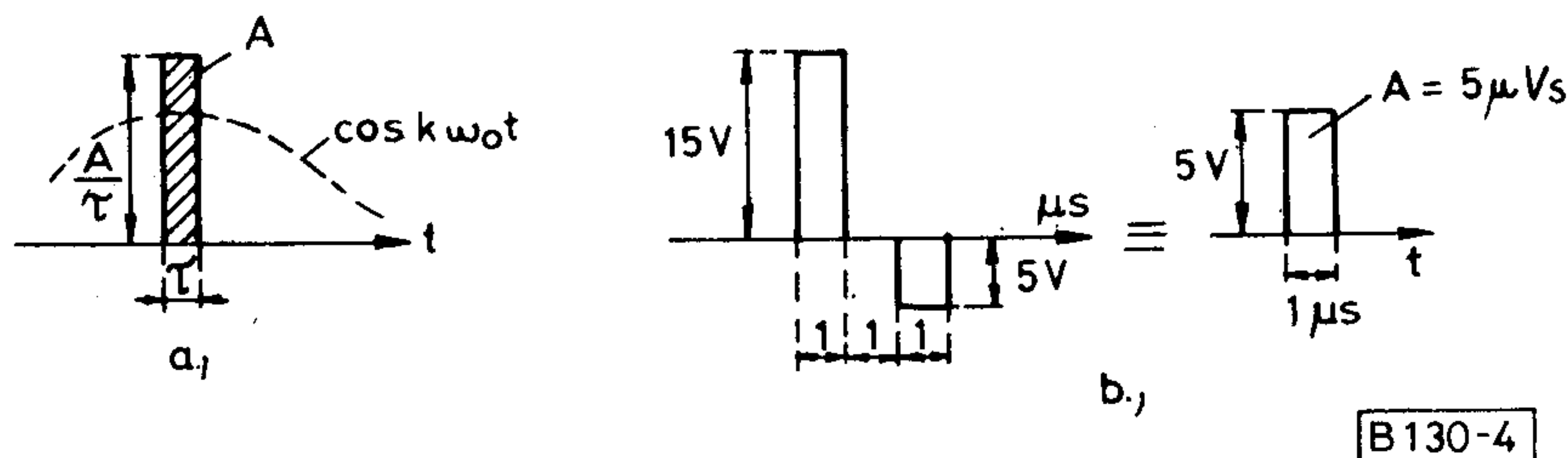
4. ábra. Az impulzus alakjának a hatása a Fourier. komponensre
