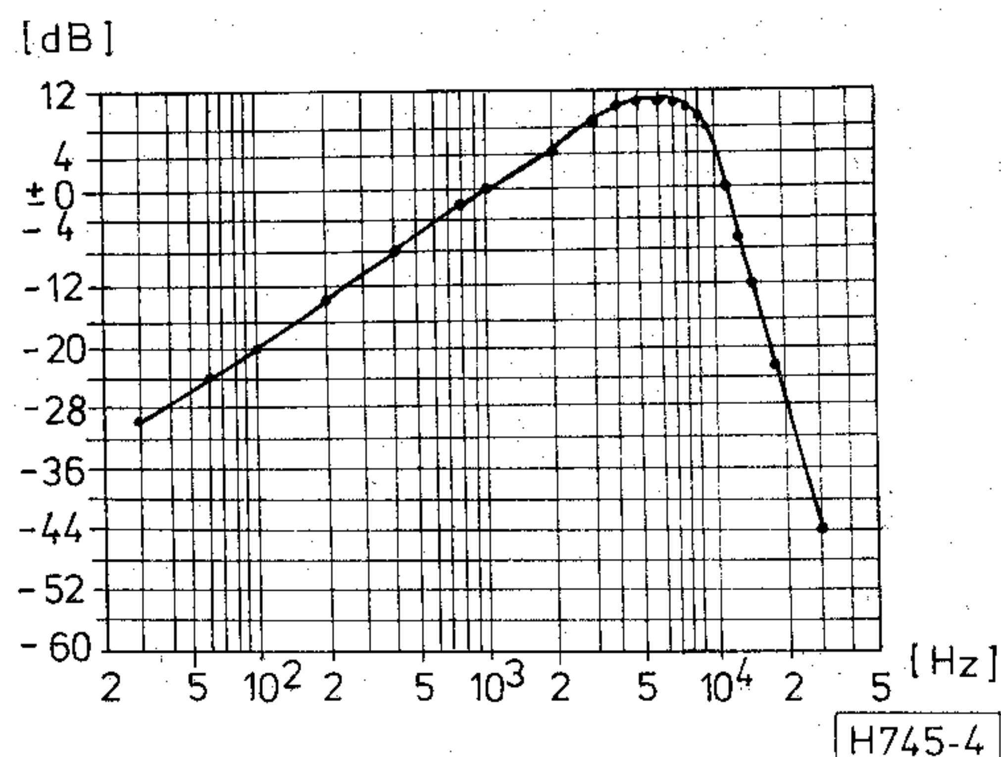
4. ábra. A CCIR 468—1 ajánlás súlyozógörbéje
