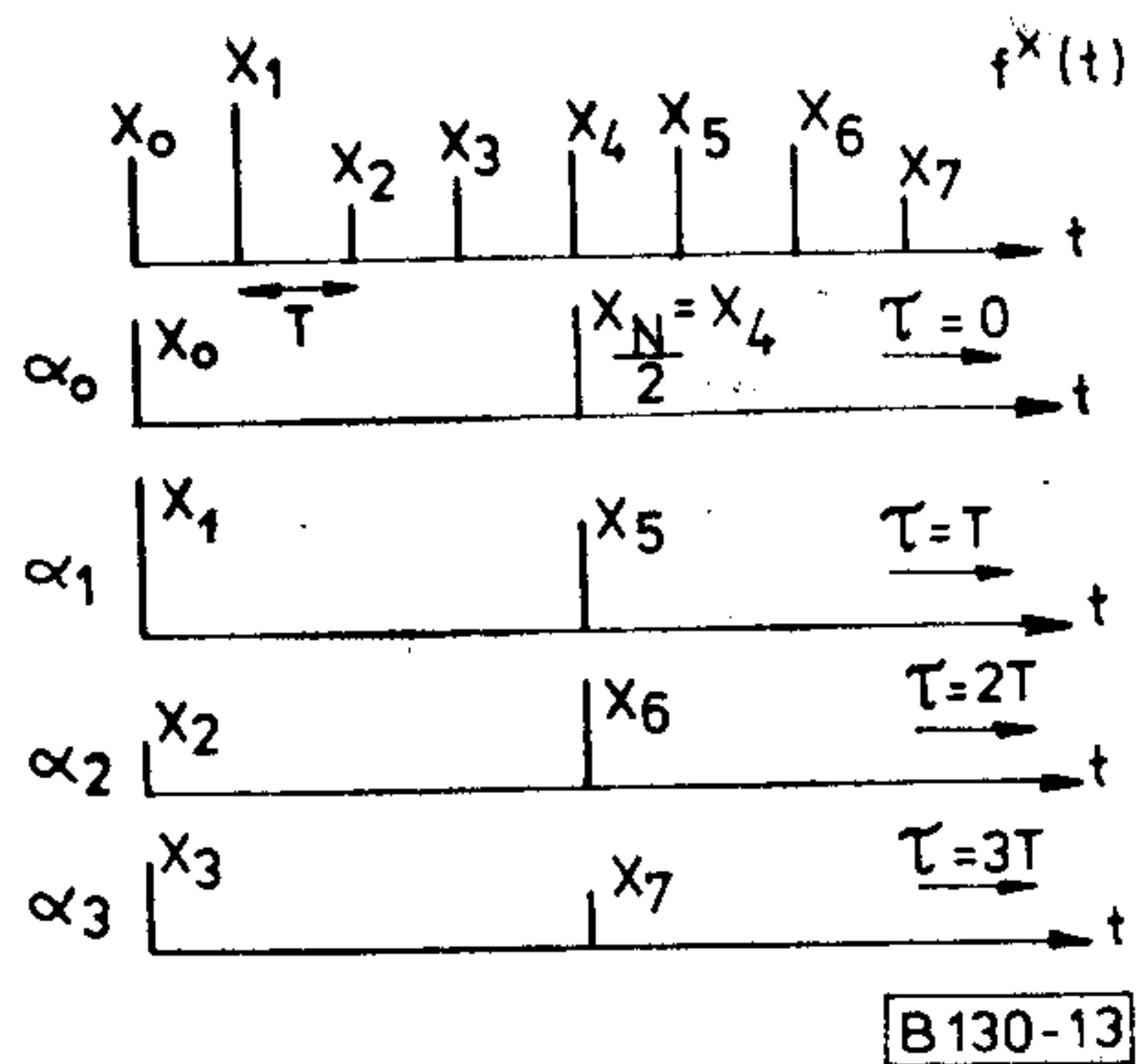
13. ábra. f^*(t) felbontása impulzuspárookra
