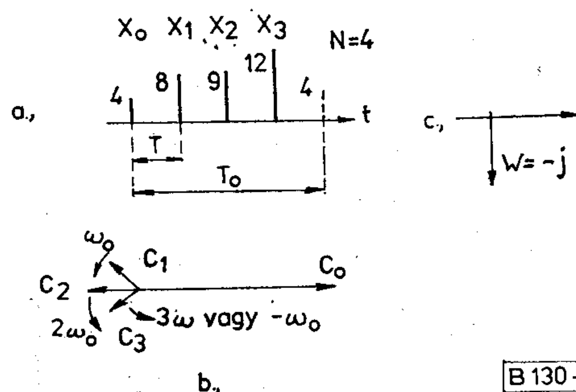
22. ábra. Példa DFT számítására
