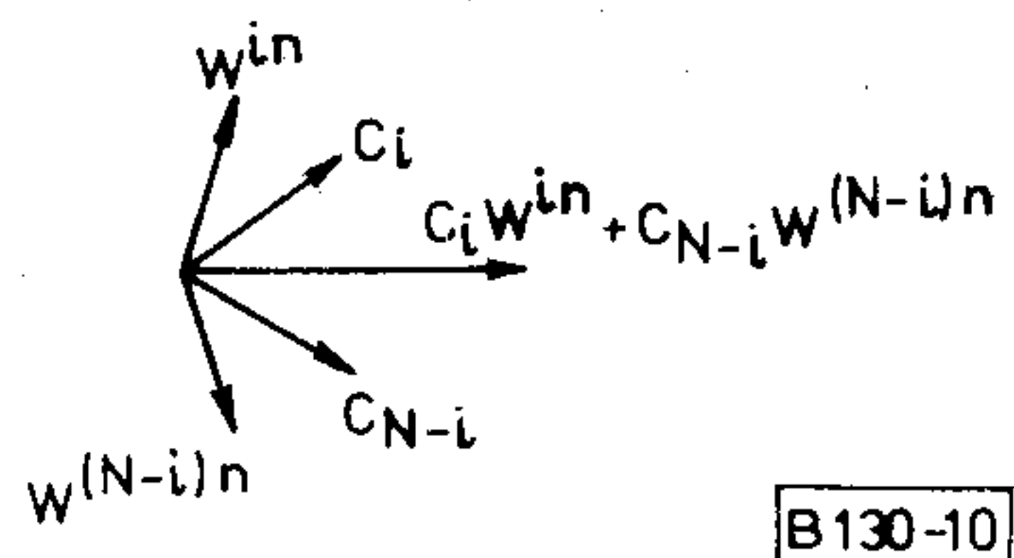
10. ábra. X_n szerkesztése
