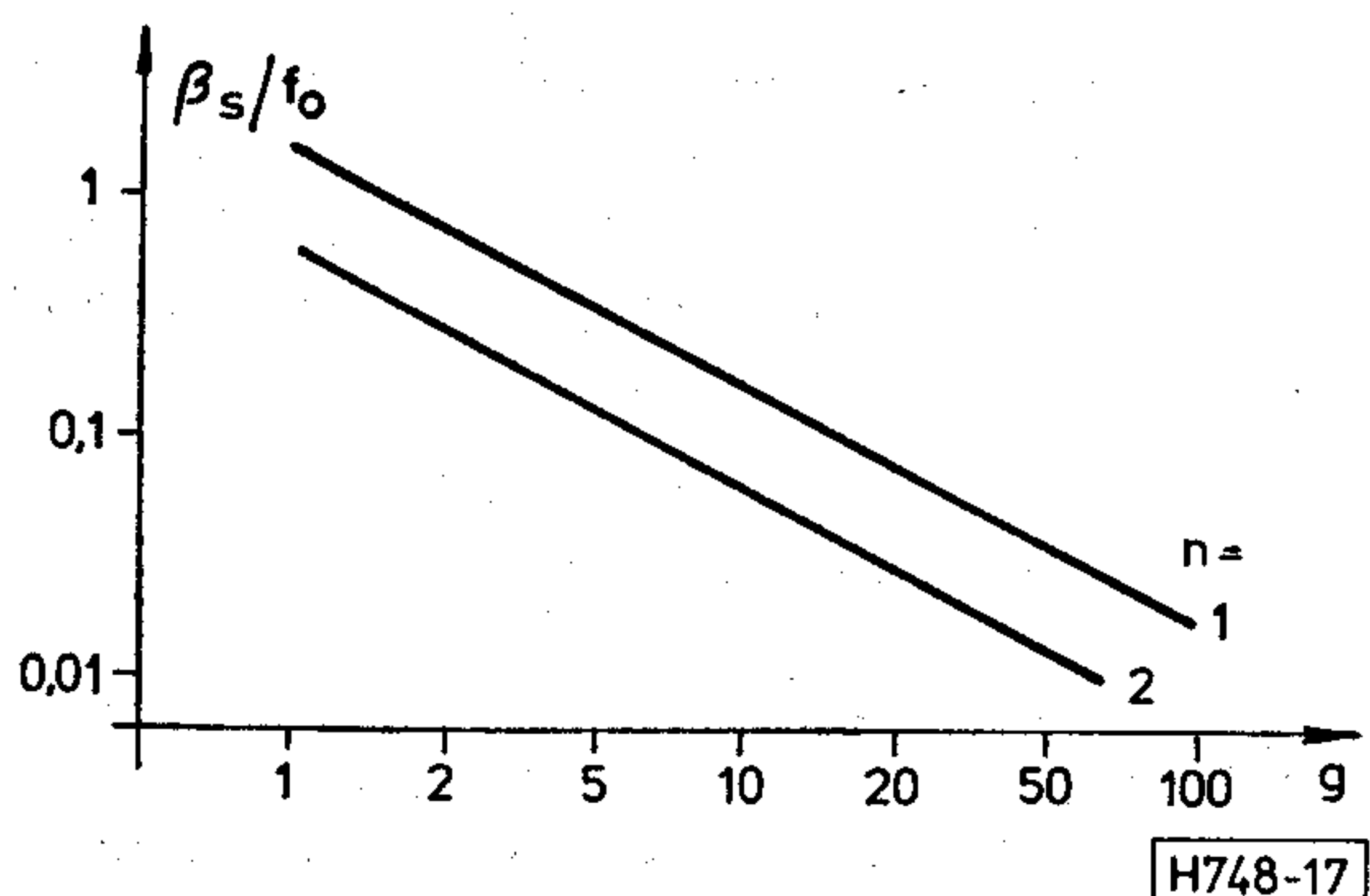
17. ábra. A komparátorszűrő ekvivalens zajszávszélessége komplex póluspárok esetén
