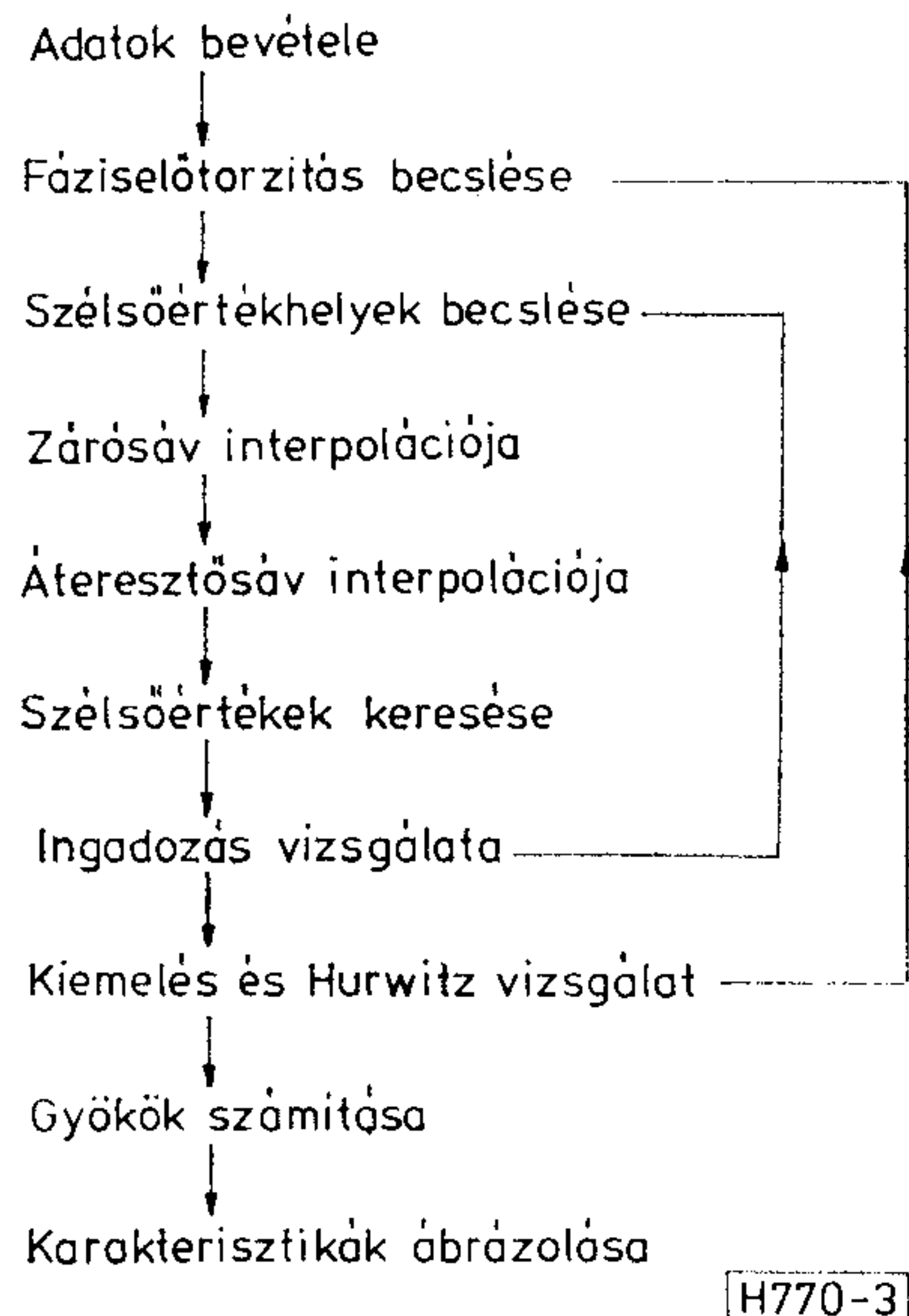
3. ábra. Egyszerűsített algoritmusvázlat
