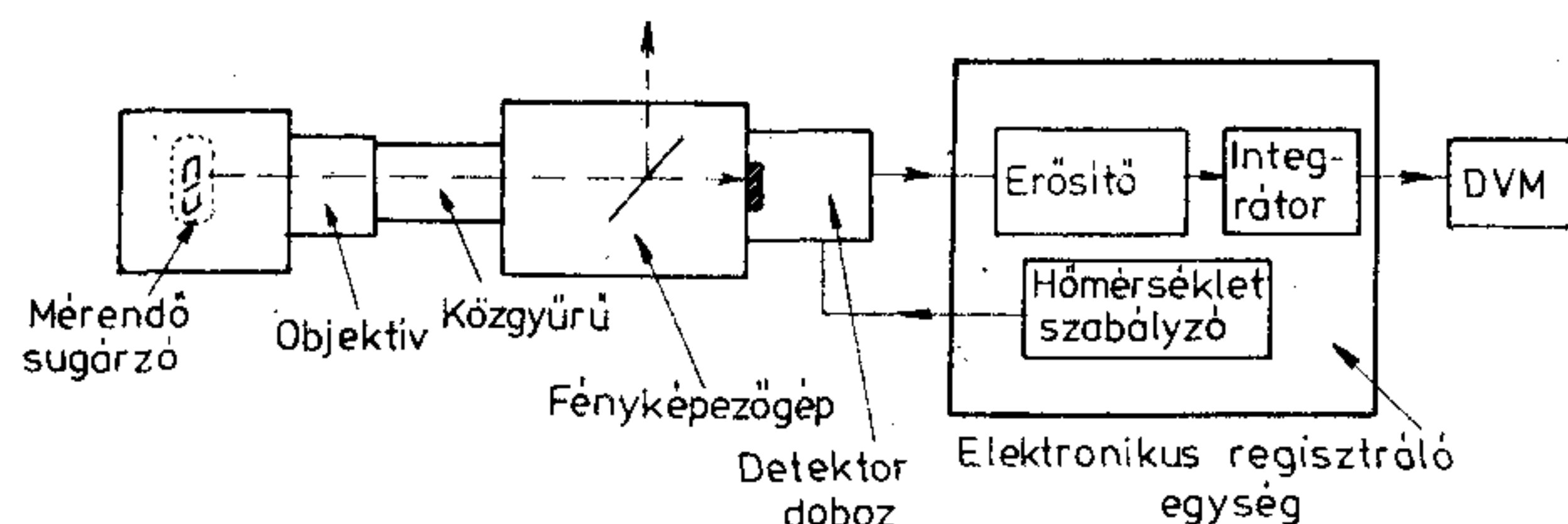
5. ábra. A fényssűrűségmérő rendszer egységei
