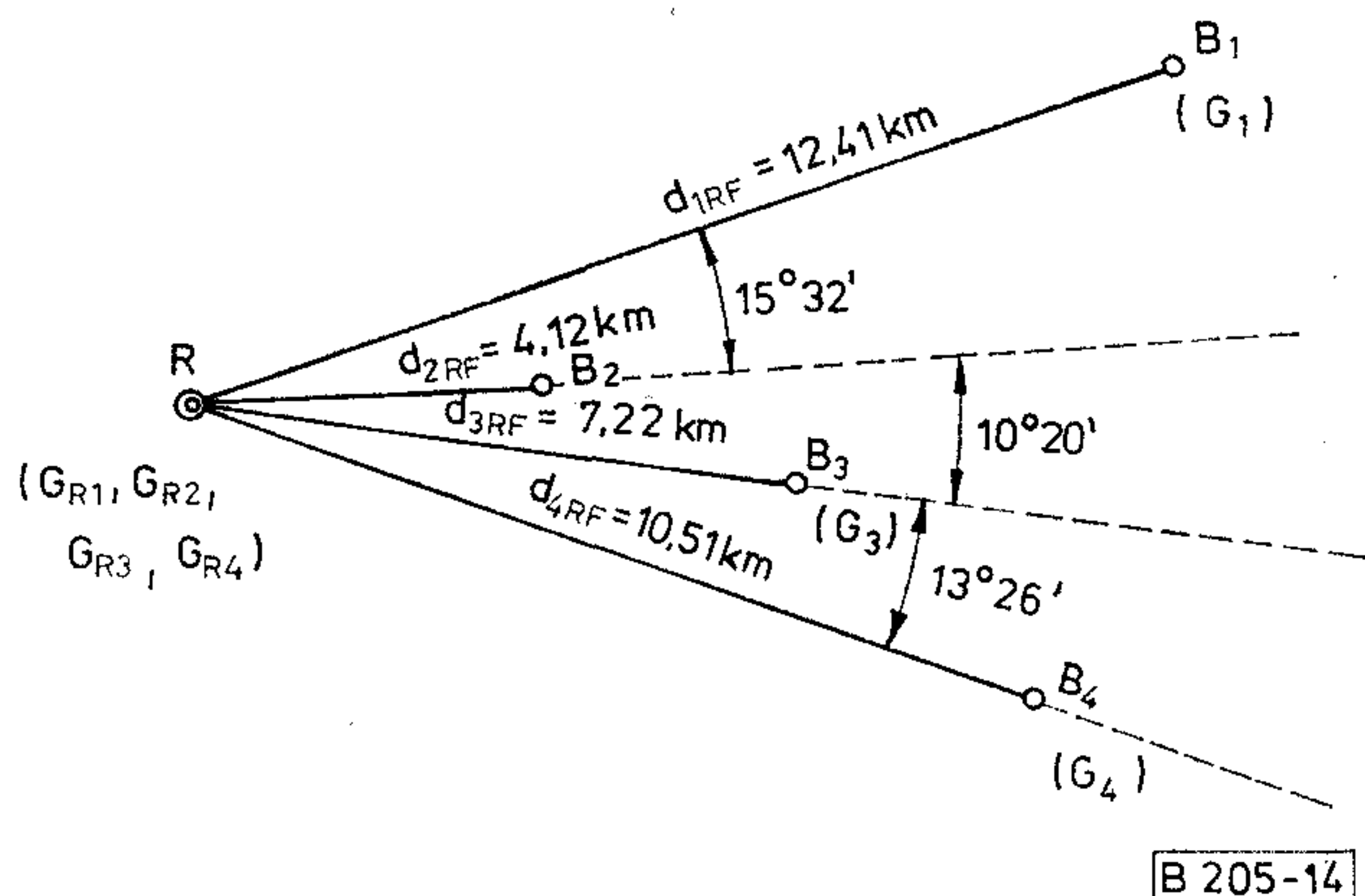
14. ábra. Átkérőhálózat
