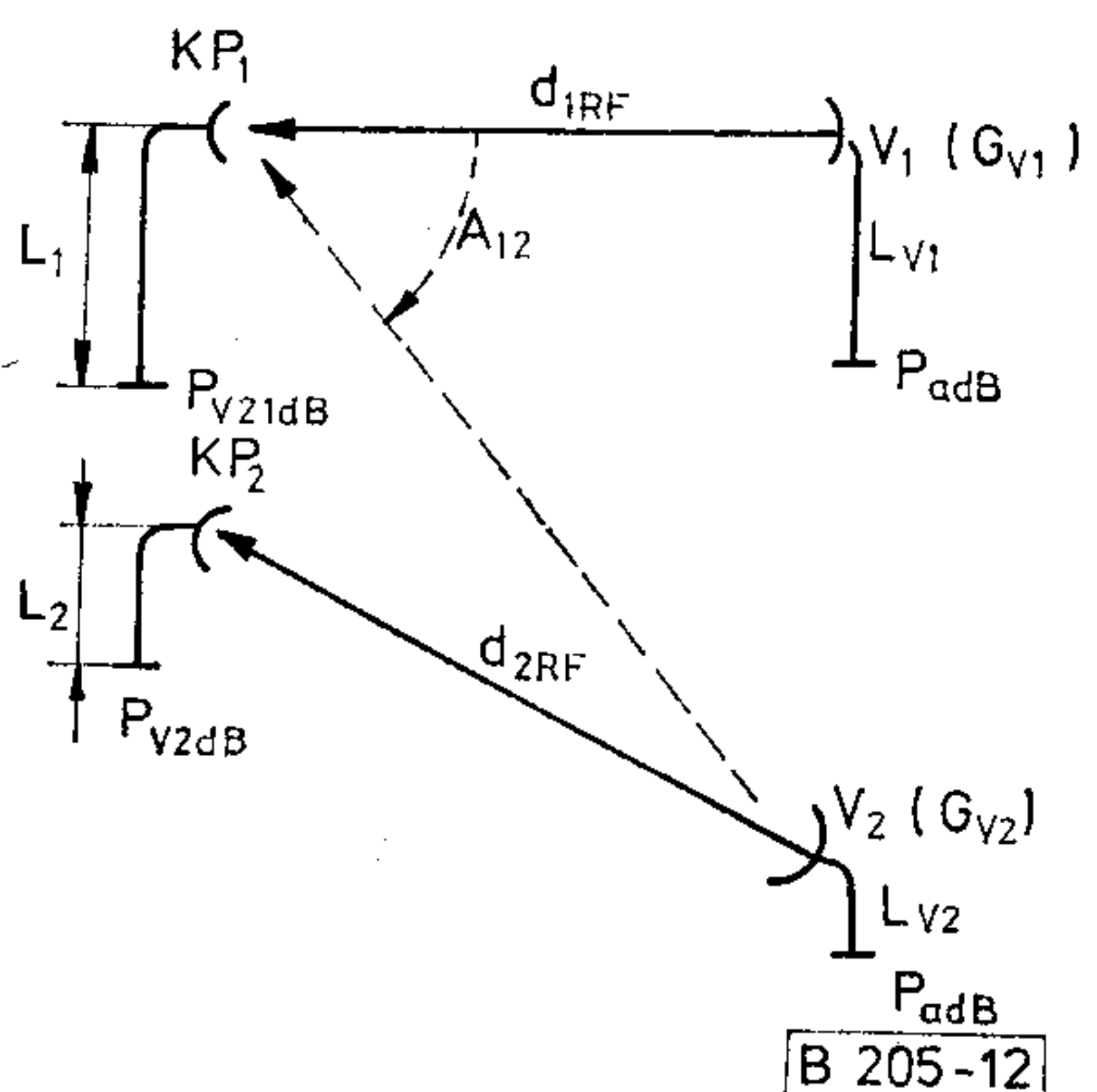
12. ábra. Vételinterferencia
