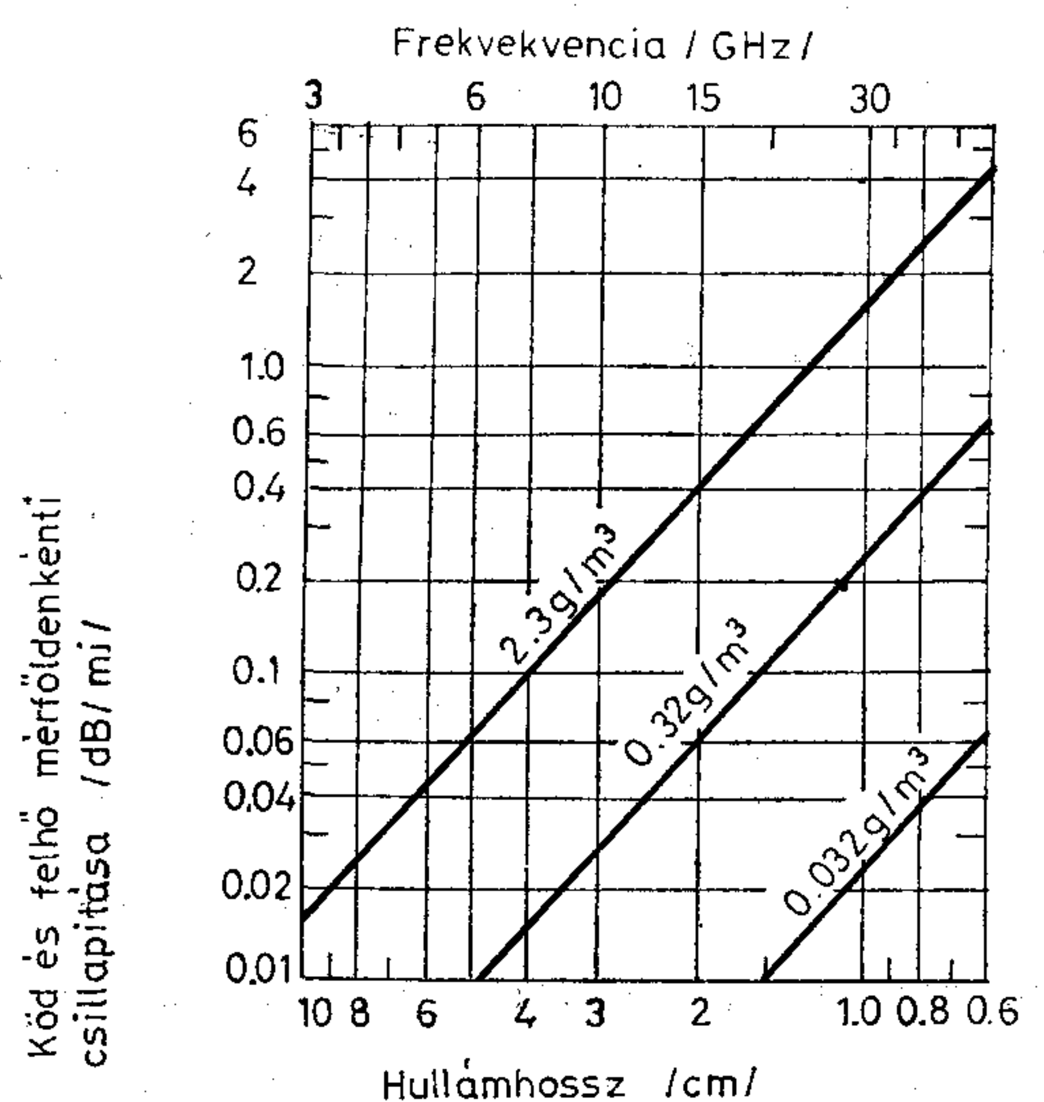
4. ábra. A köd és felhő mérföldenkénti csillapítása (1 szárazföldi mérföld = 1609,33 m)
