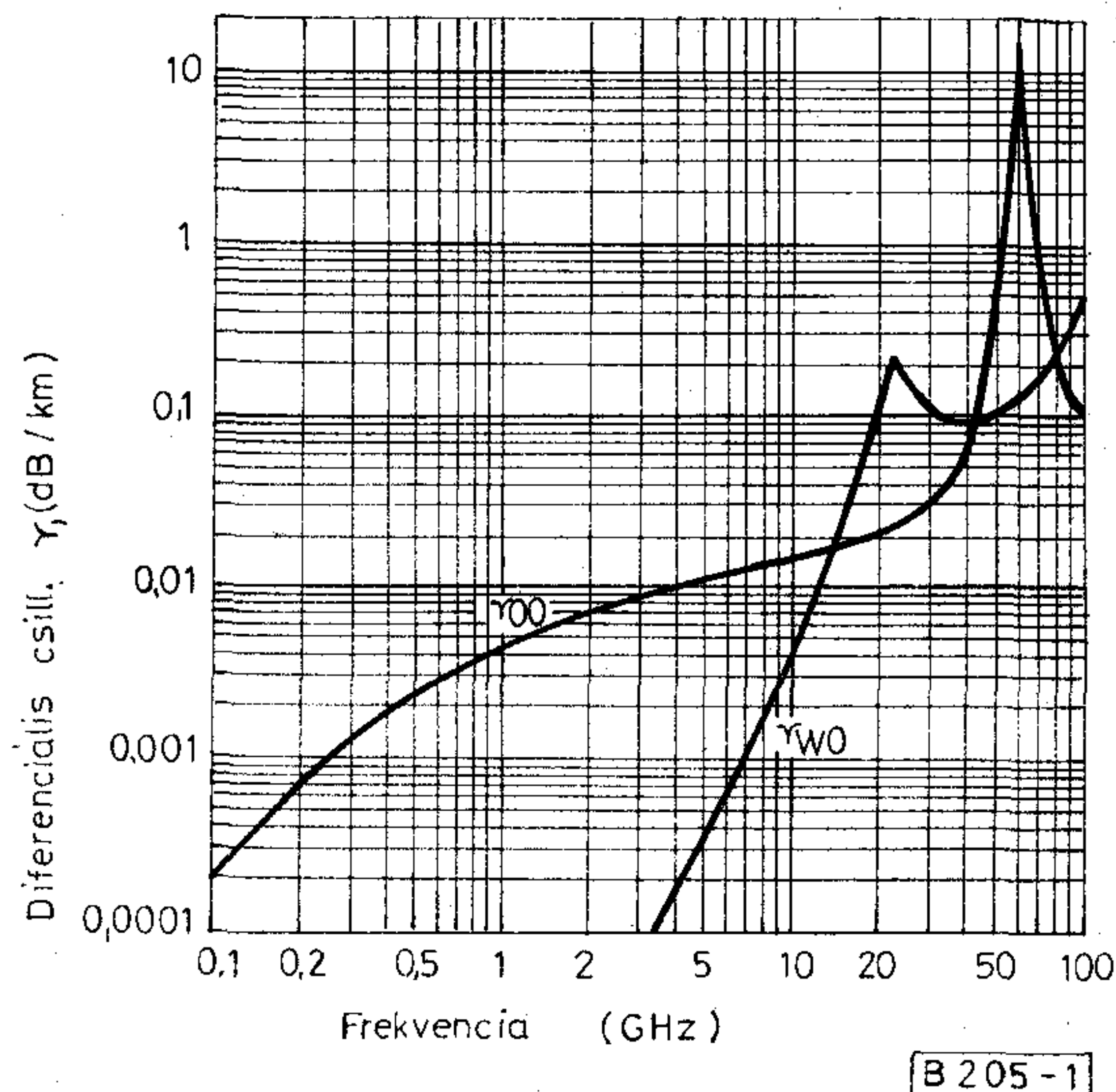
1. ábra. Az oxigén és a vízgőz csillapítása a frekvencia függvényében. Abszcissa: frekvencia (GHz); Ordináta: km-enkénti csillapítás (db/km)
