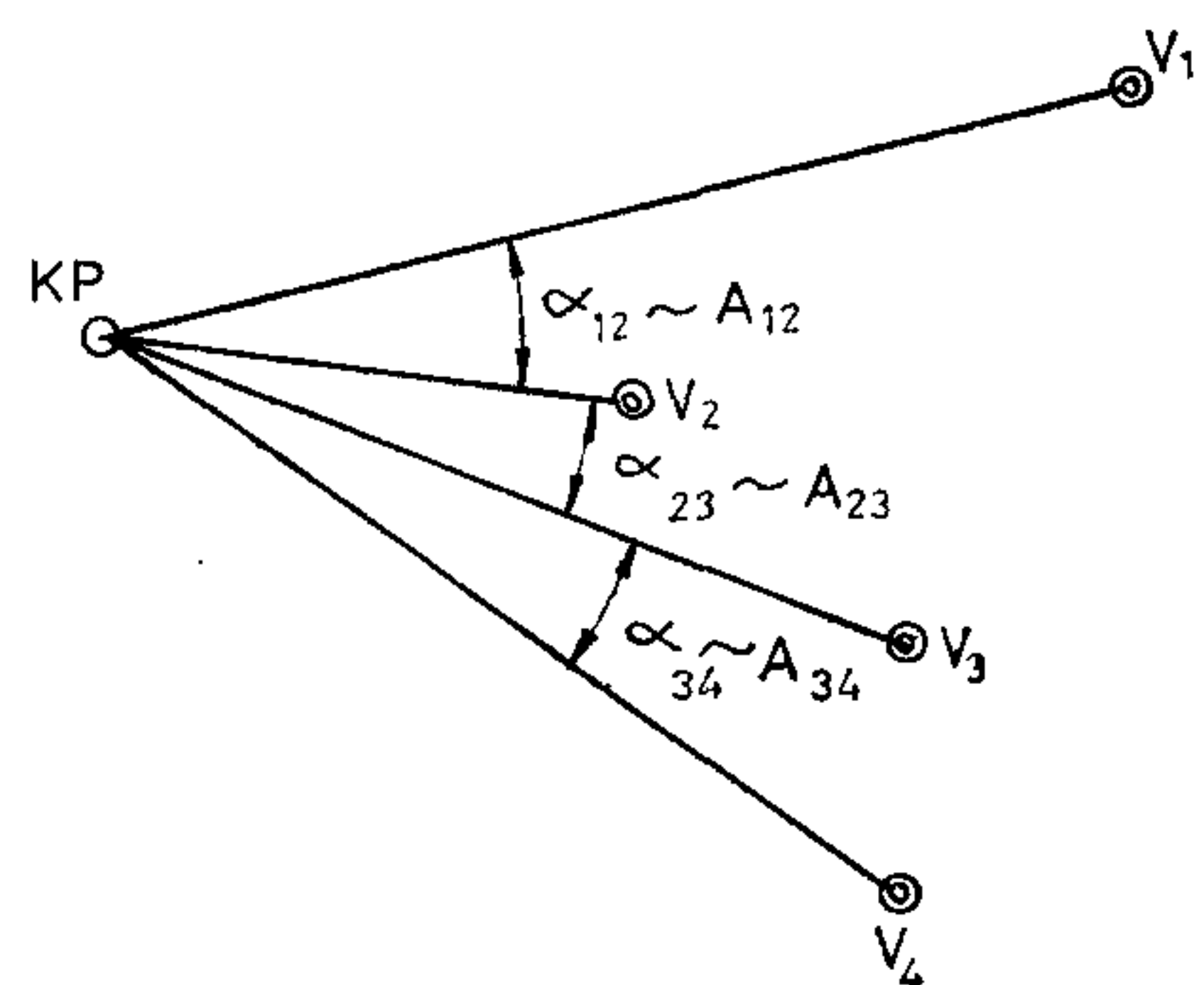
11. ábra. Csillag-hálózat
