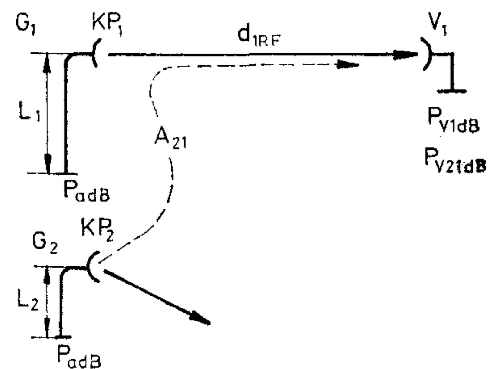
10. ábra. Adásinterferencia
