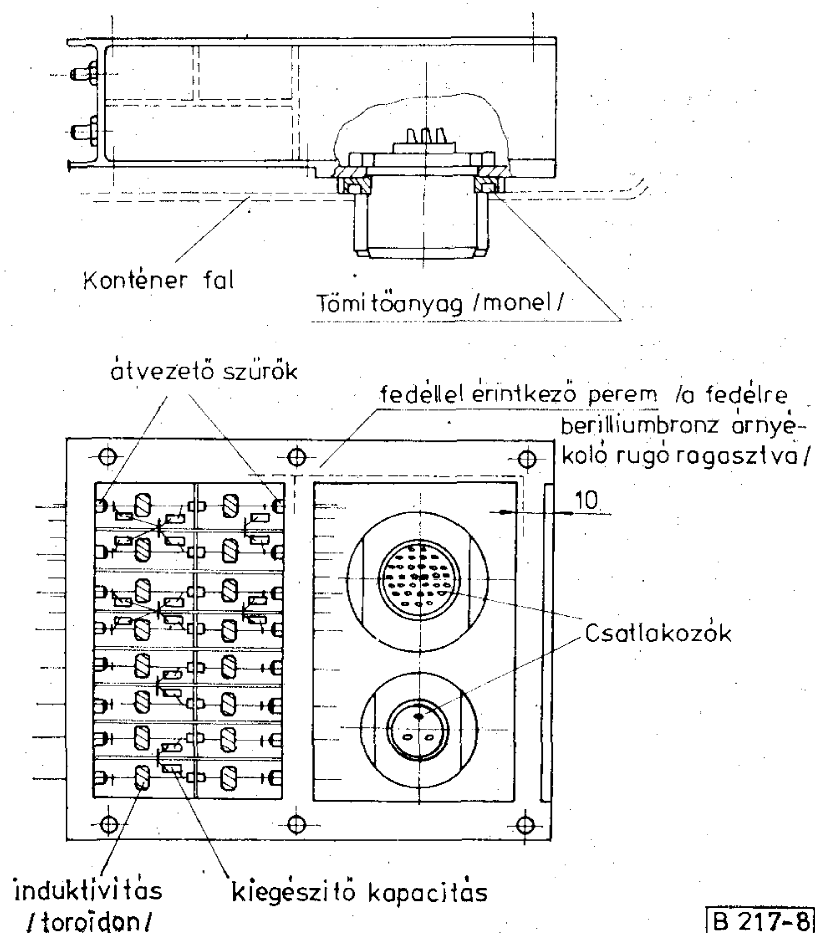
8. ábra. Szűrőegység
