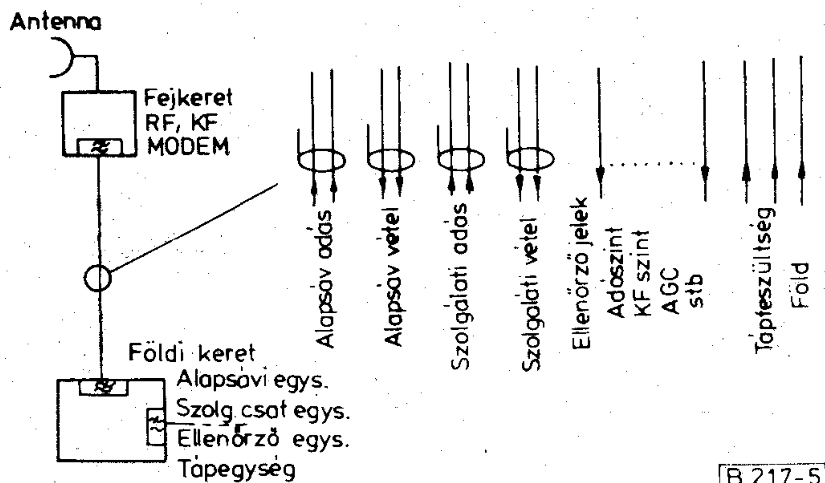
5. ábra. 24 csatornás FM berendezés elrendezési vázlata
