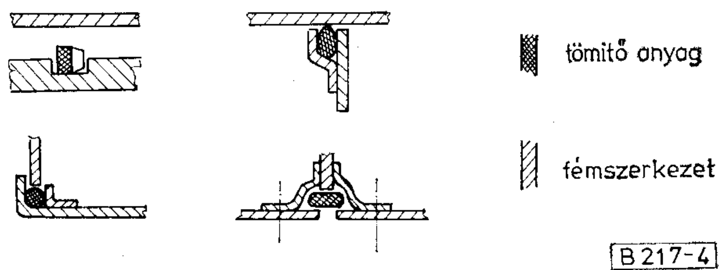
4. ábra. Tipikus RF tömítések
