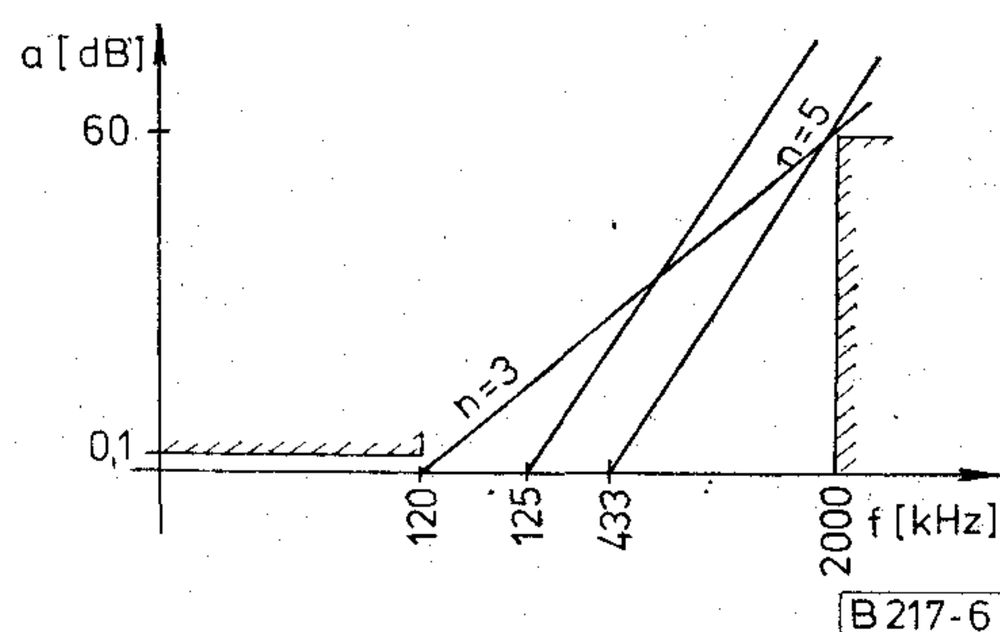
6. ábra. Tolerancia séma
