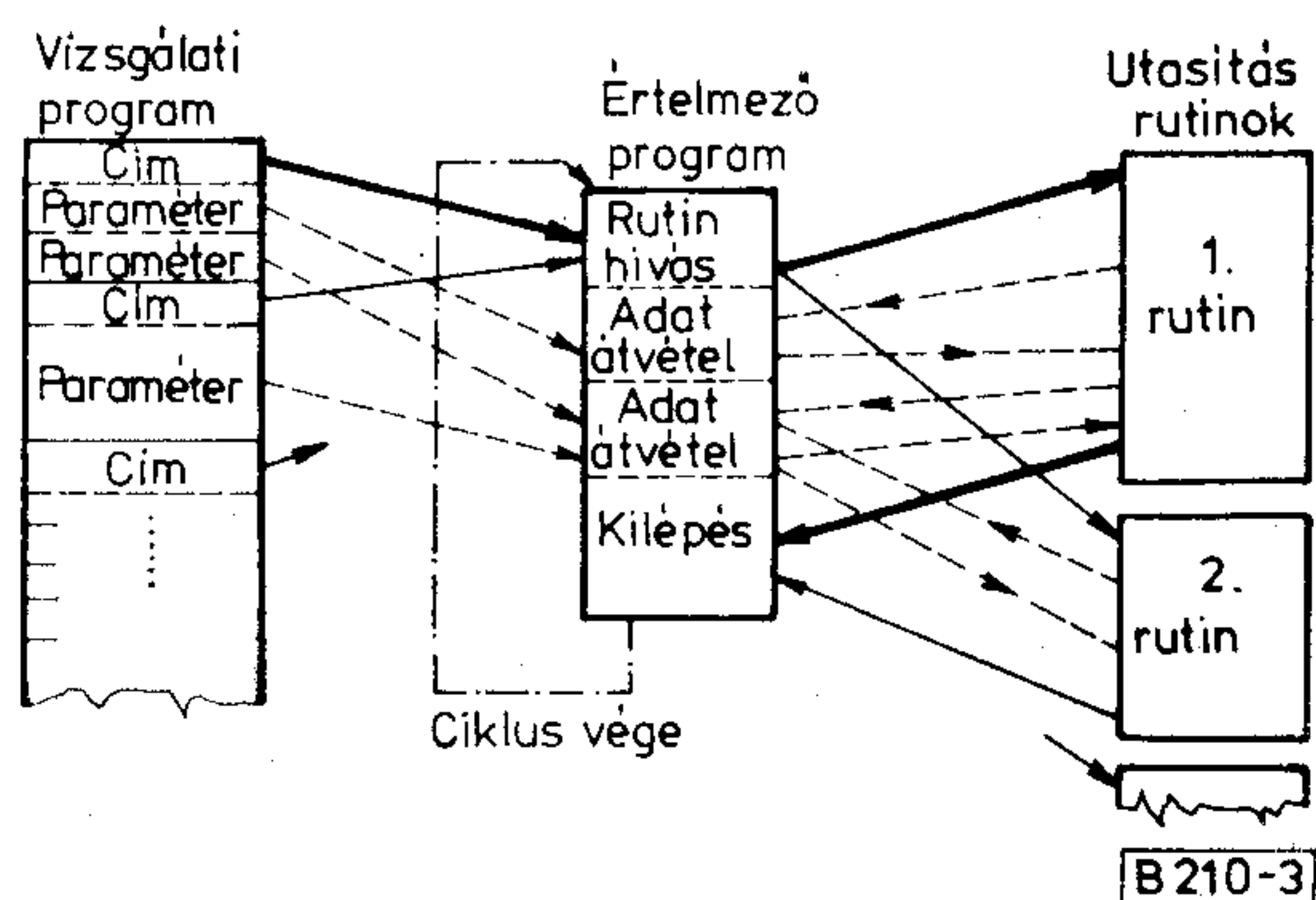
3. ábra. Vizsgálati programrendszer felépítése
