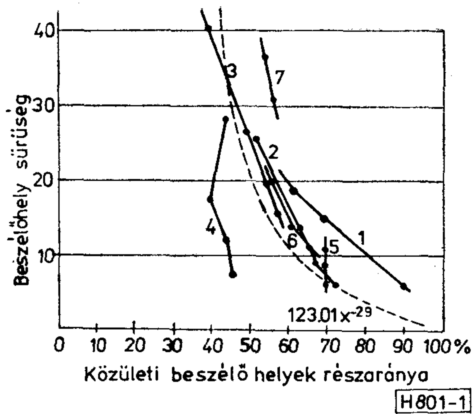
1. ábra. Közületi beszélőhelyek %-os arányának változása a beszélőhely sűrűség függvényében: 1. Japán, 2. Spanyolo., 3. Anglia, 4. Olaszo., 5. Magyaro., 6. Csehszlovákia, 7. Svájc, 8. Korrelációs görbe
