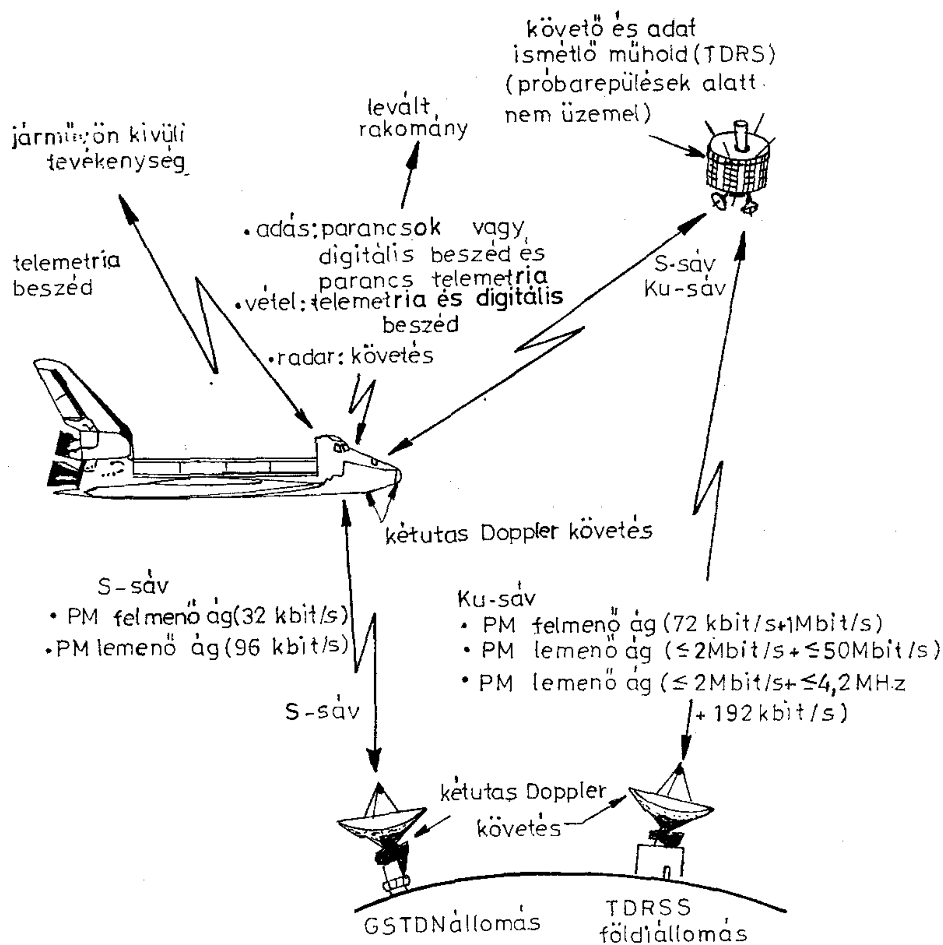
1. ábra. Az orbiter rádiófrekvenciás rendszerei
