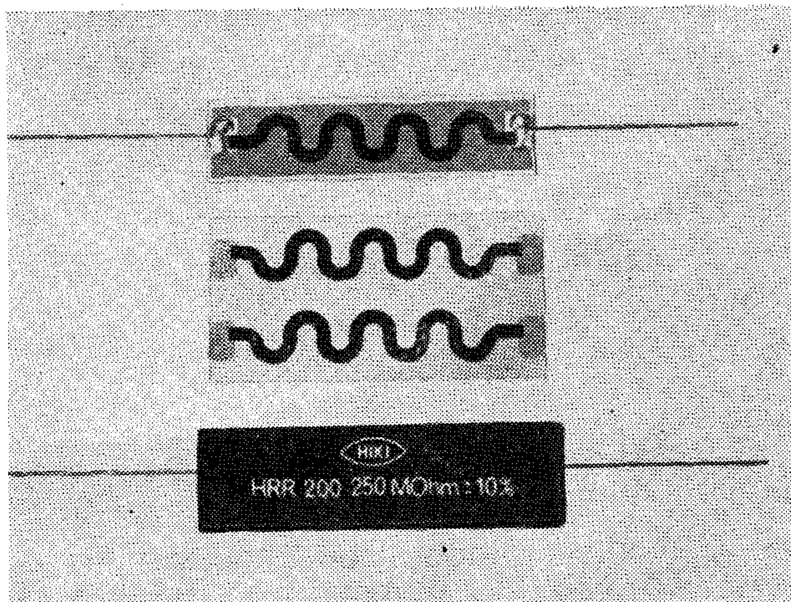
Nagyfeszültségű ellenállások
