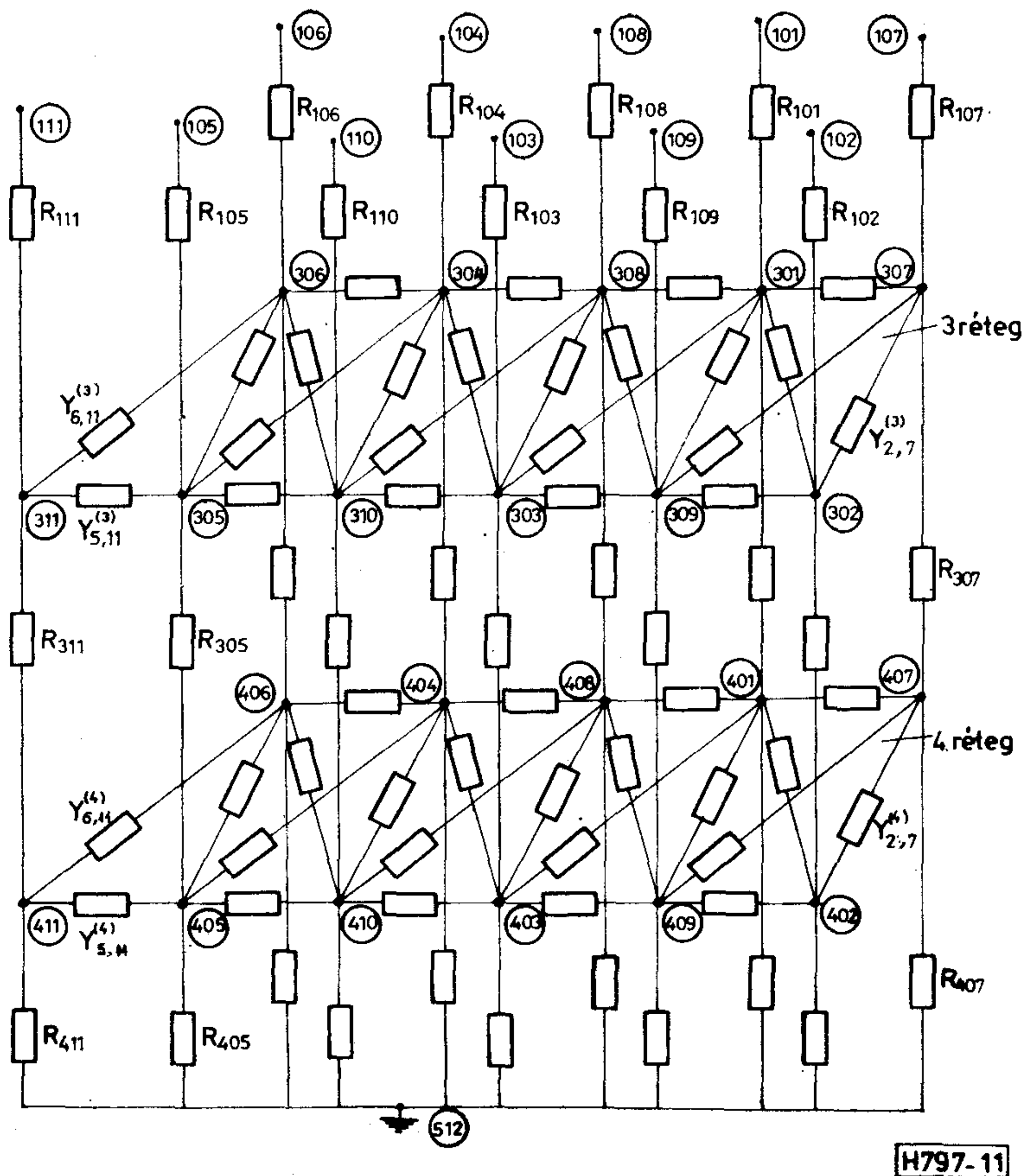
11. ábra. A memória áramkör termikus helyettesítő hálózata
