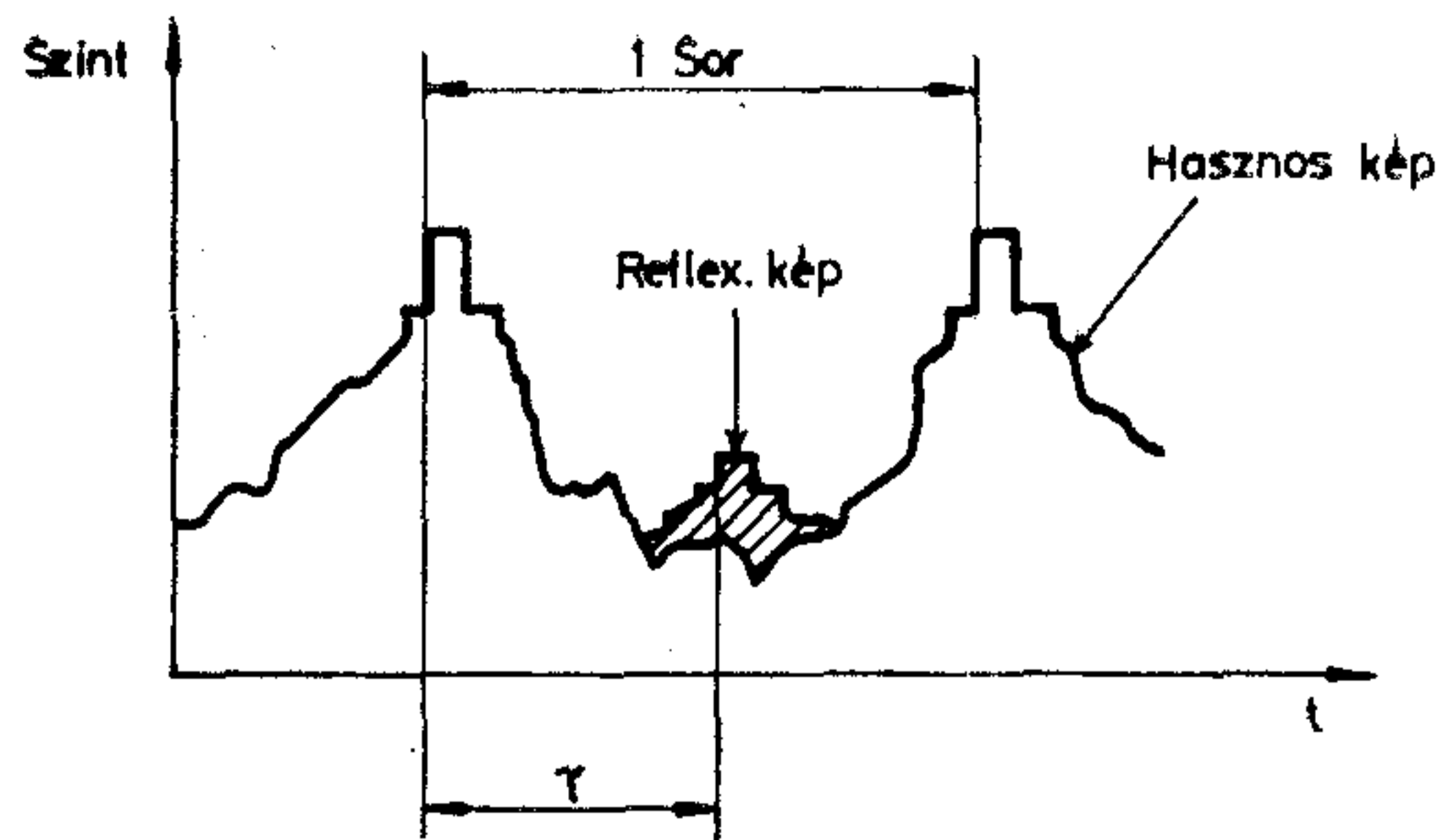
2. ábra Televíziós jel szintdiagramja zavaró szinkronimpulzussal
