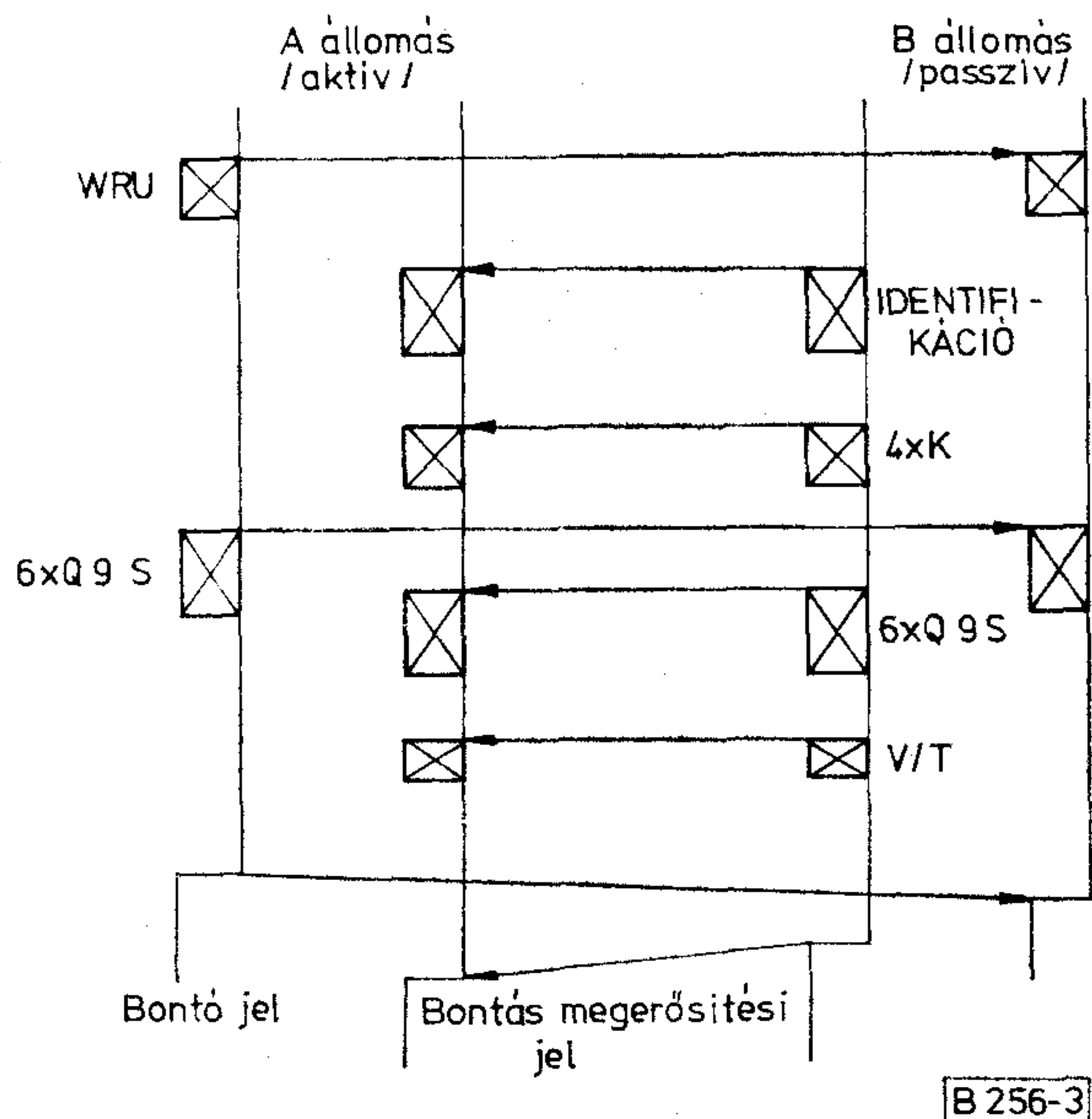
3. ábra. Aktív és passzív berendezés közötti kommunikáció idődiagramja
