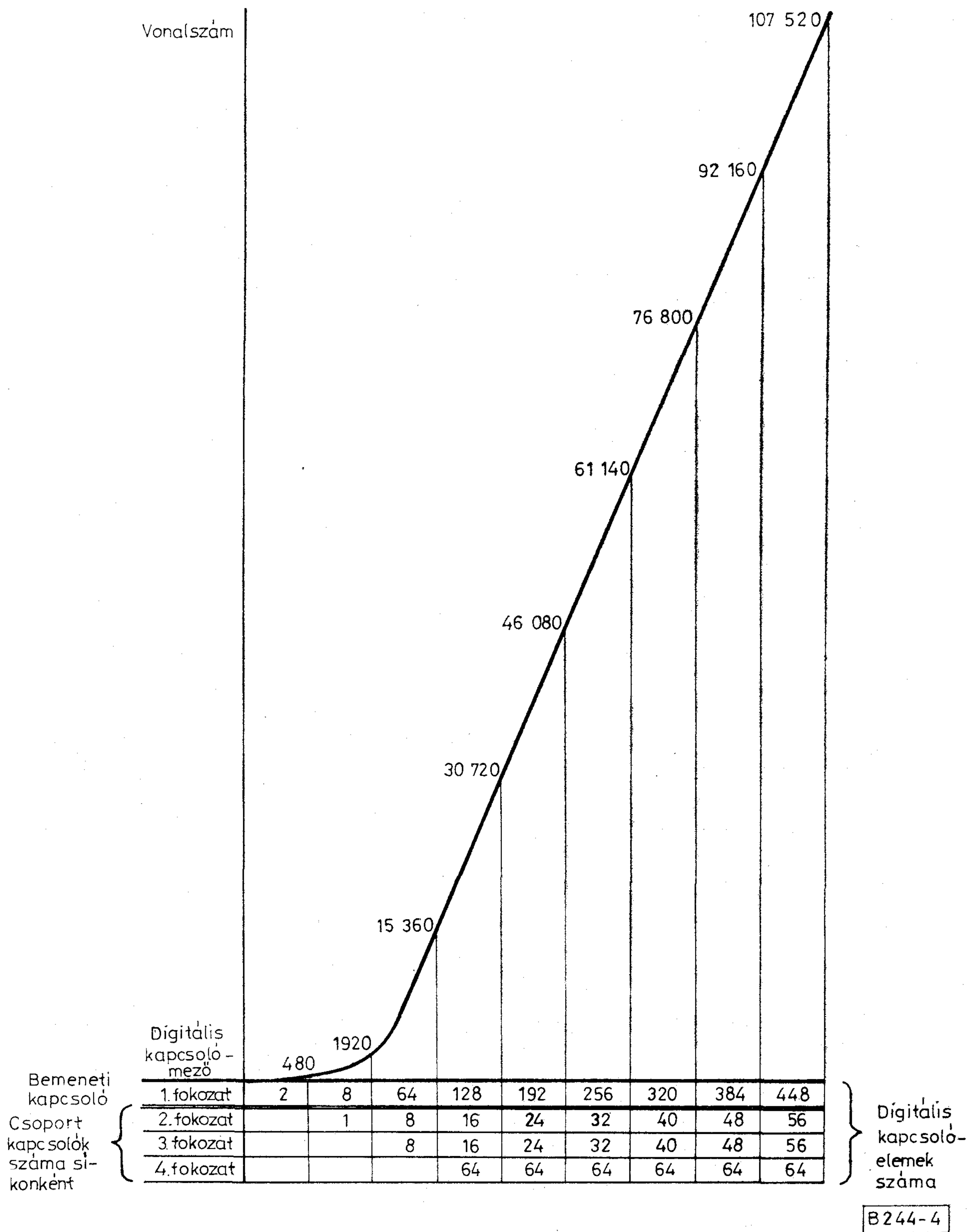
4. ábra. A központ bővíthetősége
