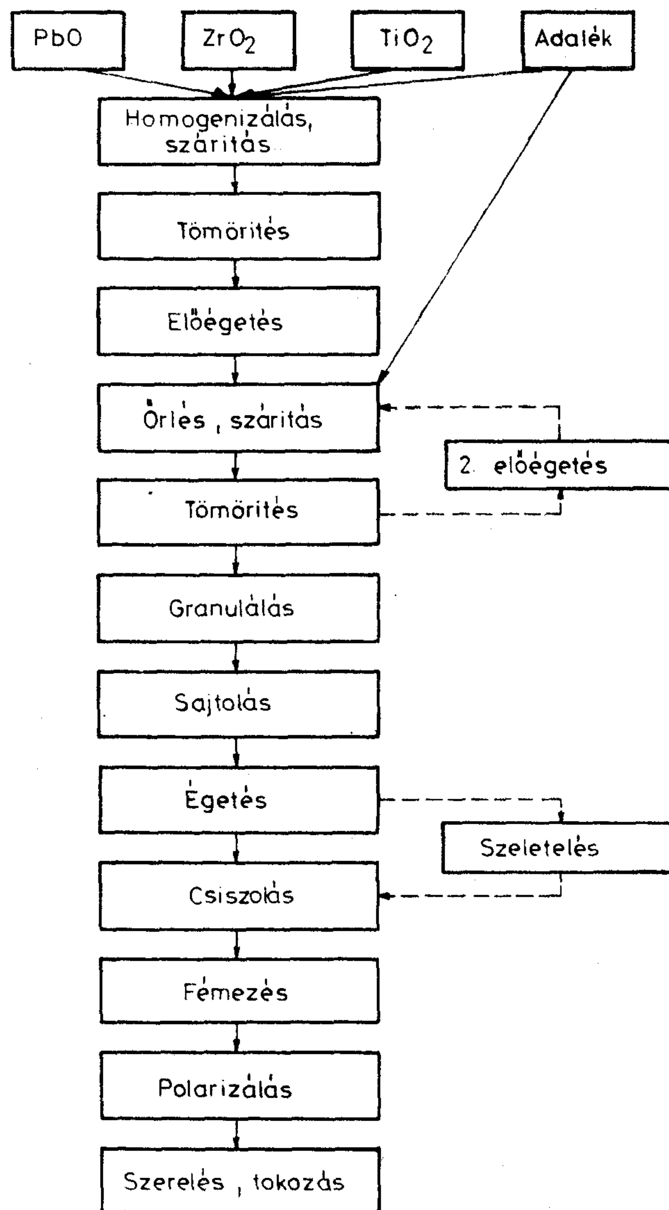
2. ábra. Piezokerámiai alkatrészek gyártása
