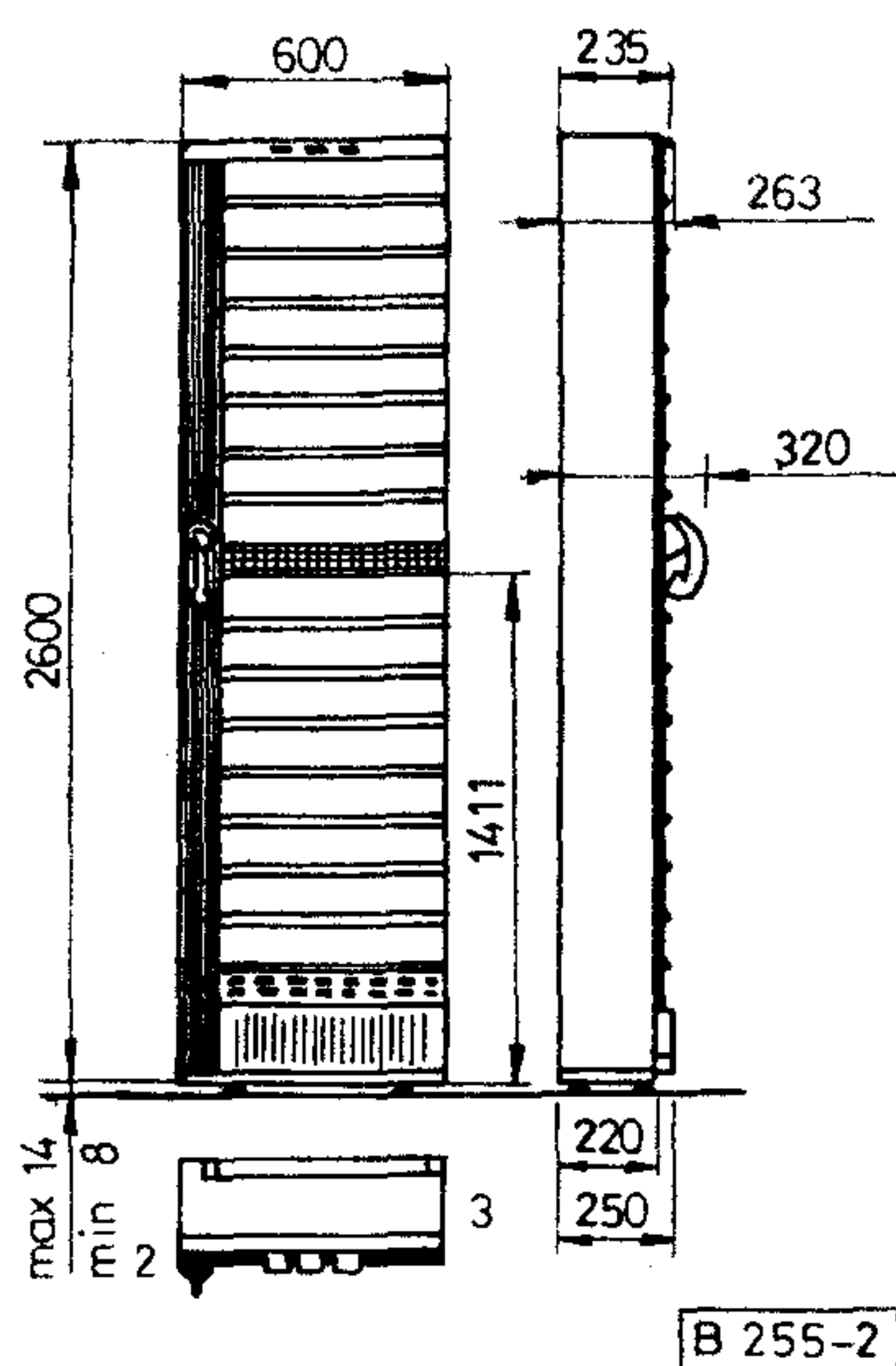
2. ábra. TERTA E 2 konstrukciója
