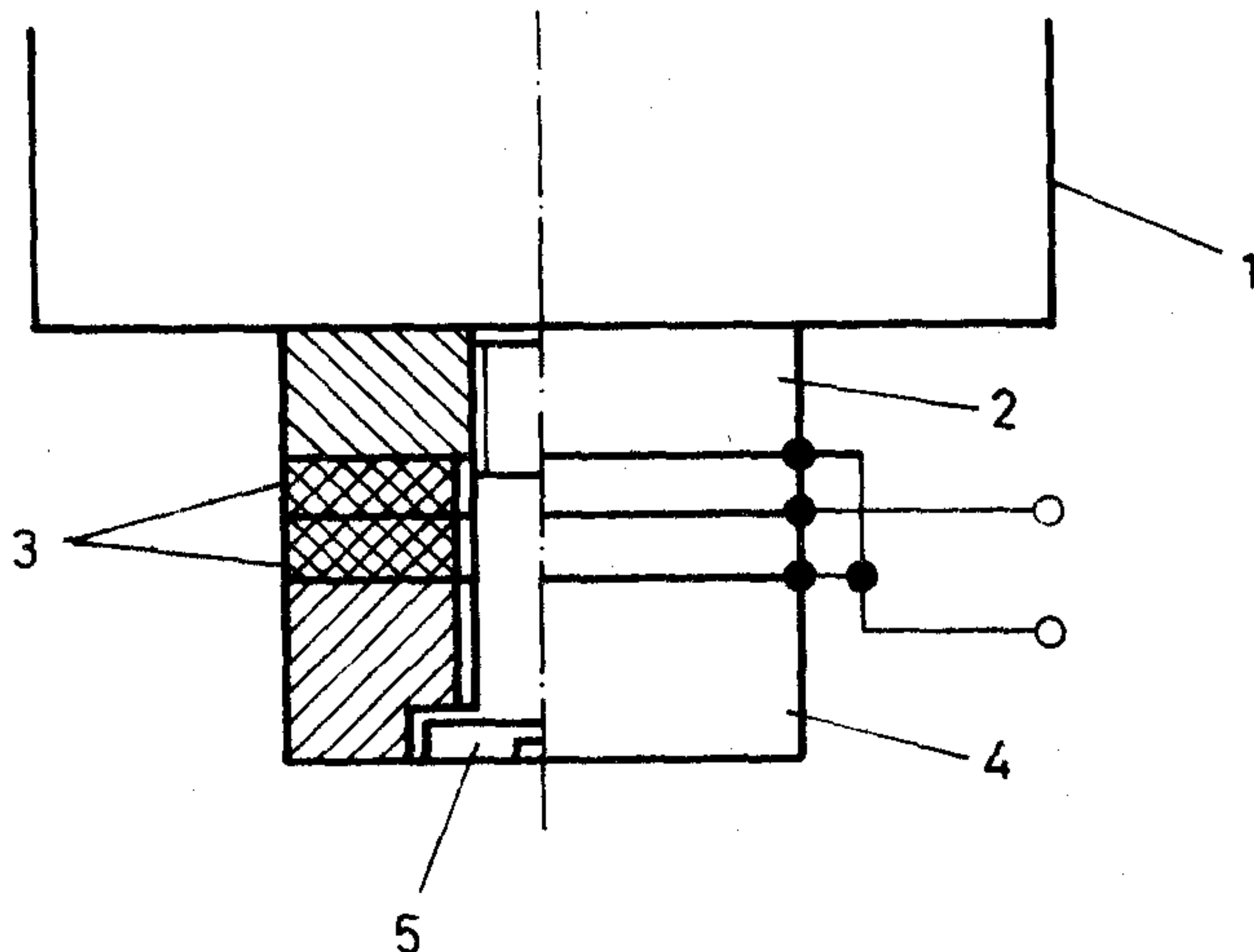
7. ábra. Ultrahangos tisztítóberendezés
