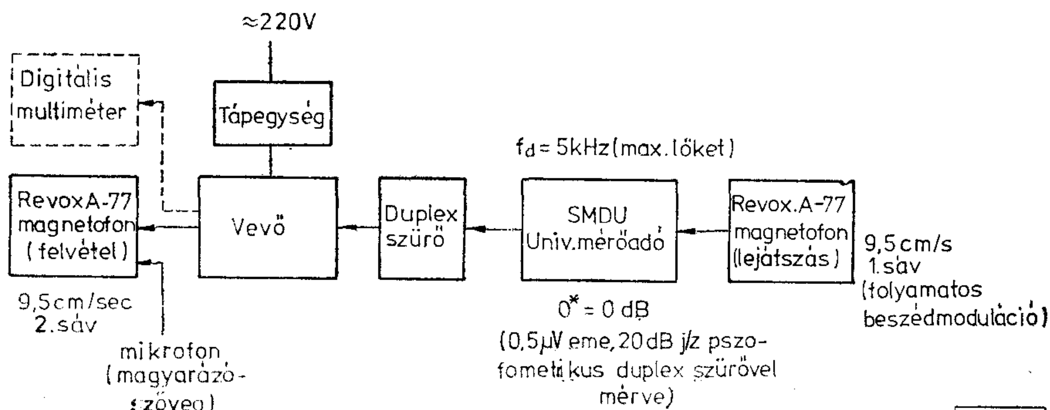
2. ábra. Laboratóriumi mérőelrendezés
