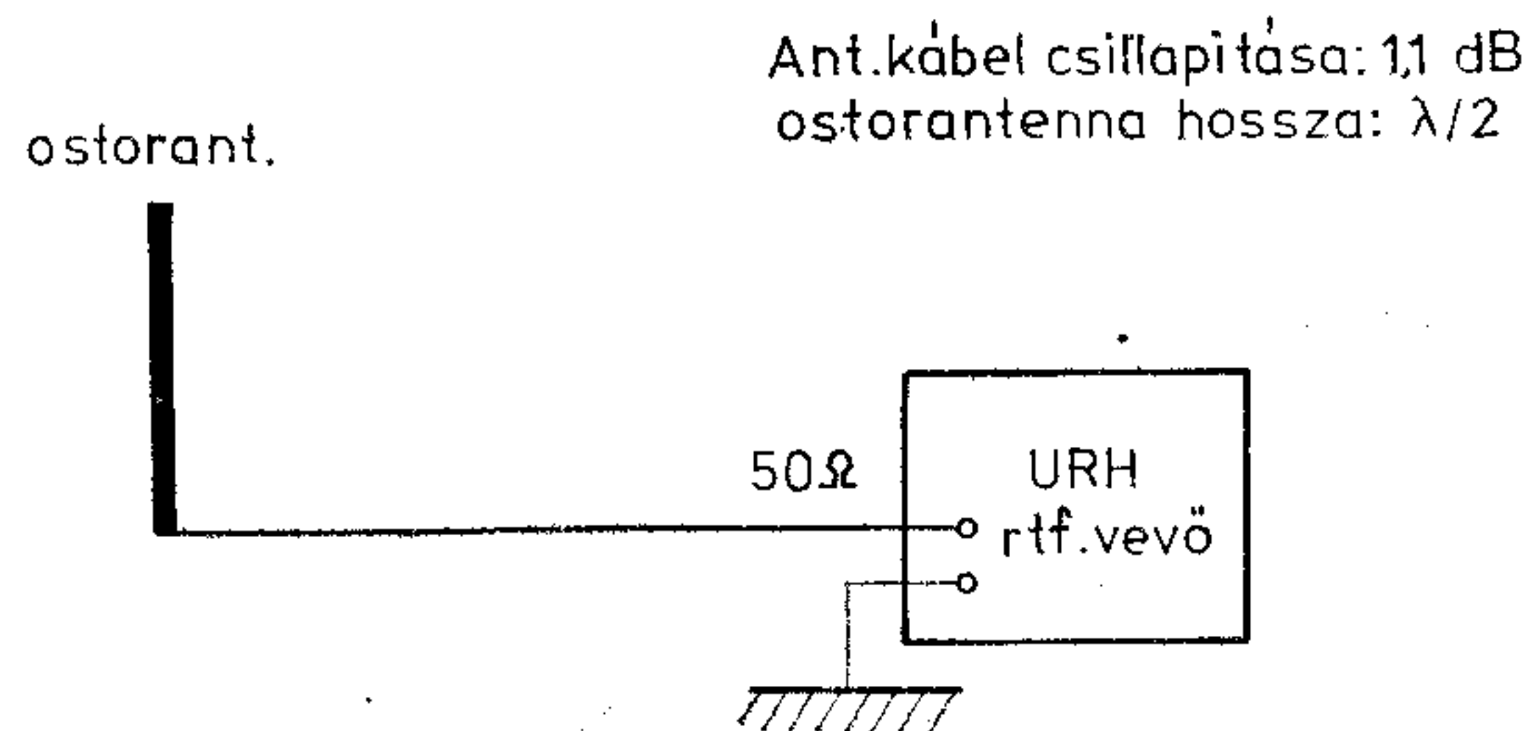
Zajmérés / 160 MHz / elrendezése
