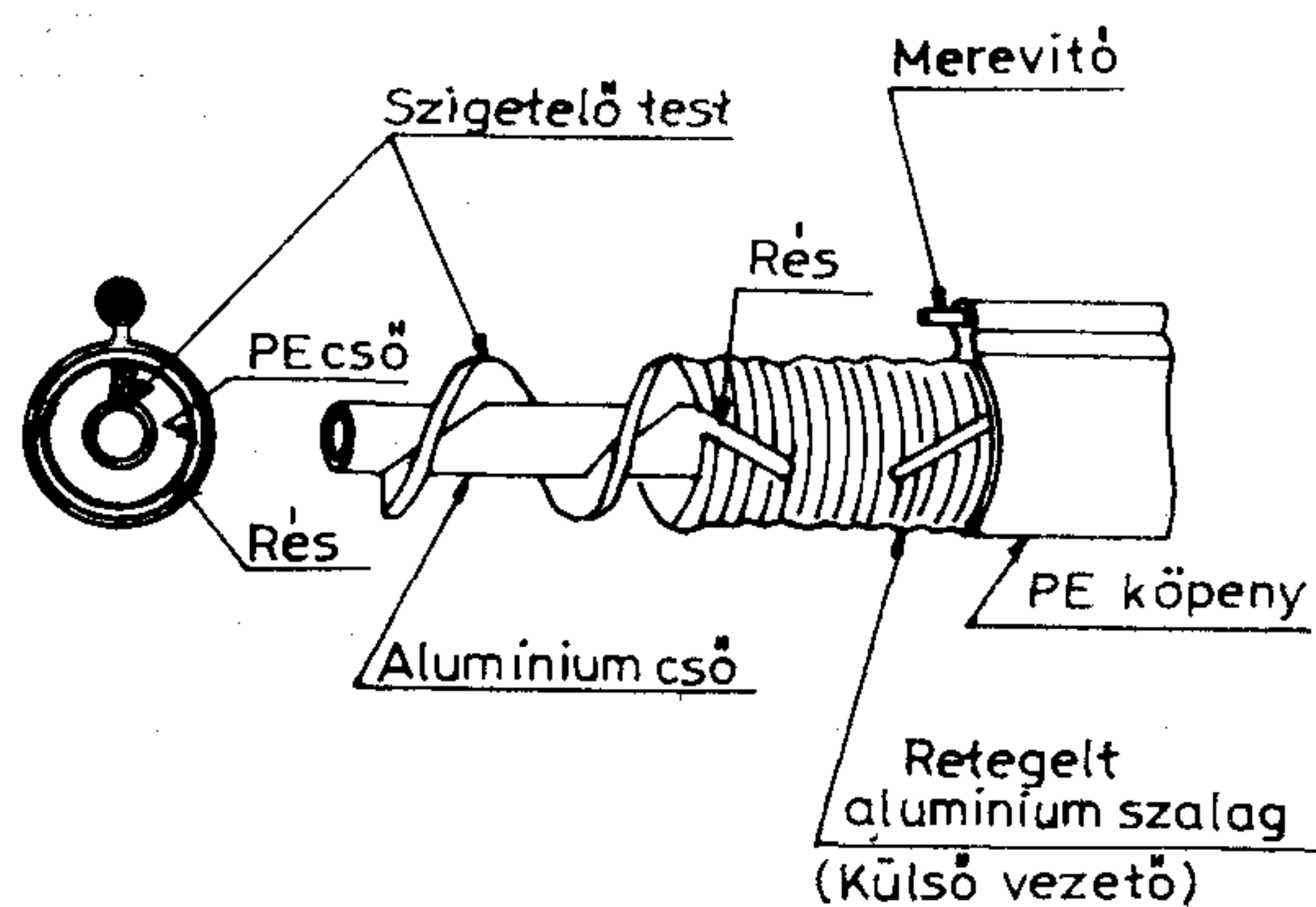
6. ábra. A felhasított koaxiális kábel struktúrája
