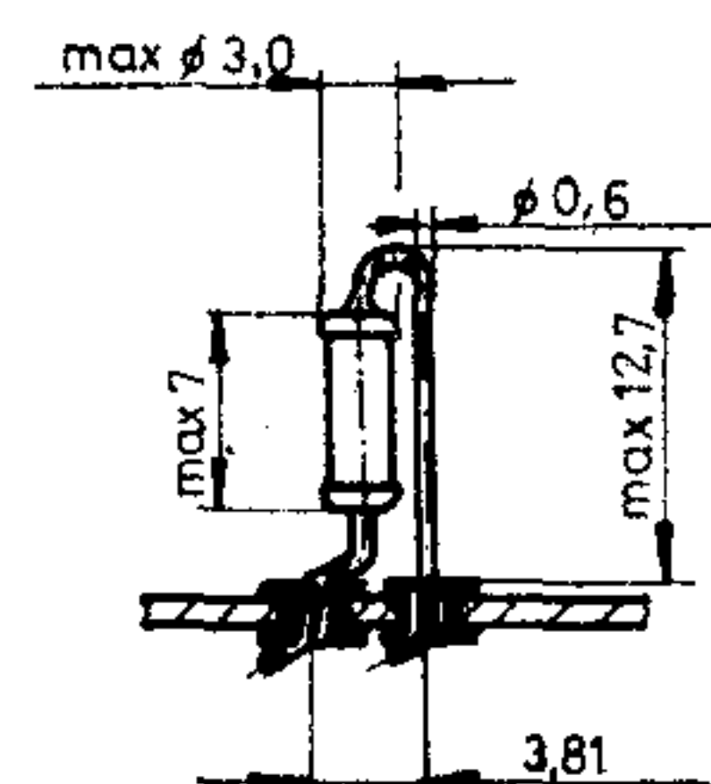
Álló helyzetben beültetett alkatrészek konstrukciója
