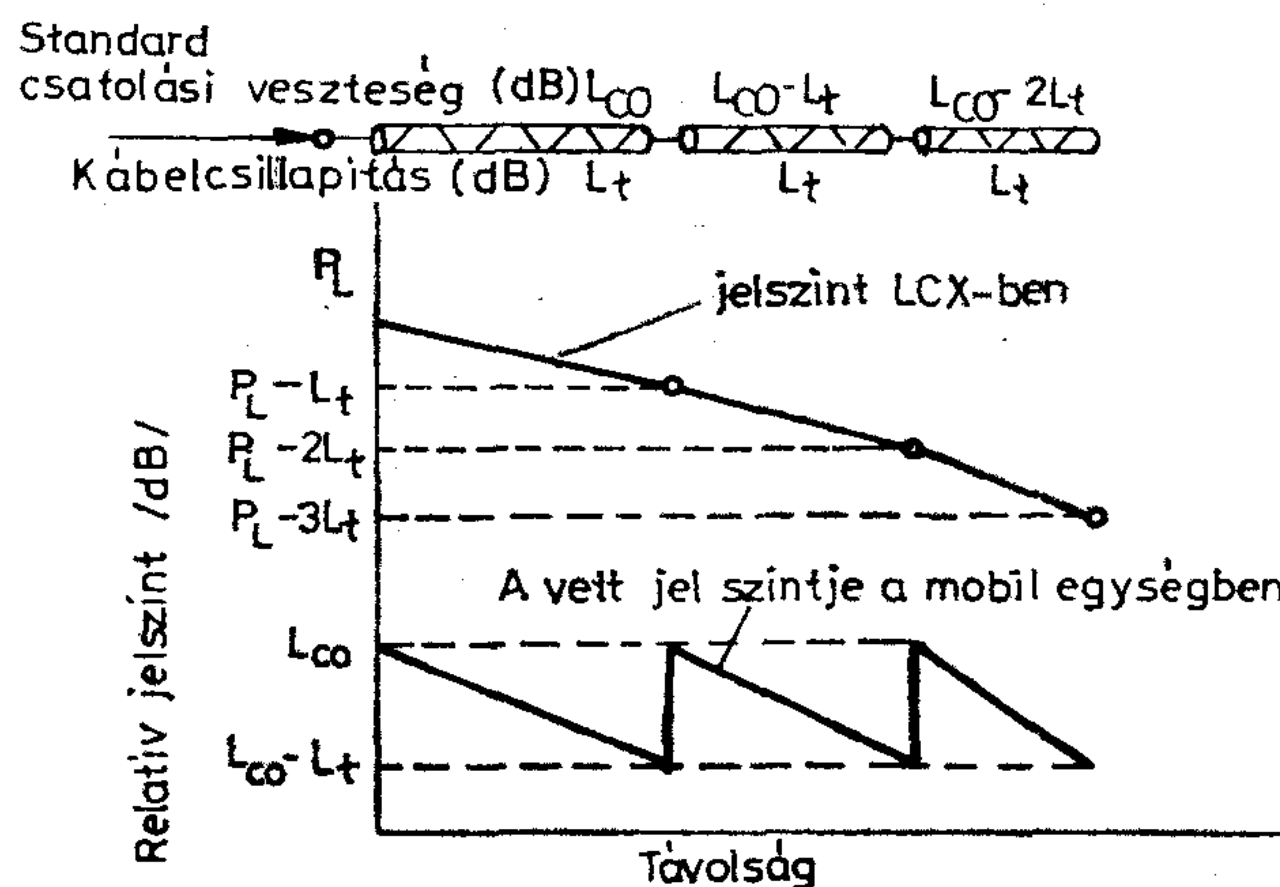
3. ábra. Lépcsőzöses technika LCX-ben
