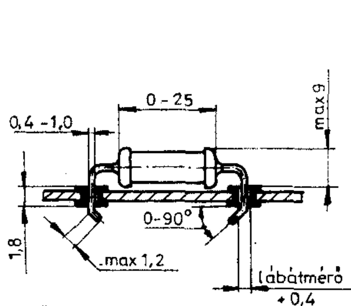
Fekvő helyzetben beültetett alkatrészek konstrukciója
