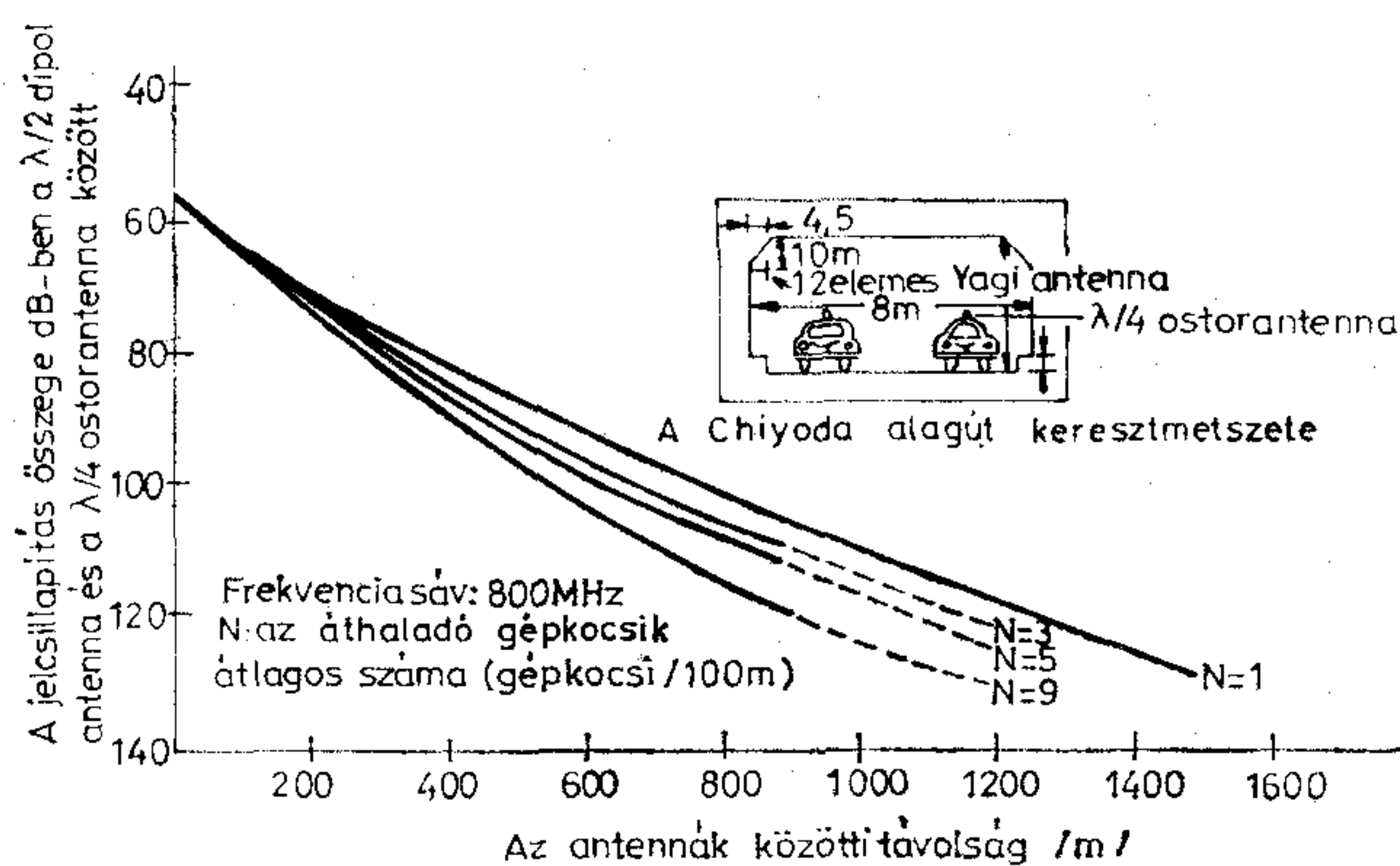
2. ábra. RF hullámterjedés csillapítási karakterisztikái egyenes alagútban
