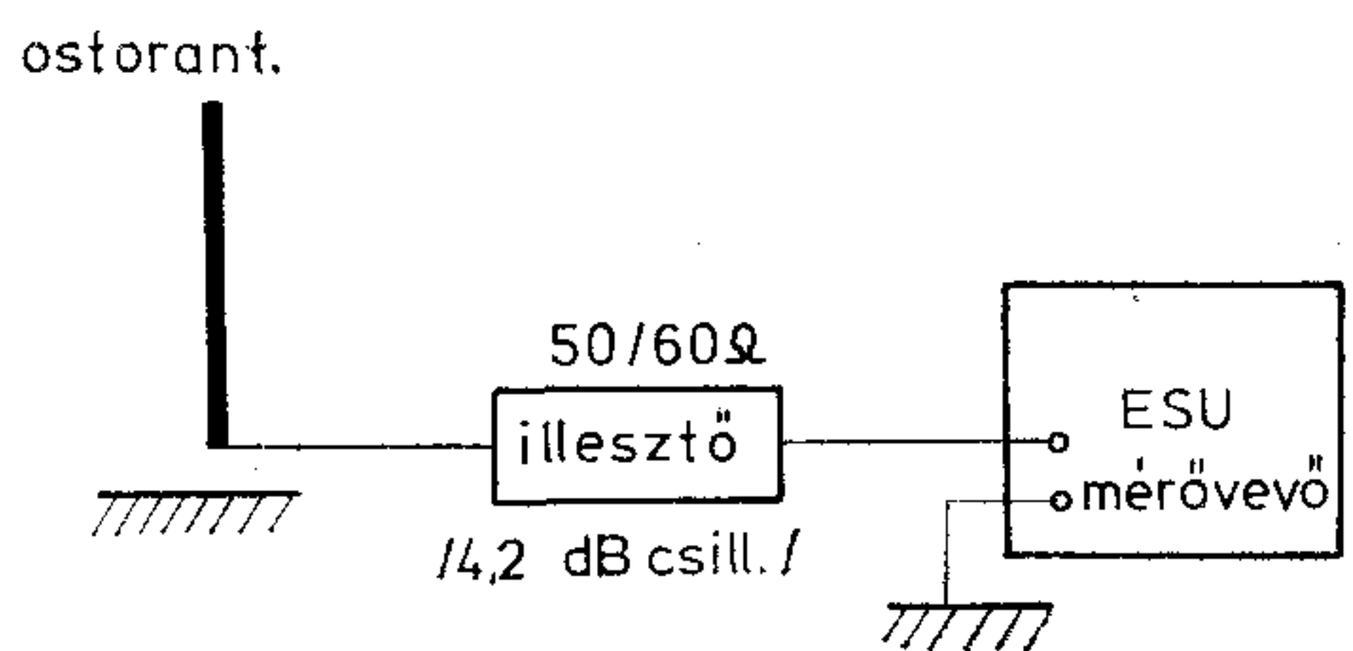
Zajmérés / 80 és 450 MHz / elrendezése
