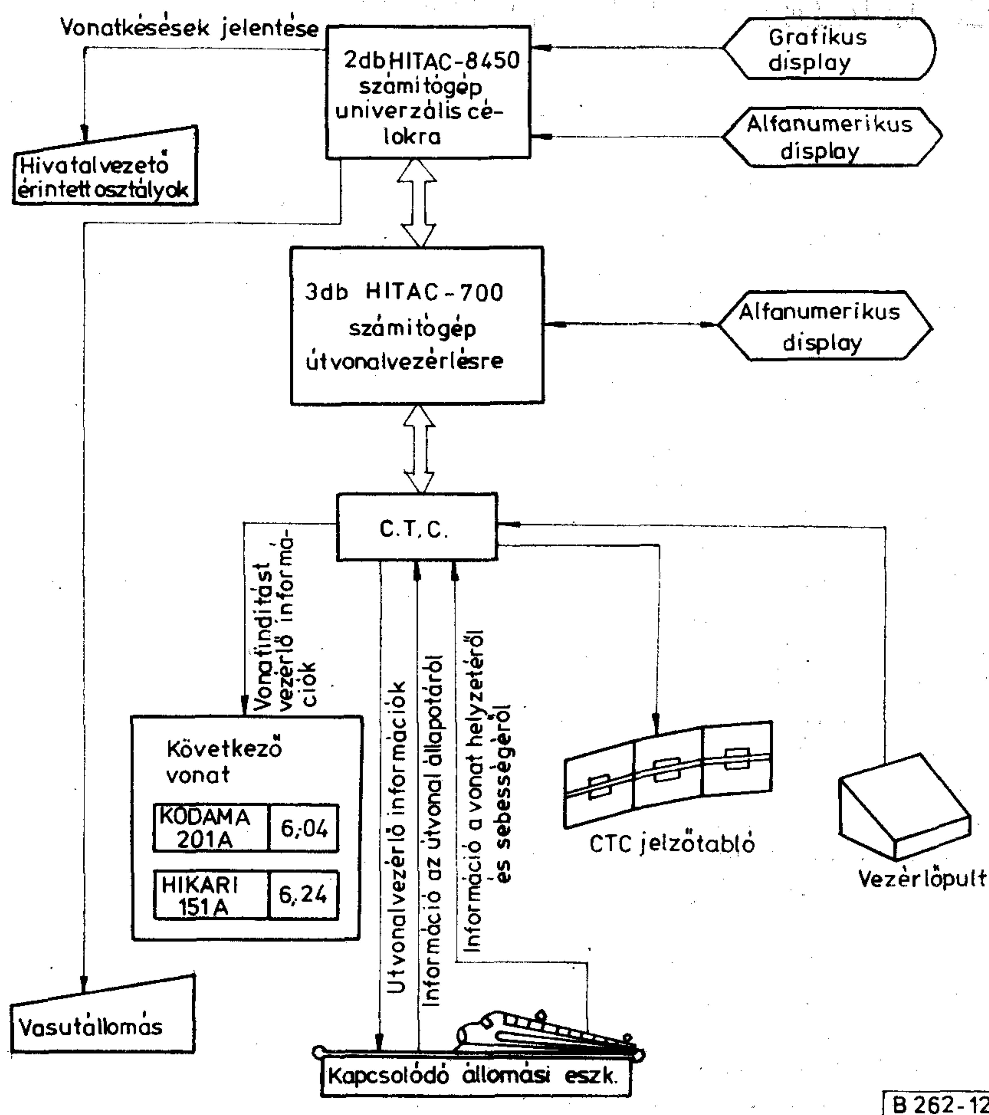
12. ábra. A COMTRAC blokkképlete
