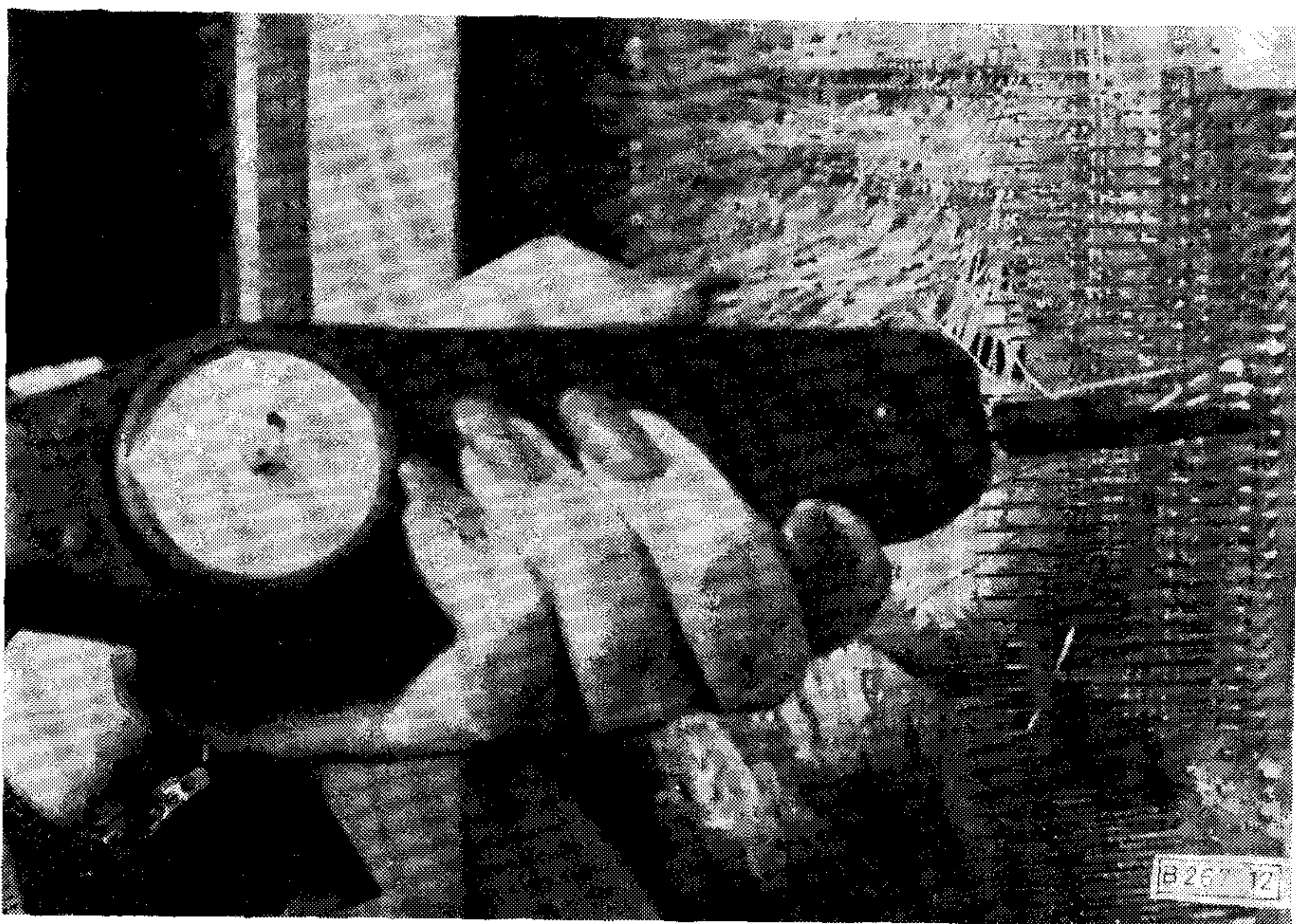
12. ábra. Wire-wrap kötés műszeres vizsgálata
