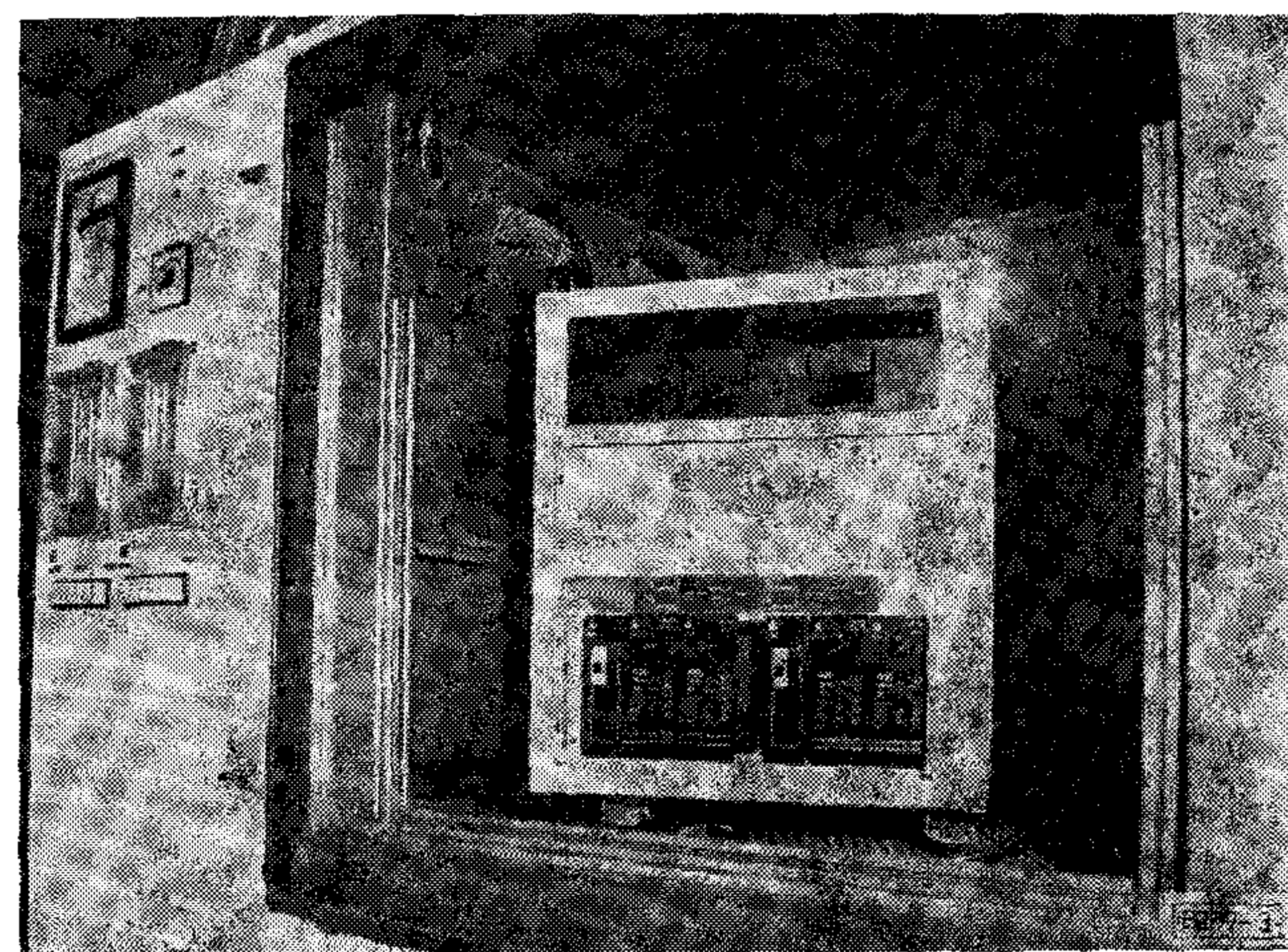
3. ábra. Kompletten szerelt részegység klímavizsgálata
