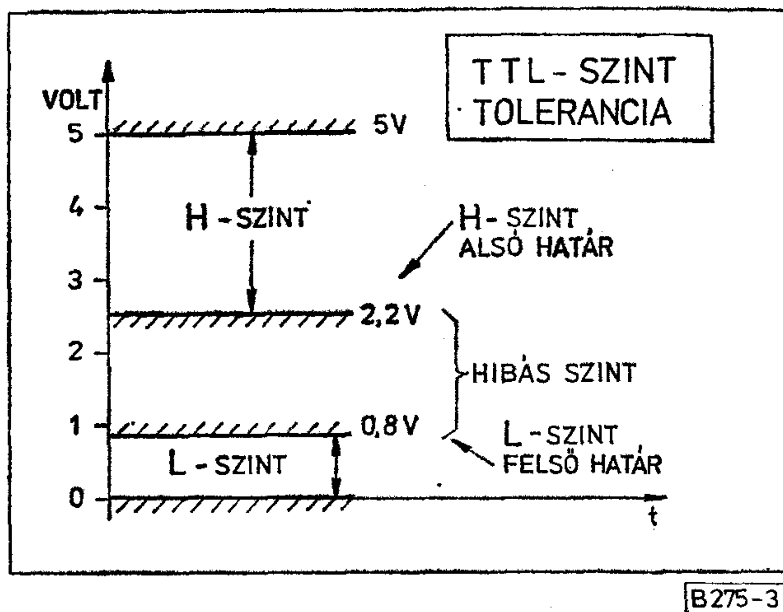
3. ábra. A TTL digitális áramkörök vezérlő jelének toleranciahatárai az L és a H szinten
