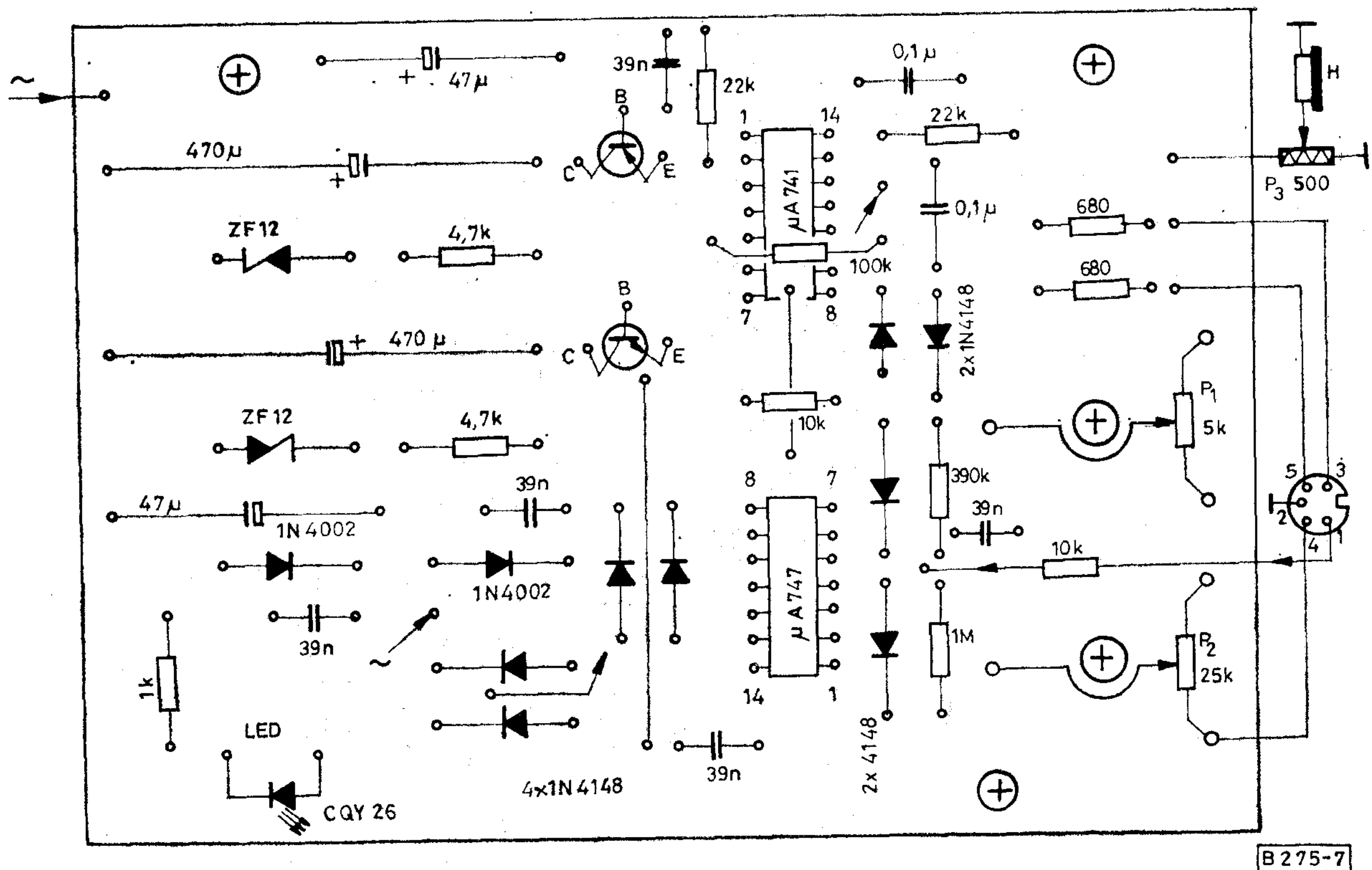
7. ábra. Az alkatrészek beültetése
