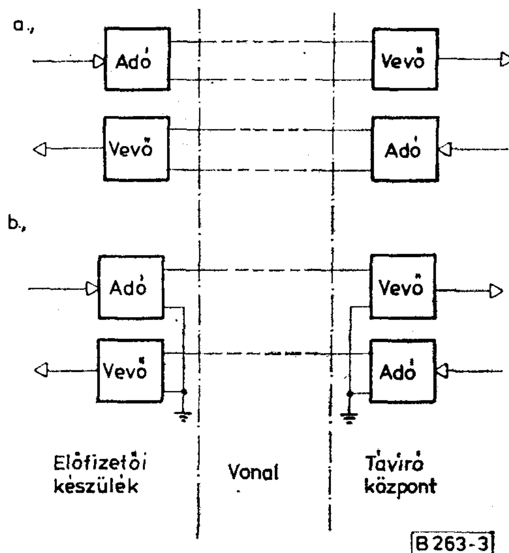
3. ábra. Előfizetői készülék csatlakoztatása kettős áramú távíróvonalhoz
