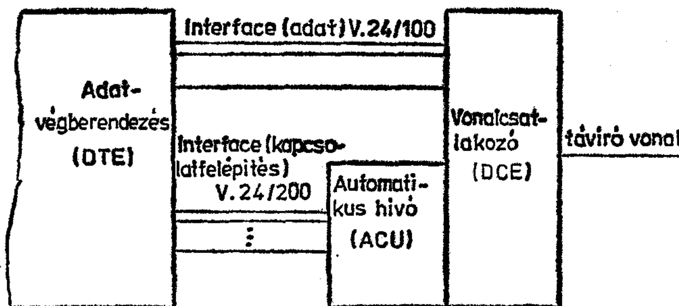
8. ábra. Csatlakoztatási elrendezés automatikus kapcsolatfelépítés esetén
