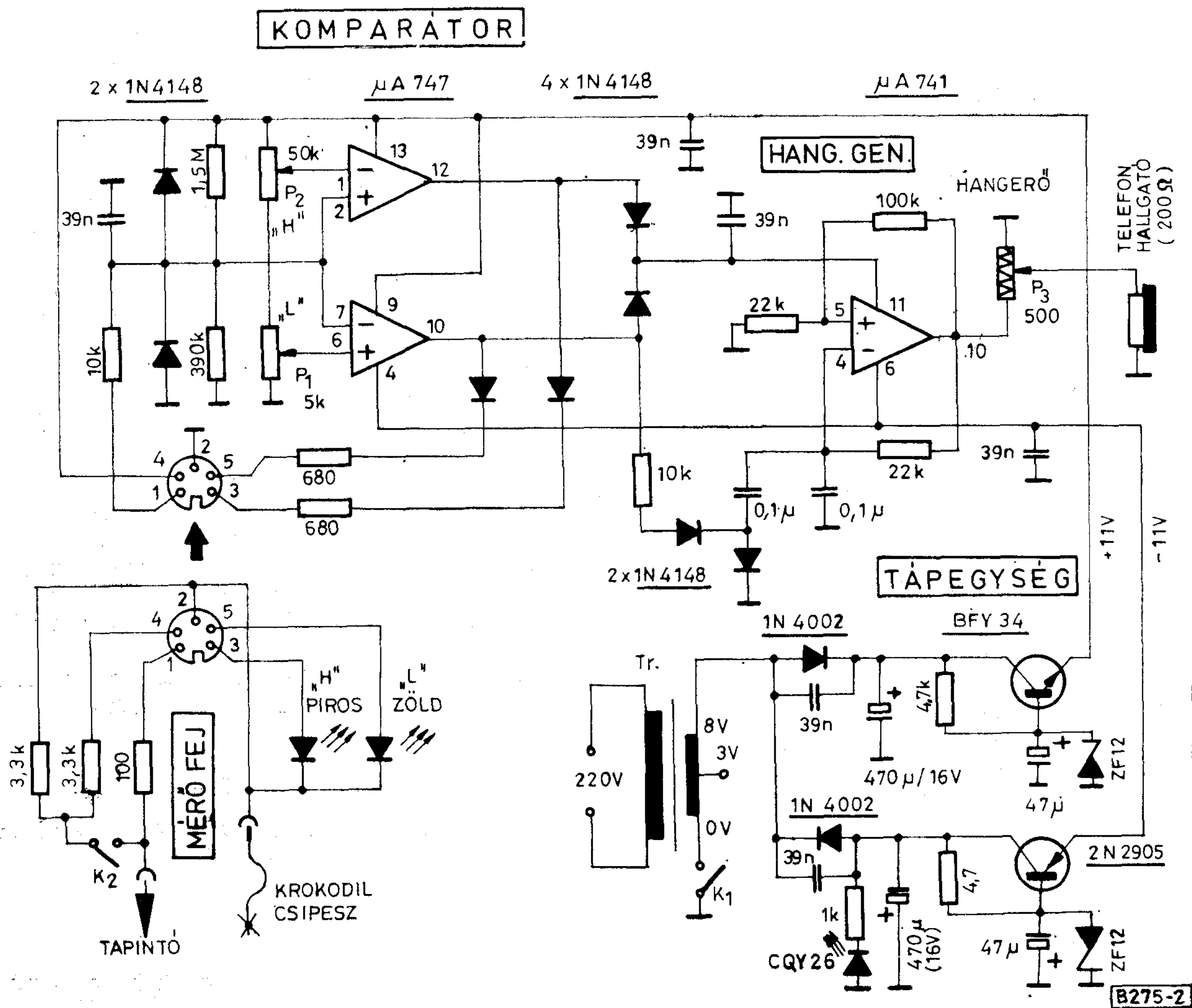
2. ábra. Az akusztikus digi-tester elektromos kapcsolási rajza
